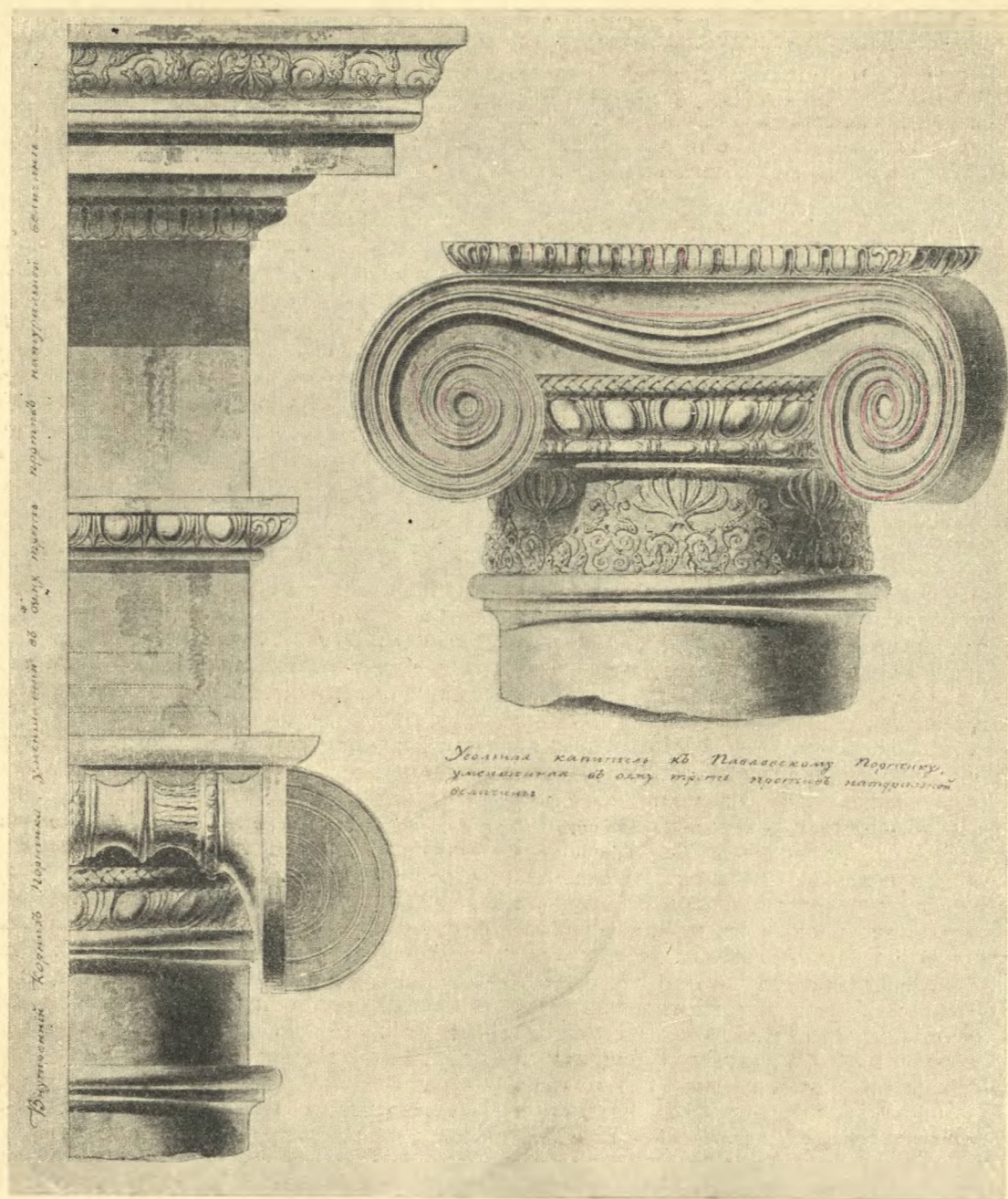
30. Чертеж угловой ионической капители к павильону «Трёх граций» в Павловске. Тушь и акварель. Из собрания Павловского дворца-музея
