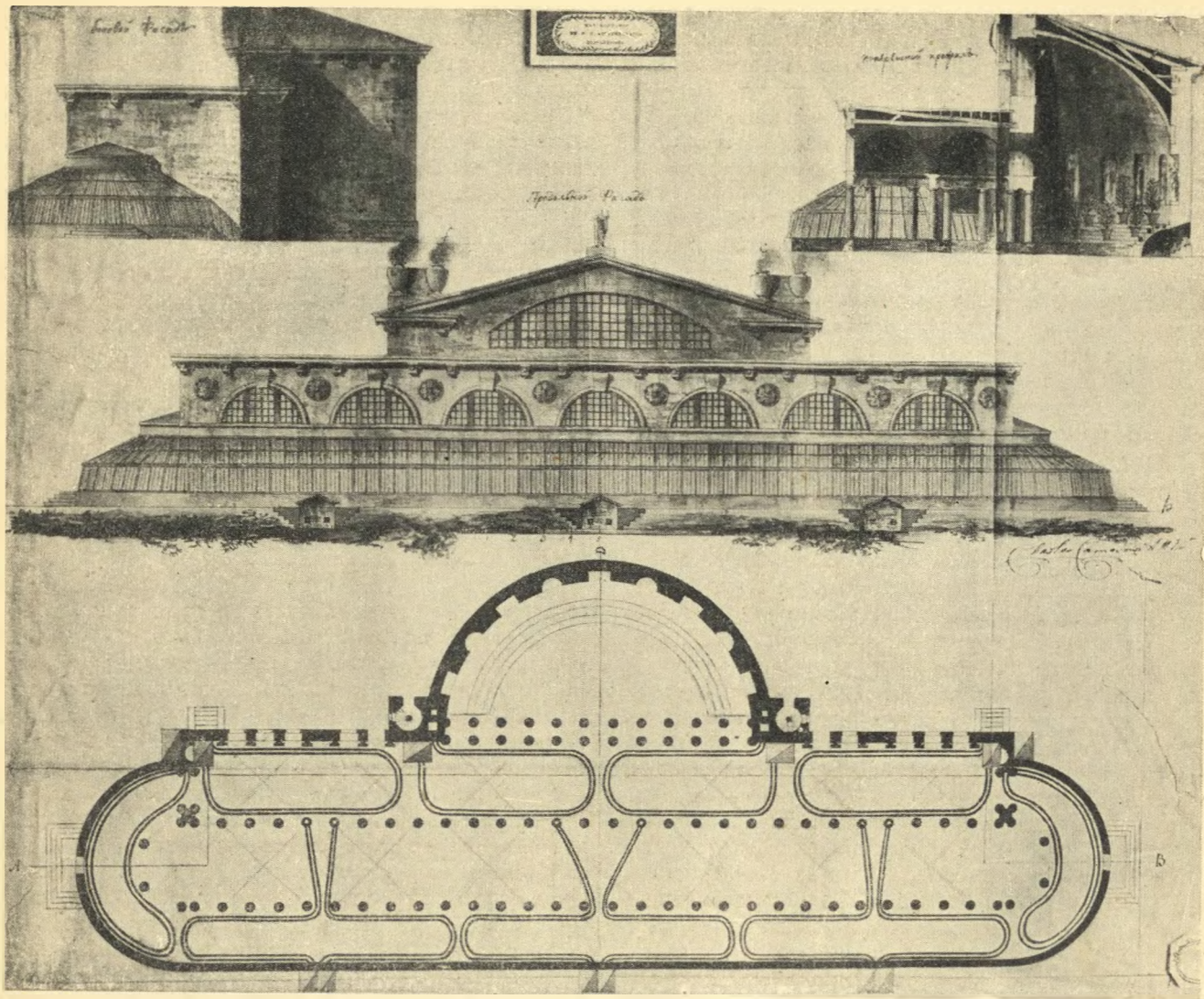
34. Проект оранжереи. Тушь. Из собрания Музея города
