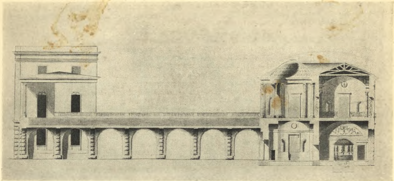
58. Термы Камерона. Разрез через площадку «Висячего сада» и здание «Холодных бань». Из собрания Гос. Эрмитажа
