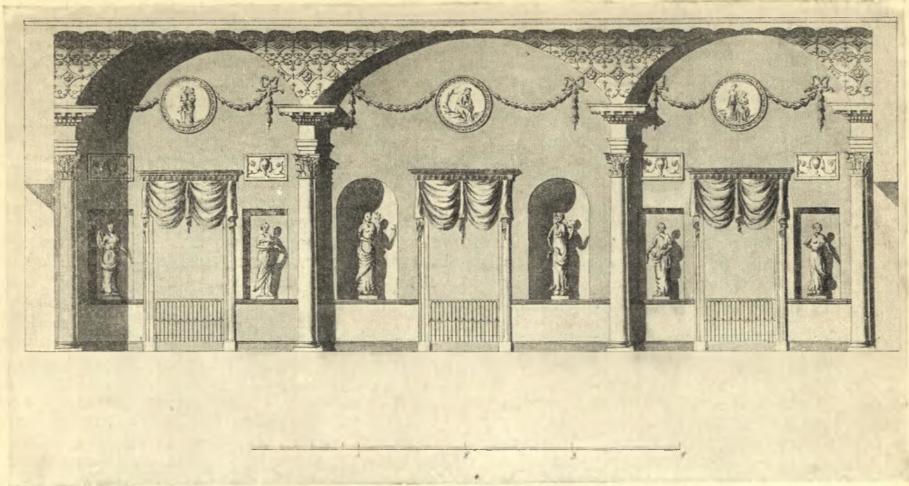
73. Термы Камерона. «Сферистерий». Продольный разрез. Неосуществленный вариант. Из собрания Гос. Эрмитажа
