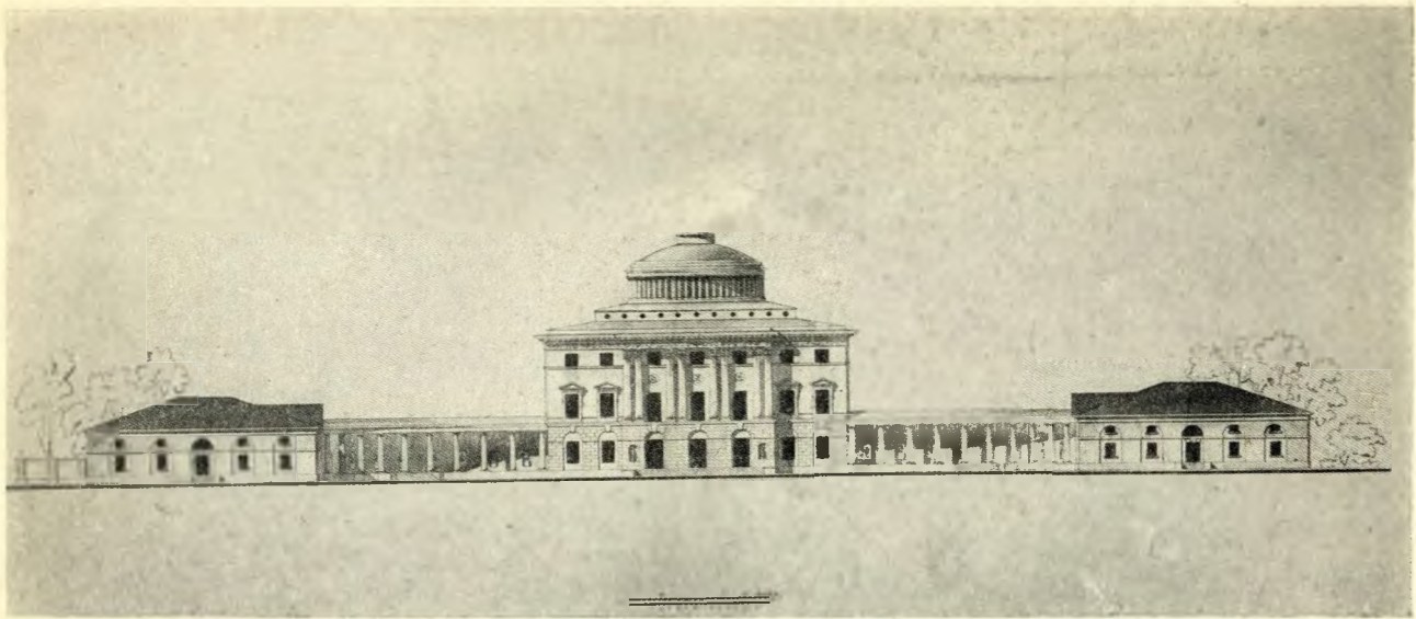
2. Павловский дворец. Фасад на р. Славянку (обмер и реконструкция архитекторов В. Н. Талепоровского и Ф. П. Милюковой, 1936)
