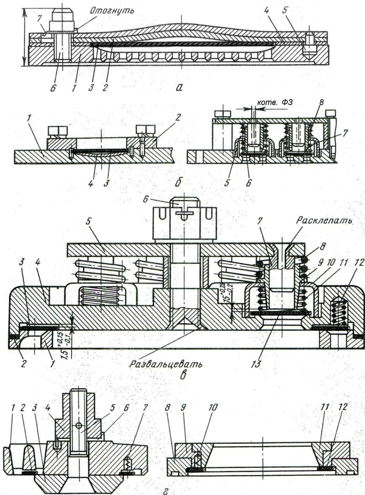
Рис. 135. Клапаны:
