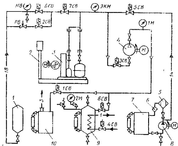
Рис. 167. Установка зарядки герметичных агрегатов:
