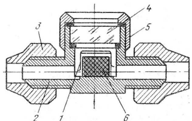
Рис. 73. Индикатор влажности: 1 — влагочувствительный элемент; 2 — корпус; 3, 5 — накидные гайки; 4 — смотровое стекло; 6 — капроновый вкладыш
