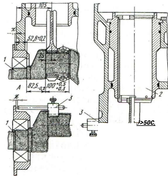
Рис. 150. Приспособление для определения толщины прокладки между фланцем корпуса подшипника и фланцем передней стенки картера:
