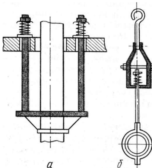
Рис. 37. Пружинные опоры для трубопроводов: а — вертикальных; б — горизонтальных
