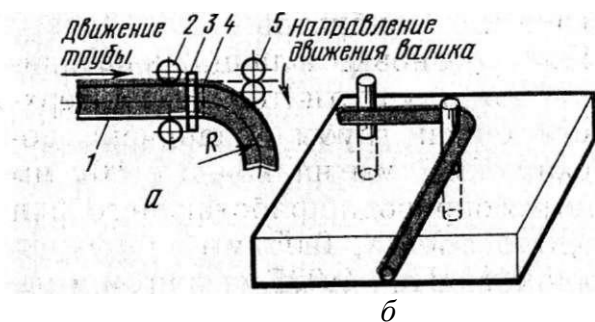
Рис. 46. Схема гнутья труб в горячем состоянии:
