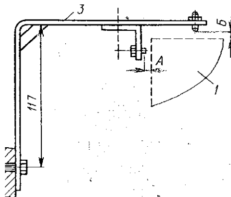
Рис. 17. Приспособление для проверки соосности валов с эластичной муфтой:
