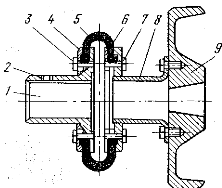
Рис. 16. Эластичная муфта:
