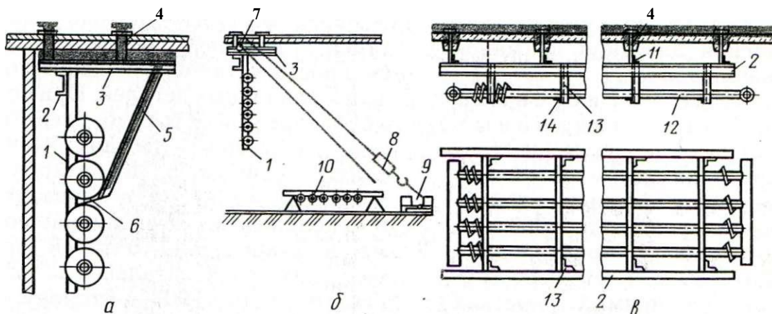
Рис. 26. Монтаж пристенной и потолочной батарей:
