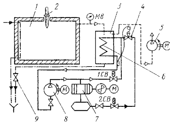
Рис. 172. Схема установки вакуумтермической регенерации адсорбентов и фильтров осушителей:
