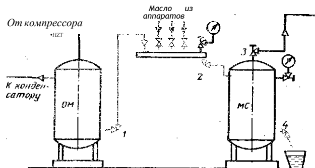
Рис. 69. Схема включения маслособиранителя: ОМ — маслоотделитель; МС — маслособиранитель; /4-4 — вентили
