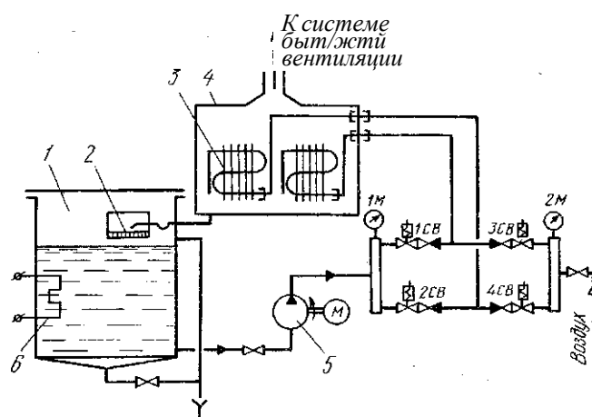
Рис. 171. Схема установки для промывки ресиверно-конденсаторных групп:
