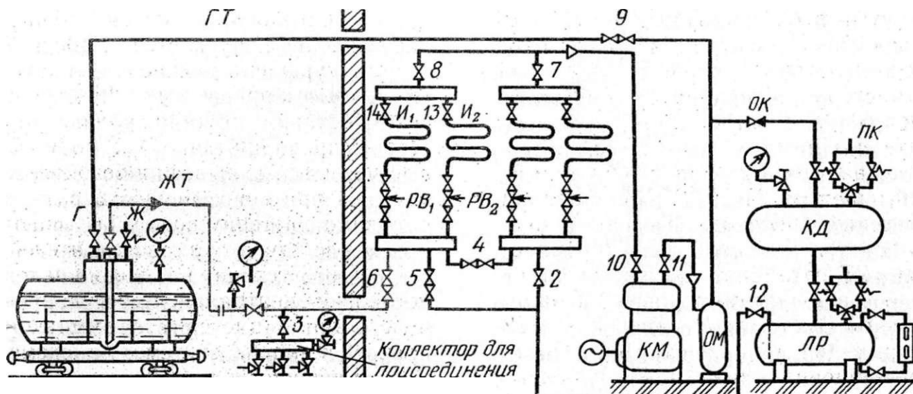
Рис. 56. Схема слива аммиака из цистерны:
