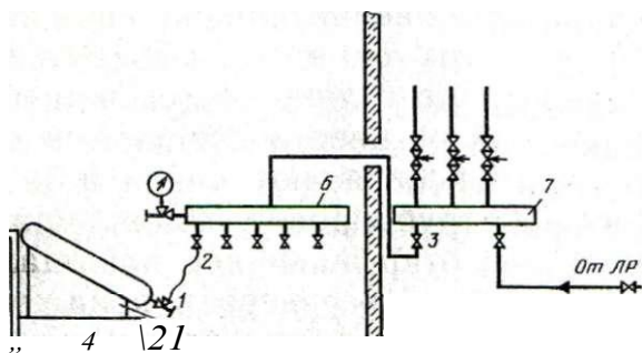
Рис. 58. Схема заправки системы аммиаком из баллонов:
