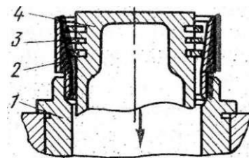
Рис. 151. Втулка с коническим отверстием для ввода поршня с кольцами в цилиндр:
