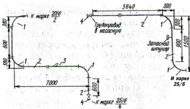
Рис. 43. Рабочие чертежи узлов трубопроводов
