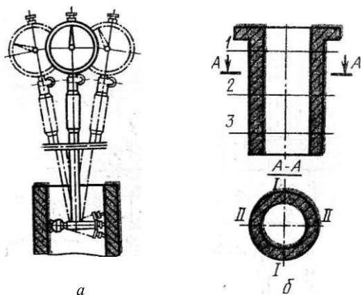
Рис. 105. Измерение диаметра цилиндра: — схема измерения индикаторным нутромером; б — схема измерения диаметра цилиндра
