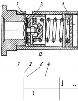
Рис. 153. Предохранительный клапан компрессора П110 и приспособления для его регулировки:
