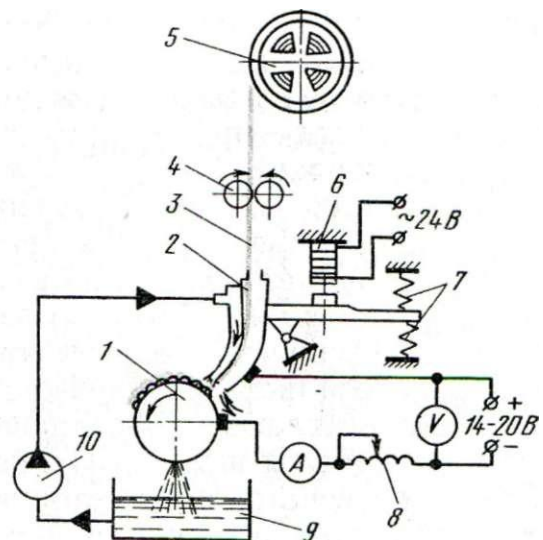
Рис. 87. Схема установки для вибродуговой наплавки:
