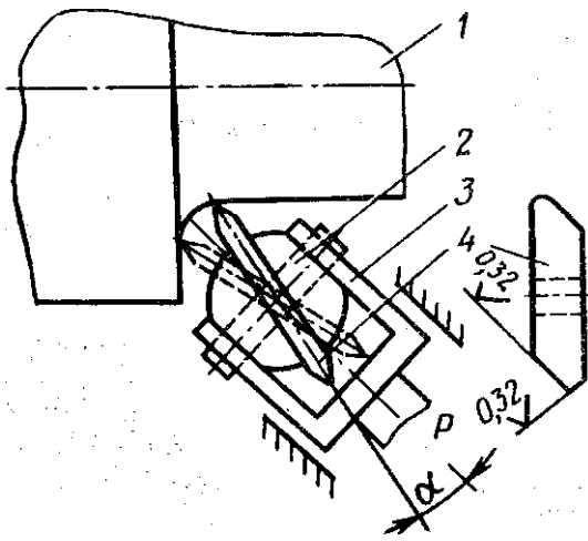
Рис. 86. Приспособление для обкатки галтелей шатунной шейки коленчатого вала: 1 — коленчатый вал; 2 — ось; 3 — вилка; 4 — ролик
