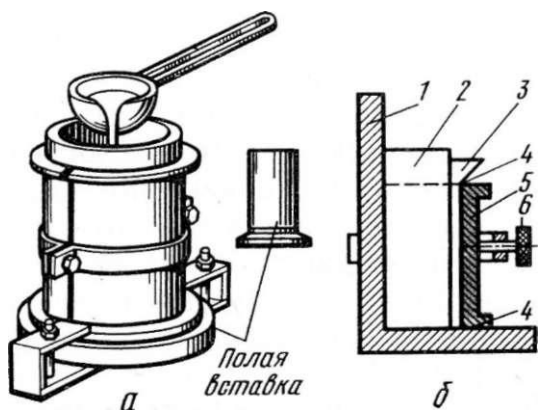
Рис. 123. Приспособление для ручной заливки баббитом:
