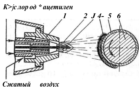
Рис. 88. Схема газопламенной металлизации напылением:
