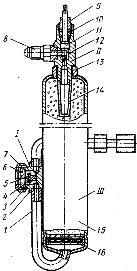
Рис. 168. Узел для обкатки герметичного агрегата:
