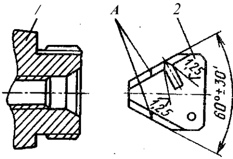
Рис. 133. Проверка центровых отверстий коленчатого вала:
