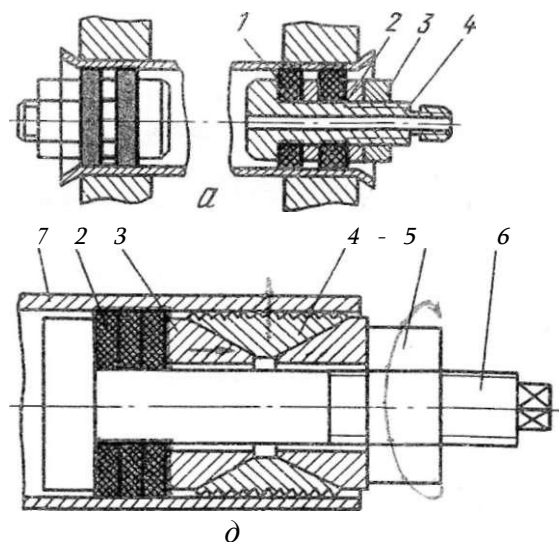
Рис. 161. Пробки:
