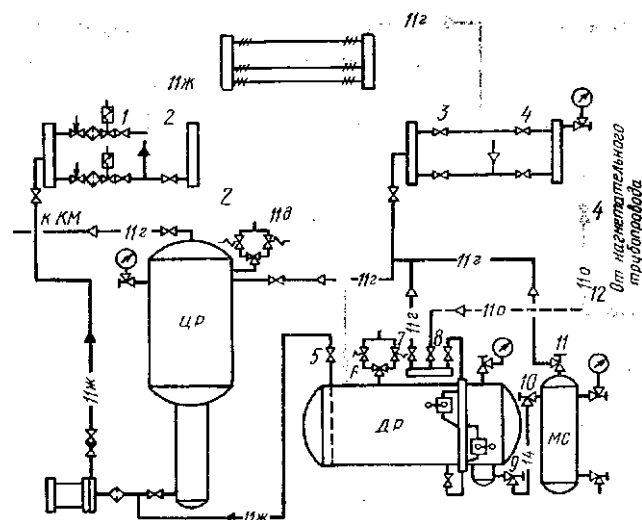
Рис. 66. Оттаивание батарей горячими парами аммиака:
