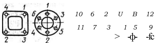
Рис. 99. Последовательность заворачивания гаек при креплении крышек и фланцев
