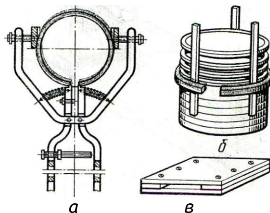
Рис. 115. Приспособления для замены и проверки поршневых колец: а — клещи для снятия и установки колец; б — пластины для снятия и установки колец; в — щелевой калибр
