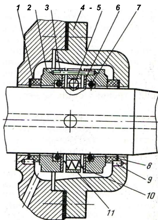
Рис. 138. Сальник компрессора 1180:
