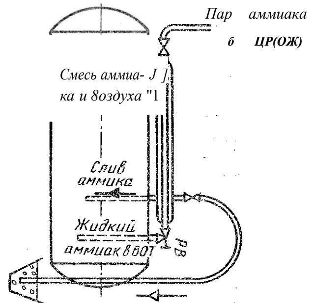
Рис. 72. Схема включения воздухоотделителя типа «труба в трубе»
