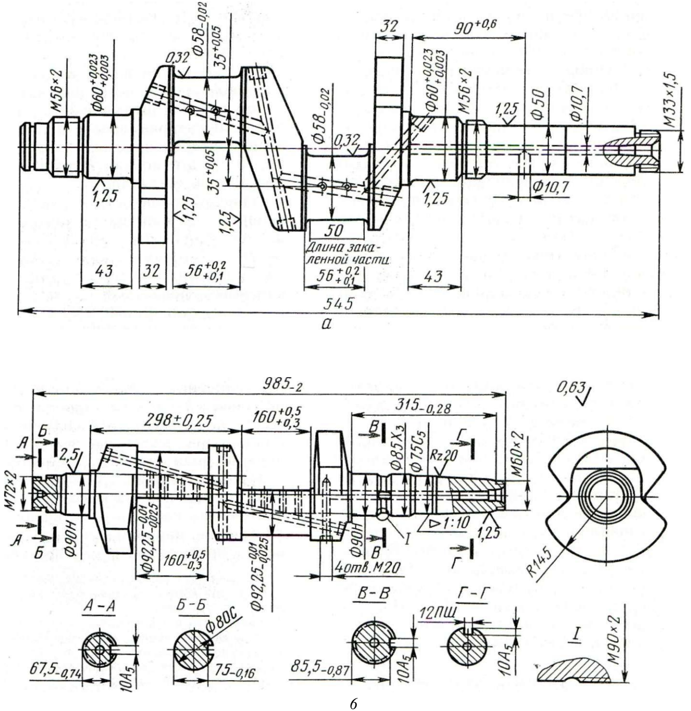
Рис. 129. Коленчатые валы: а — компрессора АУ45; б — компрессора П220
