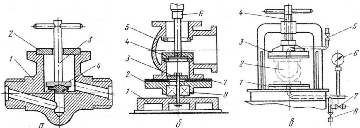
Рис. 165. Приспособления для ремонта и испытания арматуры:
