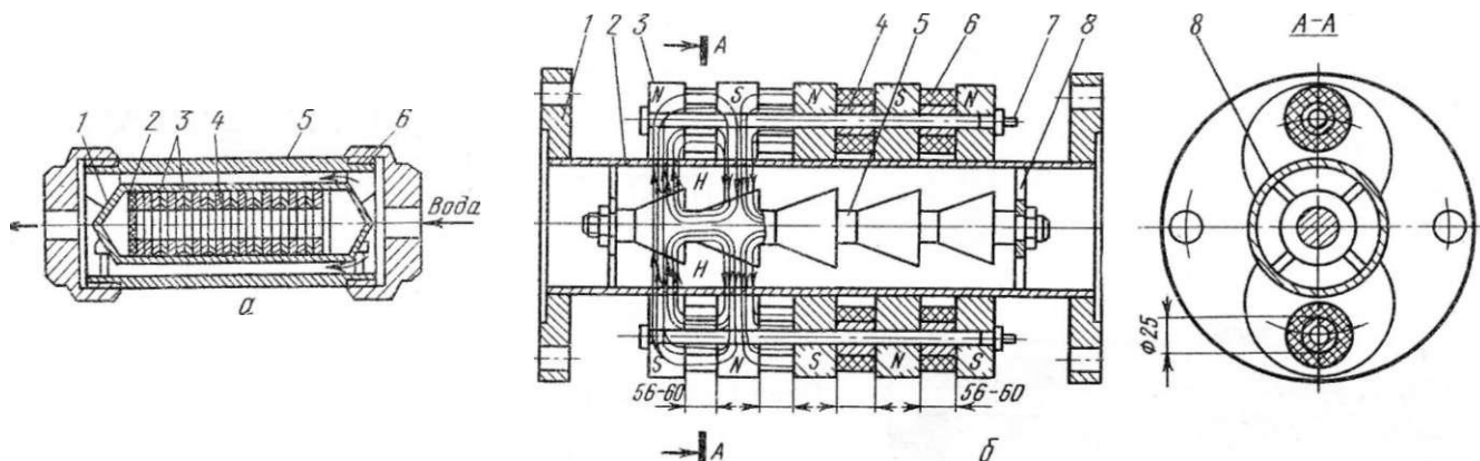
Рис. 160. Устройства для магнитной обработки воды:
