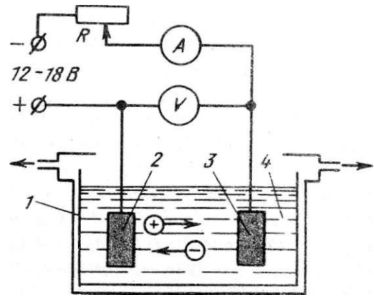
Рис. 90. Схема установки для электролитического осаждения металла:
