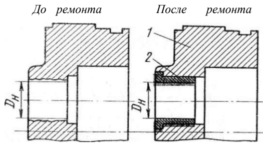
Рис. 84. Схема восстановления размера отверстия в корпусе масляного насоса: 1 — корпус масляного насоса; 2 — ремонтная деталь (втулка)
