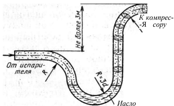
Рис. 11. Маслоподъемная петля
