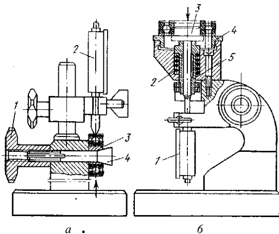
Рис. 126. Приспособления для измерения зазоров в подшипниках качения:
