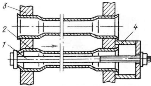
Рис. 162. Приспособление для удаления труб из трубной решетки:
