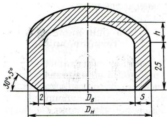
Рис. 35. Заглушка стальная сферическая
