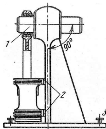
Рис. 143. Приспособление для проверки перпендикулярности оси нижней головки шатуна к образующей поршня:
