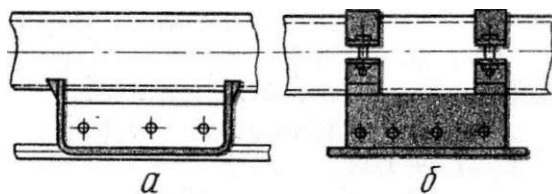
Рис. 36. Скользящие опоры: а — с приварным ползуном; б — с хомутами
