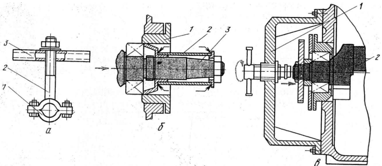
Рис. 149. Приспособления, используемые при установке коленчатого вала:
