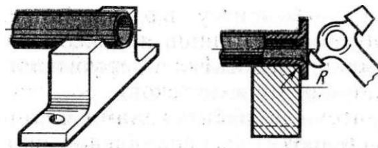
Рис. 47. Схема бортовки труб вручную на оправке
