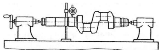
Рис. 134. Измерение величины биения коленчатого вала
