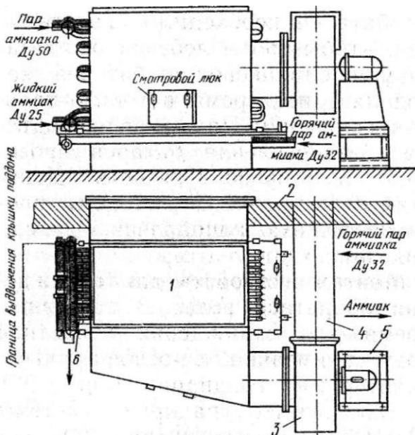
Рис. 23. Схема монтажа напольного воздухоохлаждителя:
