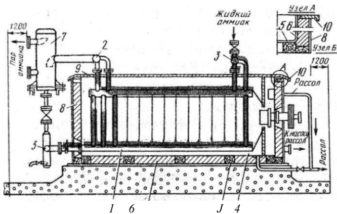
Рис. 22. Схема расположения рассольного панельного испарителя:
