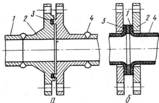
Рис. 30. Фланцевые соединения:
