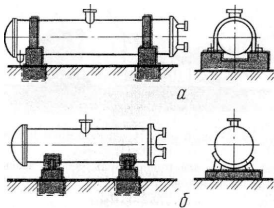
Рис. 20. Схема расположения горизонтальных аппаратов: a — без опорных лап; б — на опорных лапах
