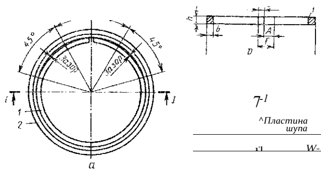
Рис. 113. Проверка поршневых колец:
