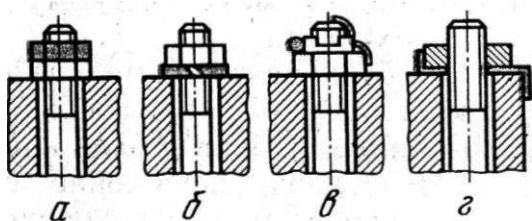
Рис. 100. Предохранение гаек от самоотвинчивания:
