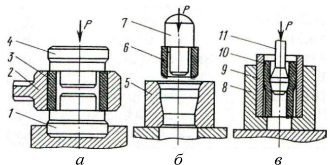
Рис. 85. Схема изменения размеров деталей пластической деформацией:
