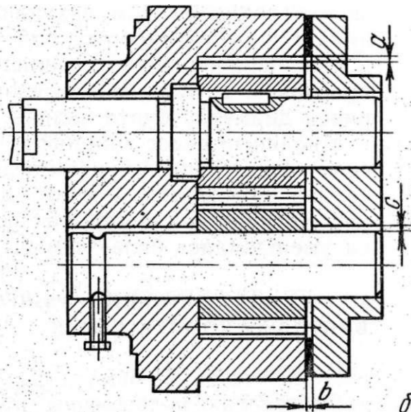
Рис. 139. Шестеренчатые масляные насосы:
