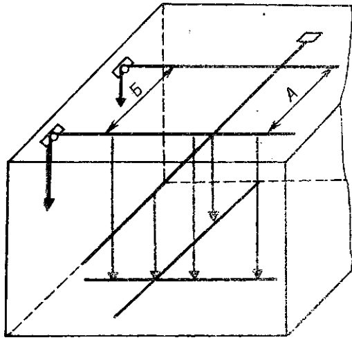
Рис. 8. Схема проверки монтажных осей
