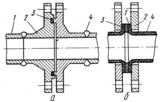
Рис. 30. Фланцевые соединения:
