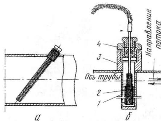
Рис. 54. Монтаж чувствительного элемента реле температуры:
