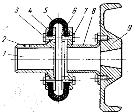
Рис. 16. Эластичная муфта:
