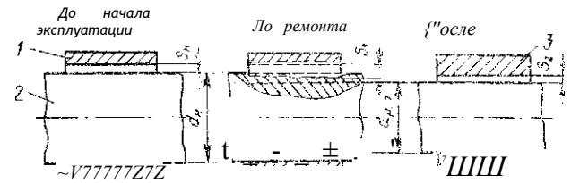
Рис. 83. Схема восстановления зазора в сопряжении шейки вала — подшипник скольжения способом ремонтных размеров:
