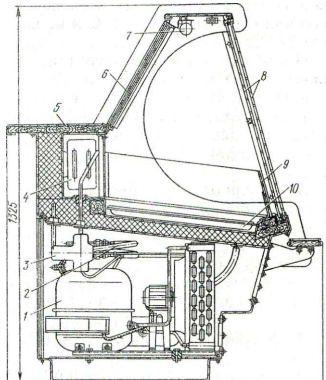
Рис. 9. Разрез прилавка-витрины «Пингвин-В»:
