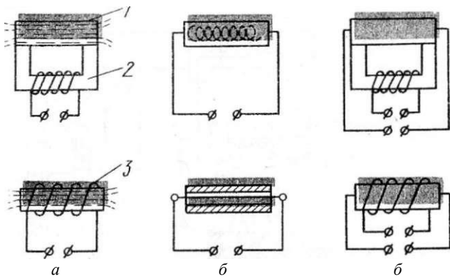
Рис. 96. Схема намагничивания деталей: а — продольное намагничивание; б — циркулярное намагничивание; в — комбинированное намагничивание; 1 — деталь; 2 — электромагнит; 3 — соленоид
