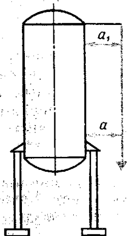
Рис. 13. Проверка оборудования на вертикальность
