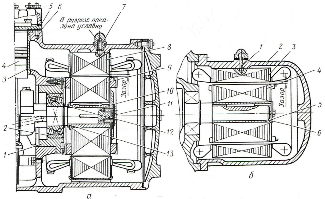
Рис. 154. Бессальниковые компрессоры (сборка):
