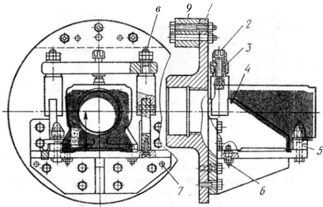
Рис. 102. Приспособление для растачивания отверстия в картере:
