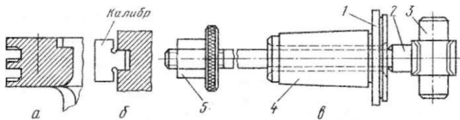
Рис. 110. Проверка выработки поршневых канавок и приспособление для ремонта:
