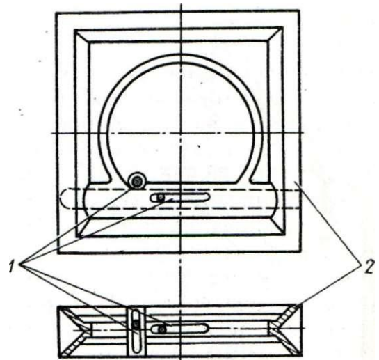
Рис. 6. Монтажно-ремонтный уровень: 1 — ампула; 2 — корпус
