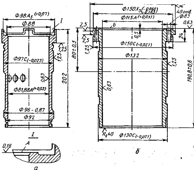
Рис. 103. Гильзы компрессоров: а — прямооточного компрессора АУ-45; б — непрямоточного компрессора П110
