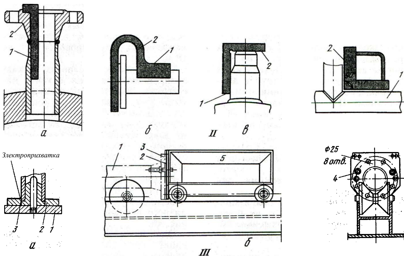
Рис. 48. Приспособления:
