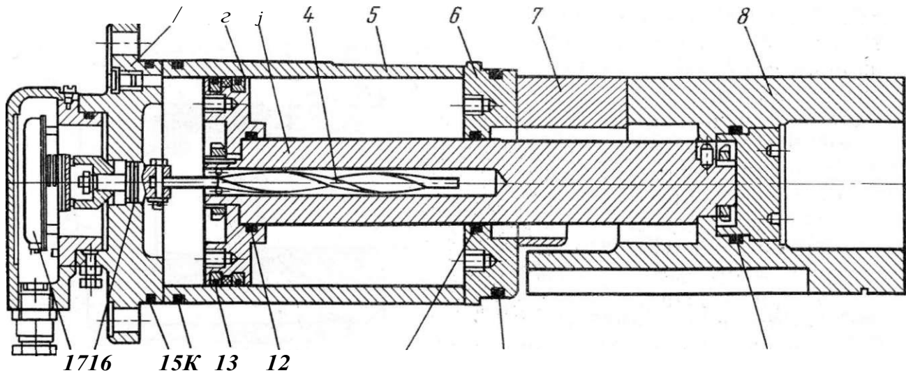
Рис. 141. Регулятор производительности компрессора S3-900:
