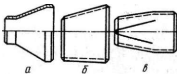
Рис. 34. Переходы а — штампованный симметричный; б — штампованный несимметричный; в — сварной из трубы; г — сварной из листа, симметричный; д — обсадной из трубы, симметричный
