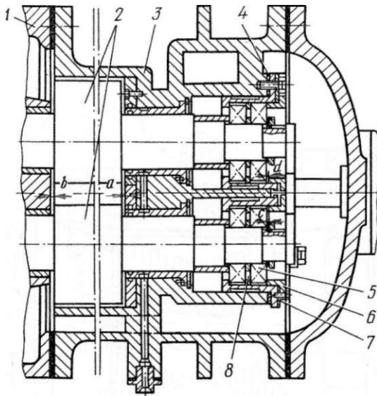
Рис. 156. Винтовой компрессор 5ВХ-350/2,6 (сборка):
