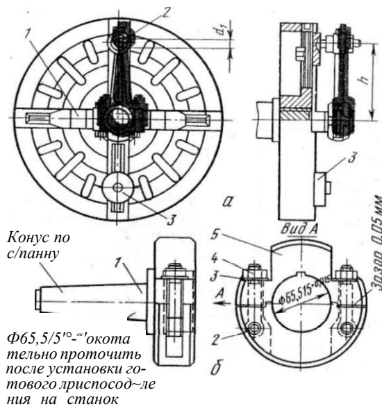
Рис. 125. Приспособления для обработки баббитовой заливки подшипников:
