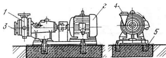
Рис. 19. Общий вид центробежного насоса на раме:
