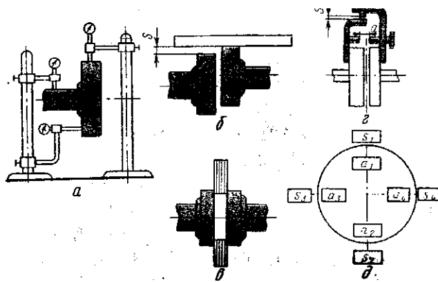
Рис. 14. Схема проверки положения машин при муфтовом сцеплении:
