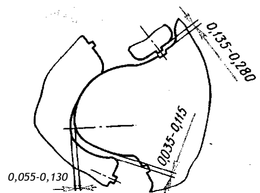
Рис. 155. Схема измерения зазоров между зубьями роторов
