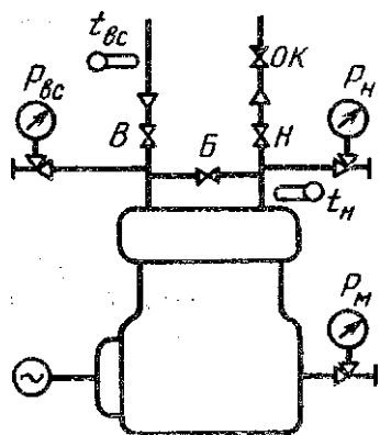
Рис. 61. Компрессор с ручным байпасом
