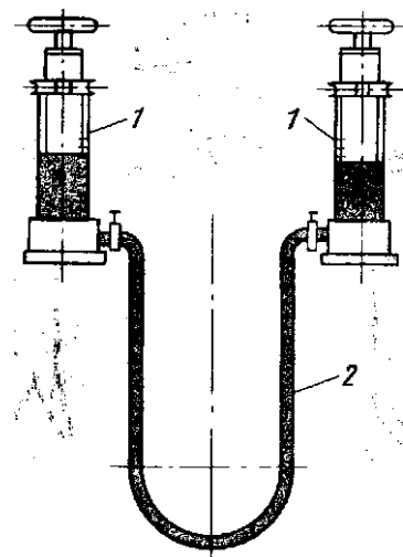
Рис. 7. Гидростатический уровень: 1 — градуированный стеклянный цилиндр; 2 — резиновая трубка
