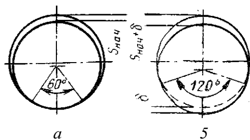
Рис. 121. Схема расположения вала и подшипника скольжения: а — до износа; б — после износа
