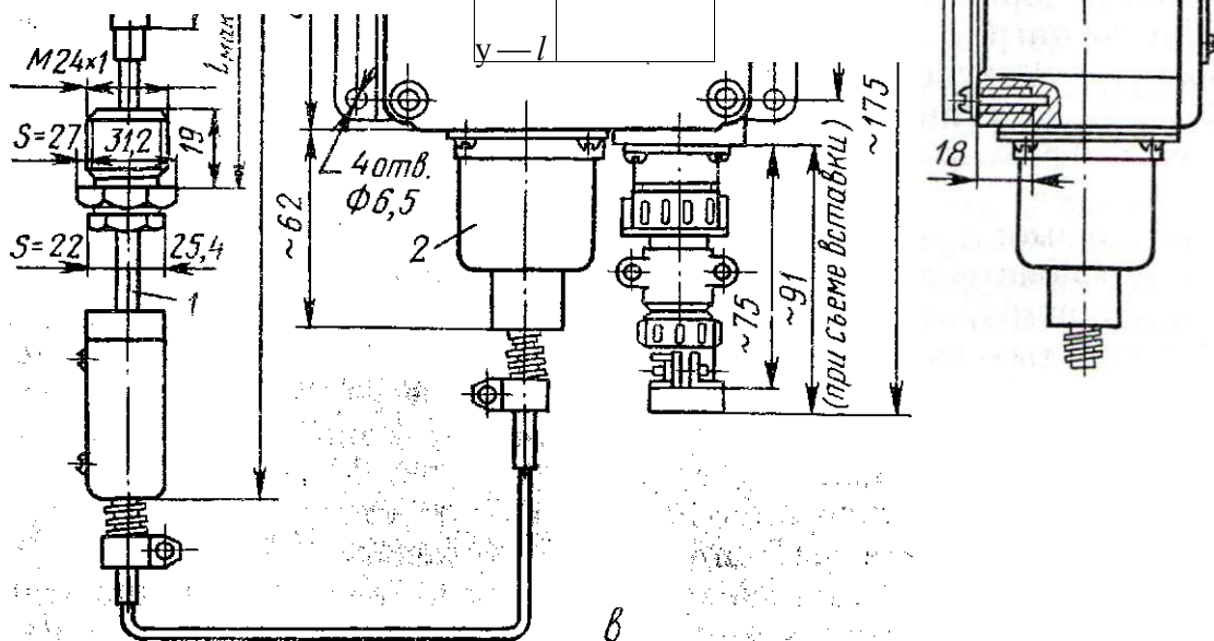
Рис. 53. Реле температуры:
