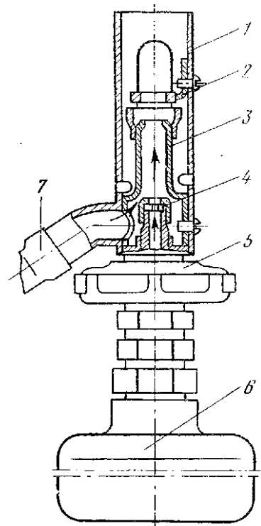
Рис. 74. Пропановая галоидная лампа: 1 — корпус горелки; 2 — красно-медная насадка; 3 — инжектор; 4 — сопло; 5 — маховик вентиля; 6 — баллон; 7 — шланг
