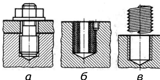
Рис. 101. Ремонт резьбового соединения: а—постановкой ступенчатой шпильки; б—постановкой переходной втулки; в—постановкой резьбовой спиральной вставки
