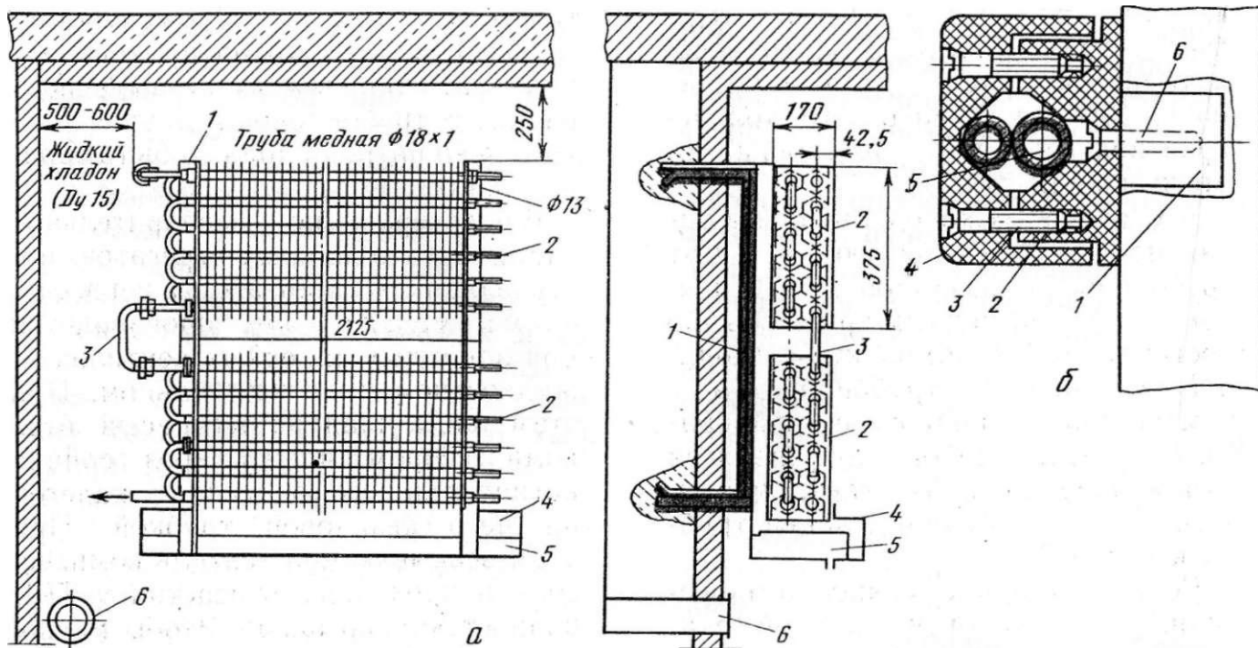
Рис. 10. Схема монтажа хладоновых батарей и трубопроводов:
