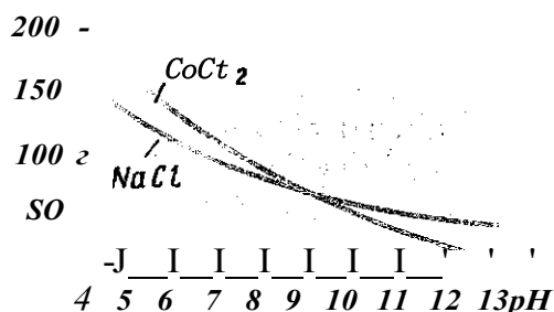
Рис. 79. Относительная скорость коррозии r в зависимости от кислотности и щелочности рассола
