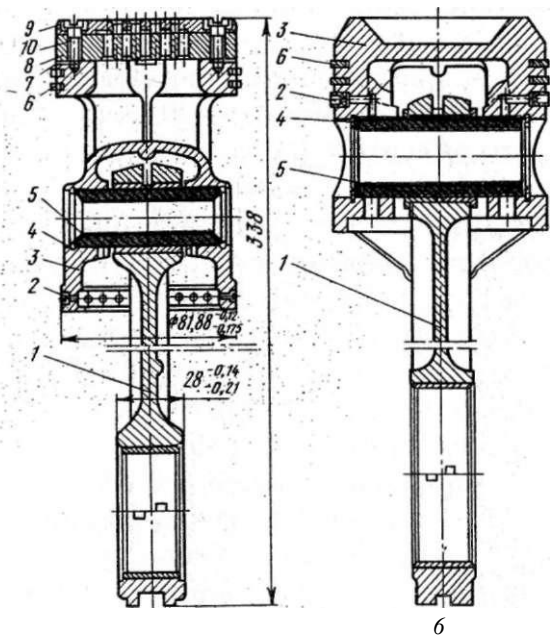
Рис. 142. Шатунно-поршневые группы:
