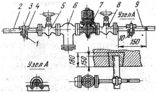
Рис. 55. Узел монтажа СВМ соленоидного вентиля трубопровода:
