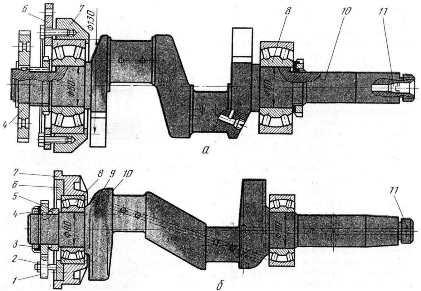
Рис. 144. Коленчатые валы в сборе:
