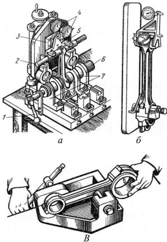
Рис. 119. Приспособления для проверки и правки шатуна:
