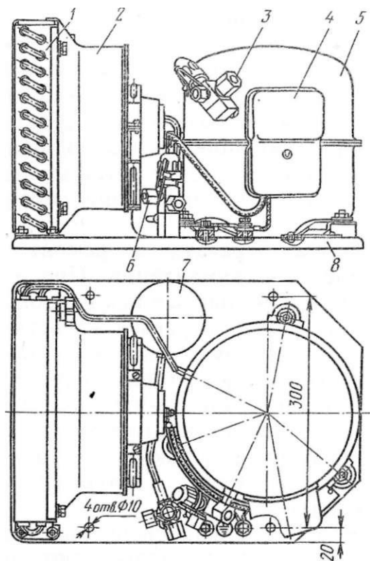
Рис. 166. Герметичный агрегат ВС:
