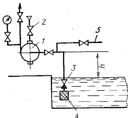
Рис. 65. Схема установки насоса выше уровня жидкости: 1 — насос; 2 — заливная воронка; 3 — обратный клапан; 4 — фильтр; 5 — водопровод
