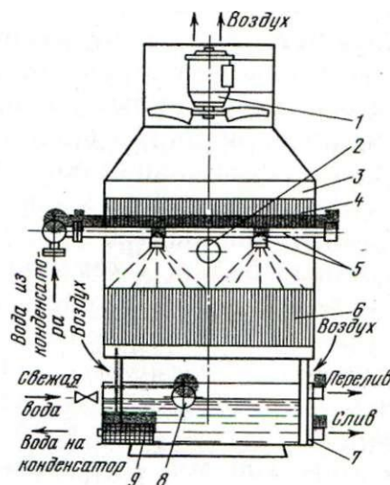
Рис. 28. Пленочная вентиляторная градирня типа ГПВ:
