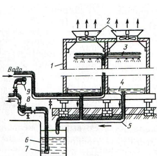
Рис. 27. Схема монтажа вентиляторной градирни:
