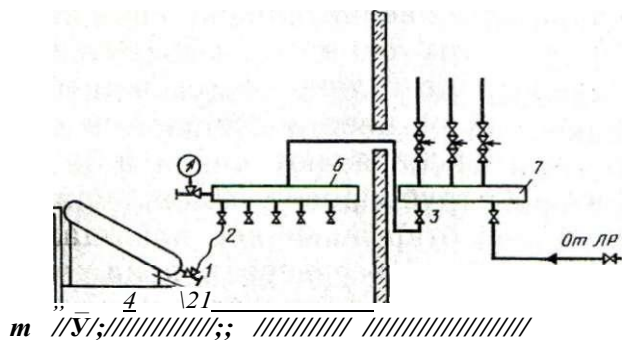
Рис. 58. Схема заправки системы аммиаком из баллонов:
