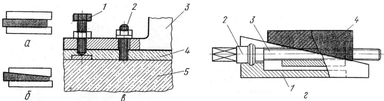
Рис. 12. Приспособления для выверки и регулировки положения оборудования:
