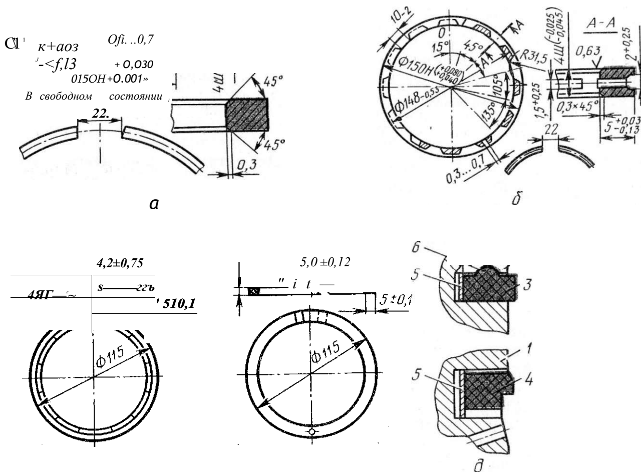
Рис. 112. Поршневые кольца:
