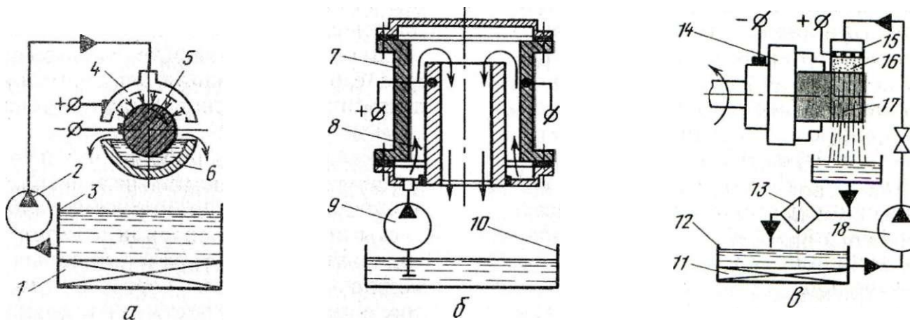
Рис. 91. Схемы вневанного электролитического осаждения металла:
