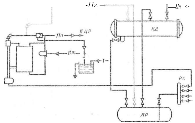
Рис. 71. Схема включения воздухоотделителя АВ-4
