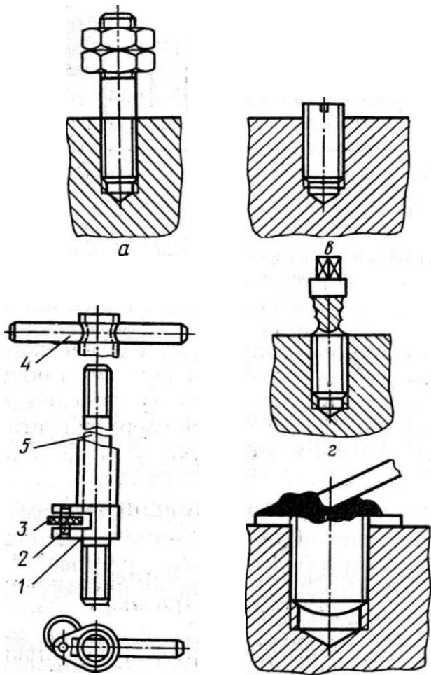
Рис. 98. Приемы вывертывания шпилек: a — с помощью двух гаек; б — эксцентриковым ключом; в — посредством шлица под отвертку; г — с помощью экстрактора; д — с помощью приваренного прутка; 1 — корпус; 2 — ось; 3 — рифленый ролик; 4 — вороток; 5 — шпилька
