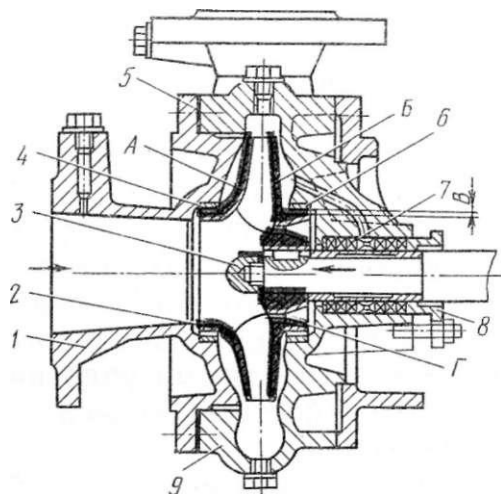
Рис. 158. Центробежный насос типа К:
