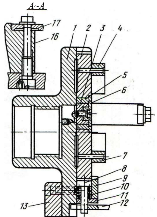
Рис. 106. Приспособление для растачивания блока цилиндров:
