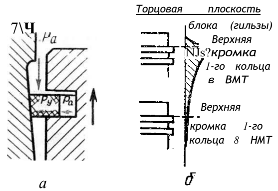
Рис. 104. Износ зеркала цилиндра:
