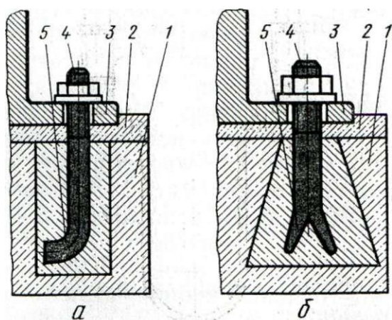
Рис. 3. Фундаментные болты:
