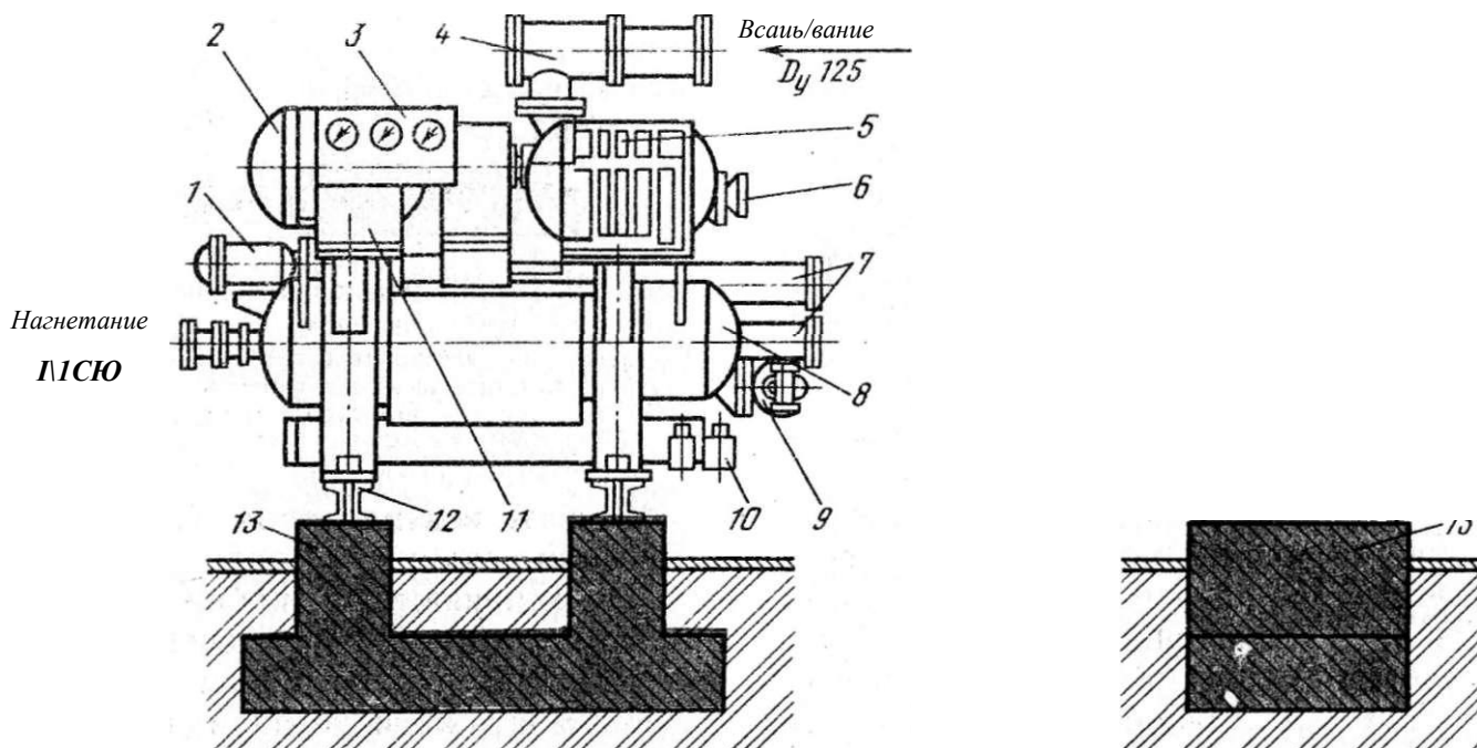
Рис. 18. Общий вид винтового компрессора на фундаменте:
