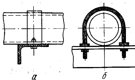
Рис. 38. Направляющие опоры: а — из полосы; б — из круглой стали
