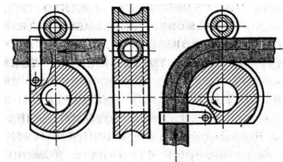
Рис. 44. Схема механического гнутья труб
