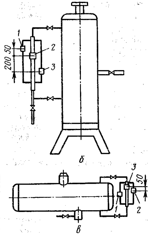
Рис. 51. Схема расположения датчиков ПРУ-5:
