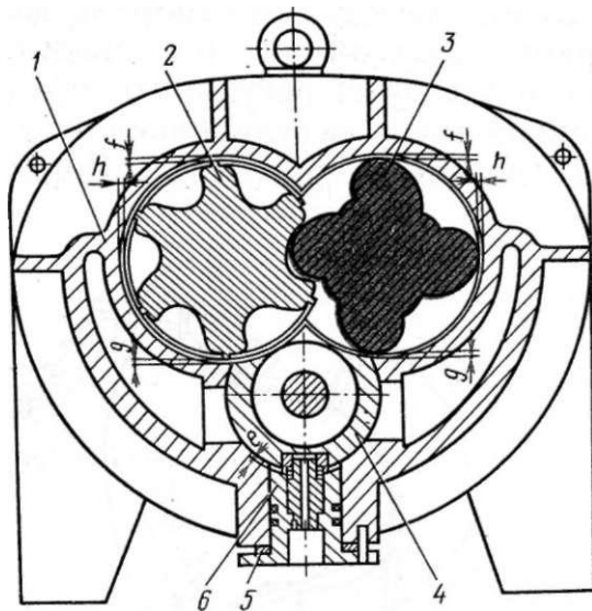
Рис. 157. Винтовой компрессор (сборка):
