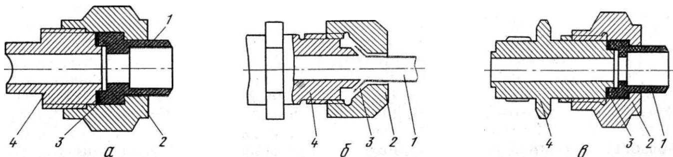
Рис. 31. Штуцерно-торцевые соединения:
