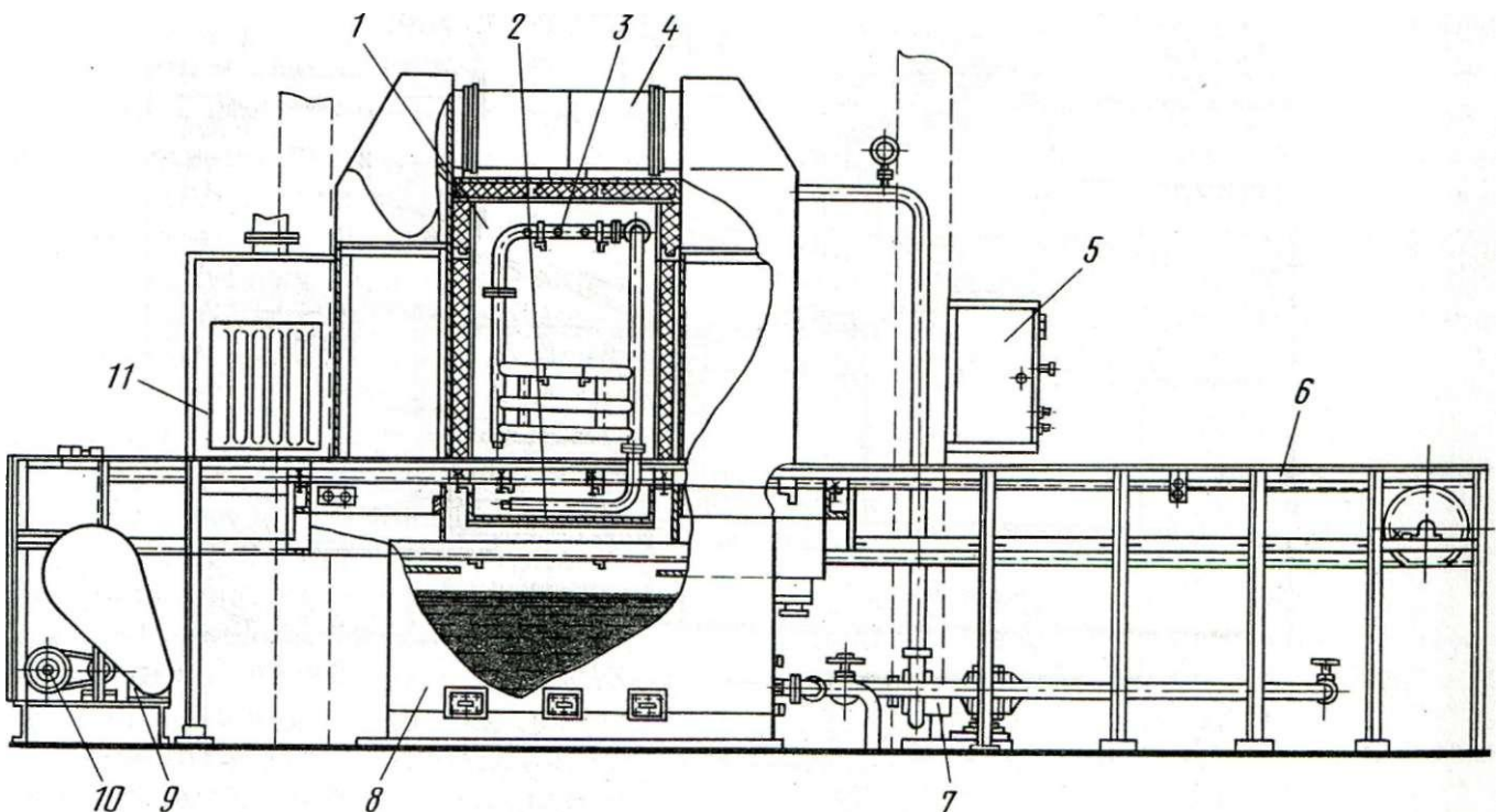
Рис. 93. Конвейерная моечная машина:
