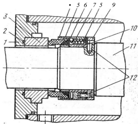
Рис. 140. Сальник винтового компрессора S3-900:
