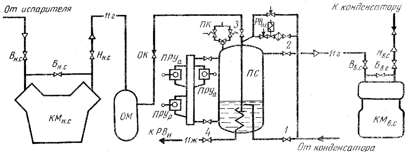
Рис. 63. Схема двухступенчатого холодильного агрегата
