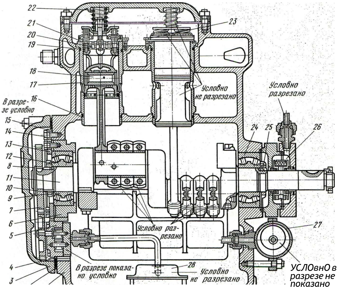
Рис. 146. Компрессор АУУ90 (общая сборка):
