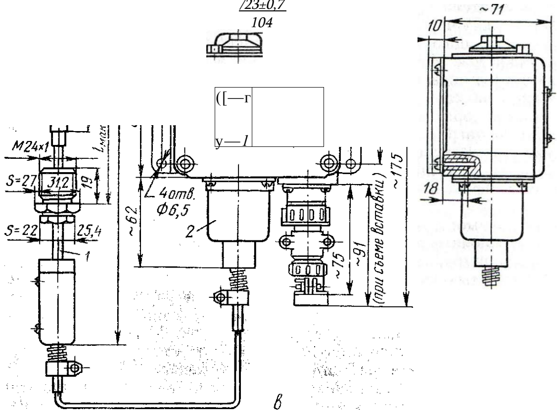
Рис. 53. Реле температуры: типа ПТР-2М; б — типа ПТРД-2; о — типа ТР-1 Б и ТР-2Б; / — датчик прибора; 2 - • корпус прибора
