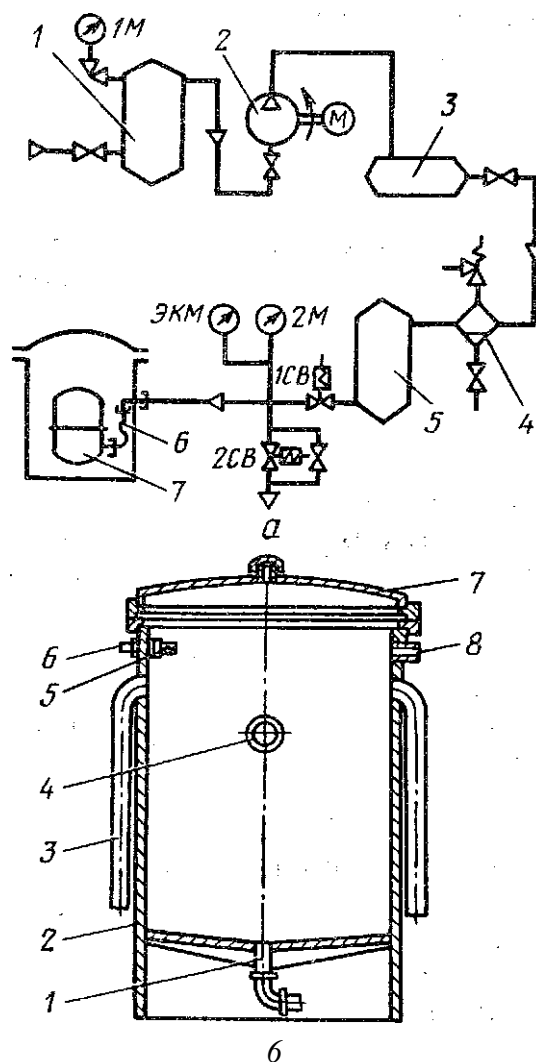
Рис. 170. Установка броневанны:
