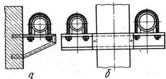
Рис. 40. Кронштейны для трубопроводов:
