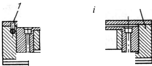
Рис. 5. Слесарный уровень: 1 — ампула; 2 — корпус
