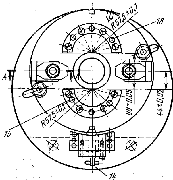
Рис. 106. Приспособление для растачивания блока цилиндров:
