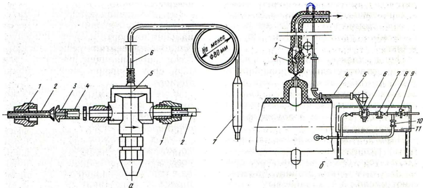
Рис. 49. Терморегулирующие вентили:
