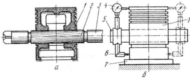
Рис. 111. Инструмент и приспособление для ремонта отверстий в бобышках поршня:
