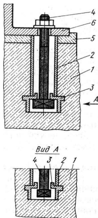
Рис. 4. Анкерный болт:
