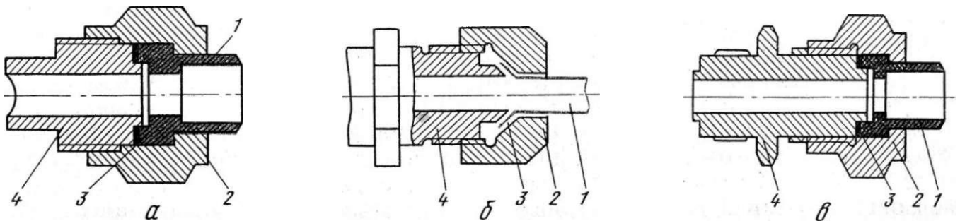
Рис. 31. Штуцерно-торцевые соединения:
