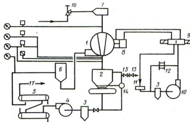
Рис. 64. Схема холодильной установки с винтовым компрессорным агрегатом:
