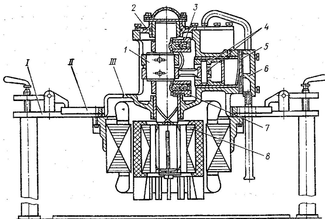
Рис. 169. Приспособление для разборки и сборки герметичных компрессоров:
