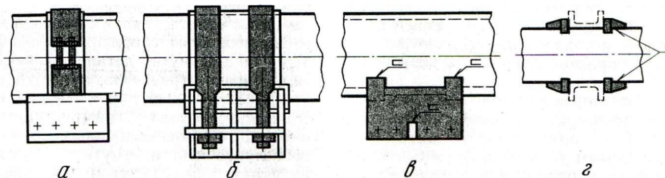
Рис. 39. Неподвижные опоры: а — однохомутовая; б — двуххомутовая; в — приварная; г — с приварными упорами
