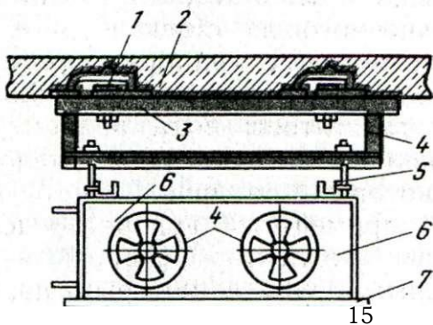
Рис. 24. Схема монтажа подвесных воздухоохлаждителей:
