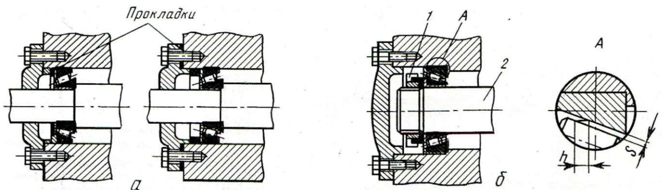
Рис. 128. Регулирование зазоров в подшипниках качения:
