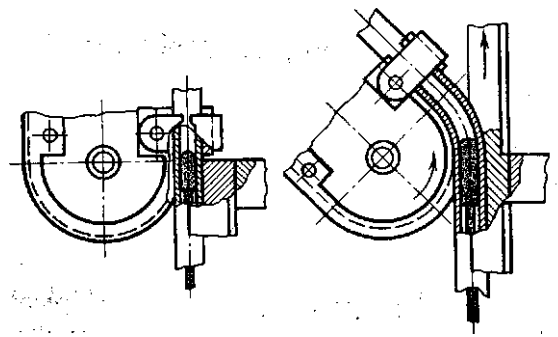
Рис. 45. Схема гнутья труб с калибрующей пробкой
