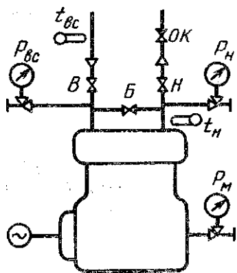
Рис. 61. Компрессор с ручным байпасом
