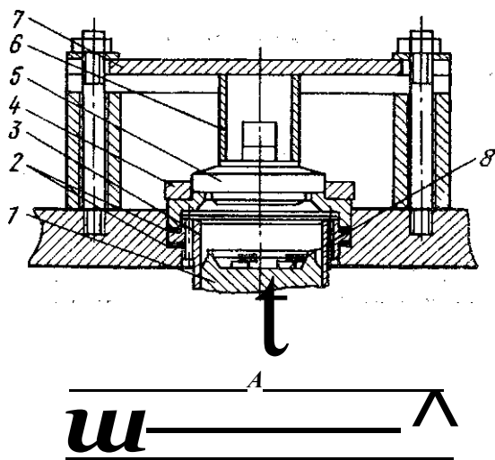
Рис. 152. Приспособление для измерения величины линейного мертвого пространства: 1 — поршень; 2 — прокладки; 3 — гильза цилиндра; 4 — корпус всасывающего клапана; 5 — клапан нагнетательный; 6 — втулка; 7 — планка; 8 — свинцовые пластинки; А — эскиз планки
