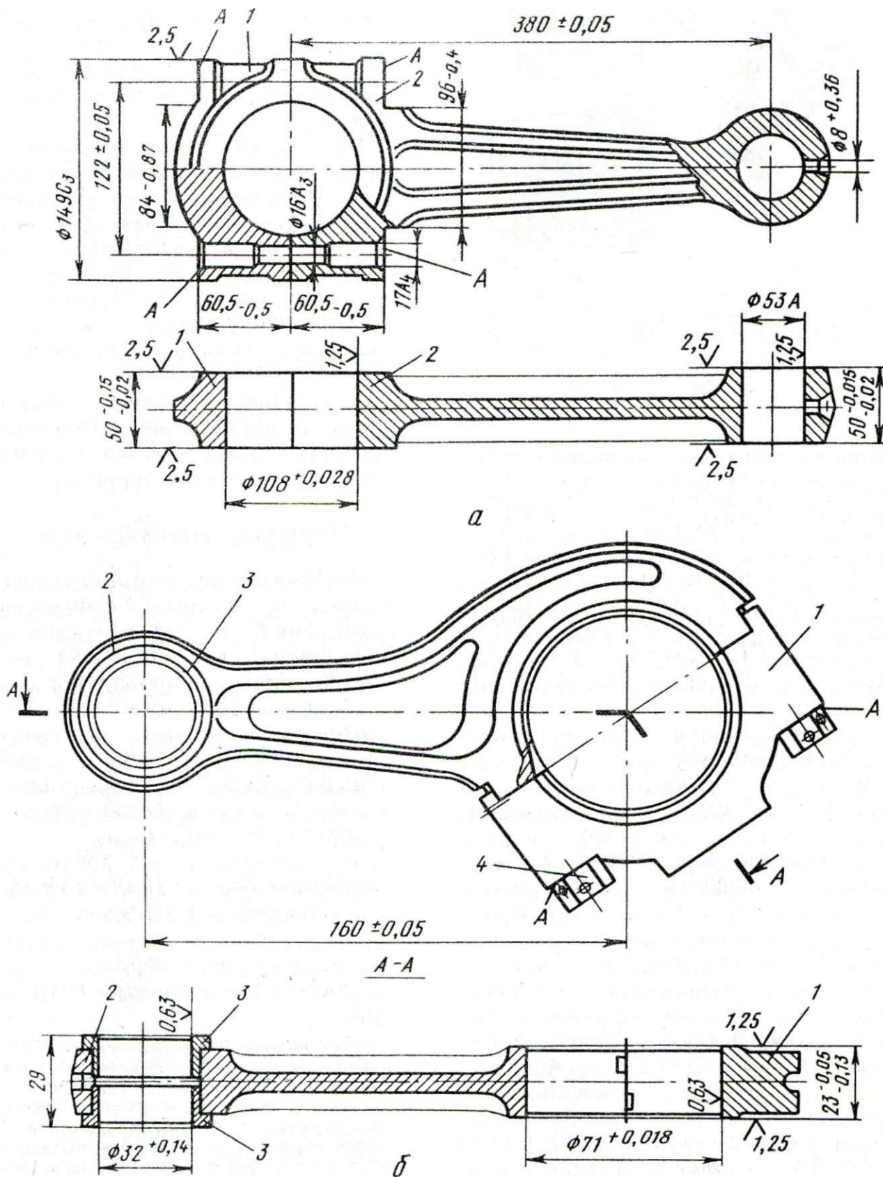
Рис. 17. Шатуны:
