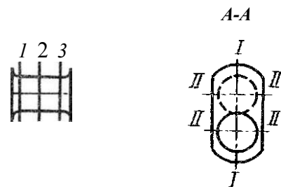
Рис. 130. Схема измерения шеек коленчатого вала
