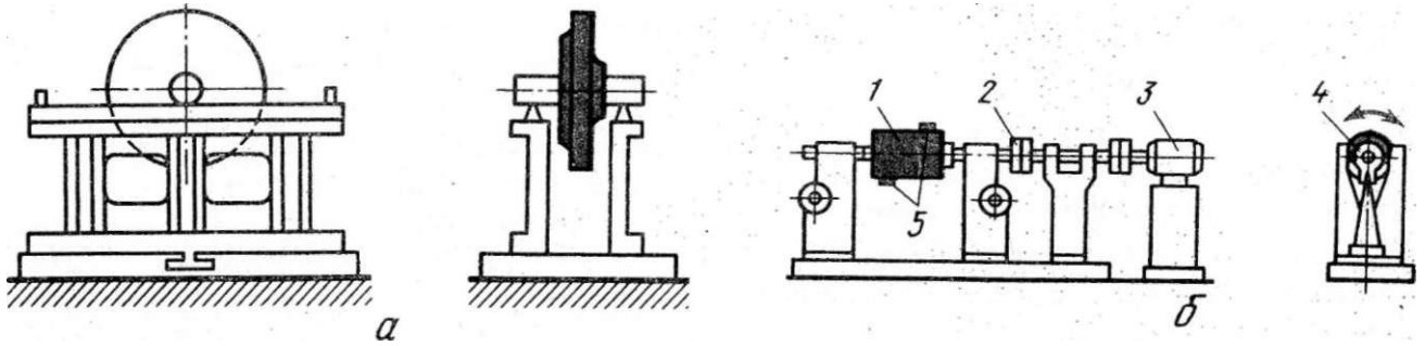
Рис. 145. Балансировка узлов машин:
