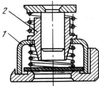
Рис. 137. Нагнетательный клапан с пяточковой пластиной:
