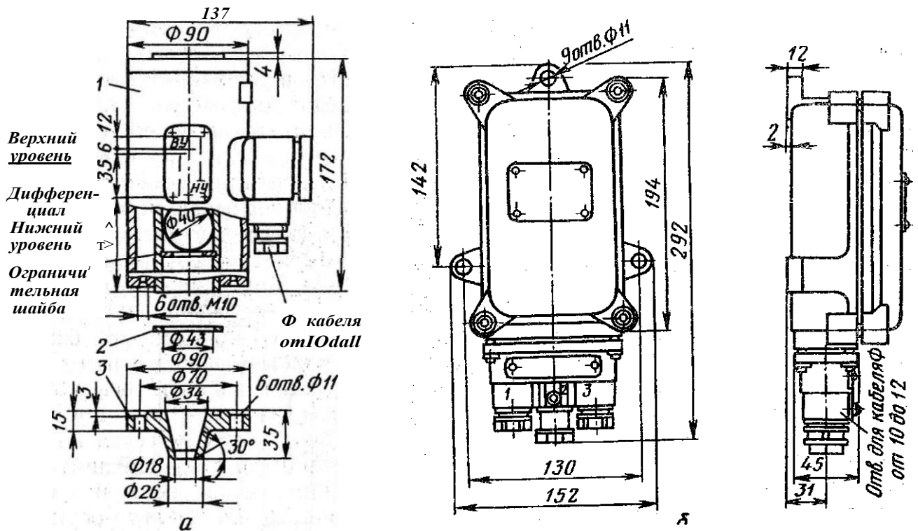
Рис. 50. Реле уровня жидкости ПРУ-5:
