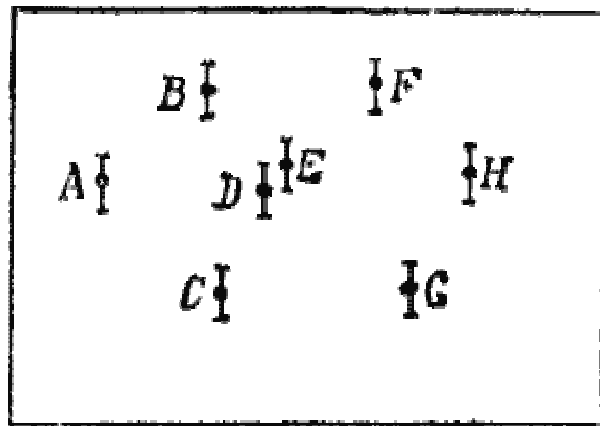
Рис. 5. Фотография, полученная с помощью искровой камеры. Взаимодействие в точке А даёт три следа: ABF , ACG , ADEH . Проведите треки. Раскрасьте их, как вам нравится, и проинтерпритируйте.
