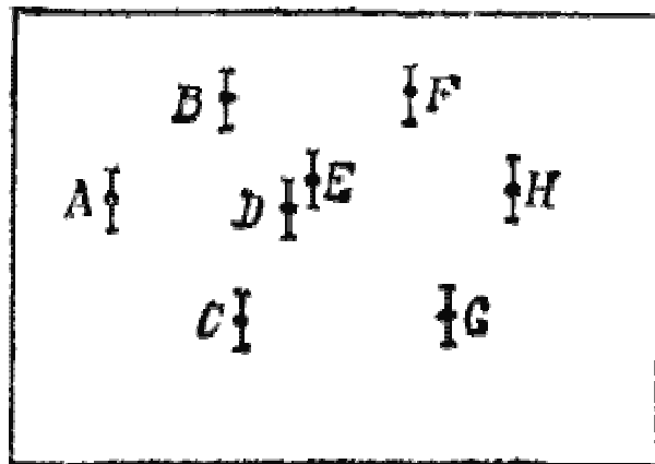
Рис. 6. Экспериментальные точки, нанесённые на идиотграмму. Если вы идиот, раскрасьте их во все цвета радуги. Если вы не идиот, не раскрашивайте. Просто примите антигистогаммную таблетку и ложитесь спать.
