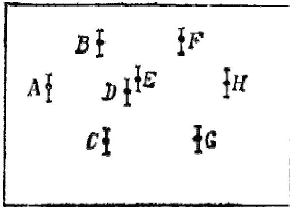
Рис. 7. Экспериментальные точки на диаграмме Фейнмана. Соедините их между собой всевозможными сплошными, пунктирными и волнистыми линиями. Раскрасьте их калибровочно-инвариантным образом.
