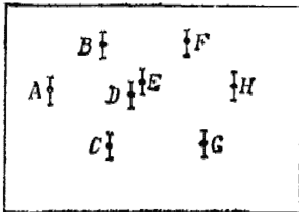
Рис. 9. Загадочный. Найдите на нём промежуточный бозон.
