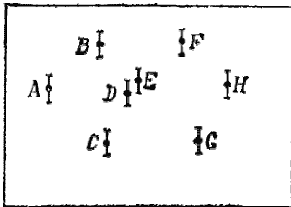
Рис. 8. Точки являются экспериментальным доказательством существования нового унитарно-симметричного октета. Некогда раскрашивать эту картинку. Отсылайте её в «Phys. Rev. Letters» или «New York Times» немедленно!
