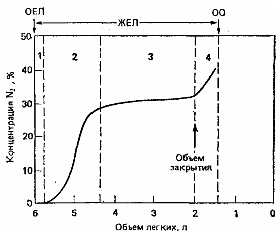
Рис. 10.7. Измерение объема закрытия воздухоносных путей. Обследуемый делает максимальный выдох, затем — максимальный вдох из емкости с чистым кислородом, после чего опять максимальный выдох. Во время второго выдоха концентрация азота в трубке, которую обследуемый держит во рту, изменяется, проходя четыре характерные стадии (подробнее см. в тексте). Последняя из этих стадий обусловлена тем, что воздухоносные пути в нижних отделах легких закрываются, и воздух преимущественно выходит из верхушек
