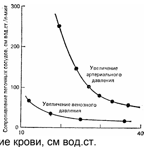
Рис. 4.4. Кривая, отражающая снижение сопротивления легочных сосудов при повышении давления в легочных артериях или венах. Артериальное давление изменялось при постоянном венозном давлении (12 см вод. ст.), а венозное—при постоянном артериальном (37 см вод. ст.). Данные получены на препарате изолированных легких собаки
