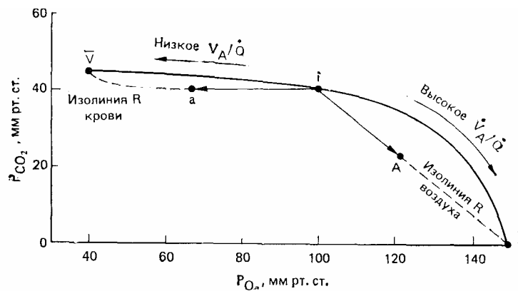
Рис. 10.4. Кривая P_{CO_2} — P_{O_2} . Точка “i” соответствует гипотетическому “идеальному” составу альвеолярного воздуха и крови конечных отрезков капилляров при полной равномерности вентиляционно-перфузионного отношения. Если эта равномерность нарушается, происходит сдвиг к точкам а (артериальная кровь) и А (альвеолярный воздух) вдоль прямых, соответствующих дыхательному коэффициенту (R). Альвеолярно-артериальная разница по P_{O_2} определяется расстоянием между точками а и А по горизонтали
