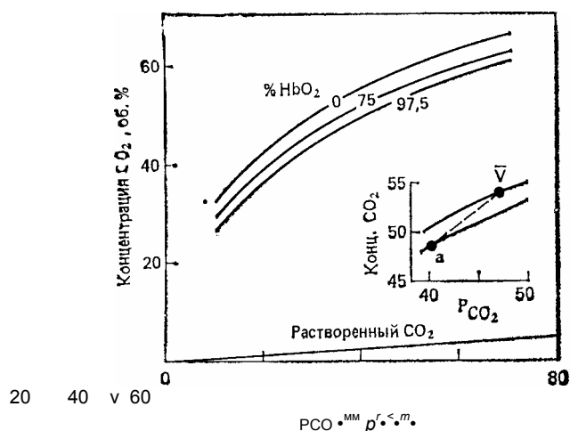
Рис. 6.6. Сатурационные кривые \text{CO}_2 в крови при различном насыщении ее кислородом. Видно, что при одном и том же P_{\text{CO}_2} оксигенированная кровь связывает меньше \text{CO}_2 , чем неоксигенированная. Приведена также эффективная кривая, отражающая переход от артериальной к смешанной венозной крови
