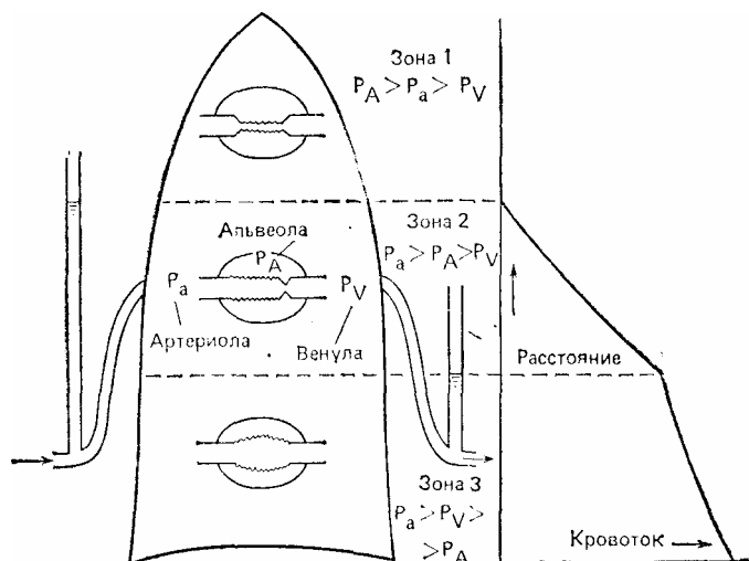
Рис. 4.9. Модель, связывающая неравномерность распределения легочного кровотока с величиной давления, действующего на капилляры (J. V. West et al.: Appl. Physiol., 19:713, 1961)
