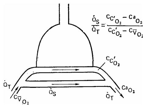
Рис. 5.3. Измерение шунтового кровотока. Количество кислорода в артериальной крови равно сумме его количеств в капиллярной крови и в крови, оттекающей по шунтам. Подробнее см. в тексте
