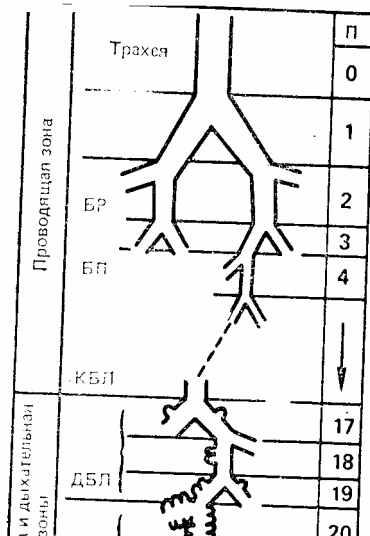
Рис. 1.4. Упрощенная схема воздухоносных путей человека по Вейбелю. Видно, что к проводящей зоне легких относятся дыхательные пути 0—16 порядков (П), а к дыхательной (или переходной и дыхательной) зоне—17—23 порядков. ВР — бронхи; БЛ — бронхиолы; КБЛ — конечные бронхиолы; ДБЛ — дыхательные бронхиолы; АХ — альвеолярные ходы; А — альвеолы (E. R. Weibel: Morphometry of the Human Lung. Berlin, Springer-Verlag, 1963, p. 111)
