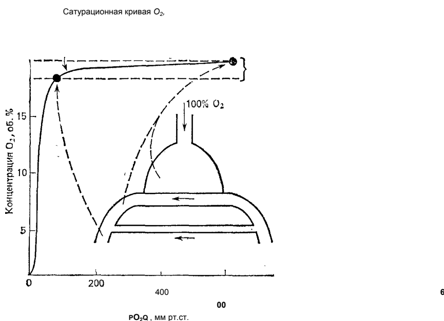
Рис. 5.4. Наличие шунтов приводит к снижению P_{O_2} в артериальной крови даже при дыхании чистым кислородом. Примешивание небольших количеств “шунтовой” крови с низкой концентрацией O_2 сопровождается значительным уменьшением P^a артериальной крови, так как сатурационная кривая O_2 идет почти горизонтально
