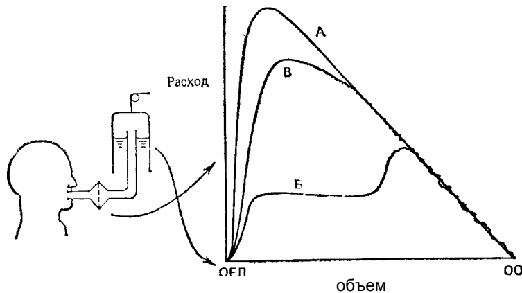
Рис. 7.16. Кривые расход—объем. А. Форсированный выдох после максимального вдоха. Б. Выдох сначала медленный, а затем форсированный. В. Выдох со скоростью выше средней. Во всех трех случаях нисходящие участки кривых совпадают
