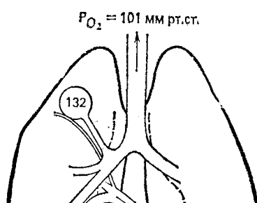
Рис. 5.11. Схема легких человека в вертикальном положении, иллюстрирующая уменьшение P_{O_2} в артериальной крови при неравномерном вентиляционно-перфузионном отношении. Приведены только два участка легких: один в области верхушки, другой в области основания. Размеры воздухоносных путей и кровеносных сосудов на рисунке соответствуют относительным величинам их вентиляции и кровотока. Поскольку большая часть крови поступает от плохо оксигенируемого нижнего участка, неизбежно понижение P_{O_2} в артериальной крови (J. B. West:
