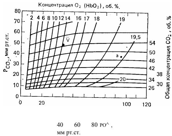
Рис. 6.7. А. Типичные сатурационные кривые CO_a и O_a , приведенные в одном масштабе. Видно, что для CO_a кривая намного круче. 5. Графики O_a — CO_2 с изоконцентрационными кривыми для этих двух газов. Эти кривые не параллельны координатным осям, что объясняется эффектами Бора и Холдейна. Приведены также типичные точки для артериальной и смешанной венозной крови
