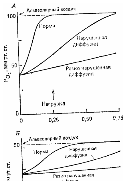
Рис. 3.3. Поглощение O 2 по ходу легочного капилляра в условиях нормальной и нарушенной (например, при утолщении альвеолярных мембран) диффузии. А — при нормальном P O 2 в альвеолярном воздухе; Б — при пониженном P O 2 в альвеолярном воздухе (видно, что оксигенация при этом происходит медленнее).
