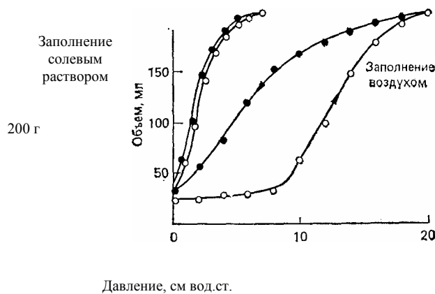
Рис. 7.5. Кривые давление—объем для легких кошки, наполненных воздухом и солевым раствором. Светлые кружки—раздувание; темные кружки — спадание. Видно, что легкие, наполненные солевым раствором, более растяжимы и гистерезис у них значительно менее выражен (E. P. Radford: Tissue Elasticity. Washington, D. C., American Physiological Society, 1957, p. 177)
