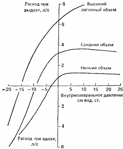
Рис. 7.17. Изоволюмические кривые давление—расход для трех различных уровней объема легких. При построении каждой кривой обследуемые делали несколько форсированных выдохов и вдохов (подробнее см. в тексте). Видно, что в случае большого легочного объема скорость выдоха увеличивается за счет повышения внутриплеврального давления, которое в свою очередь обусловлено усилением деятельности экспираторных мышц. Однако при среднем и малом легочном объеме расход воздуха, начиная с некоторой величины внутриплеврального давления, становится независимым от усилия (D. L. Fry, R. E. Hyatt: Am. J. Med. 29:672, 1960)
