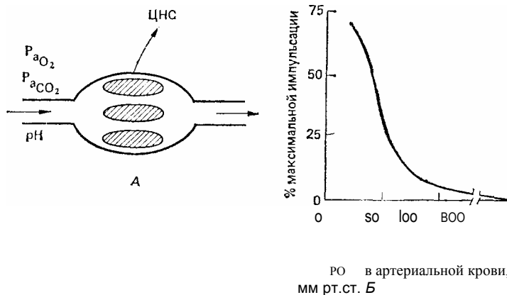
Рис. 8.3. А. Каротидное тельце, воспринимающее изменения P_{O_2} , P_{CO_2} и pH артериальной крови. Импульсы от этих телец поступают в центральную нервную систему (ЦНС) по нерву Геринга. Б. Кривая зависимости импульсации хеморецепторов от P_{O_2} , артериальной крови. Видно, что наибольшая чувствительность хеморецепторов приходится на P_{O_2} ниже 50 мм рт. ст.
