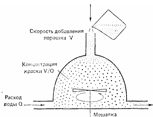
Рис. 5.5. Модель “функциональной единицы” легкого, объясняющая слияние вентиляционно-перфузионного отношения на PQ ; краска добавляется в камеру со скоростью V (аналог вентиляции) и удаляется из нее со скоростью Q (аналог кровотока). Концентрация краски (аналог PO_2 в альвеолярном воздухе) равна отношению V/Q (J. B. West: Ventilation/Blood Flow and Gas Exchange, ed. 3. Oxford, Blackwell, 1977)
