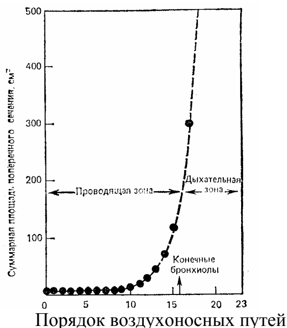
Рис. 1.5. Кривая зависимости суммарного поперечного сечения воздухоносных путей от их порядка. Видно, что в дыхательной зоне оно резко возрастает (см. для сравнения рис. 1.4). В результате в области дика". тельных бронхиол продольное перемещение воздуха во время вдоха становится очень небольшим и роль главного механизма вентиляции начинает играть диффузия
