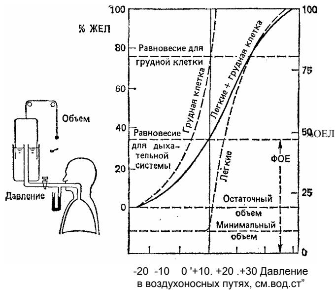
Рис. 7.11. Релаксационные кривые давление—объем для легких и грудной клетки. При построении таких кривых обследуемый делает вдох (или выдох) из спирометра до определенного объема, воздушную трубку перекрывают, после чего обследуемый расслабляет дыхательные мышцы. Общая кривая для легких и грудной клетки равна графической сумме соответствующих им кривых (по Н. Rahn et al.: Am. J. Physiol., 146: 161, 1946, с изменениями)
