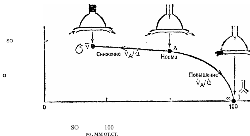
Рис. 5.7. Кривая вентиляционно-перфузионного отношения, представленная графиком зависимости PO_2 — CO_a . При увеличении вентиляционно-перфузионного отношения значения P_d^A и P_{CO_a} смещаются вдоль кривой от точки смешанной венозной крови v к точке вдыхаемого газа I (см. для сравнения рис. 5.6) (J. B. West: Ventilation/Blood Flow and Gas Exchange, ed. 3. Oxford, Blackwell, 1977)
