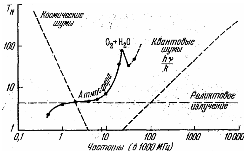
Рис. 88. Спектр шумов в радиодиапазоне
