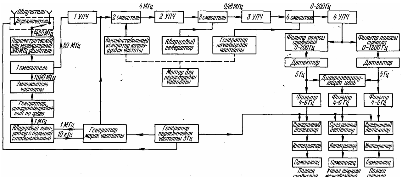
Рис. 95. Блок-схема приемника Дрэйка
