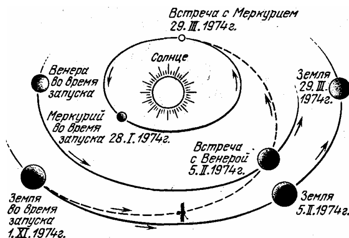
Рис. 70. Схема полета к Венере и Меркурию АМС «Маринер-10»
