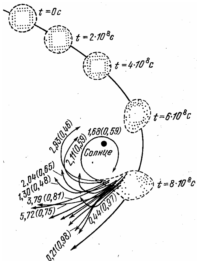
Рис. 48. Модель столкновения протосолнца с протозвездой. Орбиты захваченных сгустков характеризуются значениями большой полуоси (в единицах 10^{14} см) и (в скобках) эксцентриситета. Буквой t обозначены моменты времени, выраженные в секундах
