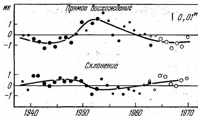
Рис. 41. Отклонения в собственном движении звезды Барнарда за 24 года
