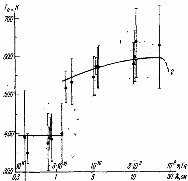
Рис. 67. Радиоспектр Венеры. Вертикальные черточки — погрешности наблюдений
