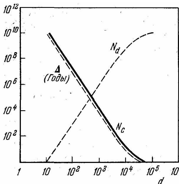
Рис. 103. Графики Брэйсуэлла По оси абсцисс откладывается среднее расстояние между инопланетными цивилизациями в световых годах, по оси ординат отложены: N_c — число одновременно существующих в Галактике цивилизаций, N_d — число звезд на расстоянии d от данной звезды, около которой имеется цивилизация, \Delta — средняя продолжительность технологической эры
