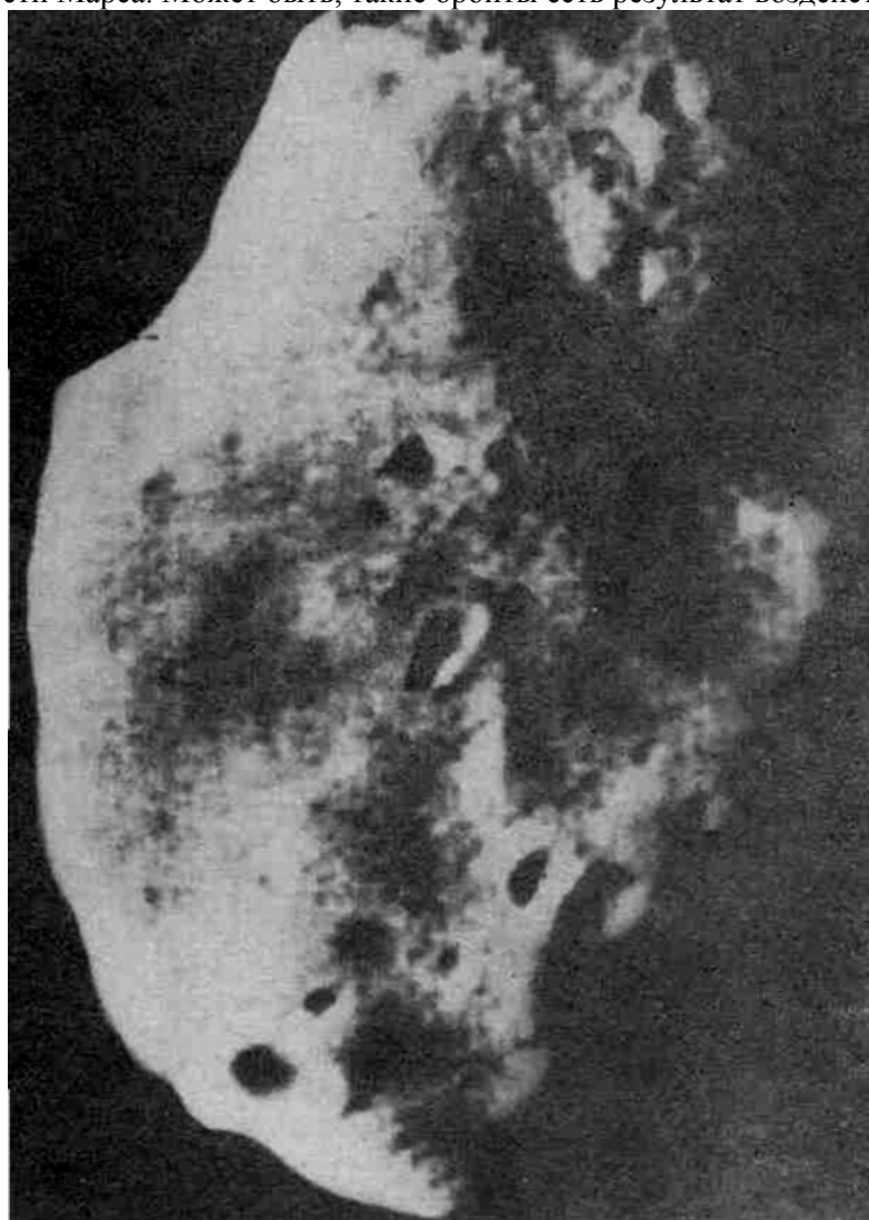
Рис.85 Фотография Фобоса, полученная АМС "Маринер-9"
