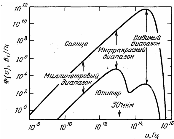
Рис. 40. Кривые зависимости мощности излучения в единичном частотном интервале от частоты для Солнца и Юпитера в идеализированном предположении о чернотельном механизме излучения
