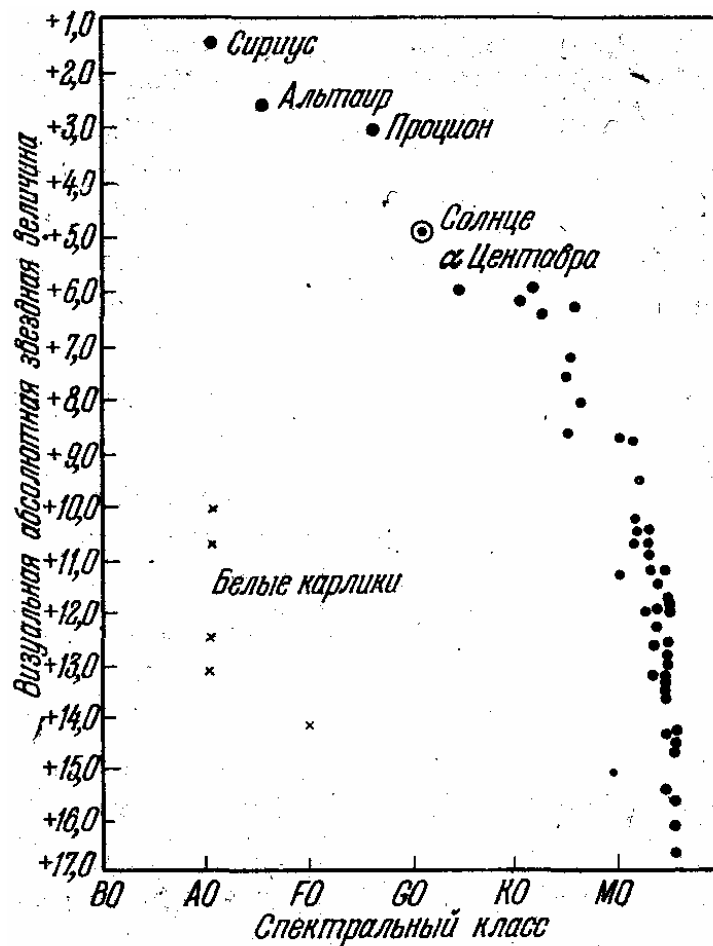
Рис. 10. Диаграмма Герцшпрунга — Рессела для близких звезд
