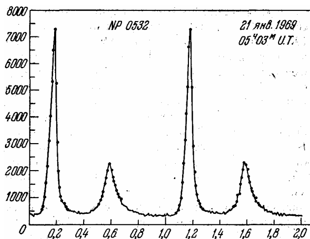
Рис. 27. «Кривая блеска» пульсара NP 0532
