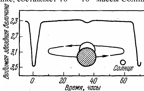
Рис. 37. Схема затменной двойной звезды
