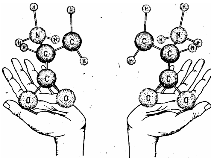
Рис. 55. «Левые» и «правые» органические молекулы
