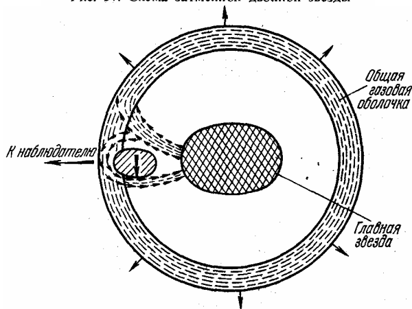
Рис. 38. Система \beta Лиры (схема)
