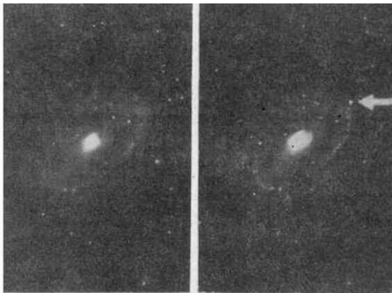
Рис. 19. Вспышка сверхновой в далекой галактике. На правой фотографии, полученной в 1940 г., сверхновая видна, на левой, полученной в 1931 г., — нет
