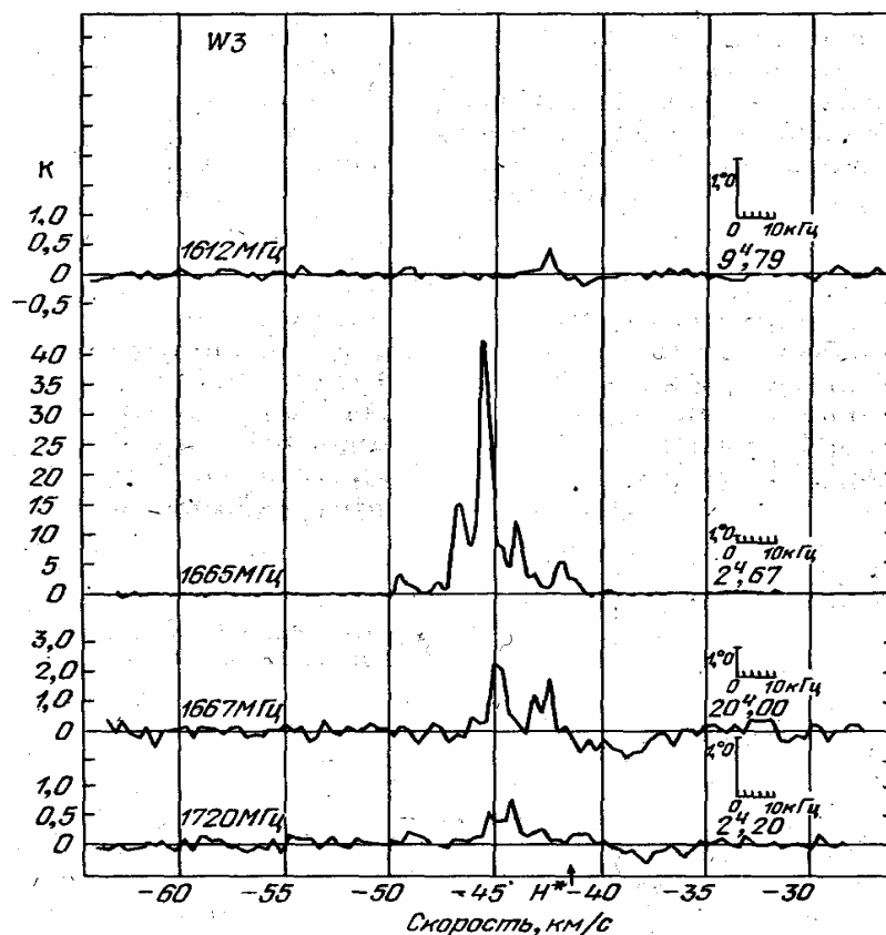
Рис. 13. Профили четырех компонент линии гидроксила, излучаемых источником W3
