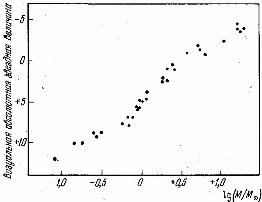
Рис. 11. Зависимость светимости звезд от их массы
