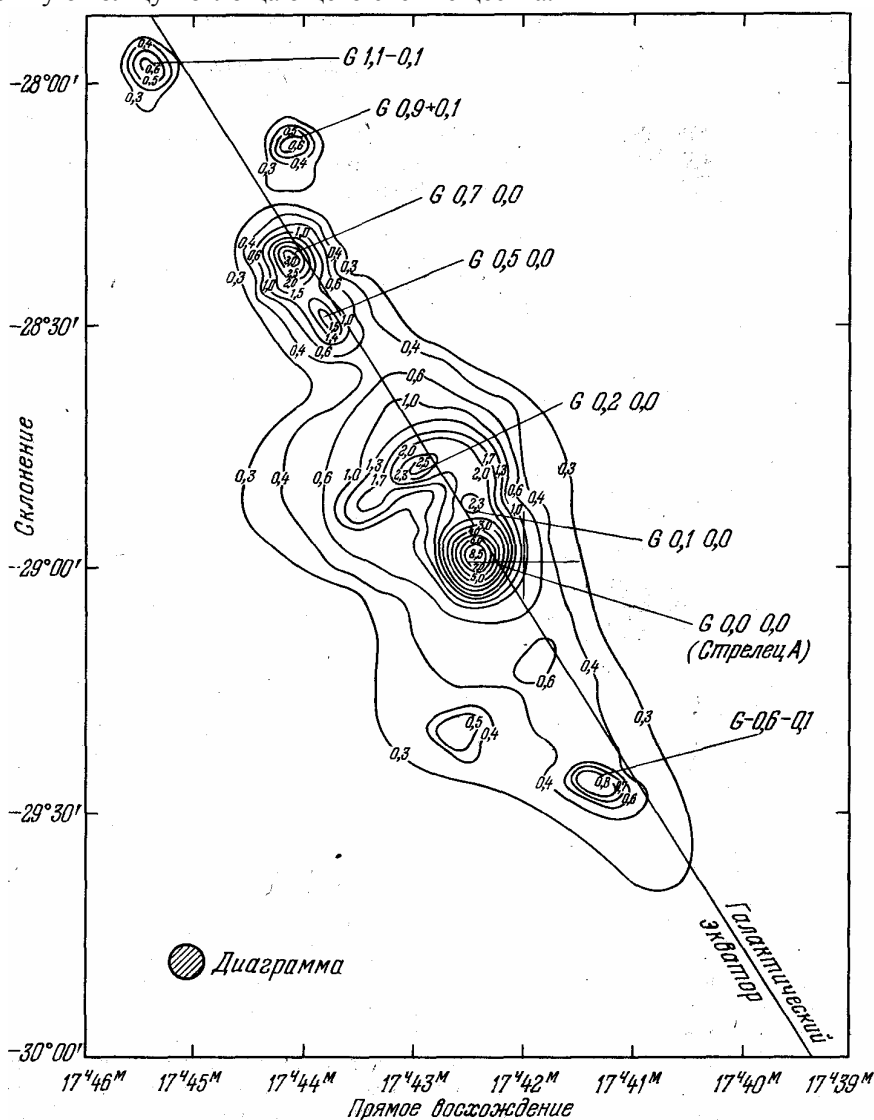
Рис. 31. «Радиоизображение» области галактического центра
