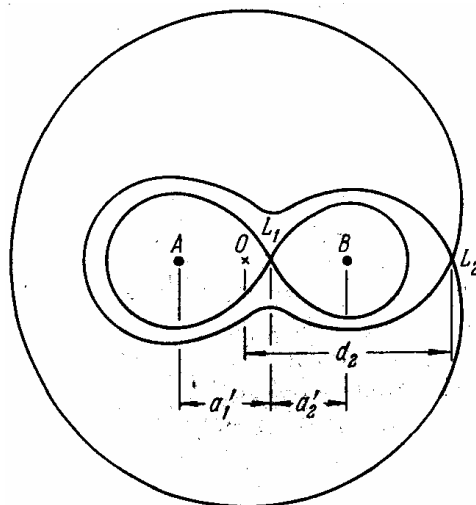
Рис. 50. Область «благоприятных» планетных орбит в двойной системе
