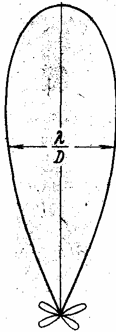
Рис. 89. Диаграмма направленности антенны (схема)
