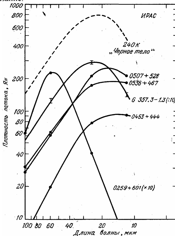
Рис. 116. Источники с максимумом в спектре из каталога спутника ИРАС. Плотность потока скорректирована к чернотельному спектру в соответствии с процедурой калибровки ИРАС (Нейгебауэр и др., 1984)
