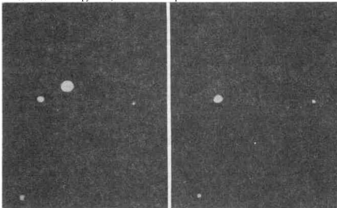
Рис. 26. Фотография пульсара NP 0532, полученная с помощью стробоскопа
