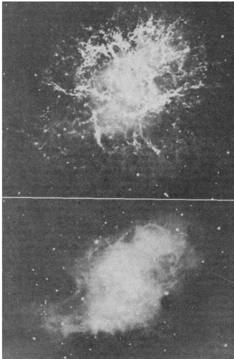
Рис. 20. Крабовидная туманность.
