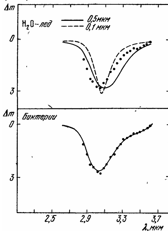
Рис. 78. Вверху: сплошная линия — теоретический профиль полосы поглощения льда при размере частиц 0,5 мкм, пунктир — то же для размеров 0,1 мкм; внизу — теоретический профиль поглощения, обусловленного бактериями; точки — данные наблюдений
