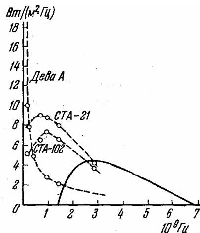
Рис. 118. Ожидаемый спектр космического искусственного радиосигнала согласно Н. С. Кардашеву (сплошная линия) и радиоспектры некоторых известных космических источников радиоизлучения (штриховые линии)
