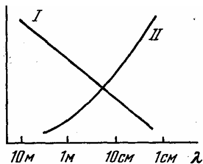
Рис. 34. Спектр галактического (I) и изотропного «трехградусного» (II) излучения
