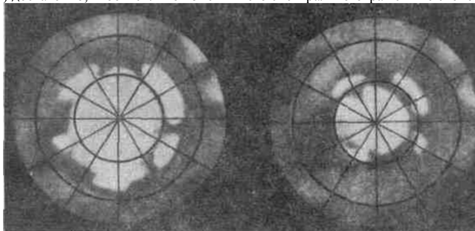
Рис. 65. Таяние полярной шапки Марса
