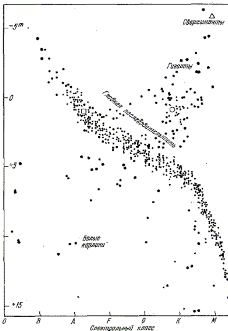
Рис. 9. Диаграмма Герцшпрунга — Рассела. По вертикальной оси — абсолютная звездная величина. По горизонтальной — спектральный класс. Количество точек на диаграмме «спектр—светимость», приведенной на рис 9, не дает
