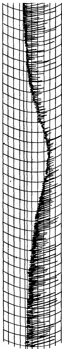
Рис. 94. Типичная запись космического радиоизлучения
