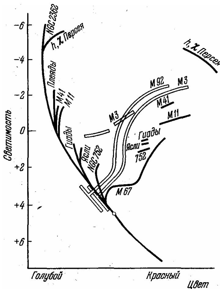
Рис. 17. Сводная диаграмма Герцшпрунга – Рессела для 11 звездных скоплений
