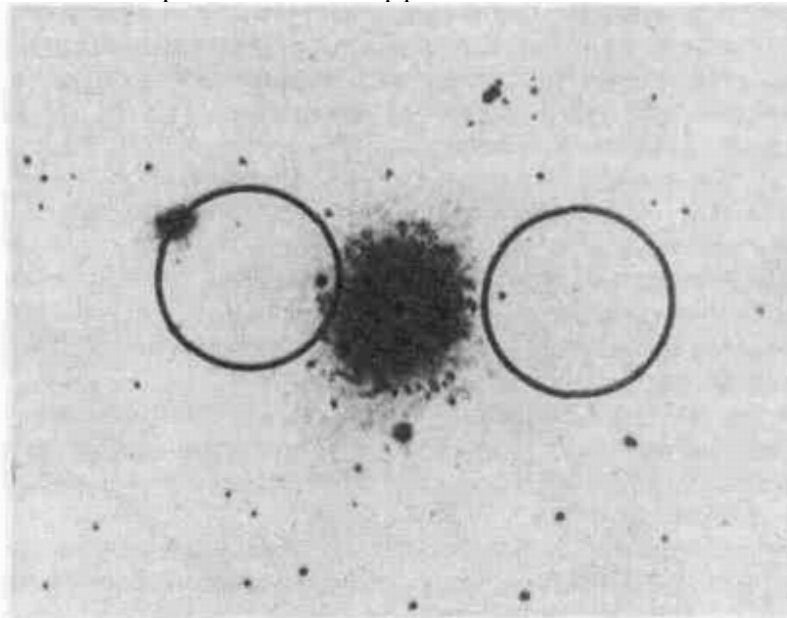
Рис. 33. Радиогалактика 3C 270. Кружками показаны области, из которых исходит излучение. Эти области не совпадают с самой галактикой, а расположены симметрично по обе стороны от нее
