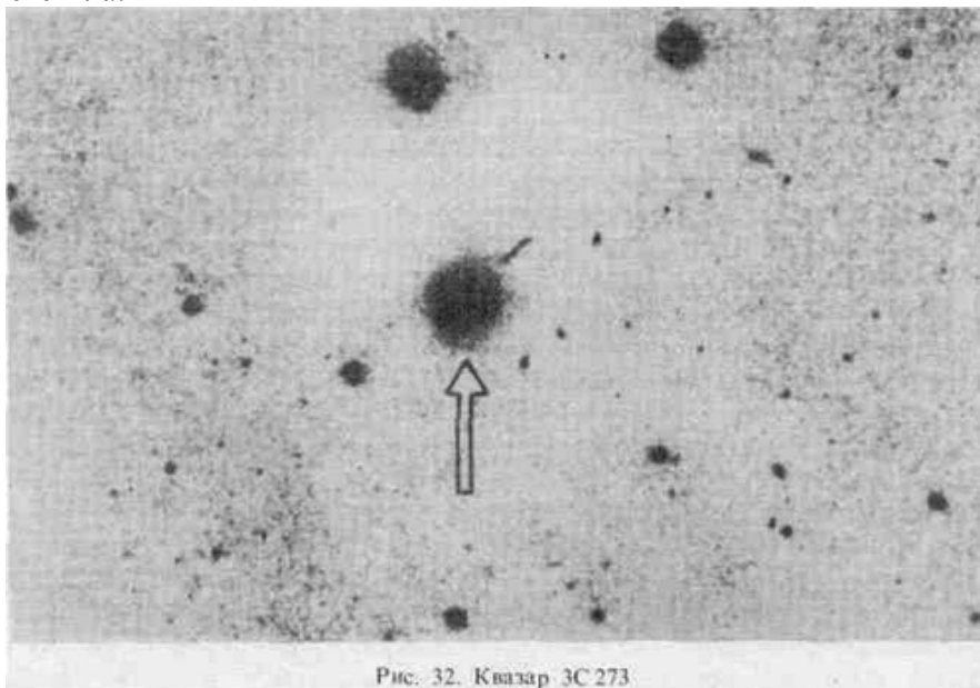
Рис. 32. Квазар 3C 273
