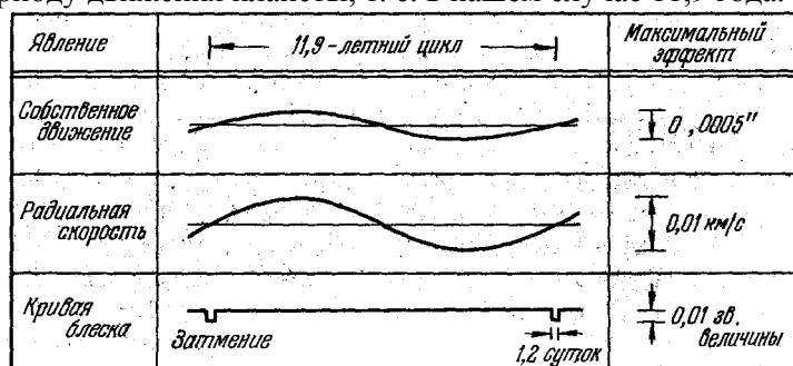
Рис. 39. Три способа обнаружения планет около звезд
