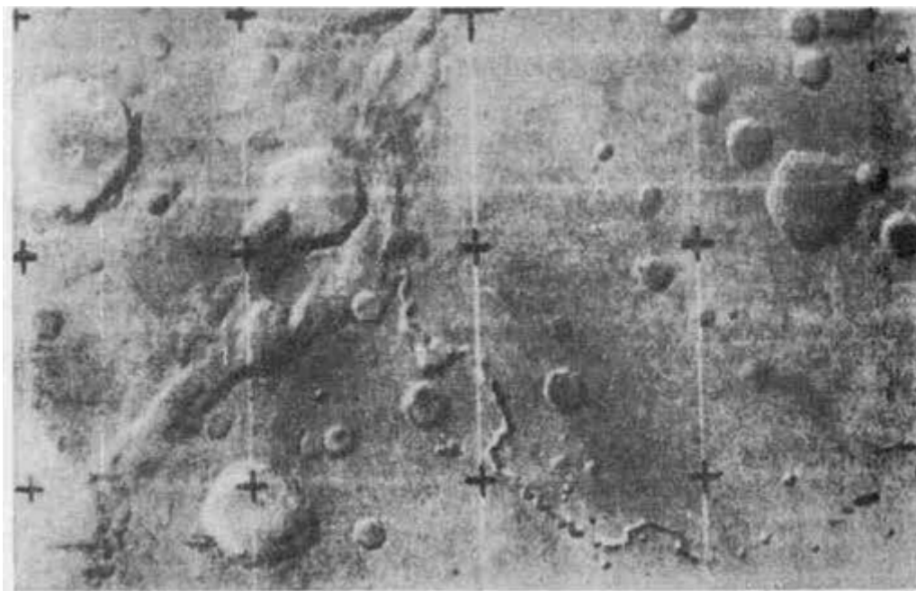
Рис. 64. «Высохшее русло реки» на поверхности Марса. Фотография получена АМС «Марс-5»
