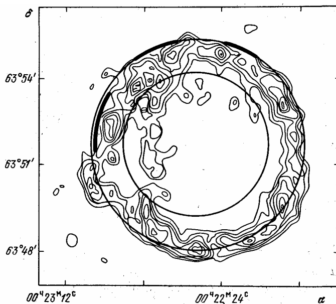
Рис. 24. Схема оптической, радио- и рентгеновской структуры остатка Сверхновой 1572 г. Жирные сплошные линии — оптические волокна. Две концентрические окружности определяют оболочку, излучающую рентгеновские кванты
