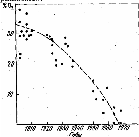
Рис. 109. Процент кислорода в воде Балтийского моря
