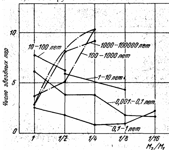
Рис. 43. Результаты анализа 123 близких звезд солнечного типа. Числа у линий указывают интервалы периодов обращения
