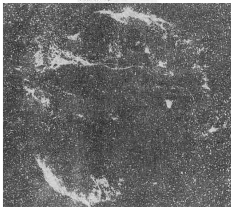
Рис. 22. Волокнистые туманности в созвездии Лебедя
