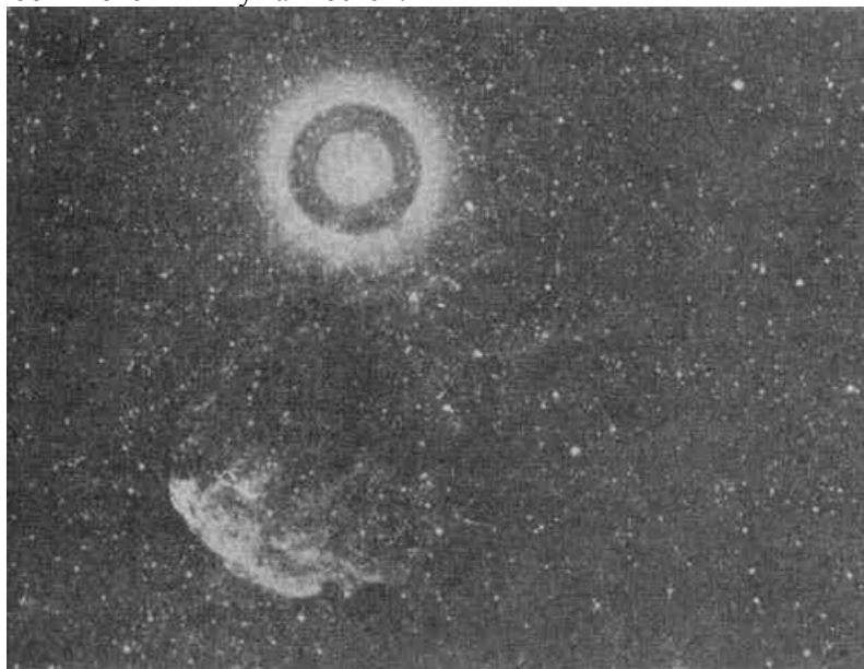
Рис. 21. Туманность IC 443
