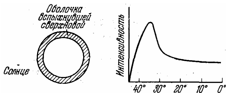
Рис. 29. Схема, поясняющая вспышку сверхновой звезды около Солнца. Справа дано распределение радиояркости оболочки в зависимости от углового расстояния до ее центра
