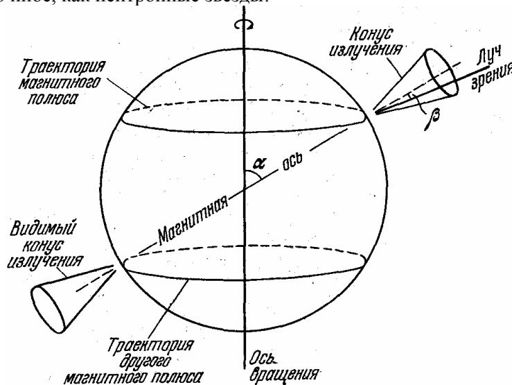
Рис. 25. Модель пульсара
