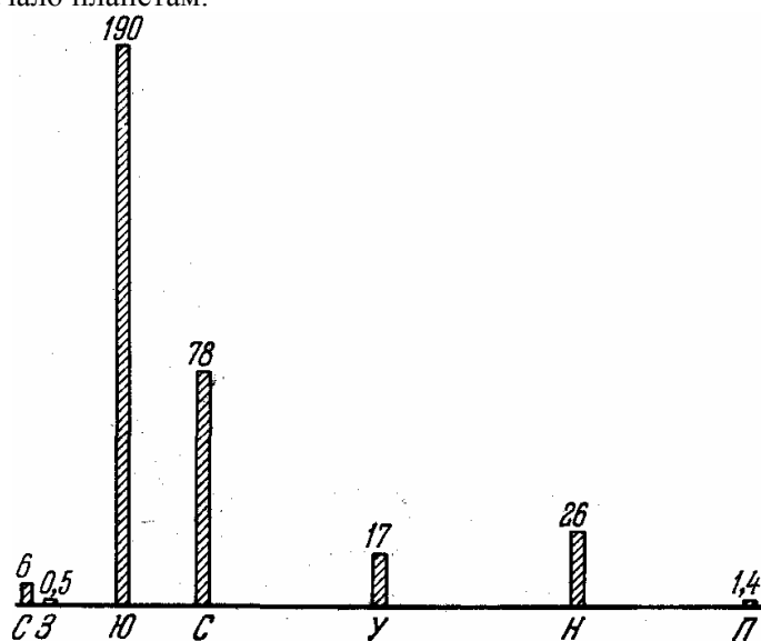
Рис. 47. Распределение вращательного момента в Солнечной системе (в единицах 10^{48} CGS)
