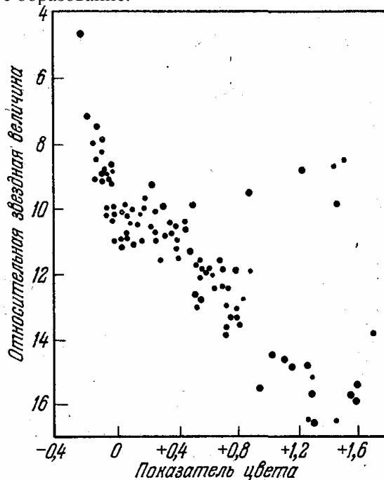
Рис. 15. Диаграмма Герцшпрунга — Ресселя для звездного скопления NGC 2254
