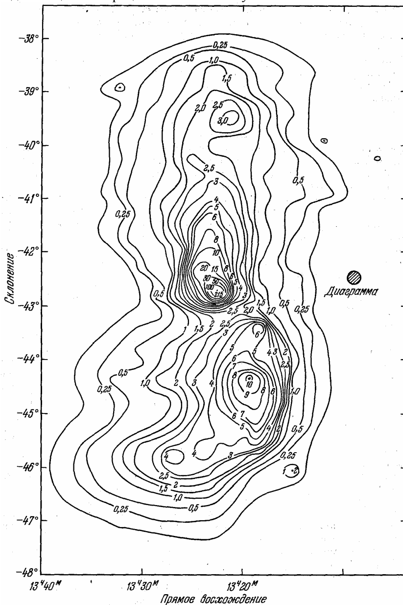
Рис. 30. «Радиоизображение» галактики NGC 5128
