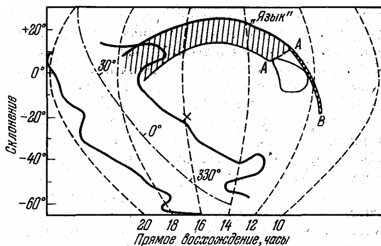
Рис. 28. Изофоты радиоизлучения Галактики (схема)
