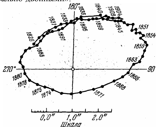
Рис. 36. Последовательные относительные положения компоненты двойной звезды на орбите
