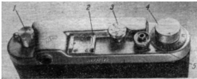
Рис. 91. Арматура камеры «ФЭД»
