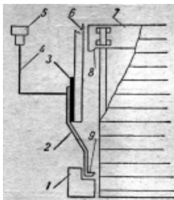
Рис. 141. Схема одноконтактного замыкания синхроустройства:
