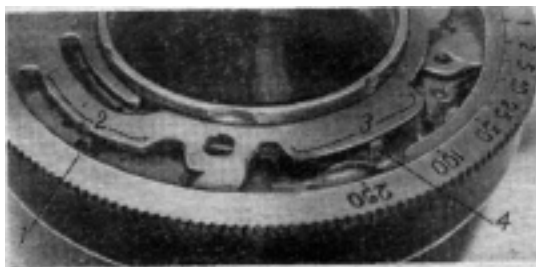
Рис. 57. Установка кольца деления скоростей
