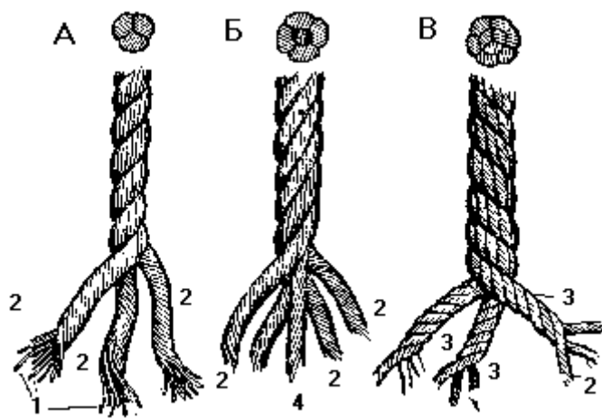
Рис. 55. Растительные тросы: А—трехрядный тросовой работы; Б—четырёхрядный тросовой работы с сердечником; В — кабельной работы; 1 — каболки; 2 — пряди; 3 — стренди; 4 — сердечник.
