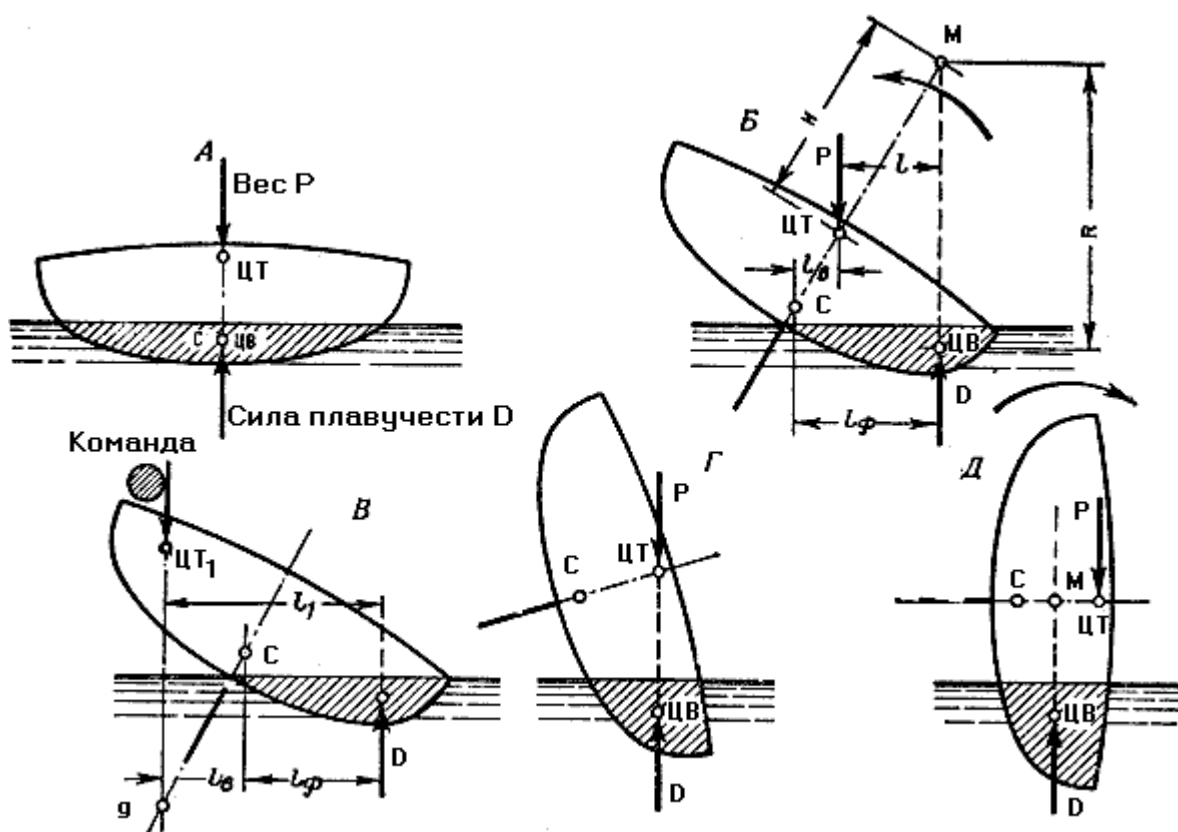
Рис. 78. Остойчивость швертбота
