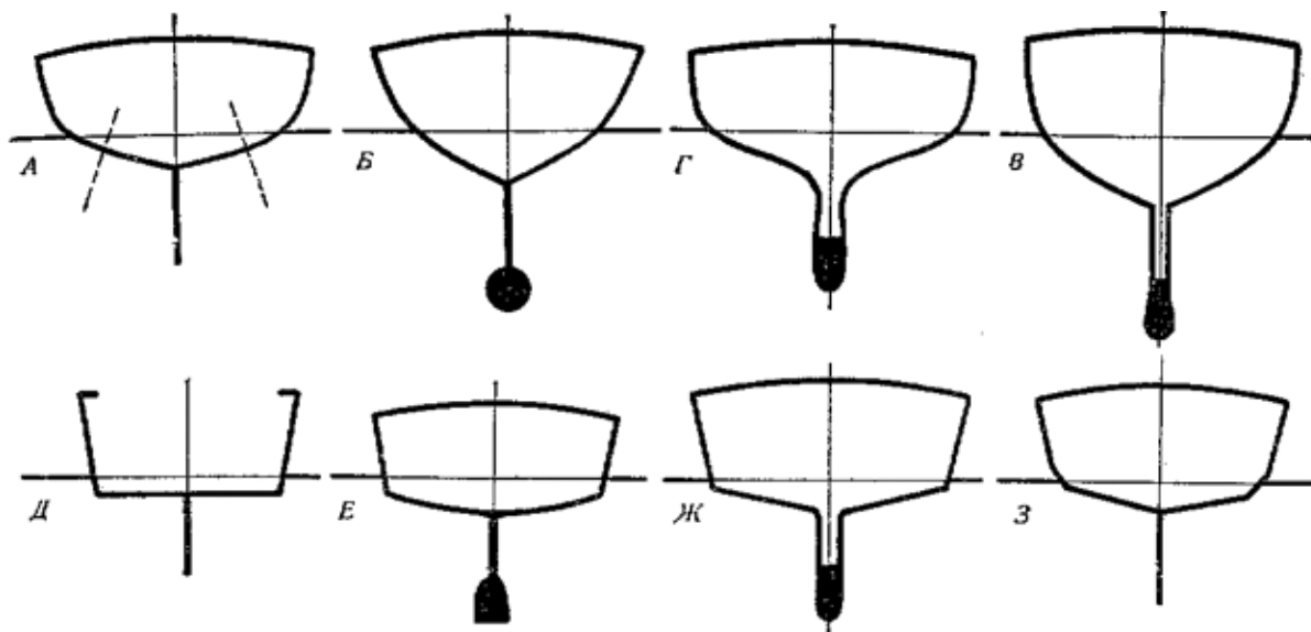
Рис. 9. Формы мидель-шпангоутов.
