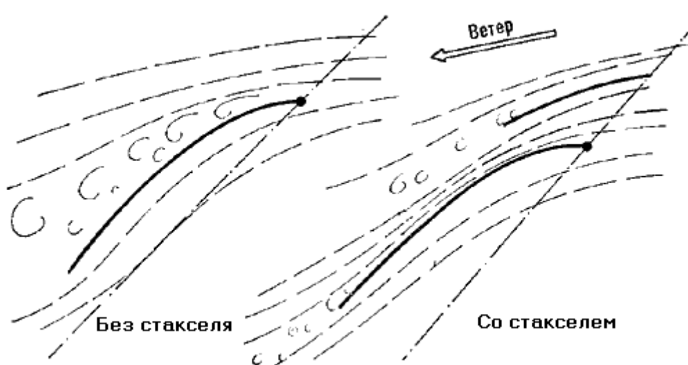
Рис. 97. Работа стакселя
