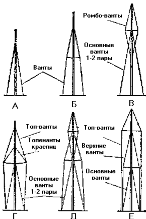
Рис. 38. Проводка вант:
