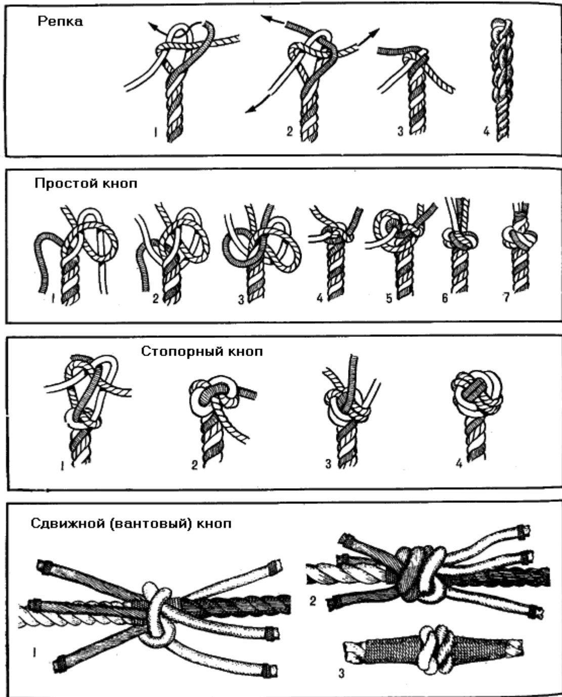
Рис. 69, Кно́пы
