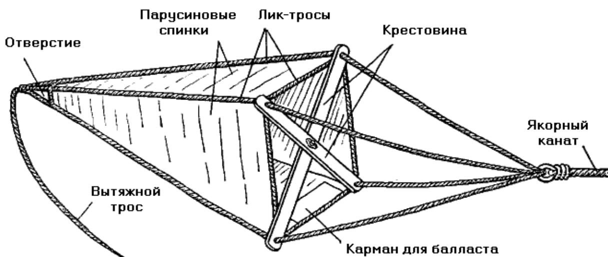
Рис. 117. Плавучий якорь
