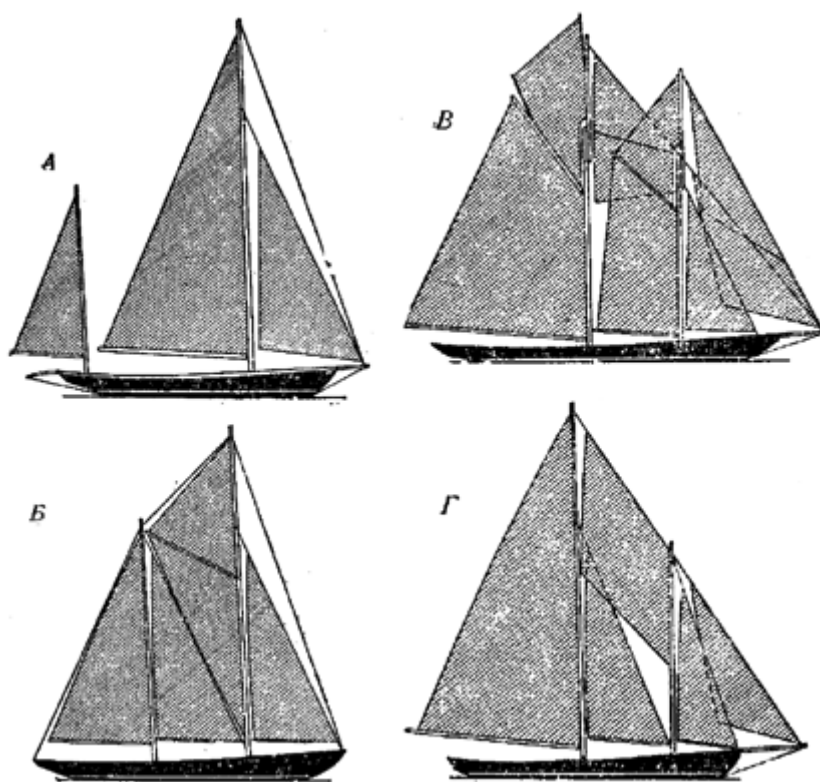
Рис. 15. Двухмачтовые яхты. А — бермудский иолом; б — стаксельный кэч. В — гафельная шхуна; Г — бермудская стаксельная шхуна
