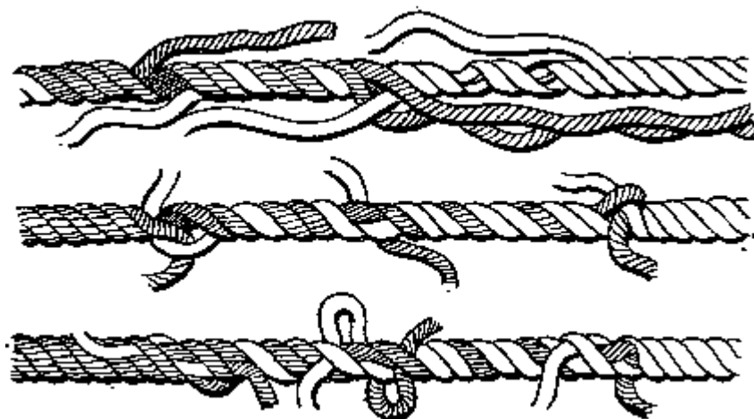
Рис. 64. Лонгосплесень (длинный сплесень)
