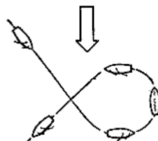
Рис. 111. Поворот «коровий оверштаг»
