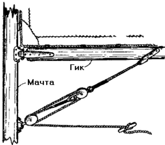
Рис. 113. Оттяжка гика
