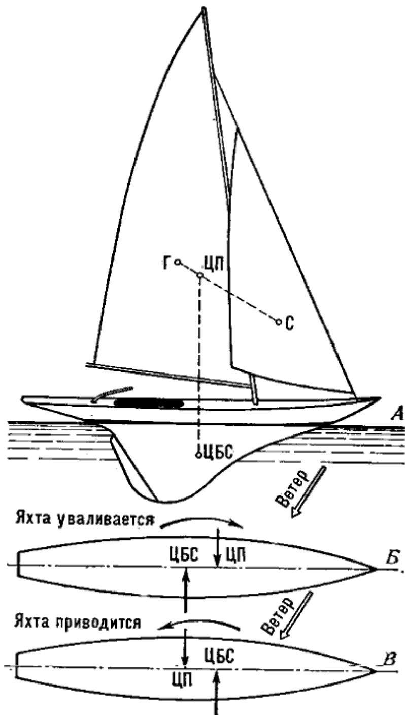
Рис. 99. Центровка яхты
