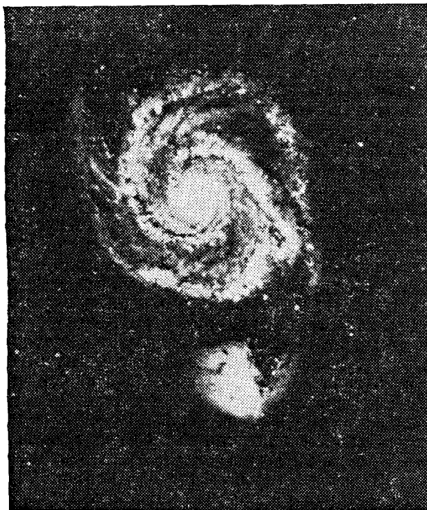
Рис. 2.9. Фотография галактики М 51.
