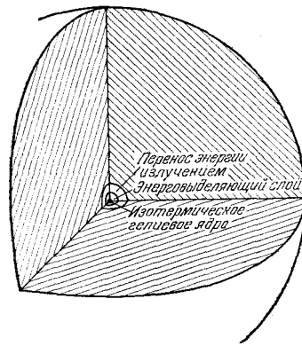
Рис. 11.4. Модель красного гиганта.
