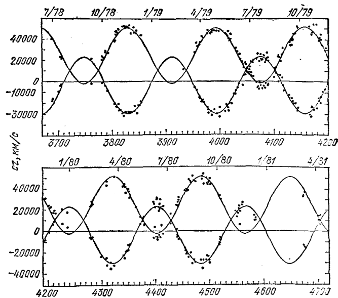
Рис. 23.13. Кривая лучевых скоростей для «красной» и «фиолетовой» компонент SS 433. По оси абсцисс внизу отложены даты в юлианских днях, вверху — даты обычного календаря.
