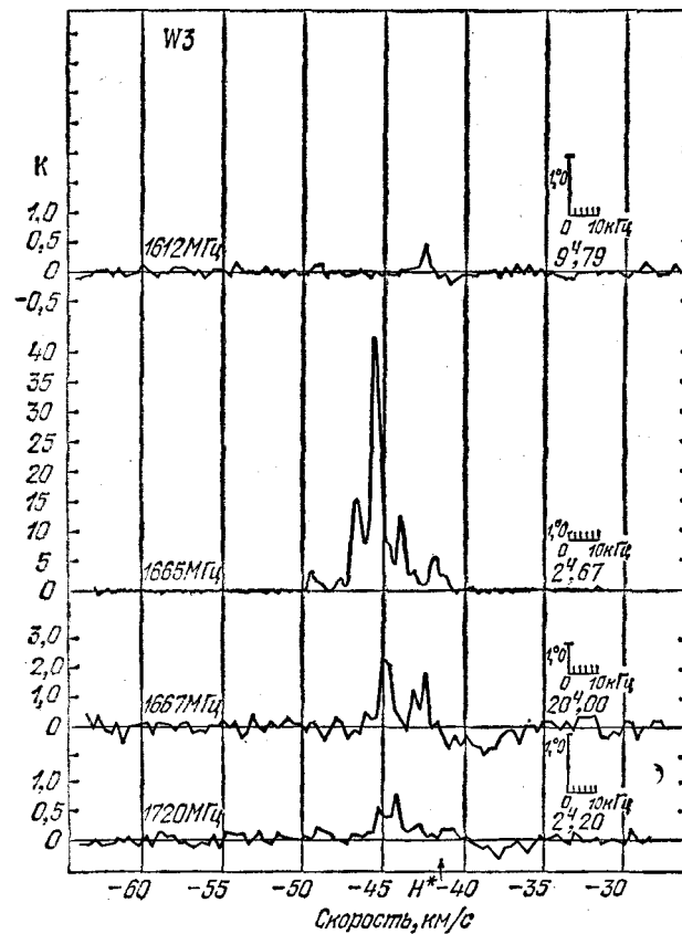
Рис. 4.1. Профили радиолиний мазерного излучения от молекулы ОН от источника, находящегося в туманности W 3.
