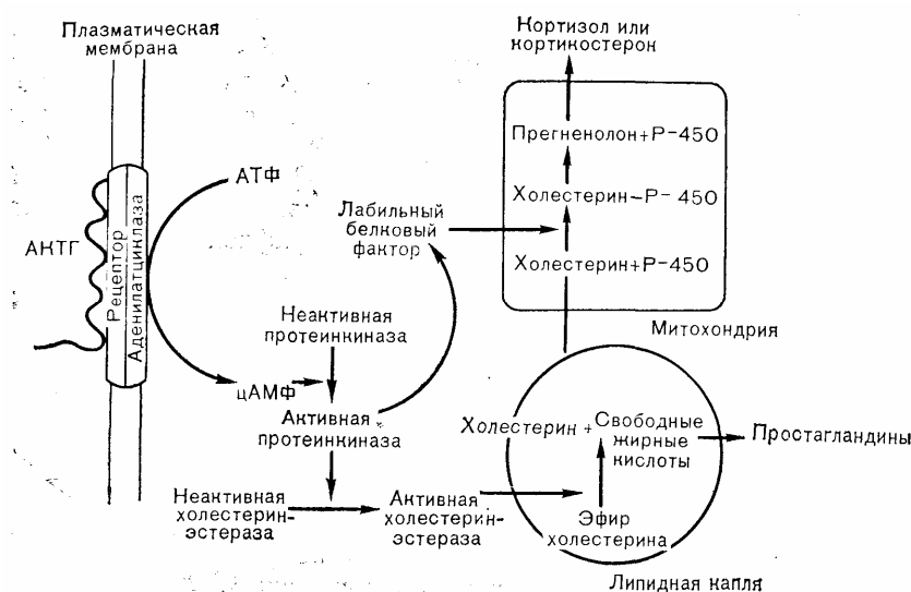
Рис. 3—20. Предполагаемый механизм действия АКТГ на клетку коры надпочечника. Согласно этой модели, АКТГ не проникает в клетку, а стимулирует продукцию второго медиатора—цАМФ—путем активации
