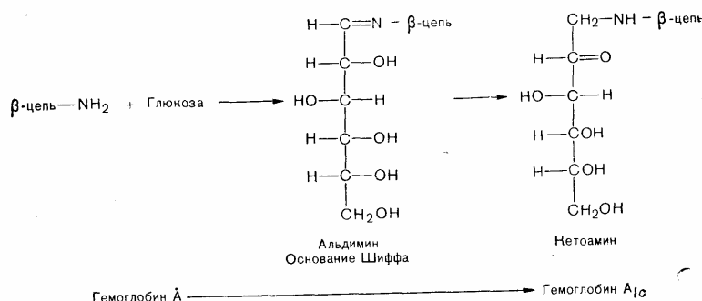
Рис. 10—45. Химические реакции, приводящие к неферментативному превращению гемоглобина А (HbA) в гликозилированный HbA 1c . В первой реакции аминоконцевая (валин) аминогруппа β-цепи HbA конденсируется с глюкозой, образуя основание Шиффа. Затем оно подвергается перегруппировке Амадори с образованием более стабильного кетоаминного основания Шиффа. тическую модификацию различных белков, включающих, возможно, белки базальной мембраны и миелина периферических нервов.
