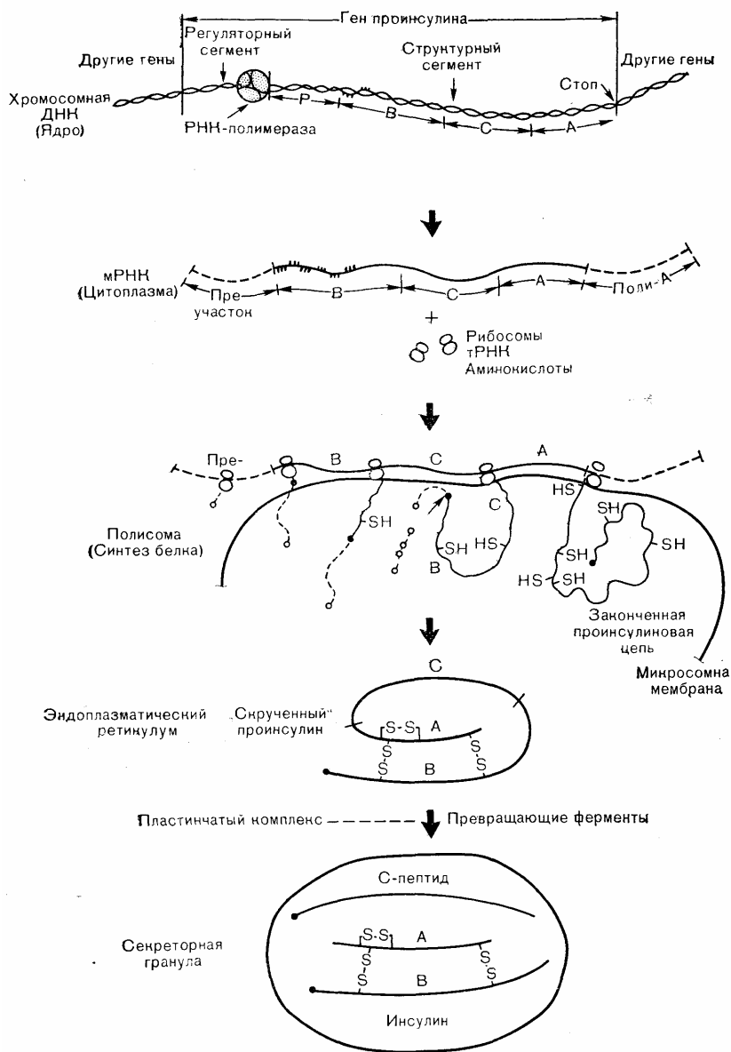
Рис. 10—11. Схематическое изображение биосинтеза проинсулина, его превращения в инсулин и С-пептид. Ген проинсулина представлен в верхней части рисунка. Эти гены содержат интроны, продукты которых исключаются из состава зрелой мРНК. Транскрипция препроинсулиновой мРНК требует присутствия фермента РНК-полимеразы. Эта мРНК служит матрицей для образования цепей препроинсулина на полирибосомах. Препроинсулин расщепляется до проинсулина (средняя часть рисунка), который затем переносится в аппарат Гольджи (пластинчатый комплекс), где и происходит его превращение в инсулин (по Steiner D. F., Diabetes, 1977, 26, 322). раздо больше. Так, инсулин свиньи отличается от инсулина человека только одной аминокислотой, тогда как С-пептид человека — цепь из 23 аминокислотных остатков с молекулярной массой 3021 — отличается от свиного С-пептида 10 остатками и содержит на 2 аминокислоты меньше [30]. Столь высокая «мутабельность» согласуется с отсутствием у С-пептида специфической гормональной функции. Хотя проинсулин обнаруживает небольшую перекрестную реакцию с антителами к инсулину, он обладает всего" 3—5% от биологической эффективности нативного инсулина, Не ясно, принадлежит ли эта небольшая биологическая, активность непосредственно проинсулину, или она обусловлена его превращением тканями-мишенями в инсулин.
