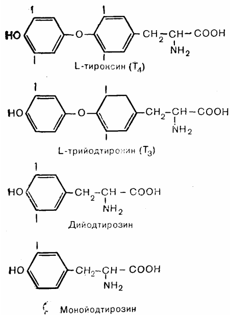
Рис. 3—9. Структура некоторых тиреоидных гормонов (Ingbar S.H., Woeber K.A. In: Textbook of Endocrinology/Ed. Williams R.H. 5th ed.— Philadelphia: Saunders, 1974).
