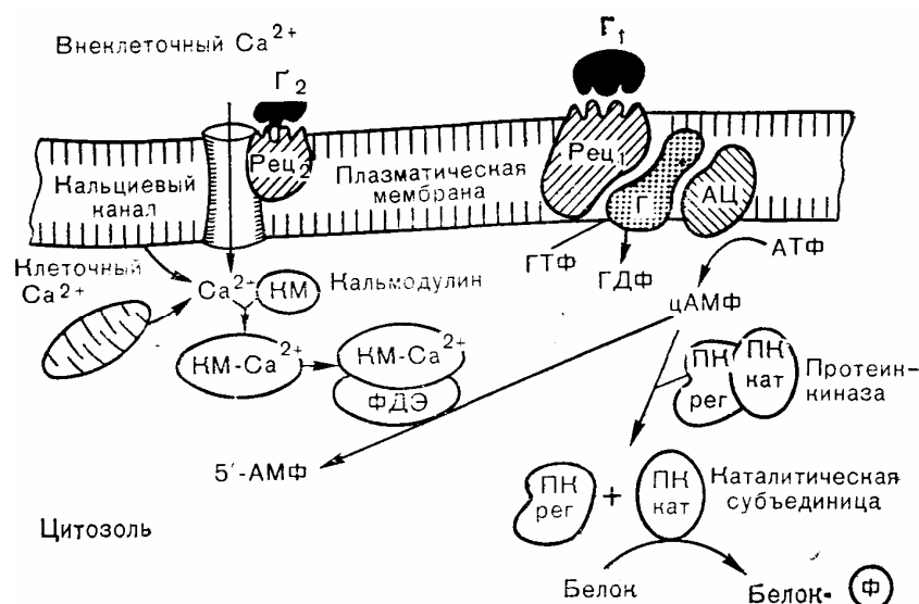
Рис. 4—19. Взаимоотношения между путями активации, «запускаемыми» гормональными рецепторами и связанными с мобилизацией кальция и аденилатциклазой. Этот пример подчеркивает роль \text{Ca}^{2+} -кальмодулина в определении скорости разрушения циклического нуклеотида фосфодиэстеразой. Другие области взаимодействия между двумя системами показаны на рис. 4—13, 4—15, 4—17 и 4—18 (Schulster, Levitski [45в] в модификации).
