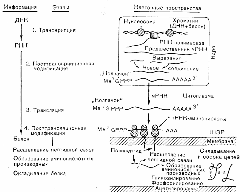
Рис. 3—1 Схема синтеза белка, демонстрирующая этапы переноса генетической информации от ДНК к РНК и белку. Схема специально предусматривает путь биосинтеза секретируемых белков, посттрансляционная модификация которых происходит в месте их синтеза в шероховатом эндоплазматическом ретикулеуме (ШЭР) (Habener, Potts [4]).
