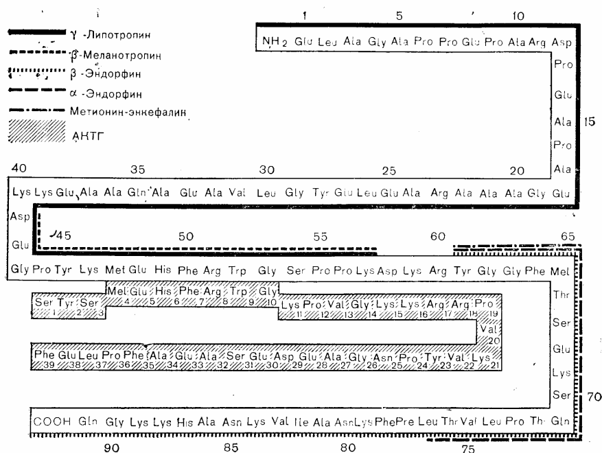
Рис. 6—8. Структурные соотношения между АКТГ, меланотропином, липотропинами, эндорфинами и энкефалинами. Приведенная 91 последовательность аминокислот отражает структуру (3-липотропина; а-МСГ включает 1—13 последовательности АКТГ. Гомологичные последовательности АКТГ и липотропина показаны лишь схематически; это не отражает их реального структурного соотношения в молекуле массой в 31000 дальтон, являющейся общим предшественником обоих пептидов.
