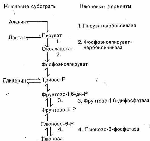
Рис. 10—4. Глюконеогенез. Основные субстраты глюконеогенеза и ключевые ограничивающие скорость ферментативные стадии.
