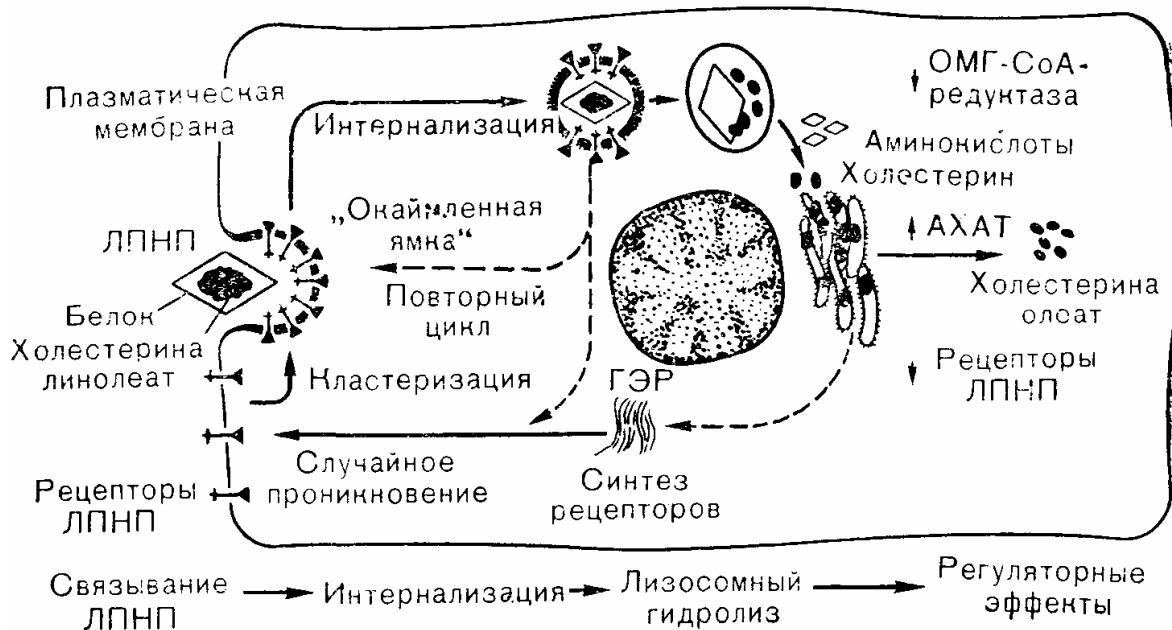
Рис. 4—8. Способ поглощения липопротеинов низкой плотности (ЛПНП) культивируемыми фибробластами. Считают, что рецепторы ЛПНП, синтезируемые на полирибосомах, в случайном порядке проникают в клеточную мембрану и непрерывно подвергаются кластеризации в «окаймленных ямках», сменяемой интернализацией в составе эндоцитозных пузырьков. После отложения ЛПНП в лизосомах рецепторы, по-видимому, используются в новом цикле, возвращаясь на клеточную поверхность, где они вновь подвергаются кластеризации в «окаймленных ямках». Поступающий холестерин подавляет образование микросомального фермента (ОМГ-СоА-редуктазы), который лимитирует скорость биосинтеза холестерина, стимулирует фермент, ответственный за синтез эфиров холестерина и угнетает синтез рецепторов ЛПНП (Brown, Goldstein [23] в модификации). ГЭР — гладкий эндоплазматический ретикулум.
