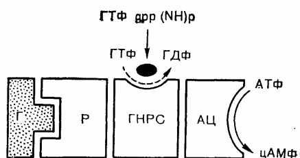
Рис. 4—4. Трехкомпонентная модель системы гормональный рецептор (P) — аденилатциклаза. Гормон-рецепторный комплекс модулирует ГТФ-связывающую активность гуанилнуклеотид регуляторной субъединицы (ГНРС), в свою очередь активирующей аденилатциклазу (АЦ). Вызываемая гормоном (Г) активация комплекса ГТФ-ГНРС прекращается после гидролиза ГТФ на регуляторной субъединице или вблизи ее.
