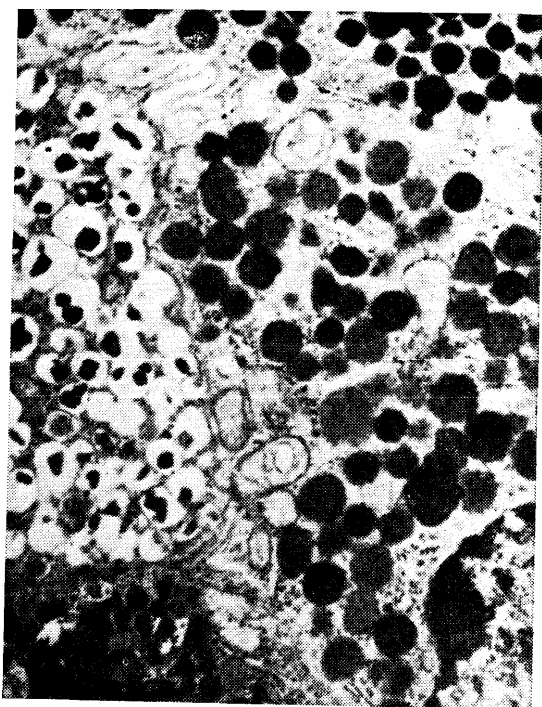
Рис. 10—1. Электронная микрофотография участка неизмененного островка поджелудочной железы (человека), содержащего \beta -, \alpha - и \delta -клетки. В секреторных гранулах \beta -клеток (справа вверху) можно видеть плотную центральную часть и бледно окрашенную периферию. В \alpha -клетках (слева) содержатся плеоморфные гранулы с кристалловидным матриком. В \delta -клетках (в центре) секреторные гранулы гомогенны и заполняют пузырьки. Видна также \delta -клетка с гранулами, содержащими, как полагают, гастрин (по Lucy P. E., Creider M. J. — In: DeGroot L. J. et al. (eds). Endocrinology , vol. 2. New York, Grune a. Stratton 1979).
