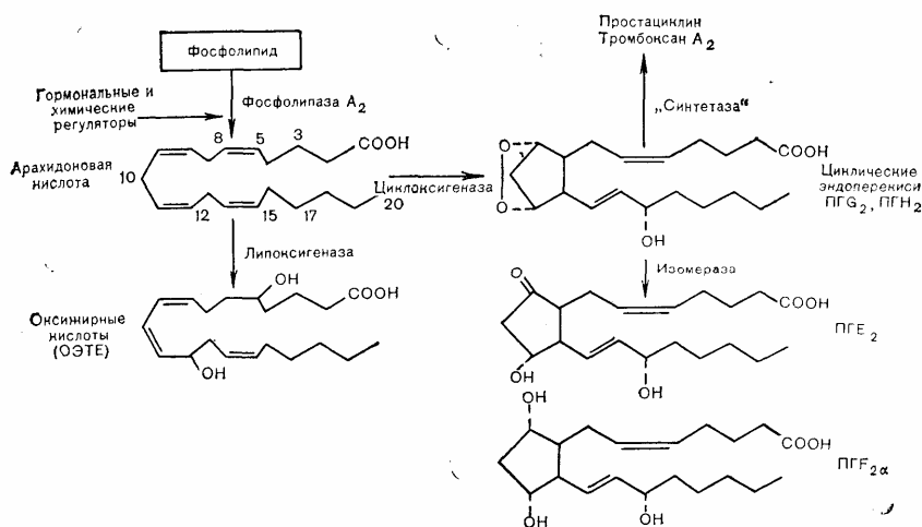
Рис. 4—22. Образование и метаболизм арахидоновой кислоты. Ненасыщенная жирная кислота, высвобождаемая фосфолипазой А 2 из мембранных фосфолипидов, превращается в активные производные в ходе липоксигеназного, циклоксигеназного и простагландинсинтетазного ферментативных процессов.
