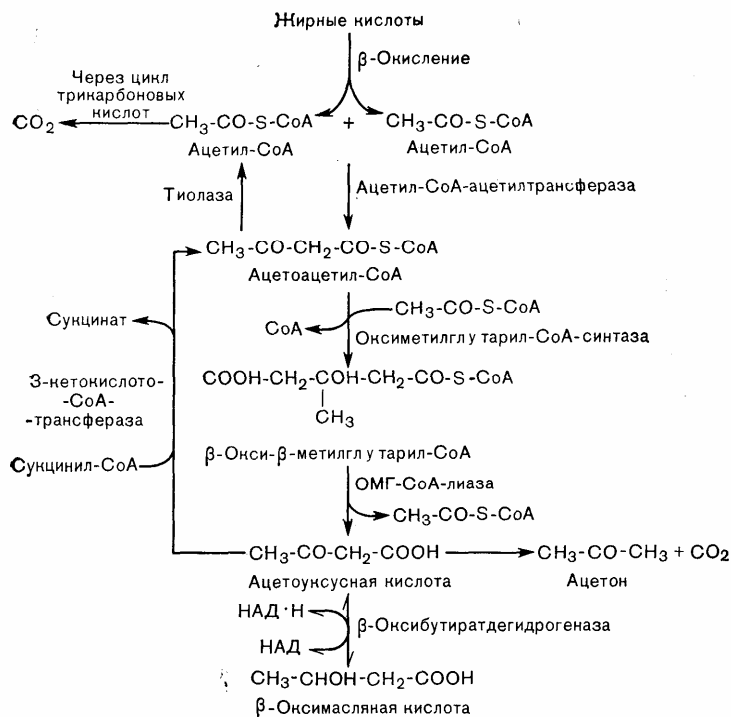
Рис. 10—7. Метаболические пути образования кетонных тел (ацетоуксусной и β-оксималяной кислоты) из ацетил-СоА и их окисления до CO 2 . Ограничивающая скорость стадия образования кетонов предшествует образованию ацетил-СоА и локализуется на этапе переноса жирного ацил-СоА через митохондриальную мембрану к месту расположения ферментов, участвующих в β-окислении (см. рис. 10—8). Образование ацетоуксусной кислоты из ацетоацетил-СоА требует вначале образования β-окси-β-метилглутарил-СоА.
