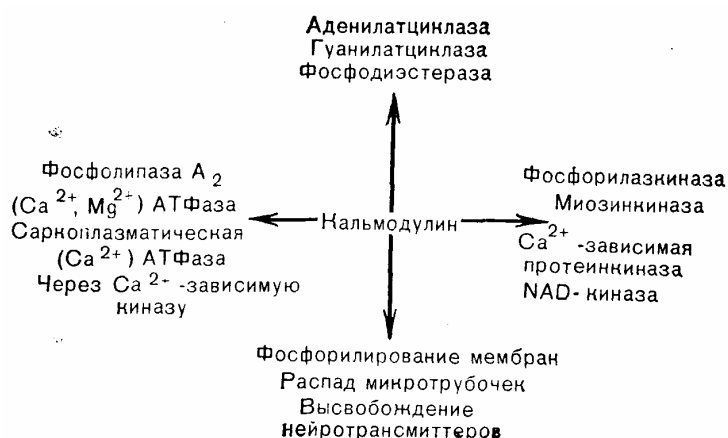
Рис. 4—16. Ферменты и клеточные процессы, регулируемые кальмодулином (Cheung в модификации).
