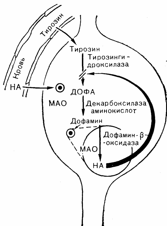
Рис. 3—14. Биосинтез норадреналина в симпатическом нерве (Axelrod J., Kopin I.J. Prog. Brain. Res., 1969, 31, 21).
