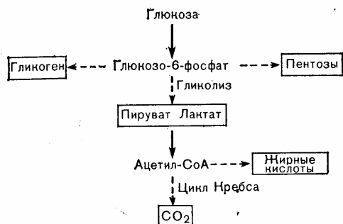
Рис. 10—2. Основные пути метаболизма глюкозы у человека. вращение в жирные кислоты и накопление в виде триглицеридов (синтез жира); 5—высвобождение из клетки в виде свободной глюкозы.
