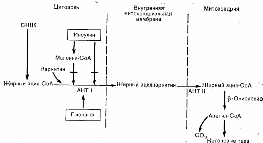
Рис. 10—8. Внутрипеченочная регуляция кетогенеза. Главным ограничивающим скоростью этапом является перенос жирных ацильных производных через митохондриальную мембрану, осуществляемый ферментами ацилкарнитинтрансферазой (АКТ) I и II. АКТ I тормозится при повышении уровня инсулина, уменьшающего доступность карнитина и увеличивающего доступность малонил-СоА—прямого ингибитора АКТ I. Наоборот, снижение уровня инсулина и повышение уровня глюкозагона приводит к увеличению содержания карнитина, снижению содержания малонил-СоА и повышению активности АКТ-I (по McGarry J. D., Diabetes, 1979, 28, 517, с модификациями). СЖК — свободные жирные кислоты.
