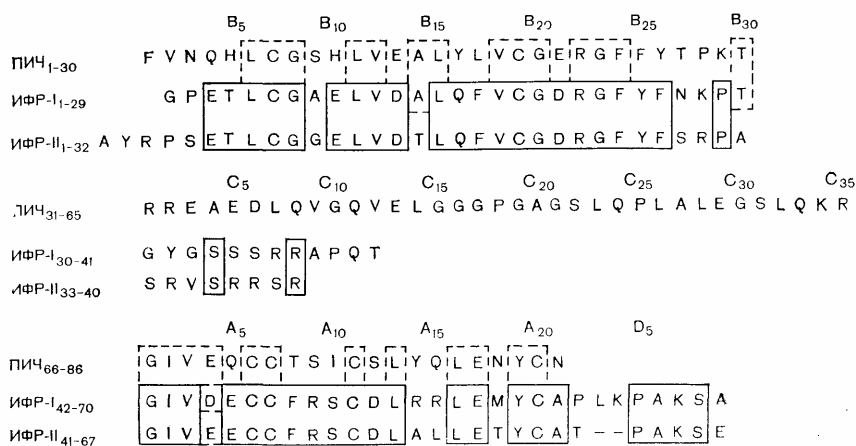
Рис. 10—24. Первичная структура проинсулина человека (ПИЧ) и инсулиноподобных факторов роста (ИФР) I и II. Участки, ограниченные сплошными линиями, включают одинаковые аминокислотные остатки в ИФР I и II; участки, ограниченные пунктирными линиями, включают аминокислотные остатки, одинаковые в ПИЧ и ИФР I и/или II (по Zapf J. et al., Metabolism, 1978, 27, 1803).
