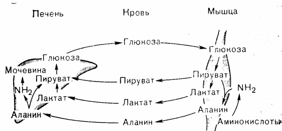
Рис. 10—5. Цикл Кори (лактат \leftrightarrow глюкоза) и глюкозоаланиновый цикл. В обоих циклах глюкоза поглощается мышцей и превращается в пируват и лактат. Часть пирувата в мышце подвергается аминированию с образованием аланина. Образующиеся из глюкозы лактат и аланин в печени вновь превращаются в глюкозу.
