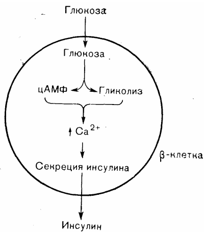
Рис. 10—14. Внутриклеточная последовательность стимулирующего эффекта глюкозы на секрецию инсулина \beta -клеткой. Проникновение глюкозы в \beta -клетку усиливает гликолиз и повышает уровень цАМФ. Эти сдвиги приводят к увеличению внутриклеточного содержания кальция, «запускающего» выброс инсулина.
