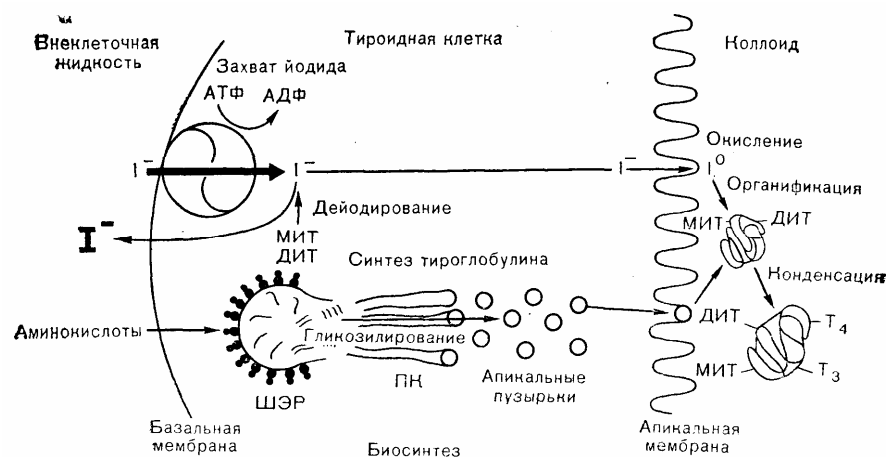
Рис. 3—10. Схематическое изображение пути биосинтеза тиреоидных гормонов в клетке. Т 3 и Т 4 образуются и хранятся связанными с тироглобулином в коллоиде.
