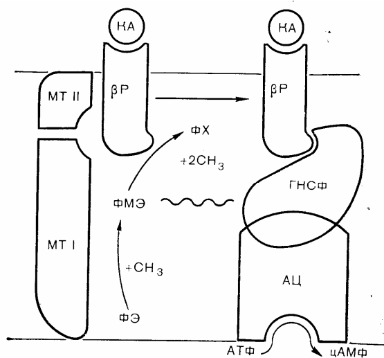
Рис. 4—24. Механизм действия катехоламинов (КА) на метилирование фосфолипидов и мобильность \beta -адренергических рецепторов (Р). Предполагают, что повышение текучести мембраны облегчает взаимодействие рецепторов с гуанилнуклеотидсопрягающим фактором (ГНСФ) и аденилатциклазой (АЦ) (Hirata, Axelrod [68]).
