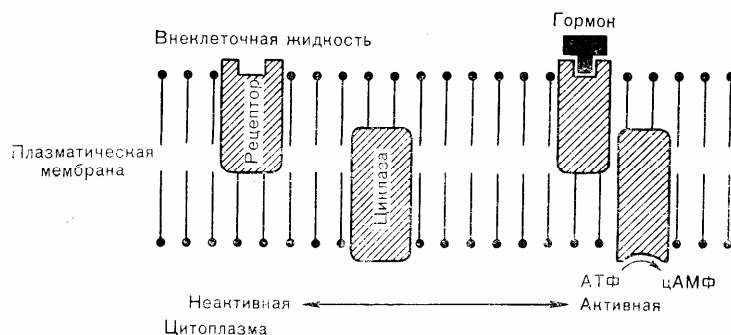
Рис. 4—3. «Плавающий рецептор»—двухступенная физическая модель взаимодействия пептидного гормона с рецептором и активации аденилатциклазы в клеточной мембране.
