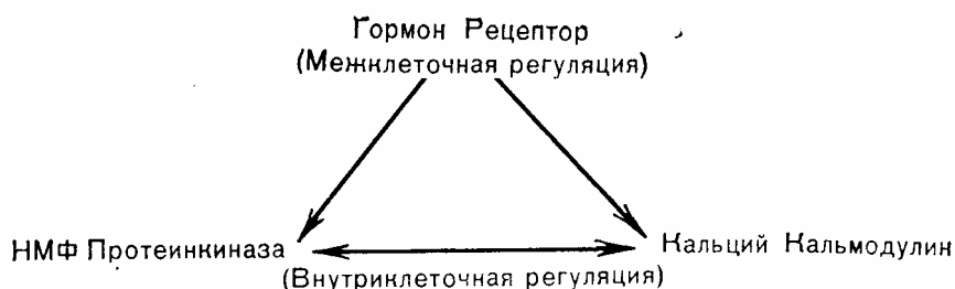
Рис. 4—15. Общая связь между главными межклеточными и внутриклеточными регуляторными лигандами и их рецепторными белками, т. е. пептидными гормонами, кальцием и циклическими нуклеотидмонофосфатами (цНМФ). Взаимодействие между этими медиаторами затрагивают их метаболизм и функции, равно как и их комплементарные роли в отношении скорости, расстояния и продолжительности действия (Cheung f55] в модификации).
