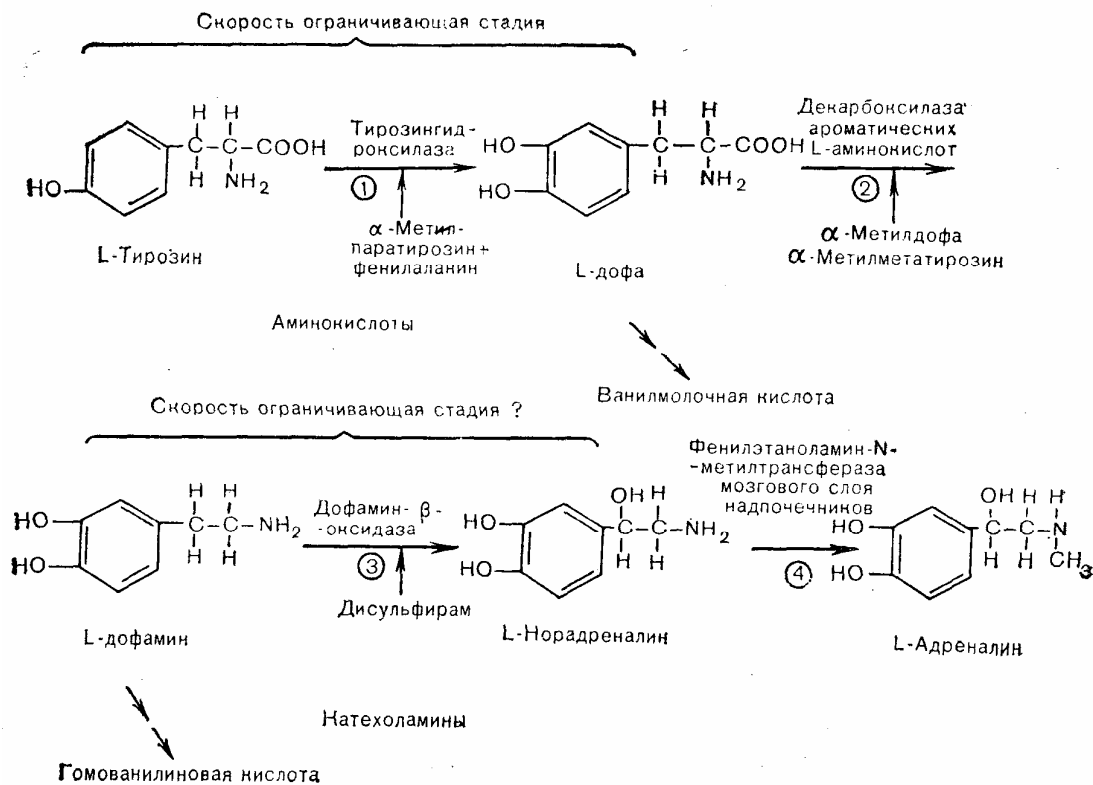
Рис. 3—13. Этапы биосинтеза катехоламинов в окончаниях симпатических нервов, мозговом слое надпочечников и головном мозге. Скорость ограничивающими этапами в процессе биосинтеза являются стадия 1 и, возможно, стадия 3. Вертикальные стрелки обозначают торможение отдельных этапов (Melmon K.L. — In: Textbook of Endocrinology/Ed. Williams R.H. 5 th ed. — Philadelphia: Saunders, 1974).
