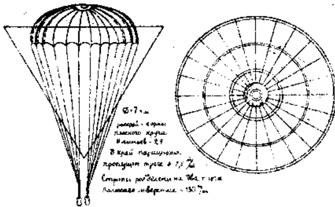
Рис. 161. Первый ранцевый парашют, изобретенный Г. Е. Котельниковым в 1911 г.
