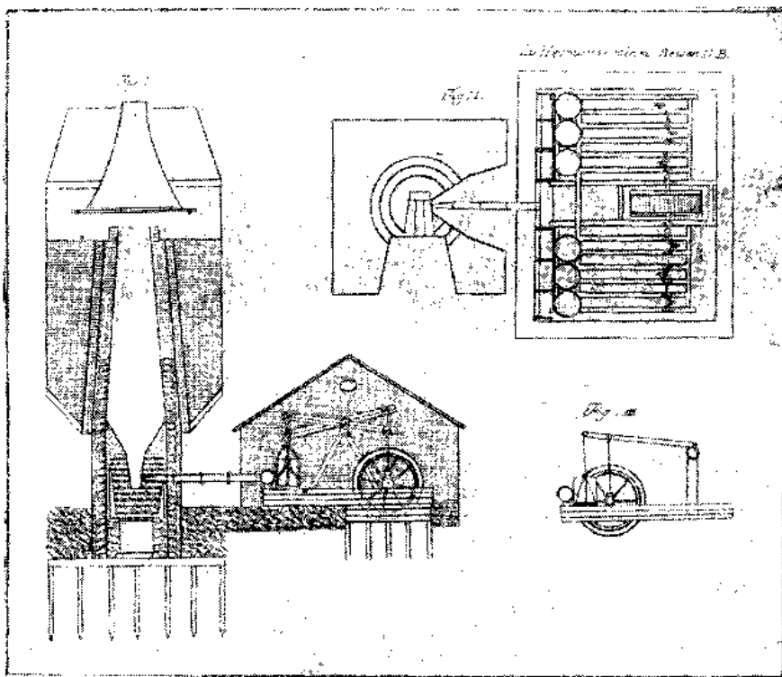
Рис. 25. Русские доменные печи—величайшие в мире—в конце XVIII века.— По чертежу в книге Германа „Минералогическое путешествие“, изданной на рубеже XVIII—XIX вв. в Вене и Петербурге.
