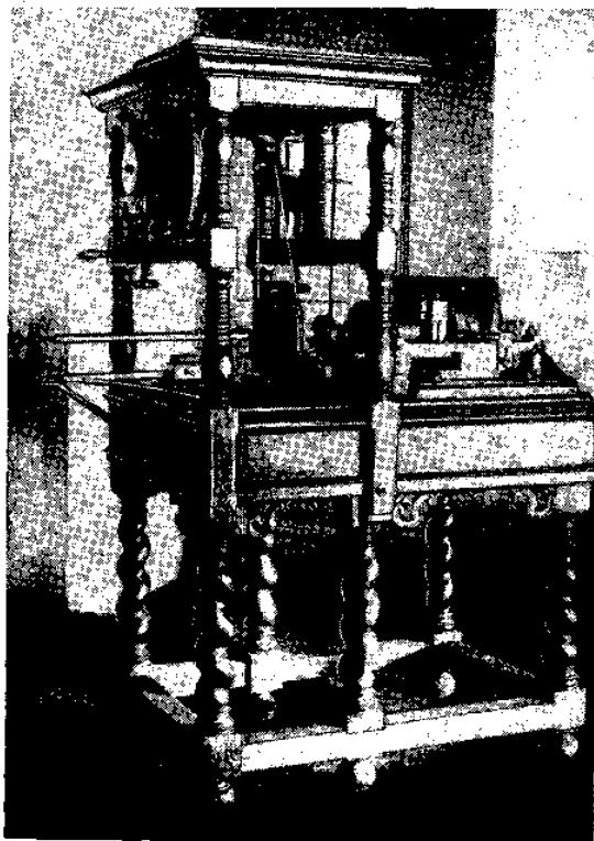
Рис. 44. Петровский токарно-копировальный станок с механическим суппортом.
