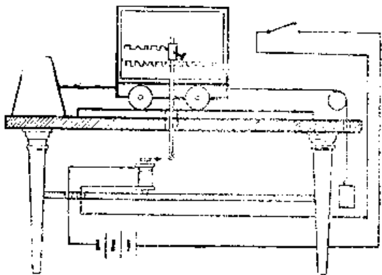
Фиг. 126. Схема электромагнитного телеграфа Б. С. Якоби, действовавшего в 1839 г. на линии Царское Село — Петербург.
