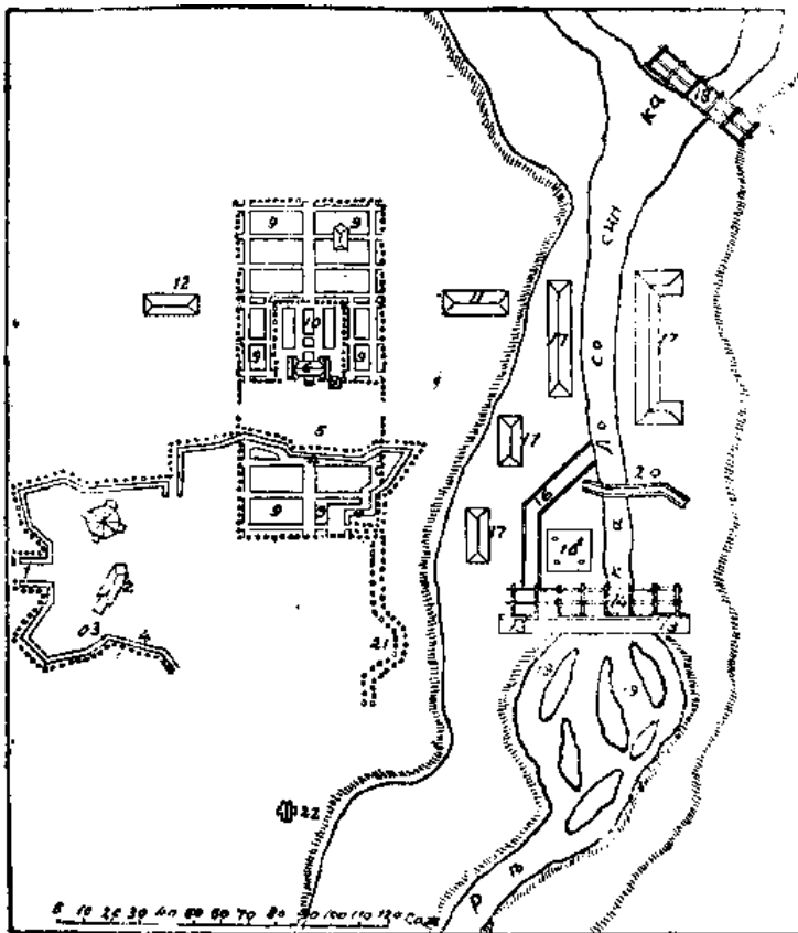
Рис. 103. Петровский завод. — По чертежу, составленному в 1819 г. 1 — ворота; 2 — церковь; 3 — могила „блаженного“ Фаддея; 4 — земляной вал с палисадом; 5 — парадное место при дворе; 6 — двор; 7 — склад; 8 — роща; 9 — пруд; 10 — пруд; 11 — квадратский дом; 12 — гауптвахта; 13 — мост через плотину; 14 — верхняя плотина; 15 — „доменный корпус о четырех печах“; 16 — „русло для действия завода“; 17 — молотовая, кузница, якорная и др.; 18 — нижняя плотина (в 100 саженах от Онежского озера); 19 — заводский пруд; 20 — мост через Лососинку; 21 — место для тюрьмы; 22 — лефортов дом.
