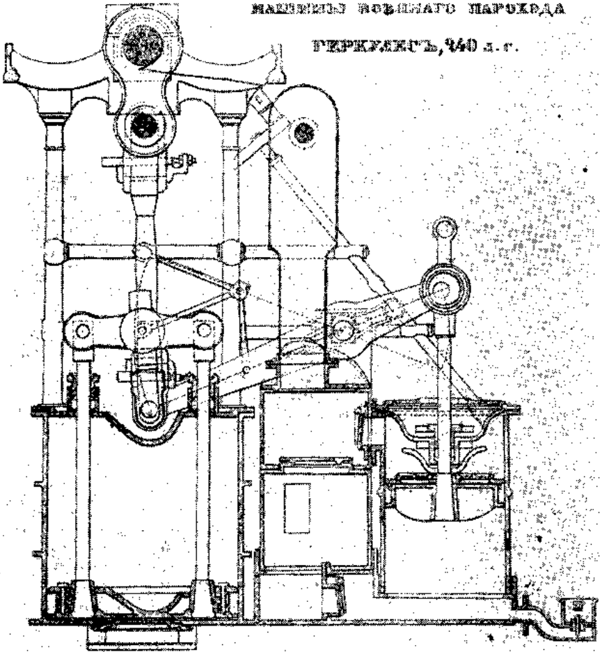
Рис. 68. Первая паровая машина без балансира. Русский военный пароход „Геркулес“, 1832 г.
