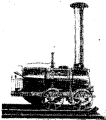
Рис. 71. Паровоз Ефима Алексеевича и Милоша Ефимовича, Черепановых, построенных в 1833—1835 гг. на Нижне-Тагильских заводах первые русские паровозы. — Модель в Музее железнодорожного транспорта, Ленинград.
