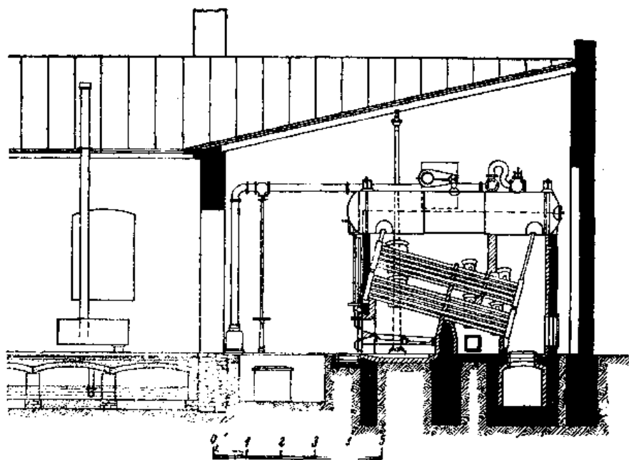
Рис. 146. Машинная и котельная установки центральной электрической станции на Васильевском острове в Петербурге, построенной в 1894 г. русскими инженерами Н. П. Булангиным и Н. В. Смирновым. — Из доклада Ч. Скрипниченко I Всероссийскому электротехническому съезду „О Васильевской центральной электрической станции инженера Н. В. Смирнова, построенной на 800 киловатт, как о типе станций подобной величины“, 9 января 1900 г.
