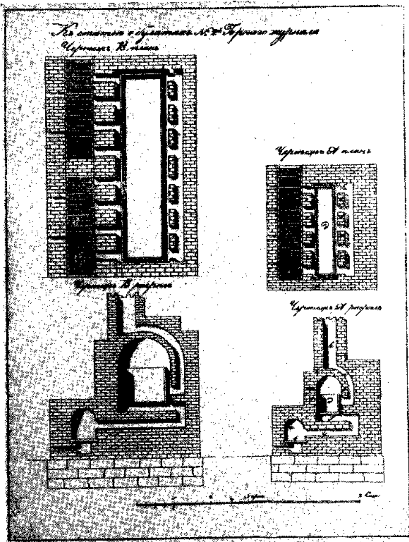
Рис. 37. Чертежи печей для производства булата. Из работы П. П. Аносова: О булатах, 1841 г. (опубликовано в «Горном журнале» и отдельной книгой).
