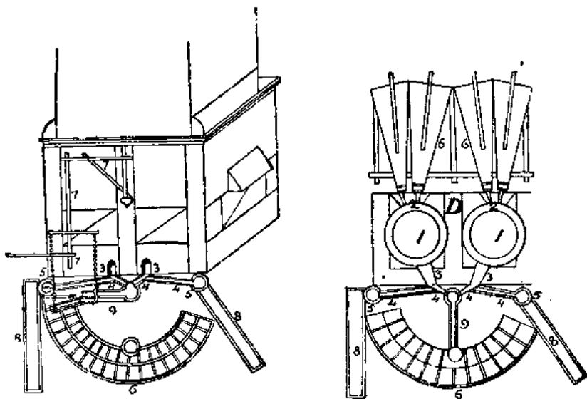
Рис. 24. Механизация разлива цветных металлов на Сузунском заводе. — По рисунку 1798 г. Центральный Государственный исторический архив в Ленинграде. 1 — под печи; 2 — фурмы; 3 — отверстия для выпуска металла; 4 — желоба; 5 — „ямки“; 6 — иважиницы, расположенные по дуге для удобства разлива в них металла; 7 — подъемный кран; 8 — „сковороды для разбегания через ямки штейну“; 9 — желоб для разлива
