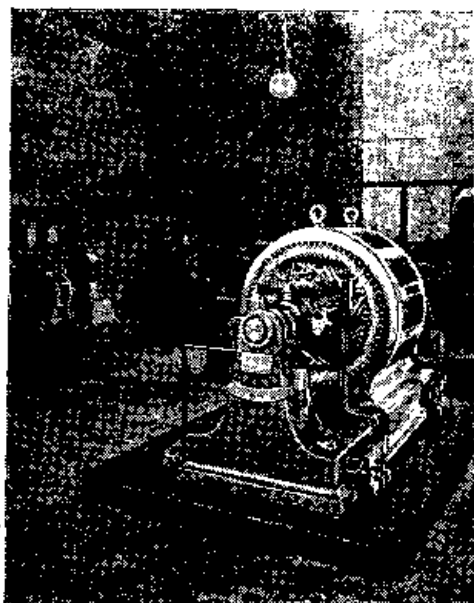
Рис. 139. Первая в мире передача переменным током, созданная русским инженером М. О. Доливо-Добровольским в 1891 г. Диния Лауфен—Франкфурт. На фотографии показано помещение выставки, в котором установлен электромотор переменного тока, изобретенные Доливо-Добровольским и действовавшие за счет электрического тока, передававшегося из Лауфена во Франкфурт.
