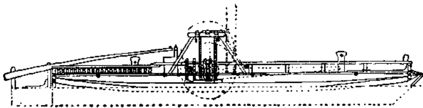
Рис. 61. «Водоход» И. П. Кулибина (1782 — 1804).
