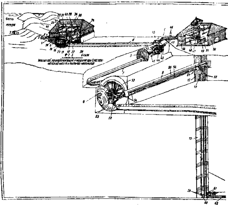
Рис. 109. Подземная гидростатическая установка К. Д. Фролова на Змеиногорском руднике, устроенная в 80-х годах XVIII века. — Центральный Государственный исторический архив в Ленинграде.
