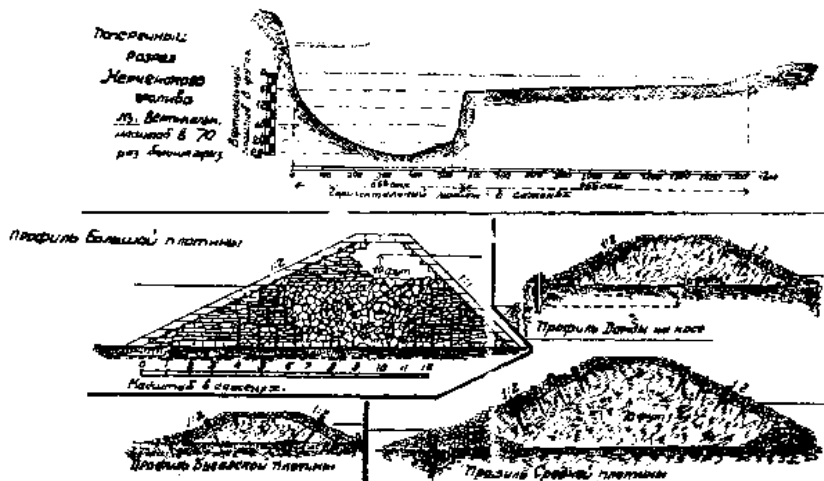
Рис. 116. Разрезы плотин и дамбы в Керченском проливе для подъема уровня Азовского моря. — Из книги В. Д. Менделеева: Проект поднятия уровня Азовского моря запрудой Керченского пролива, 1899 г.
