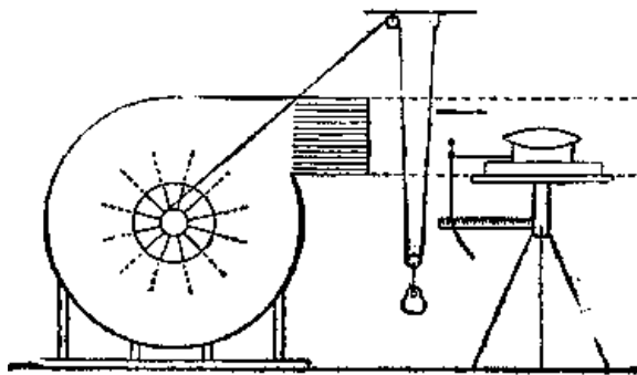
Рис. 159. Авродинамическая труба К. Э. Циолковского в 1896 г.
