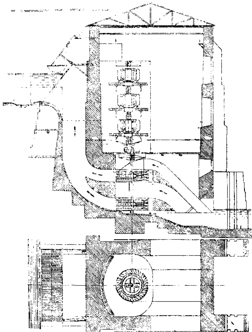
Рис. 145. Проект машинного здания гидроэлектрической станции на р. Волков, разработанный в 1894 г. инженером В. Ф. Добротворским. На общем валу по две группы турбинных колес и по три электрогенератора. Общая мощность станции, с установленными 18 турбинами (и 2 запасными) по 2082 лощ. сил., составляет 37 476 лощ. сил.; 1894 г. — Из доклада В. Ф. Добротворского I Всероссийскому электротехническому съезду: „Электропередачи силы порогов Волкова. Наровы, Вуоксы в С.-Петербург“. 29 декабря 1899 г.
