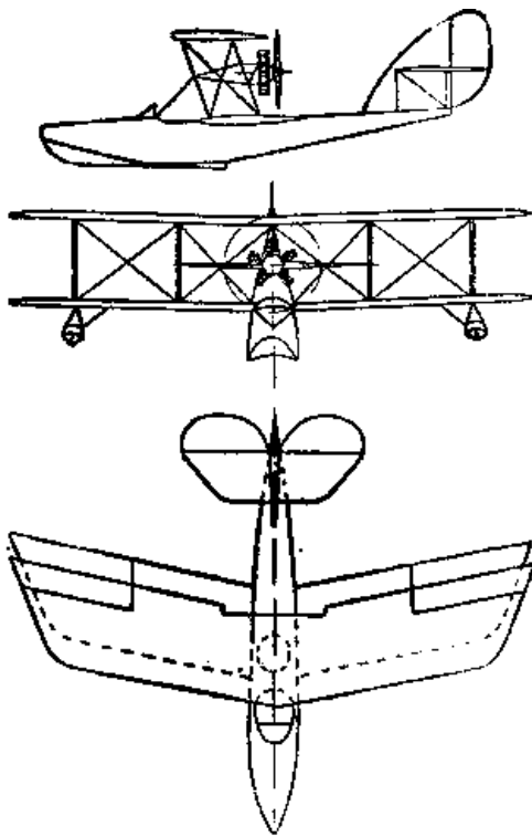
Рис. 163. Летаящая лодка М-5, созданная Д. П. Григоровичем, построившим свой первый гидросамолет в 1913 г.
