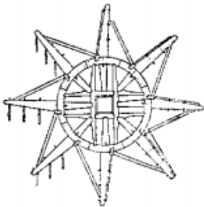
Рис. 62. Колесо «водохода» И. П. Кулибина.
