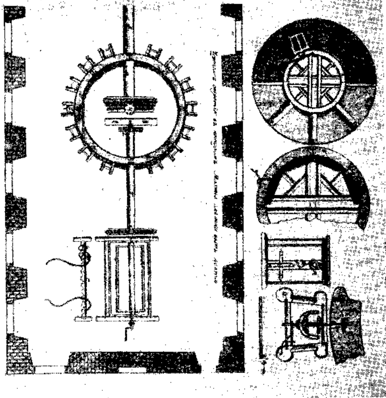
Рис. 55. „Чертеж строения, в котором машина сделана быть должна“ детали при- анально-часовой машины Р. Глинкова. — По рисунку 1771 г.
