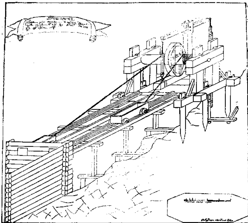
Рис. 48. „Пропспект, сочиненный для постройки на Чагирском руднике для спуска с горы руды в анбар, сего 1752 году февраля месяца“, Алтай. — Новосибирский областной государственный архив.
