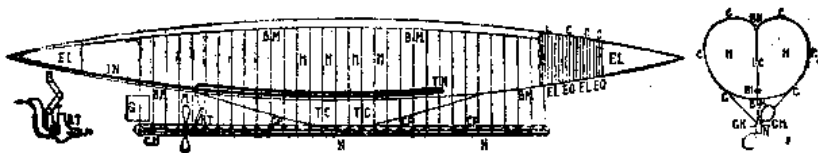
Рис. 156. Проект цельнометаллического дирижабля, разработанный К. Э. Циолковским.
