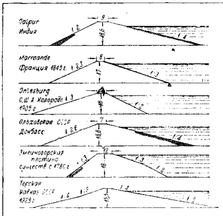
Рис. 108. Профиль Эмичоворской плотины, построенной К. Д. Фроловым около 1780 г., и профили современных земляных плотин того же типа, сооруженных примерно из одинакового материала и работающих при напорах порядка 15—18 метров
