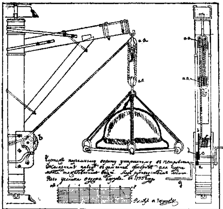
Рис. 57. «Чертеж подъемному вороту, устроенному в Петровском железном заводе в доменной фабрике для поднимания тяжелых вещей. Под руководством машинного ученика Федора Борзова, в 1793 году». — Новосибирский областной государственный архив.
