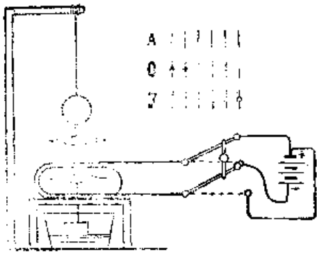
Рис. 125. Схема первого примененного для практических потребностей электрического телеграфа, изобретенного П. А. Шиллингом и действовавшего в 1832 г. в Петербурге на линии Зимний двор — министерство путей сообщения
