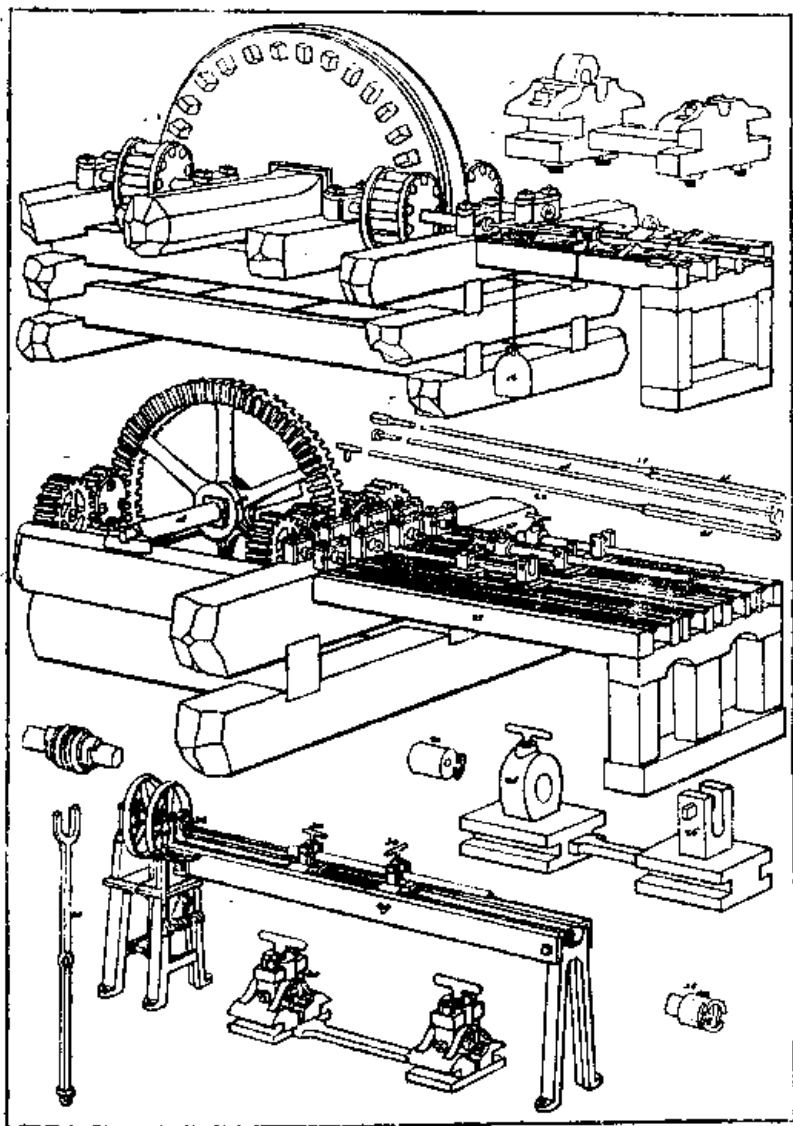
Рис. 73. Тульские станки для сверления стволов. — По книге И. Гамселя: «Описание Тульского оружейного завода», 1826 г.
