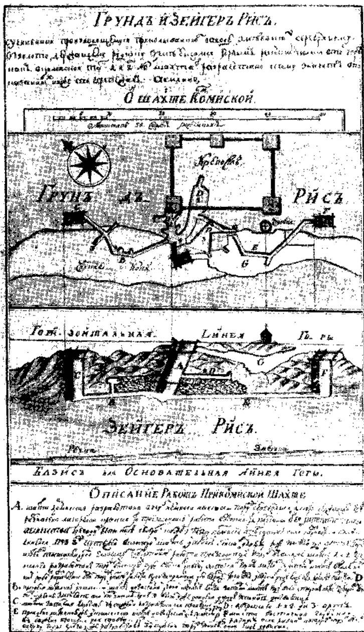
Рис. 13. План и разрез Зеннергорского «серебро-и золотодержащего» рудника на Алтае, около 1748 г. — Центральный Государственный исторический архив в Ленинграде.
