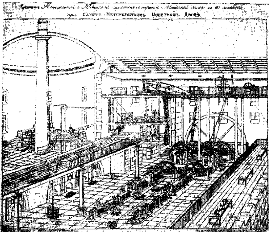
Рис. 69. „Плющильная и юстировая палаты с паровой машиной силою в 60 лошадей, при Санкт-Петербургском монетном дворе“. Паровая машина построена в 1820 г. — По Григорию Славскому.
