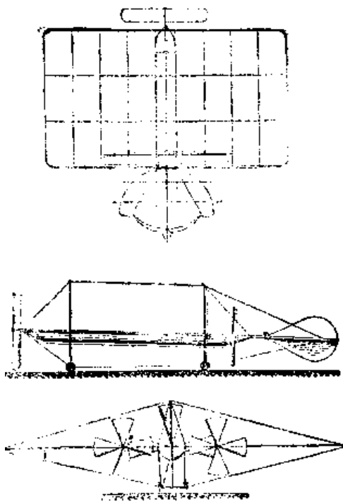
Рис. 137. Проект самолета, разработанный А. Ф. Можайским в 1878 г. — По рисунку в привилегии, выданной изобретателю в 1881 г.
