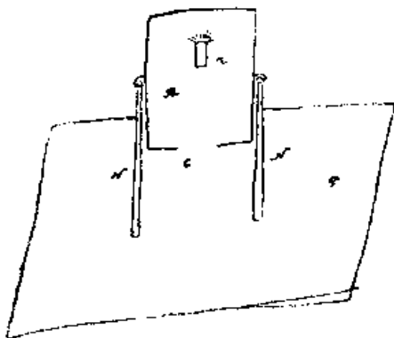
Рис. 165. Чертеж реактивного летательного аппарата Н. И. Кибальчича, 1881 г. А — цилиндр; С — выхлопное отверстие; К — пороховая свеча; NN — стойки; P — платформа для подъема.
