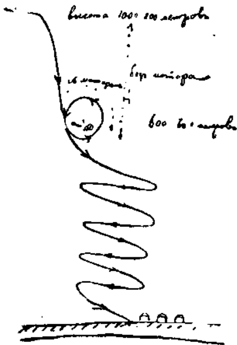
Рис. 164. Трассятория первой в мире мертвой петли, совершенной П. Н. Нестеровым в Киеве 27 августа 1913 г. — Чертеж П. Н. Нестерова.
