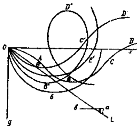
Рис. 152. Графия Н. Е. Жуковского, доказавшие возможность осуществления мертвой петли, 1891 г.
