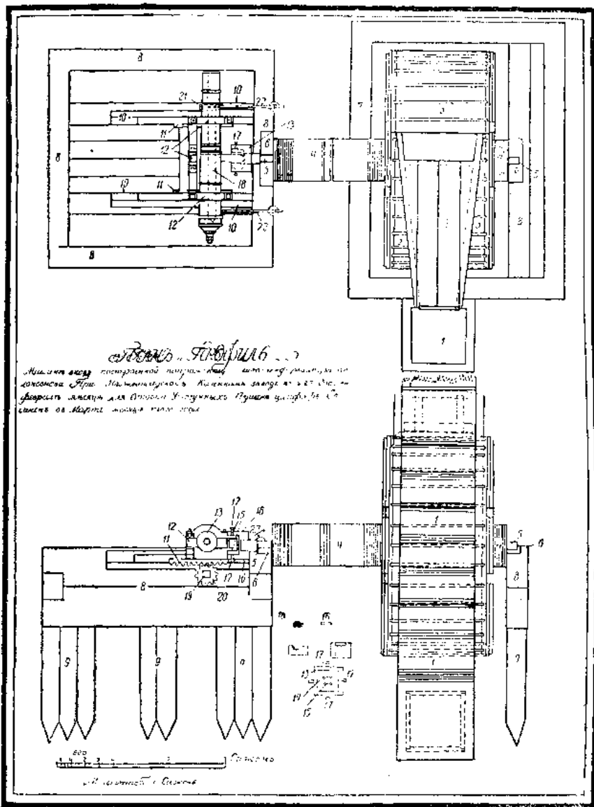
Рис. 64. Машина для обточки цапф у пушек, изобретенная Подоксоновым в 1812 г. на Нижне-Исетском заводе. — Свердловский областной государственный архив
