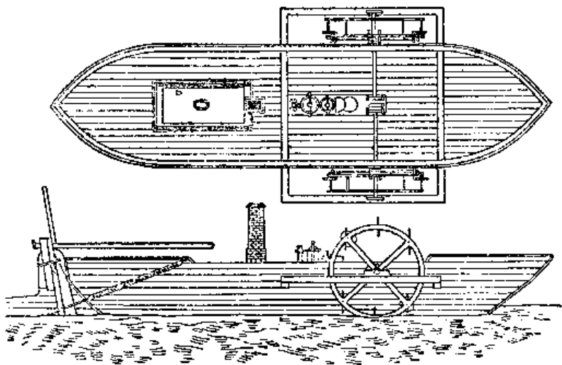
Рис. 66. Первый русский пароход „Елизавета“. Линия: Петербург — Кронштадт. 1815 г.
