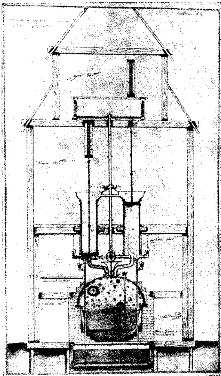
Рис. 51. Поперечный разрез первой заводской паровой машины, изобретенной И. И. Подуновым в 1763 г. и построенной в 1764—1765 гг. — Центральный Государственный исторический архив в Ленинграде.
