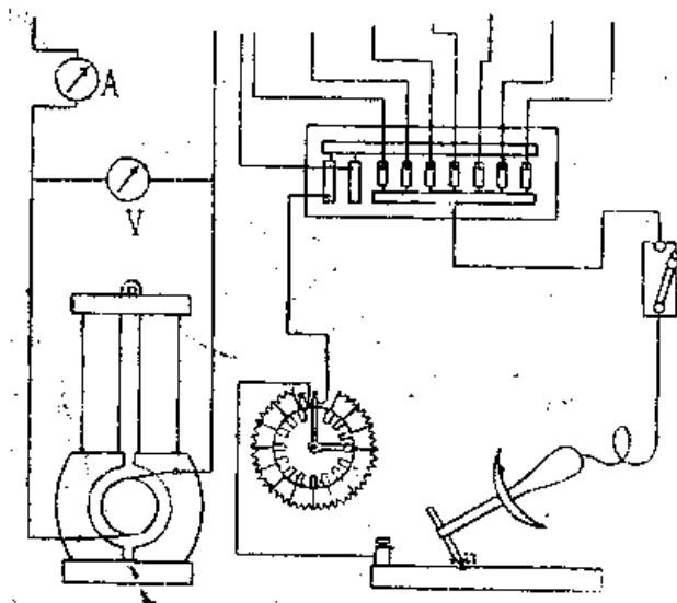
Рис. 136. Установка для электрической сварки, изобретенной Н. Н. Бенардосом в России около 1882 г.
