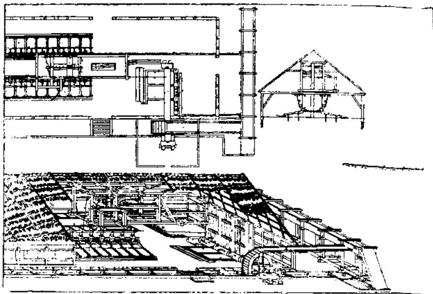
Рис. 107 Корбалихинский рудотолочный и рудопромывальный завод с механизацией технологических операций и внутризаводского транспорта, сооруженный К. Д. Фроловым в 1764 г. и представляющий прообраз будущих заводов-автоматов. — Центральный Государственный исторический архив в Ленинграде.
