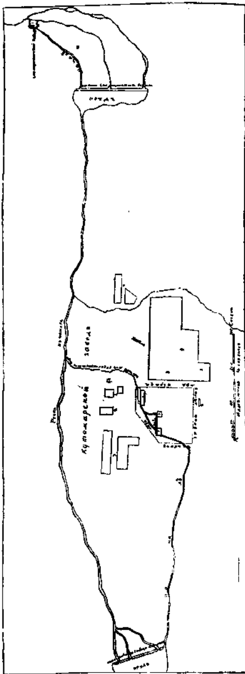
Рис. 112. Гидротехнические сооружения Кутомарского и Екатеринбургского заводов на реке Кутомаре в Забайкалье, доказавшие еще в XVIII веке возможность устройства водонапорных каналов в условиях Восточной Сибири. 1 — «фабрика» для наливки руда и отделения серебра от сплава; 2 — заводские строения; 3 — частные постройки (второй половина XVIII века). — Центральный Государственный исторический архив в Ленинграде.
