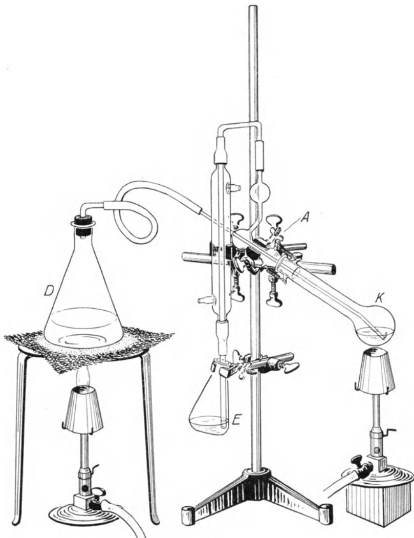
Fig. 20. Mikro-Kjeldahl. ( \frac{1}{5} natürl. Größe.)
