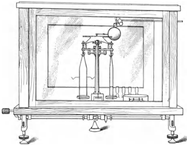
Fig. 1. Mikrochemische Wage.
