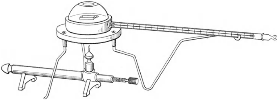
Fig. 12. Trockenblock mit Mikrobrenner und Thermometer in Verwendung. ( \frac{1}{2} natürl. Größe.)
