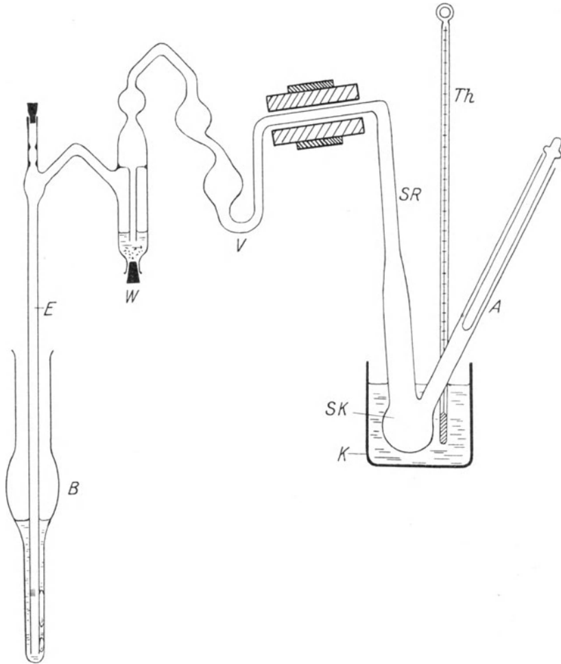
Fig. 32. Apparat für die Methylimidbestimmung.
