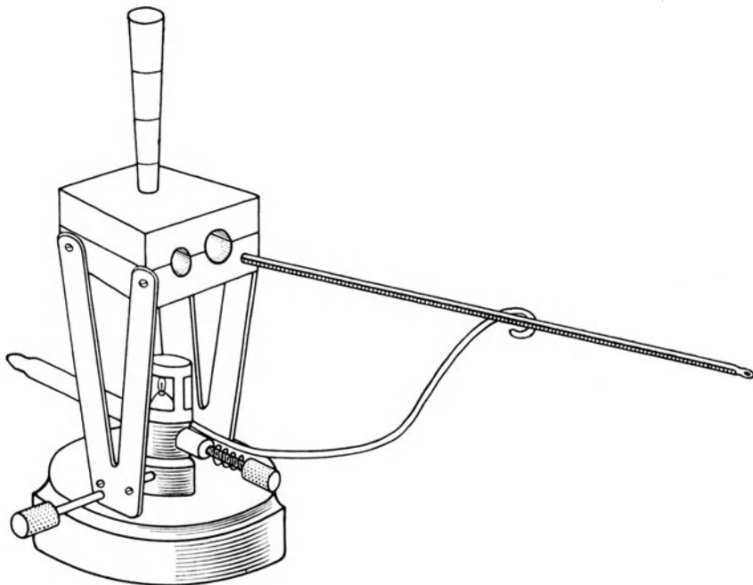
Fig. 14. Sog. Regenerierungsblock. ( \frac{1}{2} natürl. Größe.)
