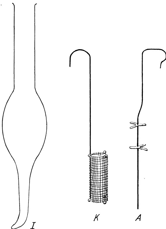
Fig. 27. Platinelektroden. (Natürl. Größe.)
