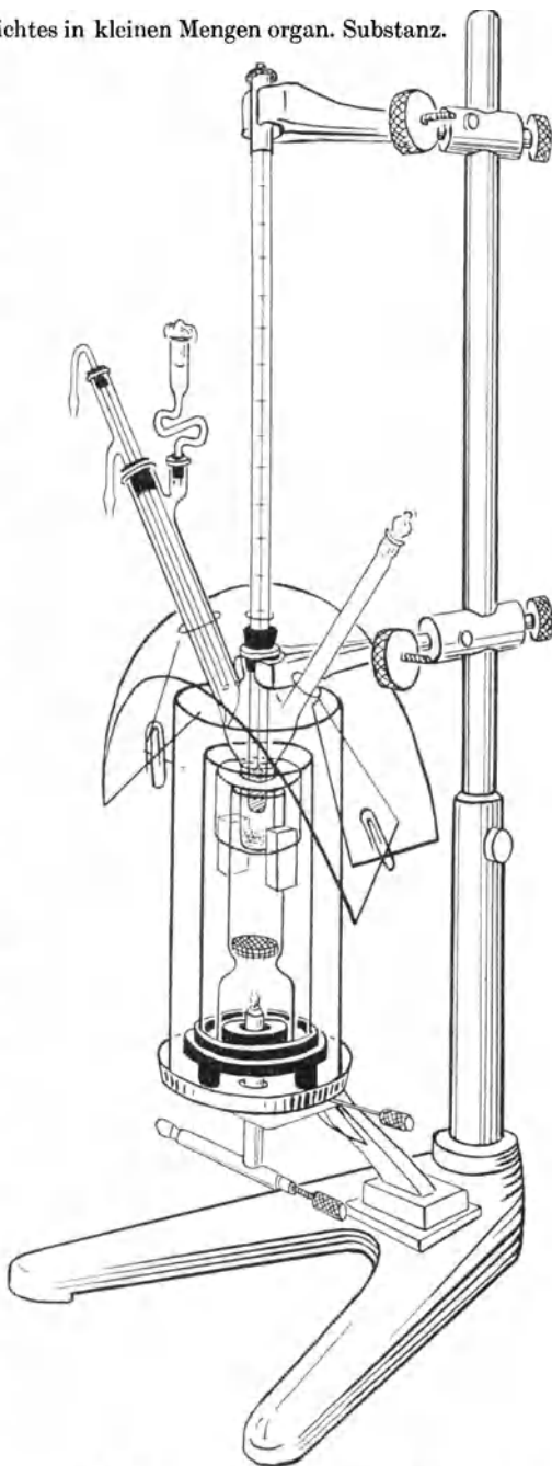
Fig. 33. Apparat zur Bestimmung des Molekulargewichtes aus der Siedepunktserhöhung an kleinen Substanzmengen. ( \frac{1}{4} natürl. Größe.)
