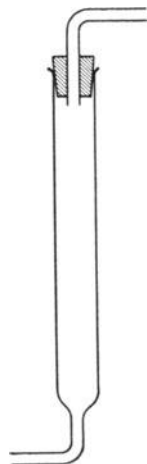
Fig. 10. Chlorkalziumrohr mit zwei rechtwinkelig abgelenkten Ansatzröhren. (Natürl. Größe.)
