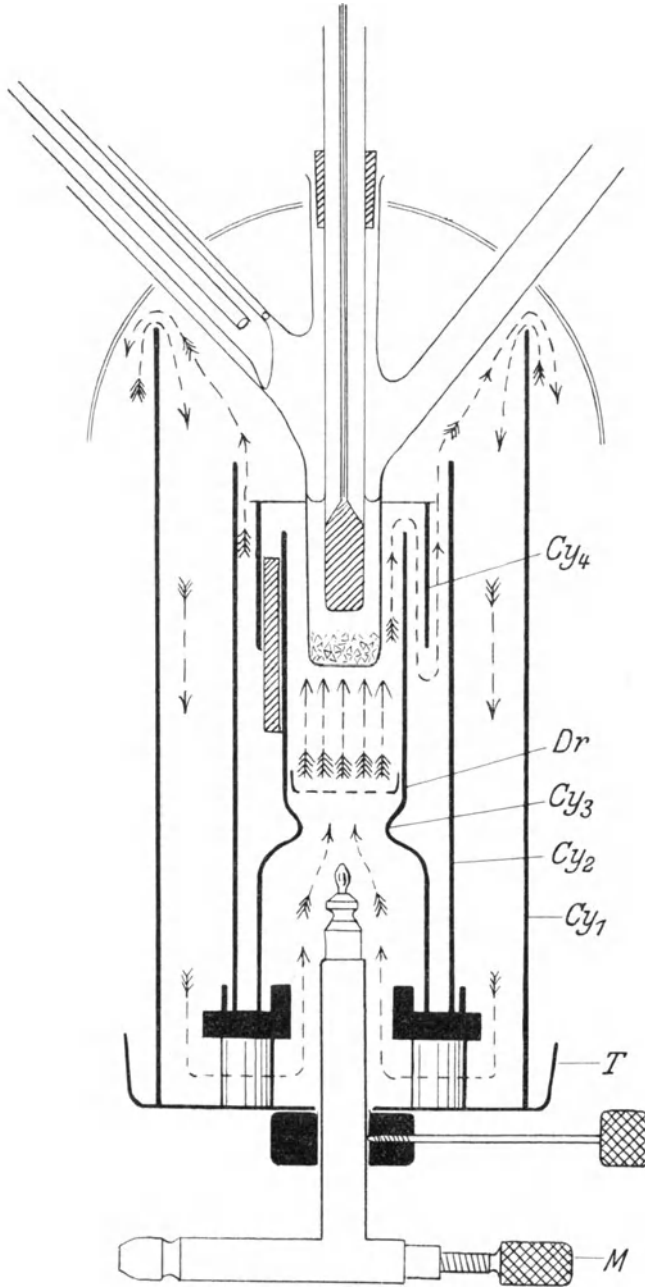
Fig. 34. Apparat zur Bestimmung des Molekulargewichtes aus der Siedepunkts- erhöhung an kleinen Substanzmengen (Durchschnitt). ( \frac{2}{3} natürl. Größe.) T Teller, M Mikrobrenner, Cy 1 , Cy 2 , Cy 3 , Cy 4 oben mit ange kitteter Glimmerplatte: die 4 Glas- zylinder, Dr Drahtnetz.
