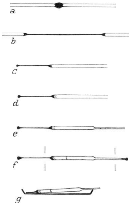
Fig. 15. Anfertigung der Kapillare zum Abwägen der Flüssigkeiten. (Natürl. Größe.) a ) Bildung eines Glastropfens in der Mitte, b ) Ausziehen desselben, c ) Eine Hälfte des in der Mitte durchgeschmolzenen Stückes, d ) Nachdem ein Kristall \text{KClO}_3 am Boden angeschmolzen und e ) sein offenes Ende zu einer Kapillare ausgezogen worden ist (I. Wägung), f ) Nach dem Einfüllen der Flüssigkeit und dem Zuschmelzen, g ) Die Kapillare nach Abschneiden des Griffes und Abbrechen der Spitze auf dem Platinblech liegend, im Momente der Einführung in das Verbrennungsrohr.
