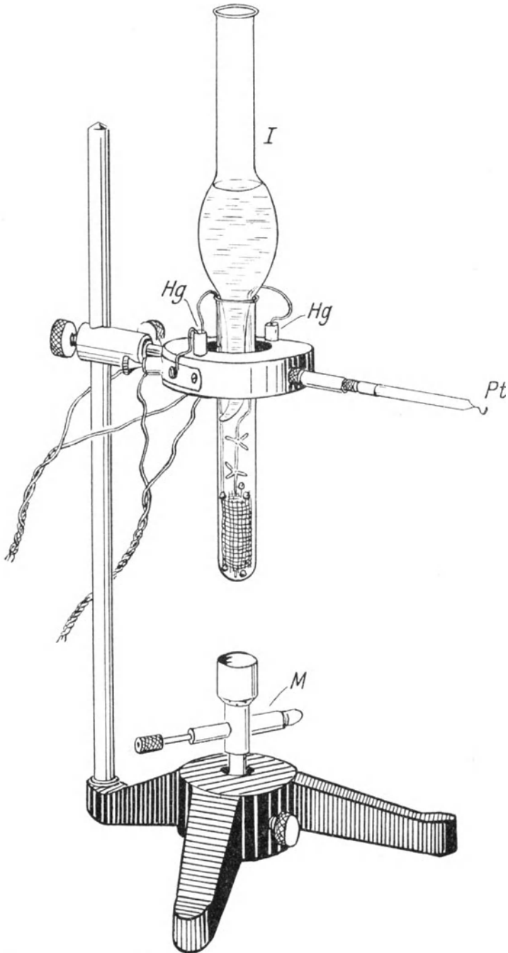
Fig. 28. Apparat zur Ausführung der elektroanalytischen Kupferbestimmung. ( \frac{1}{2} natürl. GröÙe.) I Innenkühler, Hg Quecksilbernapfchen, Pt Platinhäkchen, M Mikrobrenner.
