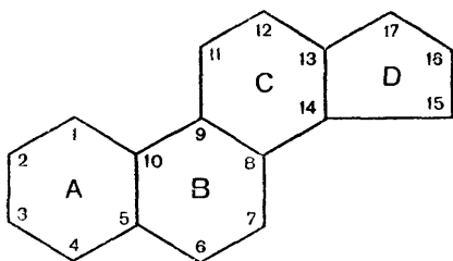
Рис. 15. Циклопентанпергидрофенантреновое ядро.
