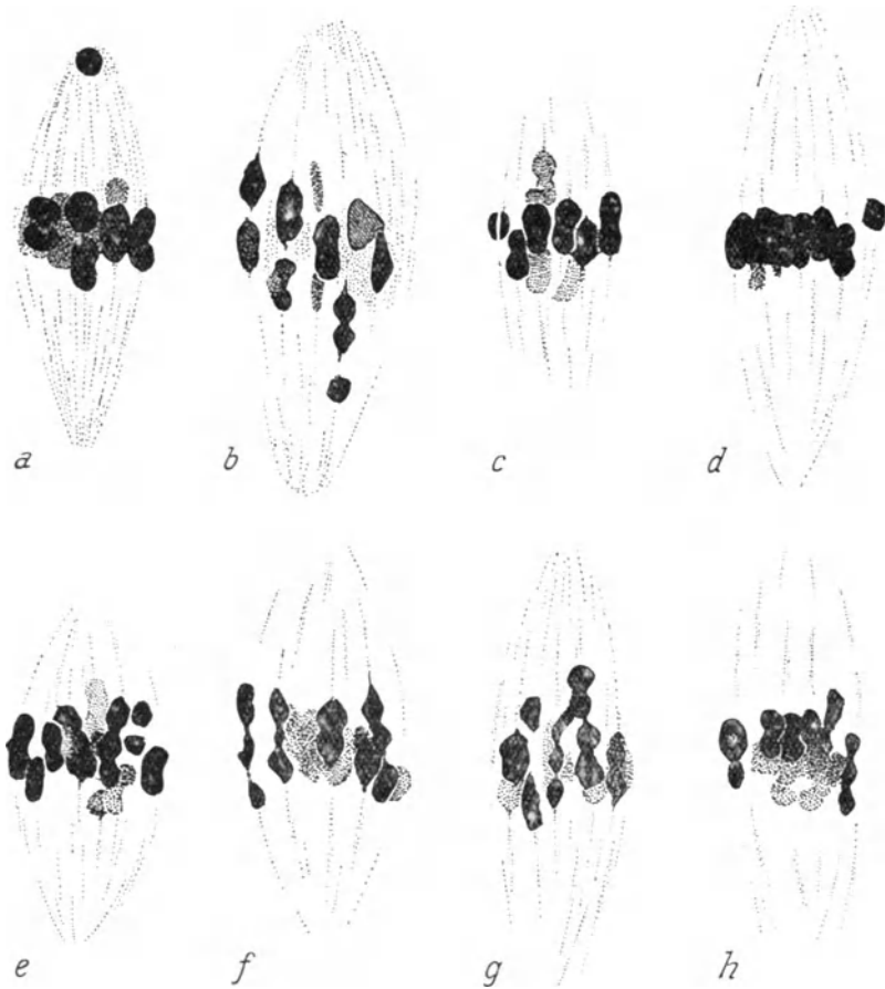
FIG. 20. Metaphase-I from male-sterile forms of Hevea . a, b. PR104. c. C.R.S. 24. d, e. KN 251. f, g. Ct 88. h. H. Spruceana × brasiliensis . 2700 ×.
