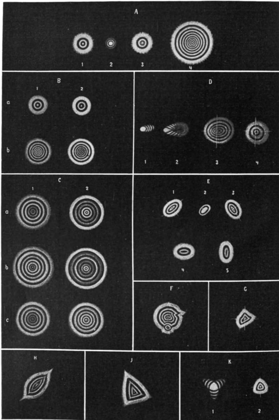
Abb. 104. Beugungsbilder eines Sterns: A. für ein gutes Objektiv; B. bei sphärischer Abweichung; C. bei Zonen; D. bei Koma; E. bei Astigmatismus; F. bei Schlieren; G., H., J. bei Spannung; K. bei Durchbiegung einer Linse. (Nach COOKE and Sons.)
