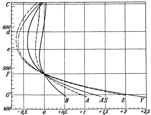
Abb. 28. Die Farbenlängsabweichung von Achromaten E , Y , zweilinsigen Apochromaten A , AS und einem dreilinsigen Apochromaten B ( F = 1000 ).
