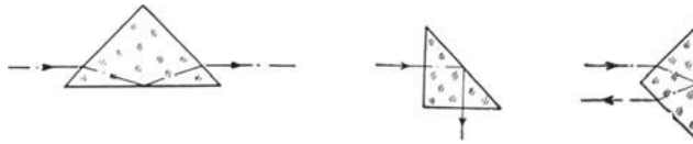
Abb. 10. Die Ablenkung des Lichts durch ein Spiegelprisma.
