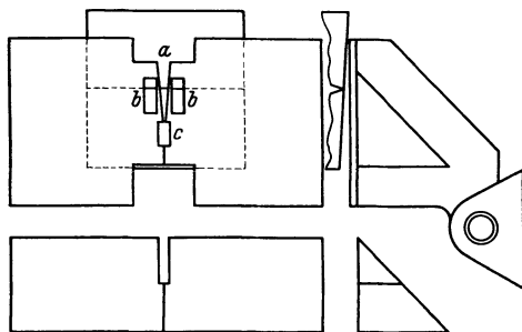
Abb. 15. Spaltblende von PLASKETT.
