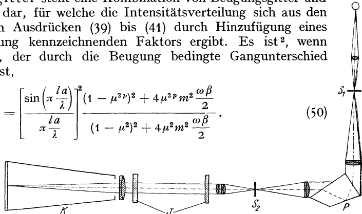
Abb. 34. Interferenzspektrograph mit getrennter Vorzerlegung.
