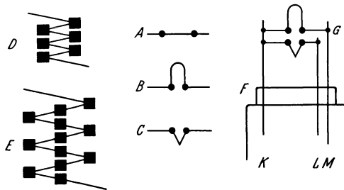
Abb. 35. Verschiedene Formen der auf dem Mt. Wilson verwendeten Thermoelemente. A , B , C drei Typen von Thermoelementen, F schematisches Bild eines Doppelthermoelementes mit seinen Platin-Zuführungsdrähten K , L und M ; D und E sind Formen von Thermosäulen, die bei Spektralarbeiten Verwendung fanden. [Ap J 56 (1922).]
