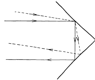
Abb. 5. Die Wirkung eines 90^\circ -Winkelspiegels.
