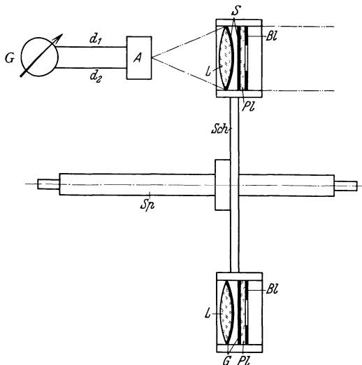
Abb. 26. Schematisches Bild des PETTITSchen Apparates zur Messung der ultravioletten Sonnenstrahlung.
