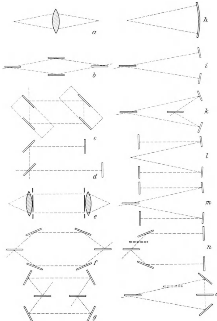
Abb. 28. Verschiedene Interferenzanordnungen nach MICHELSON.
