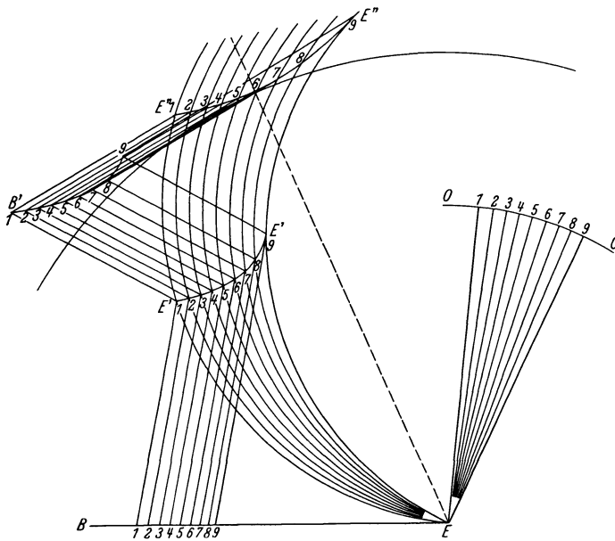
Abb. 10. Minimum der Ablenkung, Fall zweier Prismen.
