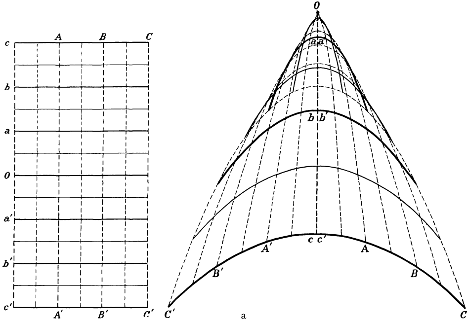
Abb. 20. a) Die Koma für eine Halböffnung von Rechteckform; b) von Halbkreisform; c) die Abbildung eines Öffnungskreises bei Koma.
