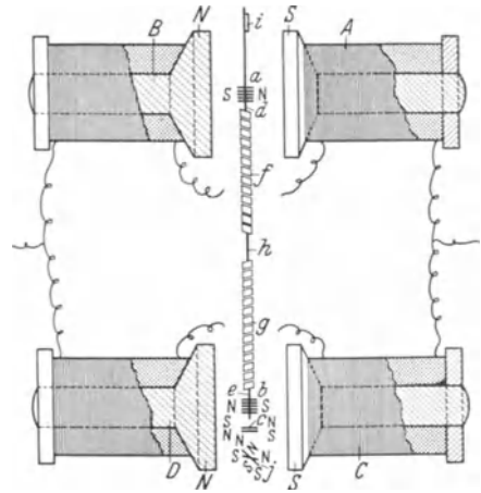
Abb. 53. Das Kampometer von C. G. ABBOT. Schematische Skizze eines neuen Gerätes von hoher Empfindlichkeit zur Messung der Gesamtstrahlung. [Smithson Misc Coll 89 (1933).]
