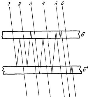
Abb. 35. BREWSTERSCHE Interferenzen.
