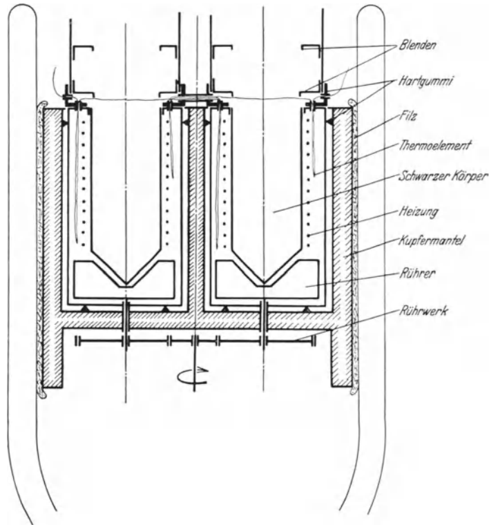
Abb. 47. Das neue Absolutinstrument der Phys.-Techn. Reichsanstalt (C. TINGWALDT) zur Messung der Gesamtstrahlung der Sonne. Schematisches Bild der zentralen Teile dieses verbesserten „Water-Stir“-Pyrheliometers. [Z f Instrk 51 (1931).]
