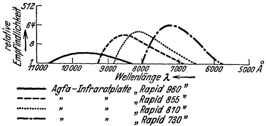
Abb. 4. Die spektrale Empfindlichkeit der Infrarotplatten der Agfa für Nitralicht. (Schematische Darstellung.) [Z f techn Phys 14, S. 177 (1933).]
