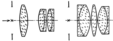
Abb. 62. 70°-Okulare nach ERFLE.
