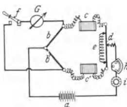
Abb. 10. Schematische Skizze der Brückenordnung des LANGLEYSchen Bolometers (Konstruktion von 1896). [Smithson Ann 1 (1900).]
