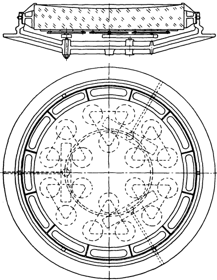
Abb. 84. Die Lagerung eines Fernrohrhohlspiegels nach Zeiss (MEYER).
