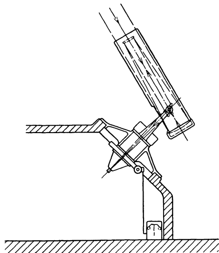
Abb. 100. Das Spiegelfernrohr nach RANYARD.
