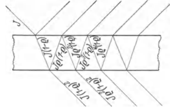
Abb. 2. Aufspaltung eines Strahles durch eine Planparallelplatte.
