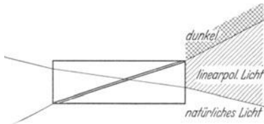
Abb. 7. Grenzen des polarisierten Gesichtsfeldes bei einem Polarisationsprisma.
