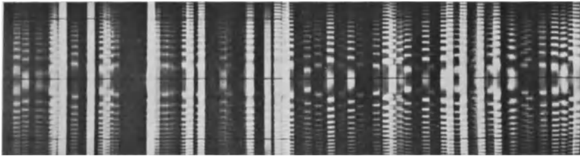
Abb. 22. Spektrum mit Interferenzen einer planparallelen Luftplatte.
