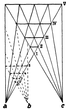
Abb. 75. Das Raumbild bei vergrößertem Abstand der Eintrittspupille.
