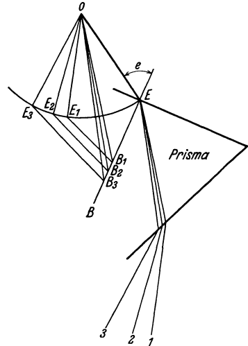
Abb. 12. Die Farbenzerstreuung durch ein Prisma.
