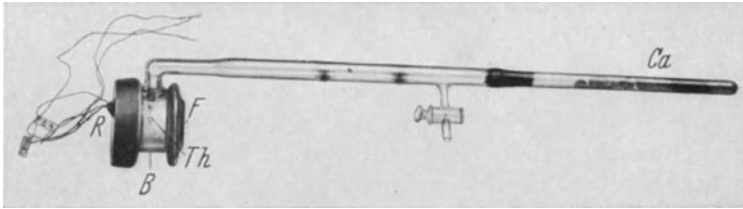
Abb. 32. Die thermoelektrischen Strahlungsmessungen von W. W. COBLENTZ. Der auf der Lick- und Lowell-Sternwarte verwendete evakuierte Behälter für die Thermoelemente. (Im übrigen siehe Text.)
