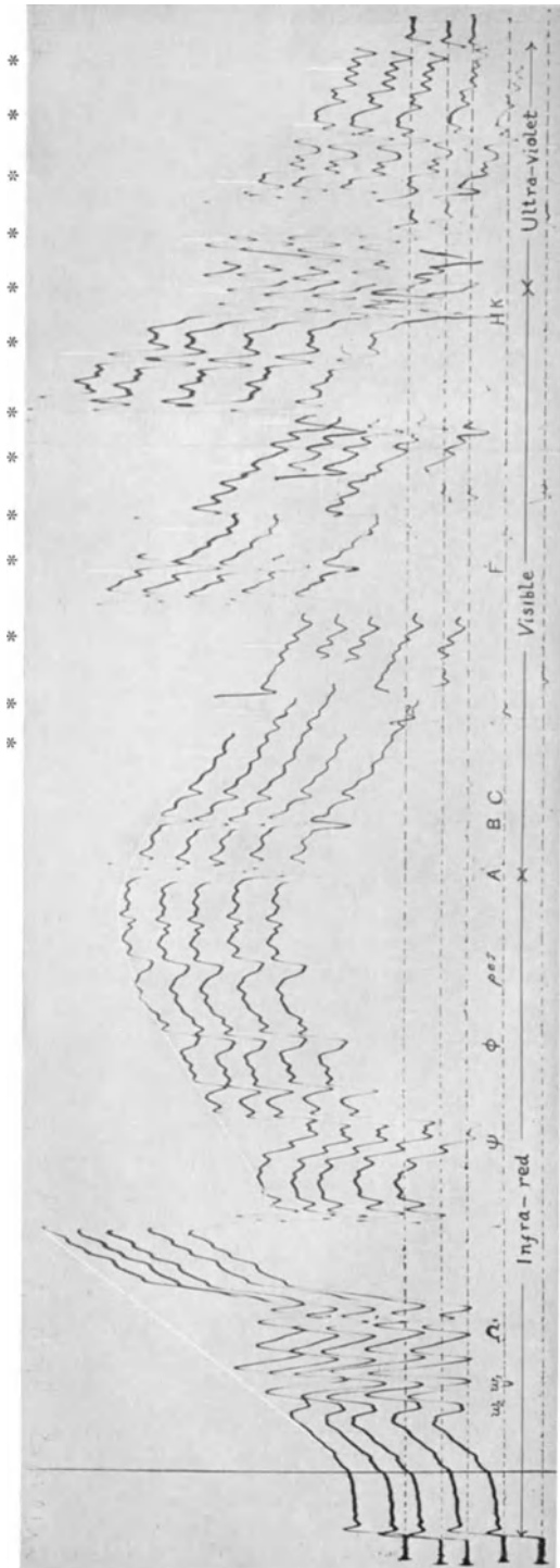
Abb. 17. Registrierstreifen des Spektrobolometers der Station Montezuma. Gewählt ist ein Tag sehr durchsichtiger Luft. Nichtsdestoweniger ist die Bande \rho\sigma\tau , im Gegensatz zu Tagen getrübler Atmosphäre, kaum merklich ist (s. diesbez. Ziff. 17 u. 18). An den mit * bzw. mit weißen senkrechten Strichen angedeuteten Stellen der Abbildung werden die Ordinaten des Bologramms ausgemessen. [Smithson Ann 5 (1932).]
