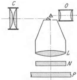
Abb. 24. Interferenzapparat zur Prüfung von Planflächen.
