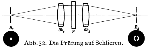
Abb. 52. Die Prüfung auf Schlieren.
