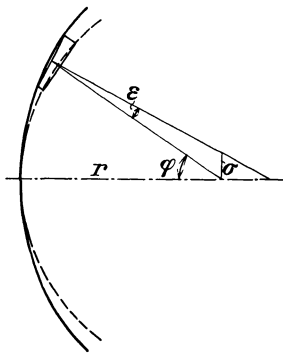
Abb. 115. Zur Prüfung nach CHALMERS.
