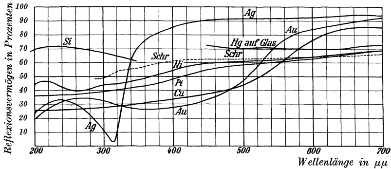
Abb. 81. Das Reflexionsvermögen einiger Metalle für verschiedene Wellenlängen: Schr SCHRÖDERSches Spiegelmetall (66 Cu + 22 Sn + 12 Zn).
