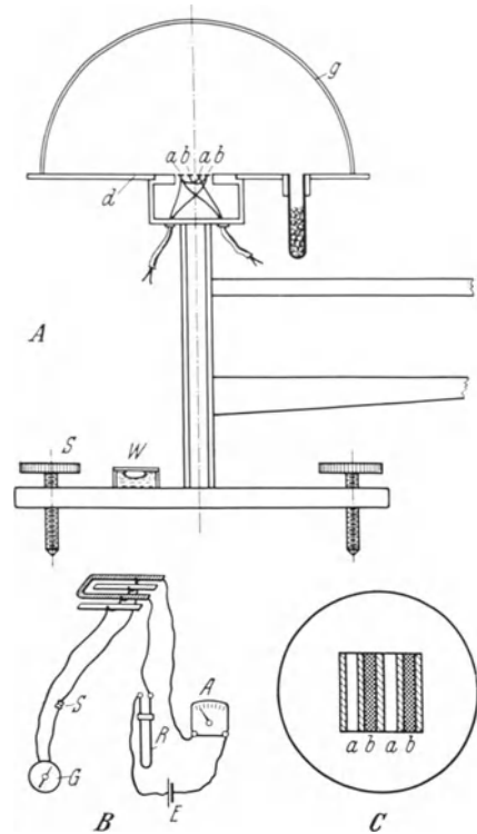
Abb. 18. Das Pyranometer von Anders Ångström. Oben (A) schematisches Bild des ganzen Apparates. Links unten (B) Schaltungsdiagramm, rechts unten (C) schematische Anordnung der Metallstreifen des Empfängers (im übrigen siehe Text). [Medd Met-Hydr Anst 4 Stockholm (1928).]
