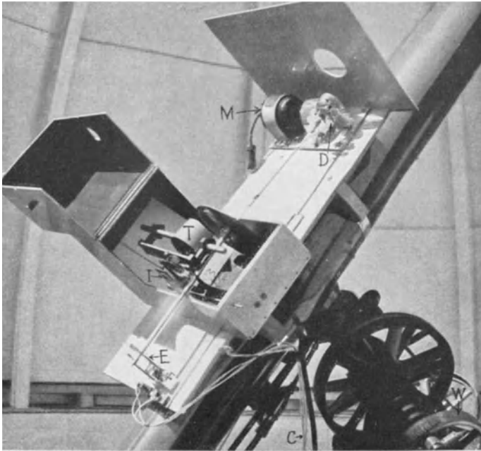
Abb. 27. Die Anordnung des thermoelektrischen Meßapparates am Sechszöller der Mt. Wilson-Sternwarte. [Ap J 75 (1932).]
