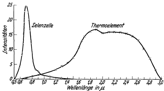
Abb. 1. Vergleichung der spektralen Empfindlichkeitsverteilung bei Selenzelle und Thermolement.
