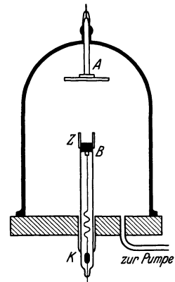
Abb. 50. Anordnung nach LO SURDO zur Beobachtung des elektrischen Effektes.
