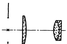
Abb. 59. Das KELLNERSche Okular.
