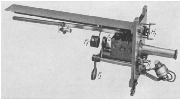
Abb. 33. Der thermoelektrische Meßapparat von W. W. COBLENTZ (siehe Abb. 32), fertig montiert zum Einsetzen in den Okularteil des Reflektors. F_1 , F_2 , F_3 sind ausschwenkbare Filter, H_1 und H_2 die zugehörigen Bedienungshandle.
