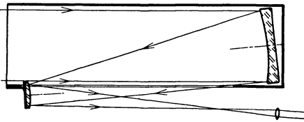
Abb. 91. Der Brachyt.
