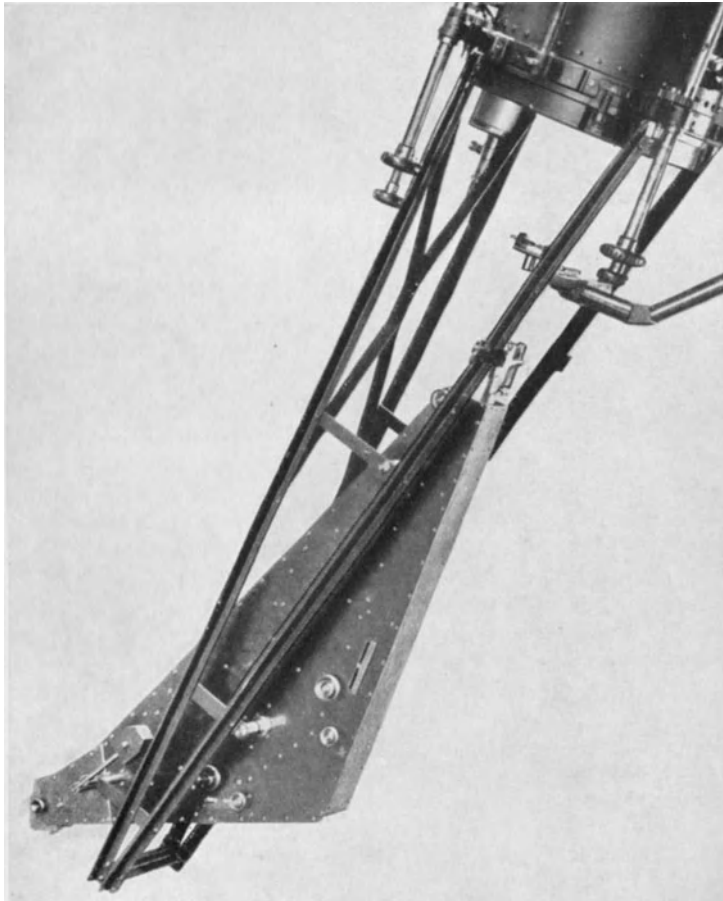
Abb. 10. Einprismenspektrograph des Ottawa-Observatoriums.
