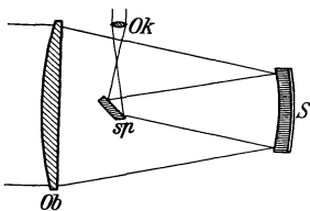
Abb. 93. Das Brachymedial.
