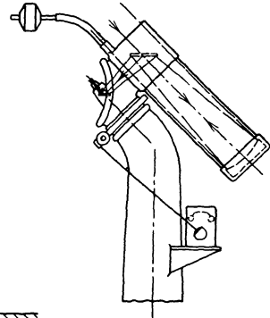
Abb. 97. Das Spiegelfernrohr nach PORTER.
