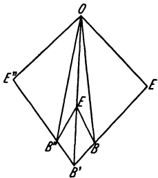
Abb. 9. Brechungsdreiecke beim geradsichtigen Prisma.
