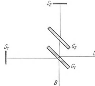
Abb. 27. MICHELSONSches Interferometer.
