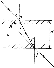
Abb. 4. Der Durchgang des Lichts durch eine Planplatte.
