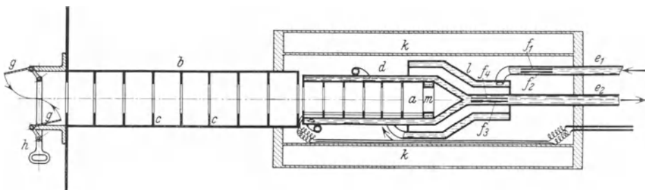
Abb. 8. Schematische Skizze des ABBOTTSchen Standardpyrheliometers, „Water-Flow-Pyrheliometer Nr. 1“. [Smithson Ann 2 (1908).]
