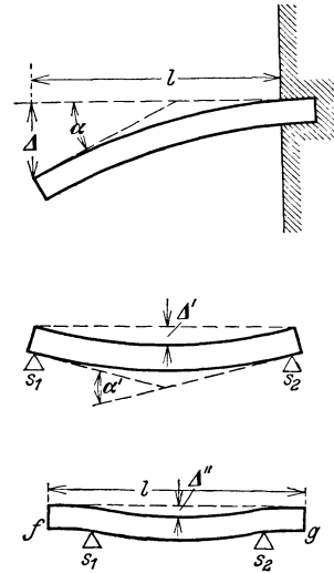
Abb. 5. Biegung eines Stabes.
