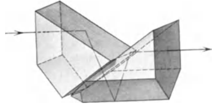
Abb. 71. Ein Umkehrprisma nach ABBE.
