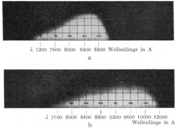
Abb. 3. Die spektrale Empfindlichkeit der Infrarotplatten „P“ und „Q“ der Eastman-Kodak-Gesellschaft. (Die Intensitätsskalen der beiden Teile der Abb. sind voneinander unabhängig.) [J Opt Soc Amer 23 (1933).]
