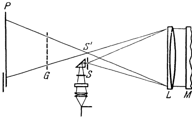
Abb. 118. Die Anordnung von BENNETT.
