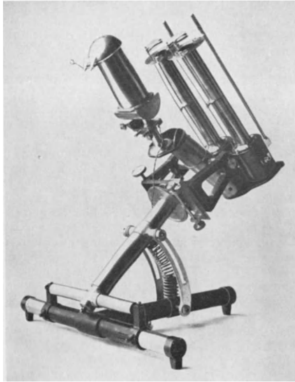
Abb. 21. Die neueste Pyranometertype (links) in gemeinsamer Montierung mit der verbesserten Form des Silver-Disk-Pyrheliometers (Zwillingssystem), wie sie nunmehr auf den Stationen des Smithsonian-Observatoriums in Verwendung stehen. [Smithson Ann 5 (1932).]
