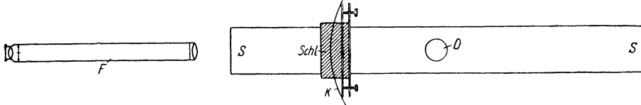
Abb. 136. Die Messung von Radien nach WETHAUER.
