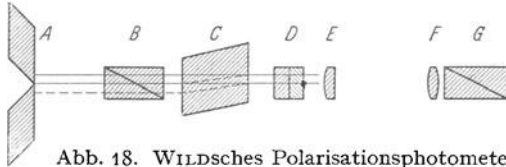
Abb. 18. WILDSches Polarisationsphotometer.
