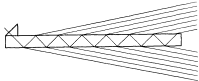
Abb. 19. LUMMER-GEHRCKE-Platte.
