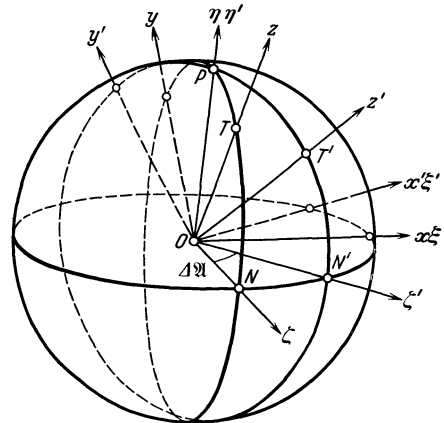
Abb. 2. Zur Darstellung der Richtungskosinus zwischen den Systemen Oxyz und Ox'y'z' durch \mathfrak{D}, \mathfrak{D}', \Delta\mathfrak{A} . NT = \mathfrak{D} , N'T' = \mathfrak{D}' , \sphericalangle NON' = \Delta\mathfrak{A} .
