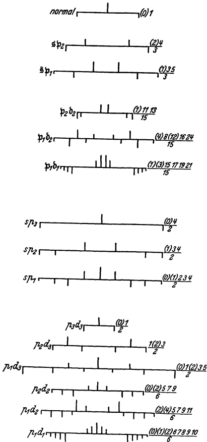
Abb. 43. Intensitäten der Komponenten bei magnetischer Zerlegung.
