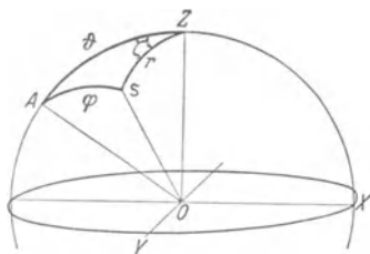
Abb. 15. Sphärisches Dreieck Wellennormale - Kristallachse - Plattennormale.
