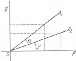
Abb. 3. Zusammensetzung zweier linear polarisierter Wellen.
