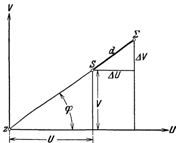
Abb. 6. Wirkung der Refraktion in einer im Zenit Z berührenden Ebene. \Sigma = Projektion des wahren, S = Projektion des scheinbaren Sternorts.
