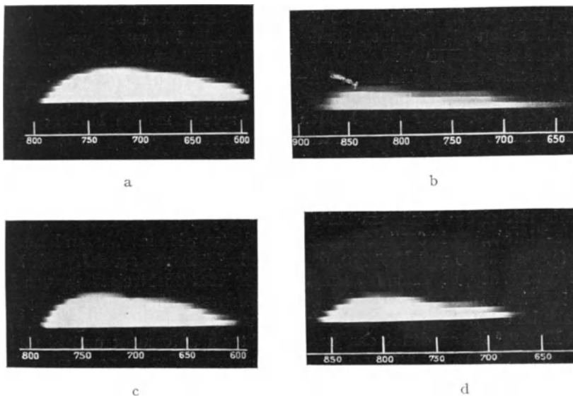
Abb. 2. Die spektrale Empfindlichkeit infrarot sensibilisierter Platten, aufgenommen durch Agfa-Rotfilter Nr 42. Folgende Sensibilisatoren sind angewendet: a) Rubrozyanin, b) Allozyanin, c) Agfa-Farbstoff 730, d) Agfa-Farbstoff 810. Die Belichtungszeit ist bei a, c und d dieselbe, bei b zehnmal so groß. [Veröff d wiss Zentr Lab d I. G. Farben A. G. 1 (1930).]
