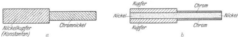
Abb. 52. Neue Mikrothermoelemente nach C. MÜLLER. Links (a): Schematisches Bild des Thermolementes vor dem Ausglühen. Rechts (b): Schematisches Bild des Elementes mit den Diffusionslegierungen nach dem Ausglühen. [Naturwiss 19 (1931).]
