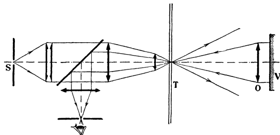
Abb. 111. LENOUEVELS Verfahren mit Gitter.
