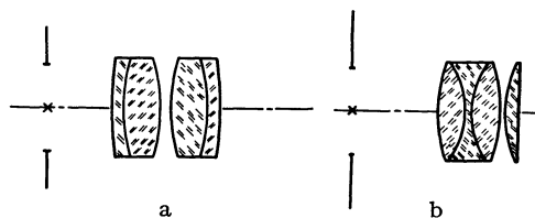
Abb. 61. Orthoskopische Okulare: a) nach PLÖSSL, b) nach ABBE.
