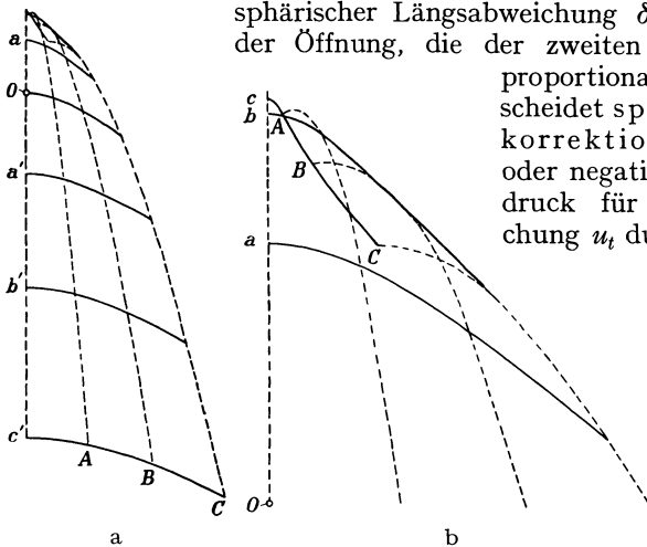
Abb. 25. Das Bild außer der Achse beim Königsberger Heliometerobjektiv für eine Rechtecköffnung.
