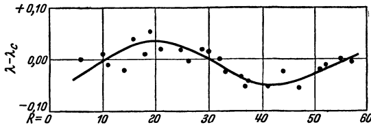
Abb. 20. Graphische Ausgleichung der \lambda - \lambda_c .
