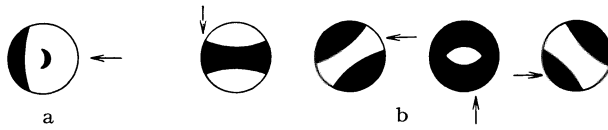
Abb. 128. Bilder beim Schneidungsverfahren für a) sphärische Abweichung, b) Koma.
