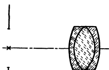
Abb. 60. Das monozentrische Okular.
