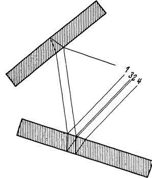
Abb. 36. Interferenzen bei geneigten Platten gleicher Dicke.
