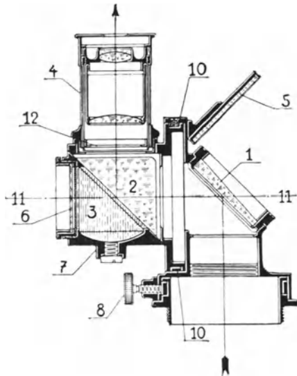
Abb. 63. Das Sonnenokular nach COLZI.
