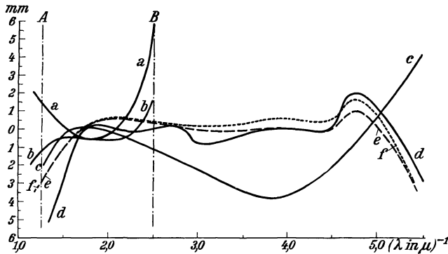
Abb. 50. Das sekundäre Spektrum von Spektrometerobjektiven, Abszisse Kehrwert der Wellenlänge in \mu , Ordinate Abweichung in mm für F = 1000 ; a) für einen Achromaten aus Silikatgläsern, b) für einen dreiteiligen Apochromaten, c) für ein Objektiv aus Quarz und Flußspat, d) für ein Objektiv aus Quarz, Flußspat und Steinsalz, e) und f) für ein Objektiv aus Quarz, Flußspat und Sylvin. (Nach PERRY.)
