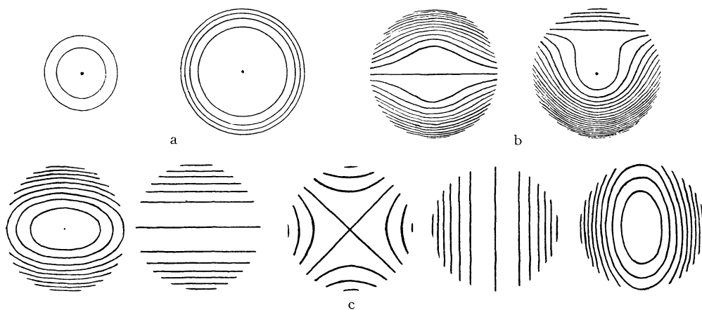
Abb. 107. Interferenzbilder bei TWYMAN'S Verfahren: a) sphärische Abweichung, b) Koma, c) Astigmatismus.
