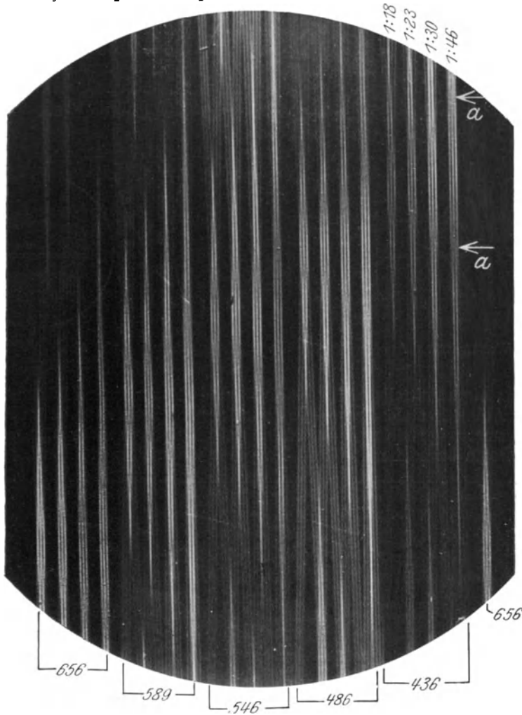
Abb. 121. Eine Aufnahme der sphärischen und chromatischen Abweichung nach WETTHAUER.
