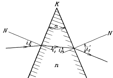
Abb. 3. Der Durchgang des Lichtes durch ein Prisma.
