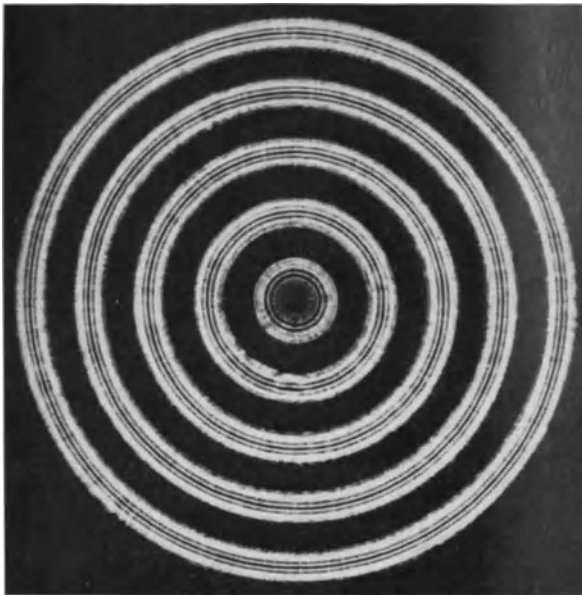
Abb. 119. Das Interferenzbild beim Verfahren von BENNETT.
