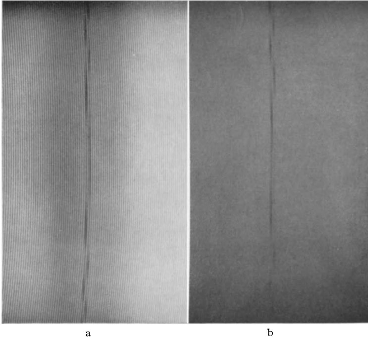
Abb. 23. Interferenzen einer Planparallelplatte im kontinuierlichen Licht.
