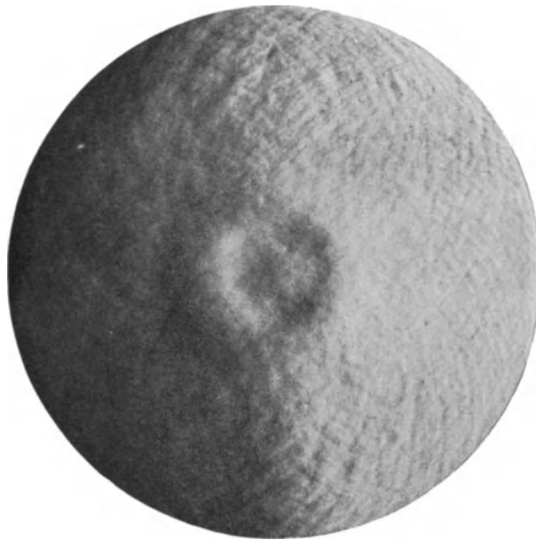
Abb. 129. Der Anblick eines Objektivs bei der Schneidprobe.
