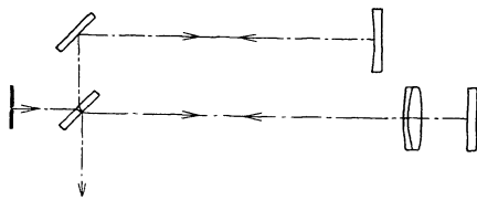
Abb. 106. Die Prüfung größerer Objektivs nach TWYMAN.
