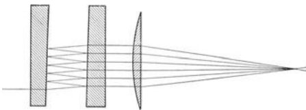
Abb. 32. PEROT-FABRY-Platte.
