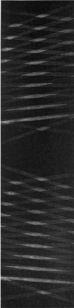
Abb. 126. Eine Aufnahme der Koma im Hauptschnitt nach WETTHAUER.
