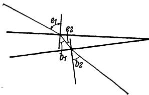
Abb. 4. Brechungsdreiecke eines Prismas und der Durchgang des Strahles durch das Prisma.
