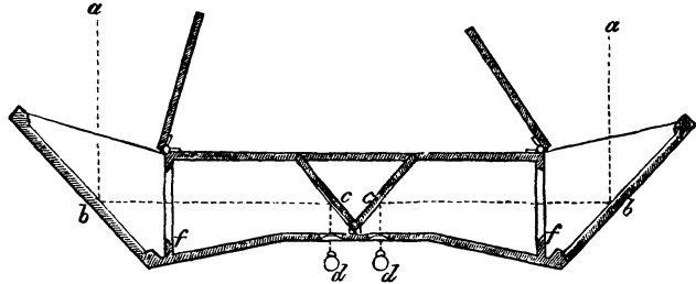
Abb. 74. Das Telestereoskop von HELMHOLTZ.
