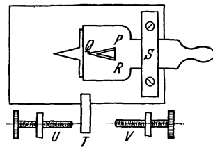
Abb. 13. Spaltblende nach HARTMANN.
