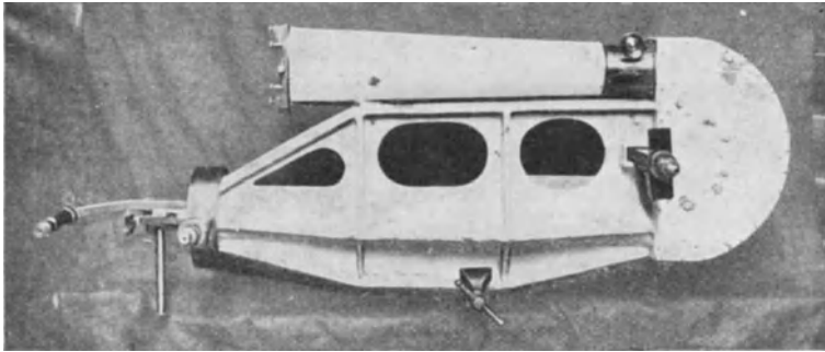
Abb. 6. Zweiter MILLS-Spektrograph des Lick-Observatoriums.
