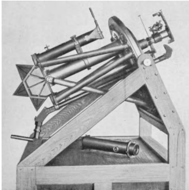
Abb. 2. Der BRUCE-Spektrograph des Yerkes-Observatoriums.
