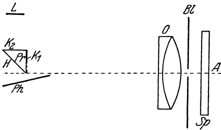
Abb. 122. WETHAUERS Autokollimationsverfahren.
