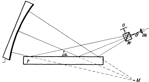
Abb. 132. Die Prüfung einer Planfläche mit Kugelspiegel.
