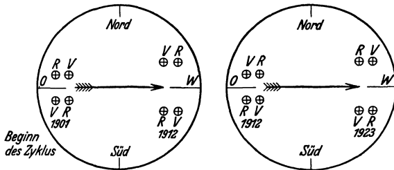
Abb. 47. Polaritäten der Sonnenflecke in einer 11½-jährigen Periode.
