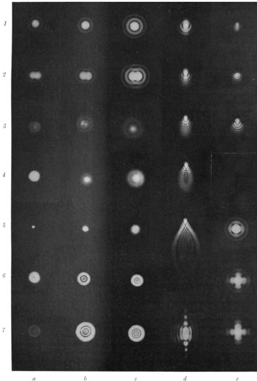
Abb. 34. Aufnahmen von Beugungsbildern: A. eines Lichtpunkts, a) bei kreisförmiger Öffnung mit verschiedener Belichtung ( a_1, b_1, c_1 ), b) bei Halbkreisöffnung ( d_7 nach SCHEINER), c) bei sphärischer Abweichung verschiedener Größe mit verschiedener Einstellung (Reihen 3 bis 7 bis zu c nach Mrs. GRIFFITHS), d) bei Koma von verschiedener Stärke ( e_1, e_2, e_3 ) und mit verschiedener Öffnung ( d_1 bis d_6 ), e) bei Astigmatismus verschiedener Stärke ( e_5, e_6, e_7 ), B. eines Doppelsterns mit verschiedener Belichtung ( a_2, b_2, c_2 ).
