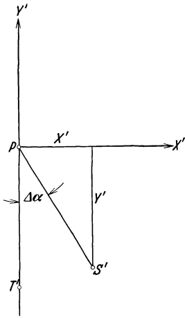
Abb. 3. Beziehung zwischen X', Y' und \alpha, \delta . T' und S' sind die Zentralprojektionen des Tangentialpunkts bzw. Sterns vom Kugelmittelpunkt auf die im Himmelspol P tangierende X'Y' -Ebene. PS' = \text{cotg } \delta , \sphericalangle T'PS' = \alpha - \mathfrak{D} = \Delta\alpha .
