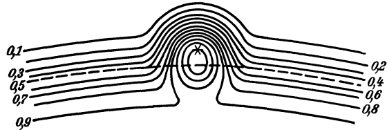
Abb. 36. Die Lichtverteilung in Schichtendarstellung beim Durchgang eines Sterns.
