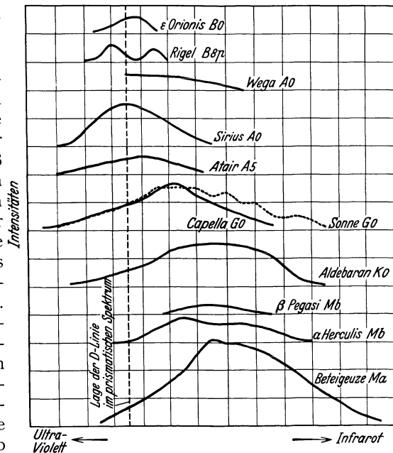
Abb. 41. Spektrobolometrische Messung der Energieverteilung in den Sternspektren. Gemittelte Kurven der extraterrestrischen Energieverteilung in der Skala des 36^\circ UV-Kronglas-Prismas. (Mt. Wilson-Versuche aus dem Jahre 1922.) [Smithson Misc Coll 74 (1923).]
