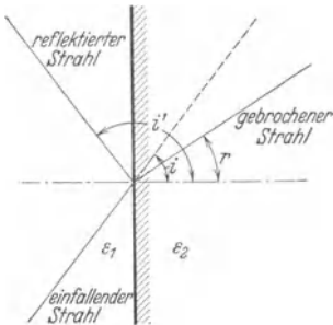
Abb. 1. Reflexion und Brechung bei isotropen Körpern.
