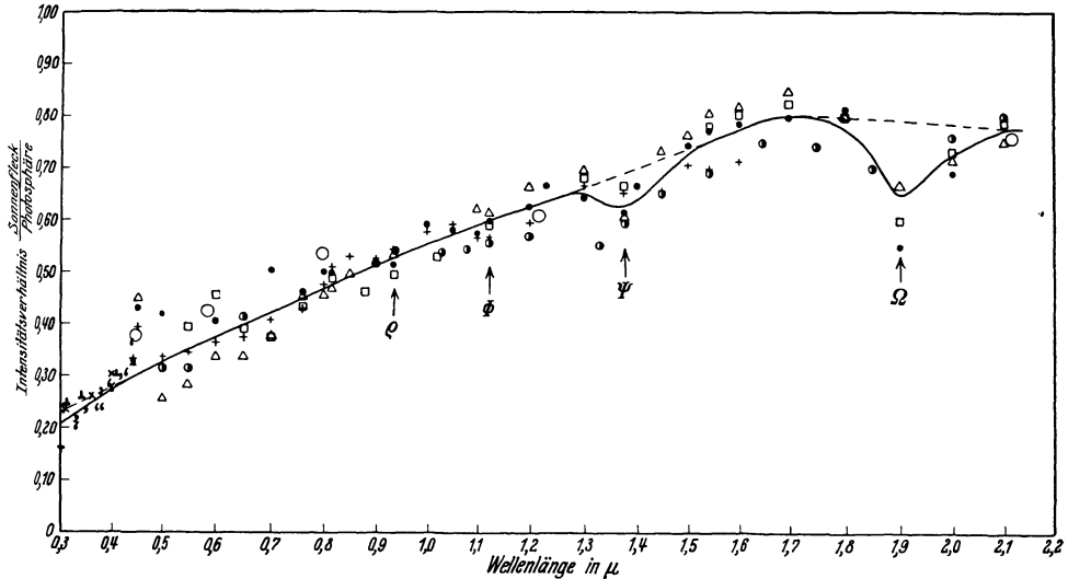
Abb. 23. Die Energiekurve des Intensitätsverhältnisses Sonnenfleck auf Photosphäre auf Grund bolometrischer und thermoelektrischer Messungen. Die Zeichen o entsprechen den bolometrischen Ergebnissen von ABBOT, die übrigen Zeichen stellen die Ergebnisse verschiedener Meßserien dar, die PETTIT und NICHOLSON mit Thermoelement und Monochromator gewonnen haben. Die Pfeile unterhalb der Kurve geben die Stellen der Absorptionsbanden \phi , \Phi , \Psi und \Omega an. (Siehe auch Abb. 17, S. 440.) [Ap J 71 (1930).]
