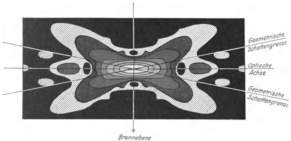
Abb. 42. Lichtverteilung in der Nähe des Fokus. Wenn man die Helligkeit in der Mitte gleich 100 setzt, so bedeuten die einzelnen Schraffierungen: ganz dunkel 1, dann zunehmend 2\frac{1}{2} , 5, 10, 25, 50, 75, 100. Die Abbildung ist im Sinne der geometrischen Optik aberrationslos vorausgesetzt. (Aus F. JENTZSCH, Beugungstheorie der optischen Instrumente, Handb. d. Physik Bd. 21. Herausgegeben von H. GEIGER und K. SCHEEL. Berlin: Julius Springer 1929.)
