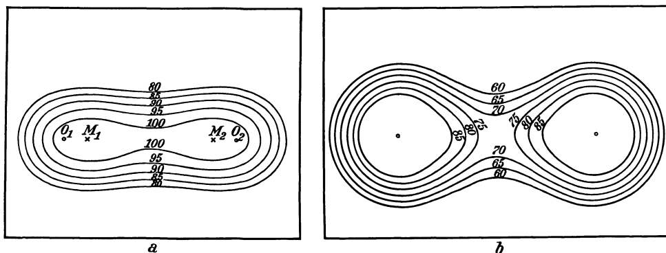
Abb. 35. Die Lichtverteilung in Schichtendarstellung bei Überlagerung zweier Beugungsscheibchen: a) für \mathfrak{z} = 3,2 , b) für \mathfrak{z} = 3,83 (Auflösungsgrenze eines Doppelsterns).
