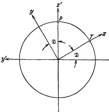
Abb. 4. Zur Ableitung der Richtungskosinus für die Transformation von X, Y in X', Y' und umgekehrt. P = Himmelspol, T = Tangentialpunkt. Die zusammenfallenden x - und x' -Achsen stehen auf der Zeichenebene senkrecht.
