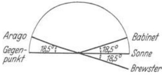
Abb. 11. Lage der neutralen Punkte am Himmel.
