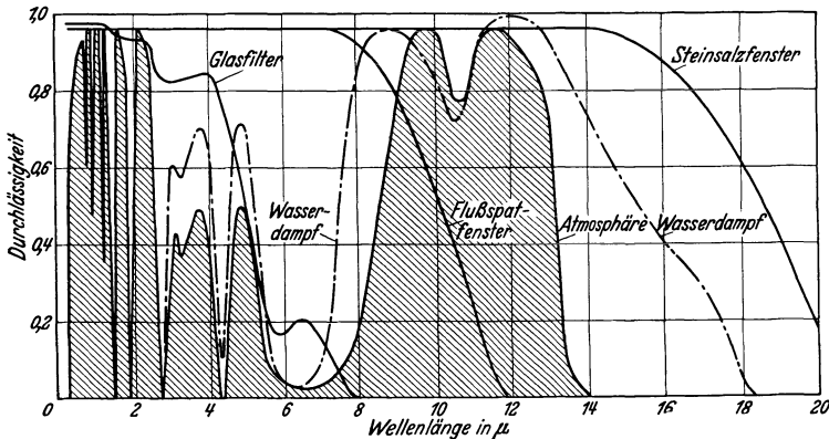
Abb. 38. Die angenommene Durchlässigkeit der Atmosphäre über dem Mt. Wilson in verschiedenen Wellenlängen (Begrenzungskurve der gestrichelten Fläche), sowie Transmissionskurven des Wasserdampfes und einiger bei den thermoelektrischen Untersuchungen verwendeten Filter. [Ap J 71 (1930).]
