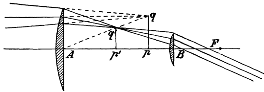
Abb. 57. Das HUYGENSSCHE Okular.
