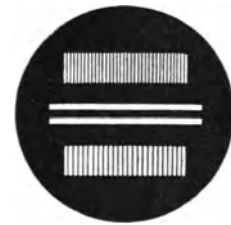
Abb. 124. WETHAUERS Doppelspalt mit Quergitter.
