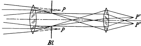
Abb. 31. Die Eintrittspupille PP und die Austrittspupille P'P' als Bilder der Öffnungsblende Bl .
