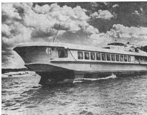
Теплоход на подводных крыльях «Ракета» конструкции Р. Е. Алексеева. Из сборника «Советские инженеры».
