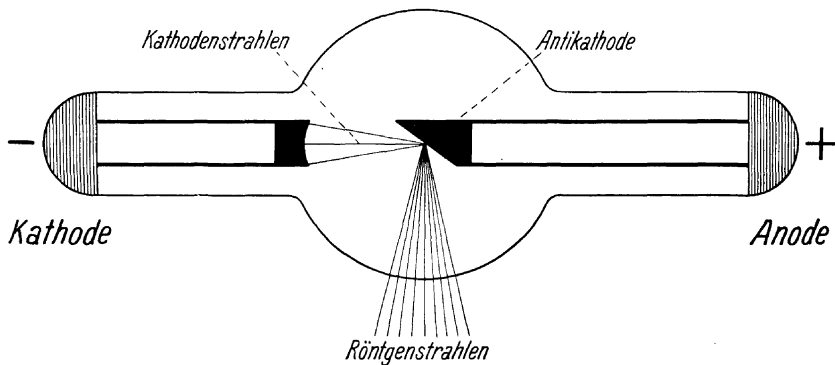
Abb. 1. Röntgenröhre.
