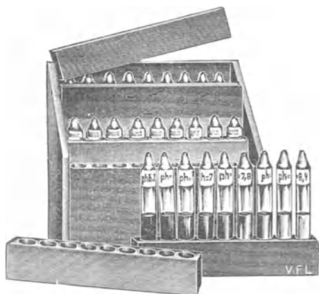
Abb. 7. Gestell mit den fertigen Indikator-Dauerreihen, für p_H = 2,3-8,4 .
