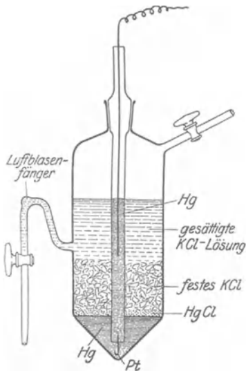
Abb. 29. Kalomelelektrode. Als Füllung ist die der „gesättigten“ Kalomelelektrode dargestellt (siehe 75. Übung). Hier wäre an Stelle von „gesättigte KCl-Lösung“ zu setzen: „0,1 n. KCl-Lösung“, und die Schicht „festes KCl“ würde fortfallen.
