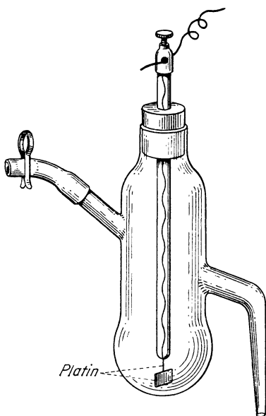
Abb. 41. Chinhydronelektrode \frac{1}{1} bis \frac{1}{2} nat. Größe.
