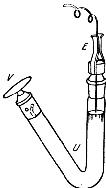
Abb. 34. U-Elektrode.
