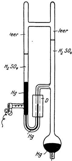
Abb. 25. Kapillarelektrometer.
