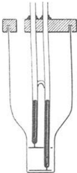
Abb. 23. Widerstandsgefäß.
