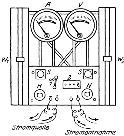
Abb. 17. Schematische Ansicht einer einfachen Schalttafel. Der Strom der Elektrizitätsquelle (Gleichstrom von 110 oder 220 Volt) wird zu den gezeichneten 2 Polklemmen geführt. Der in den Überführungsapparat zu schickende Strom wird aus zwei anderen Polklemmen abgenommen. W_1 und W_2 sind regulierbare Gleitwiderstände, ein gröberer und ein feinerer. A Amperemeter, V Voltmeter, beide mit drei Meßbereichen; das Amperemeter genau ablesbar zwischen 3 und 0,001 Ampère; das Voltmeter ablesbar zwischen 220 und 0,001 Volt. 1 Umstellvorrichtung für die verschiedenen Meßbereiche des Amperemeters, 2 ebensolche für das Voltmeter. SS Sicherungen. H Einschalter für den Strom. N Einschaltung für Stromentnahme durch Nebenschluß.
