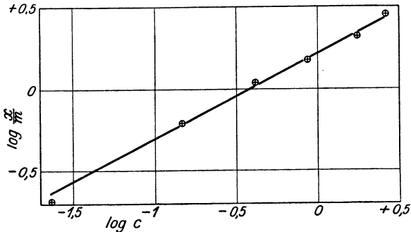
Abb. 20. Adsorptions-Isotherme für Azeton.
