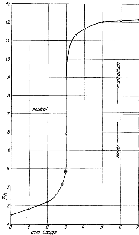
Abb. 37. 3 ccm 0,1 n HCl werden mit steigenden Mengen 0,1 n NaOH versetzt. Abszisse: ccm der Lauge. Ordinate: p H .
