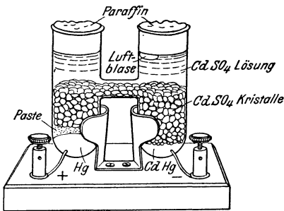
Abb. 24. Normalelement.
