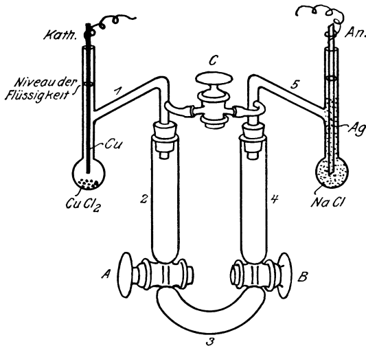
Abb. 15. Apparat für elektrische Kataphorese. \frac{3}{10} natürl. Größe.
