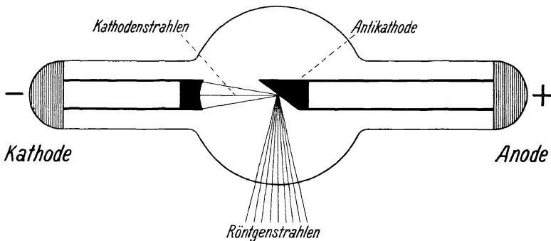
Abb. 1. Röntgenröhre.
