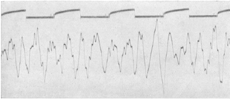
Abb. 13. Vesiculäralmen, aufgenommen mit Kondensatormikrophon und Oszillographen. Grundschwingung 120, daneben Oberschwingungen von 500 erkennbar. Oben Zeitschreibung.
