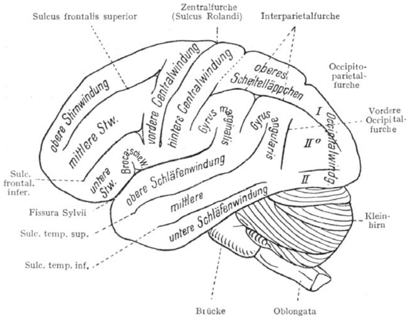
Abb. 115. Seitenansicht des Gehirns.
