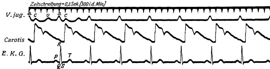
Abb. 43. Normaler Rhythmus des Herzens 1 .
