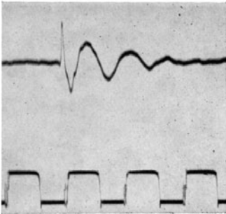
Abb. 9. Normaler tiefer lauter Lungenschall. Die untenstehenden Markierungen bedeuten die Zeitschreibung in \frac{1}{50} Sekunde.
