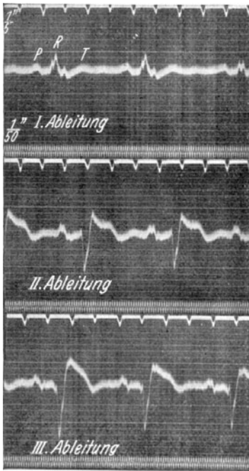
Abb. 39. Elektrokardiogramm bei schwerer Myokardschädigung. (Schenkelblock.)
