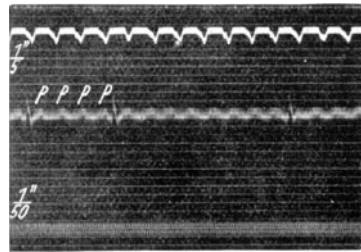
Abb. 40. Arrhythmia absoluta mit Vorhofflattern. Zwischen den unregelmäßigen Abständen der R-Zacken erkennt man deutlich die sehr viel häufigeren Vorhofkontraktionen (P-Zacken).
