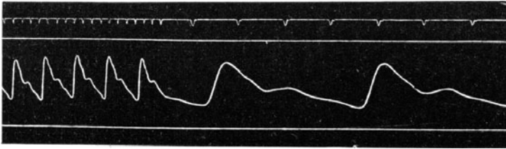
Abb. 49. Normaler Puls eines gesunden jungen Mannes. Systolische Nebenwelle schwach, dikrotische Welle deutlich ausgeprägt. Maximaler Blutdruck 120, minimaler 70 mm.
