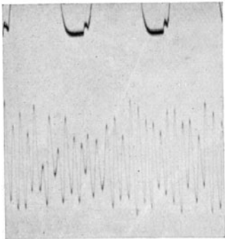
Abb. 14. Trachealmen in derselben Weise aufgenommen. Schwingungen zwischen 500 und 600.
