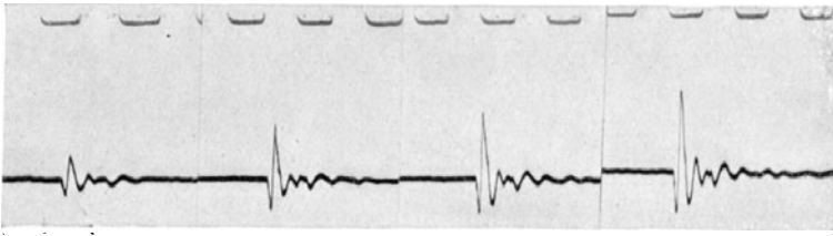
Abb. 12. Perkussion der rechten unteren Lungengrenze während der Inspiration. Der leise Leberschall macht bei dem inspiratorischem Herabrücken des unteren Lungengrandes dem lauten Lungenschall Platz; dementsprechend wächst von links nach rechts die Amplitude und die Dauer des Perkussionsschalles.
