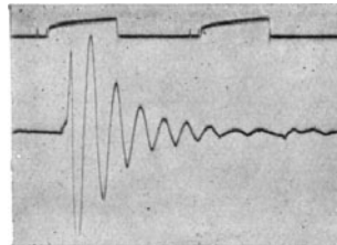
Abb. 11. Tympanitischer Bauchschall. Ganz regelmäßig verlaufende Sinuskurve mit 208 Schwingungen in der Sekunde.
