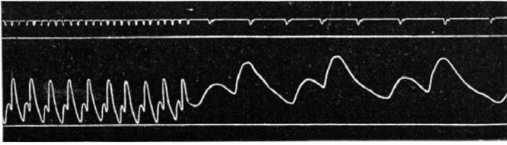
Abb. 52. Überdikroter Puls bei Sepsis und hohem Fieber. Die systolische Hauptwelle beginnt, bevor die dikrotische des vorausgegangenen Pulses ganz abgelaufen ist. Maximaler Blutdruck 100, minimaler 50 mm.
