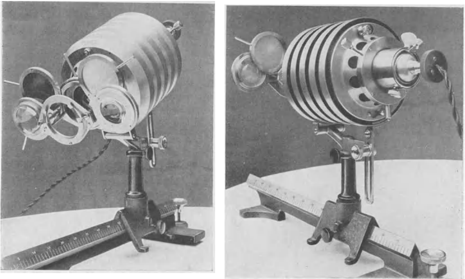
Abb. 26. Universal-Mikroskopierlampe „Lux S“ nach ROMEIS.
