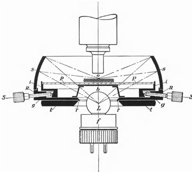
Abb. 142. Schematischer Durchschnitt des Epi-Spiegels. gg = kreisrunde Grundplatte; tt = Tischplatte; rr = Rand der Grundplatte zum Einsetzen in die Tischöffnung; RR = äußerer Ring für den ringförmigen Hohlspiegel SS ; pp = Glas-Objektträger aus wärmeabsorbierendem Glas; o = Objekt; ii = Haltering, bewegbar durch die Schrauben SS ; L = Lampe mit Fassung ( f ). (Aus F. HAUSER [5]).
