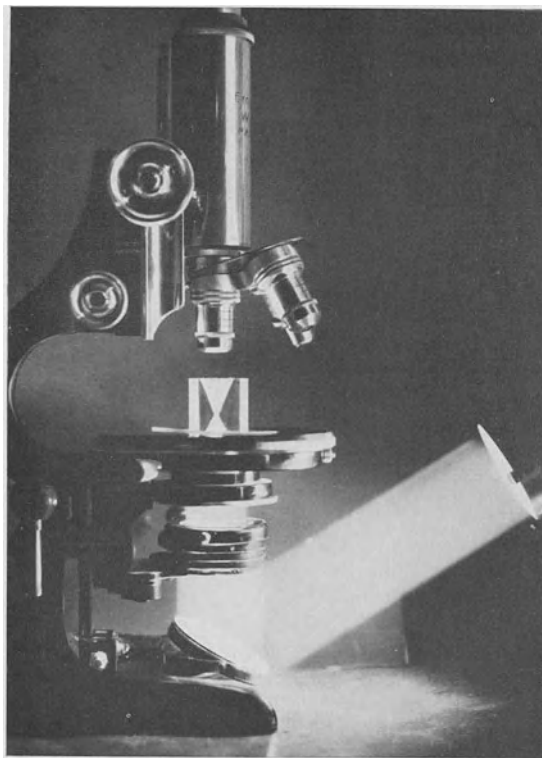
Abb. 106. Strahlengang im Dunkelfeldmikroskop. Der Strahlengang oberhalb des Kondensors wird durch einen Uranglaswürfel sichtbar gemacht. (Aus W. E. ANKEL [1, Abb. 1].)
