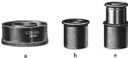
Abb. 15. Homal (b) mit Paßstück (a) und Zwischenstück (c) mit aufgesetztem Okular. (Aus ZEISS-Druckschrift: Mikro 401.)
