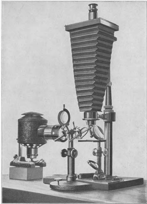
Abb. 117. Mikrophotographische Einrichtung der Firma E. BUSCH A.-G. für Auflicht bei schwachen Vergrößerungen. (Aus M. WOLFF [1, S. 15, Abb. 11].)
