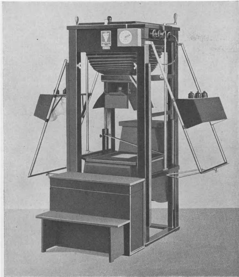
Abb. 57. Simplex-Universalapparat der Firma H. TRAUT.
