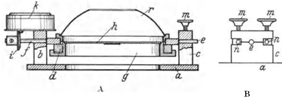
Abb. 164. Wippe für mikrosteroskopische Aufnahmen. A Wippe im Längsschnitt. B Lager der Wippe in der Ansicht. a = Grundplatte; b , e = die Lager der Wippe; d = Rahmen; e , f = Zapfen; g = Ring zum Halten des Objektträgers h ; i = Hebel; k = Zeigerwerk; m , m = Stellschrauben zur Regelung. (Aus der Gebrauchsmusteranmeldung der Firma O. HIMMLER.)
