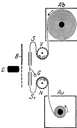
Abb. 225. Schema eines Aufnahmeapparates.
