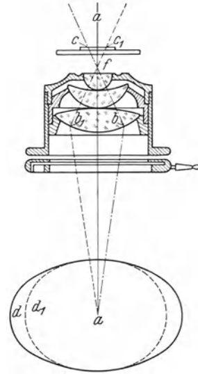
Abb. 170. Strahlengang im Kondensatorsystem des ABBESchen Beleuchtungsapparates.
