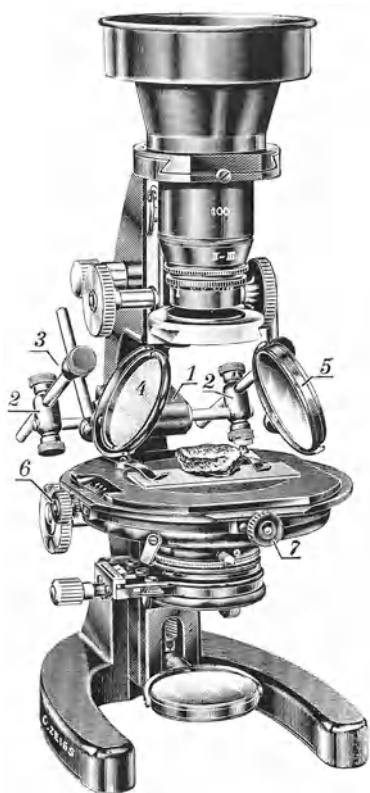
Abb. 118. Mikrophotographische Einrichtung der Firma C. ZEISS für schwache Vergrößerungen im Aufsicht mit Mattscheibe und Spiegel auf Haltern.
