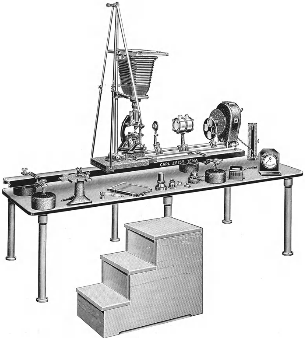
Abb. 71. Die Horizontal-Vertikal-Kamera 18 > 24 der Firma C. ZEISS. (Aus ZEISS-Druckschrift: Mikro 401.)
