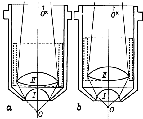
Abb. 12. Schematische Darstellung einer Korrekptionsfassung.
