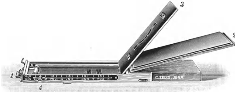
Abb. 48. Schiebekassette. (Aus der ZEISS-Druckschrift: Mikro 314.)
