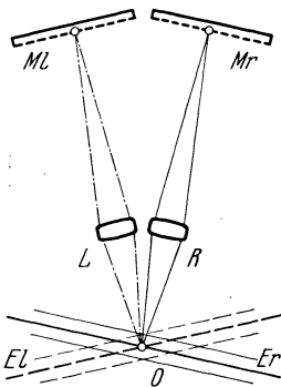
Abb. 163. Der gemeinsame Schärfenraum der Halbbilder bei Aufnahme eines körperlichen Objekts. (Aus A. KÖHLER [8, Fig. 951a, S. 1954].)
