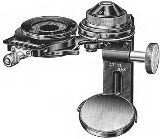
Abb. 17. ABBEScher Beleuchtungsapparat mit ausgeklapptem dreh- und verschiebbarem Blendenträger. (Aus A. KÖHLER [9, Abb. 230, S. 287].)
