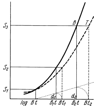
Abb. 52. Schwärzungskurven (Schema). B = Intensitätskurve; T = Zeitkurve. An die Ordinate sind die Schwärzungen, an die Abszisse die Belichtungen aufgetragen. (Aus A. KÖHLER [8, Abb. 890, S. 1753].)
