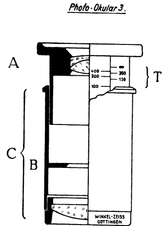
Abb. 16. Photographisches Okular der Firma WINKEL-ZEISS (Beschreibung ohne Abbildung in WINKEL-Druckschrift Nr. 208).
