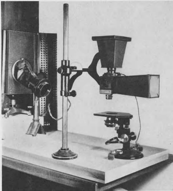
Abb. 90. Mikrophotographische Einrichtung mit einer Spiegelreflexkammer (nach SCHEFFER) und einem Lupenstativ für Aufnahmen bei schwachen Vergrößerungen.) Besonders für Momentaufnahmen geeignet.)
