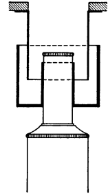
Abb. 8. Schematischer Durchschnitt von einem lichtdichten Abschluß zwischen Mikroskop und Kamera (Licht- schutzmanschette). (Aus HEIM u. SKELL [1, S. 34].)
