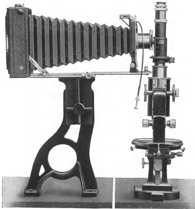
Abb. 83. Mikrophotographische Einrichtung der Firma ZEISS-Ikon mit dem „Mikrophot“ und einer Balgkamera.
