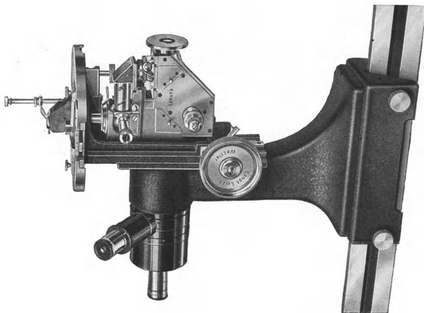
Abb. 153. Großes Metallmikroskop der Firma E. LEITZ. (Aus LEITZ-Druckschrift; Metalle 51 B I.)
