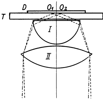
Abb. 18. Beleuchtung eines Präparats durch ein Kondensorsystem.
