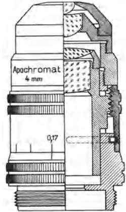
Abb. 11. Trockenapochromat der Firma E. LEITZ mit Korrekptionsfassung (schematischer Durchschnitt).
