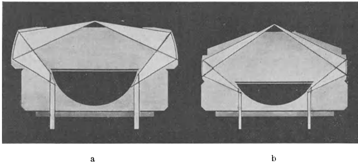
Abb. 108. Strahlengang im Leuchtfeld-Kondensator (a) und im Kardioidkondensator (b) nach H. SIEDENTOPF. (Aus H. ZOCHER [1, Abb. 350].)
