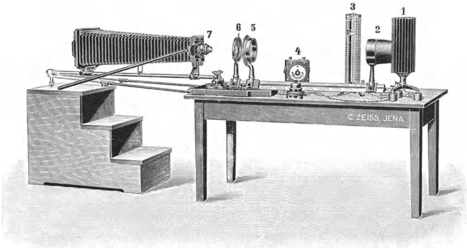
Abb. 100. Horizontal-Vertikalkamera der Firma C. ZEISS für Aufnahmen großer Objekte mit einem photographischen Objektiv (z. B. Tessar 1 : 6,3) und mit Einstellvorrichtung ausgerüstet.
