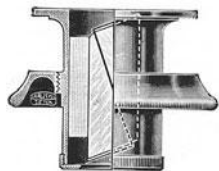
Abb. 179. Polarisator mit Pfanne und Deckel zum Einhängen in den Diaphragmenträger. (Aus ZEISS-Druckschrift: Mikro 400.)
