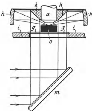
Abb. 135. Dunkelfeldkondensor nach F. HAUSER für Auflicht.
