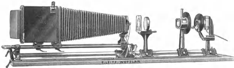
Abb. 98. Der große mikrophotographische Apparat „Uma“ der Firma E. LEITZ mit einem Summar ausgerüstet. (Aus LEITZ-Druckschrift Nr. 49 G.)
