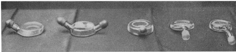
Abb. 211. CARRELSche Flaschen. (Aus G. LEVI [7, Abb. 371, S. 538].)
