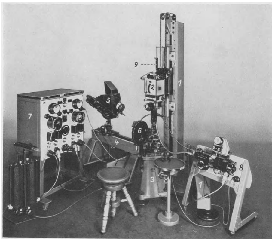
Abb. 221. Großer mikrokinematographischer Apparat der Askania-Werke nach K. HÖFER.
