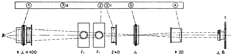
Abb. 66. Anordnung für Mikrotare und Planare.
