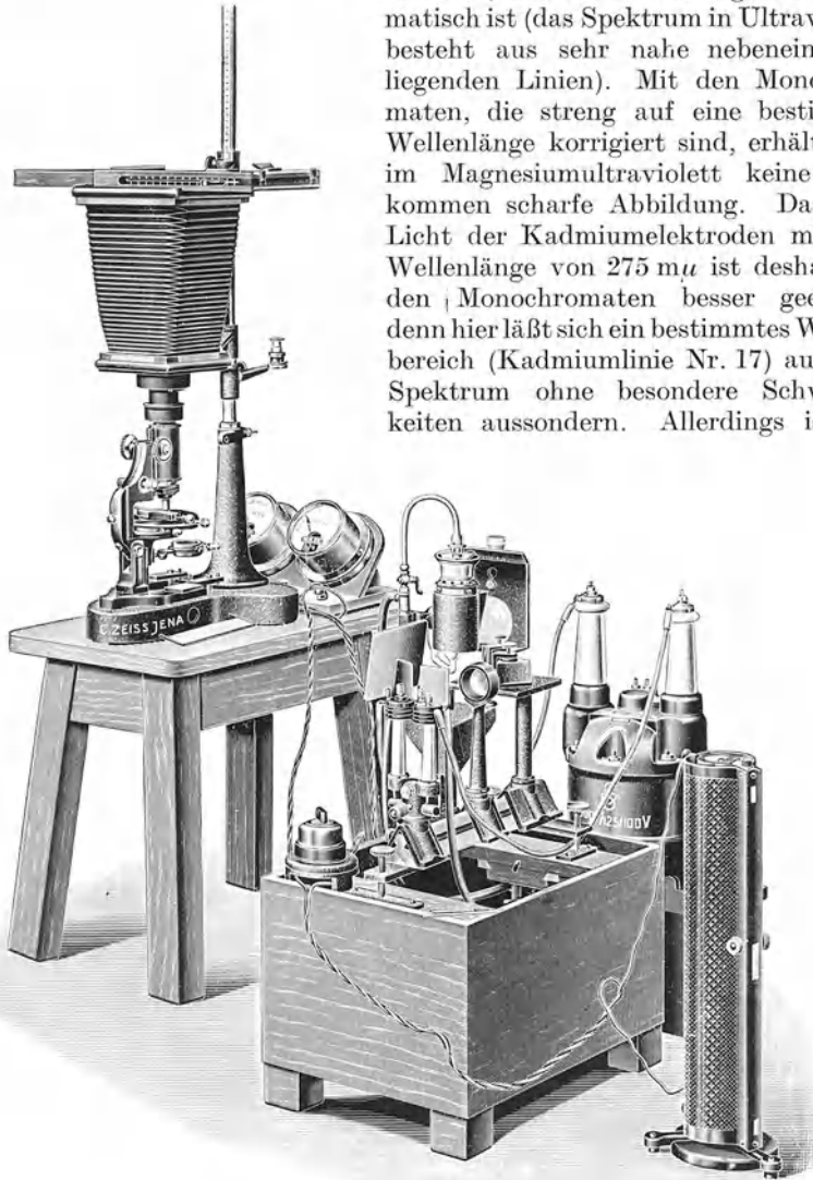
Abb. 190. Einrichtung für Mikrophotographie mit ultraviolettem Licht. (Aus A. KÖHLER [8, Fig. 944 S. 1934].)
