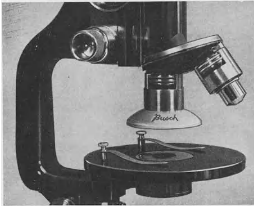
Abb. 125. Der LIEBERKÜHNSche Spiegel. (Aus BUSCH-Druckschrift: Anleitung zum Gebrauch von Mikroskopen und Nebengeräten für Untersuchungen in auffallendem Licht.)
