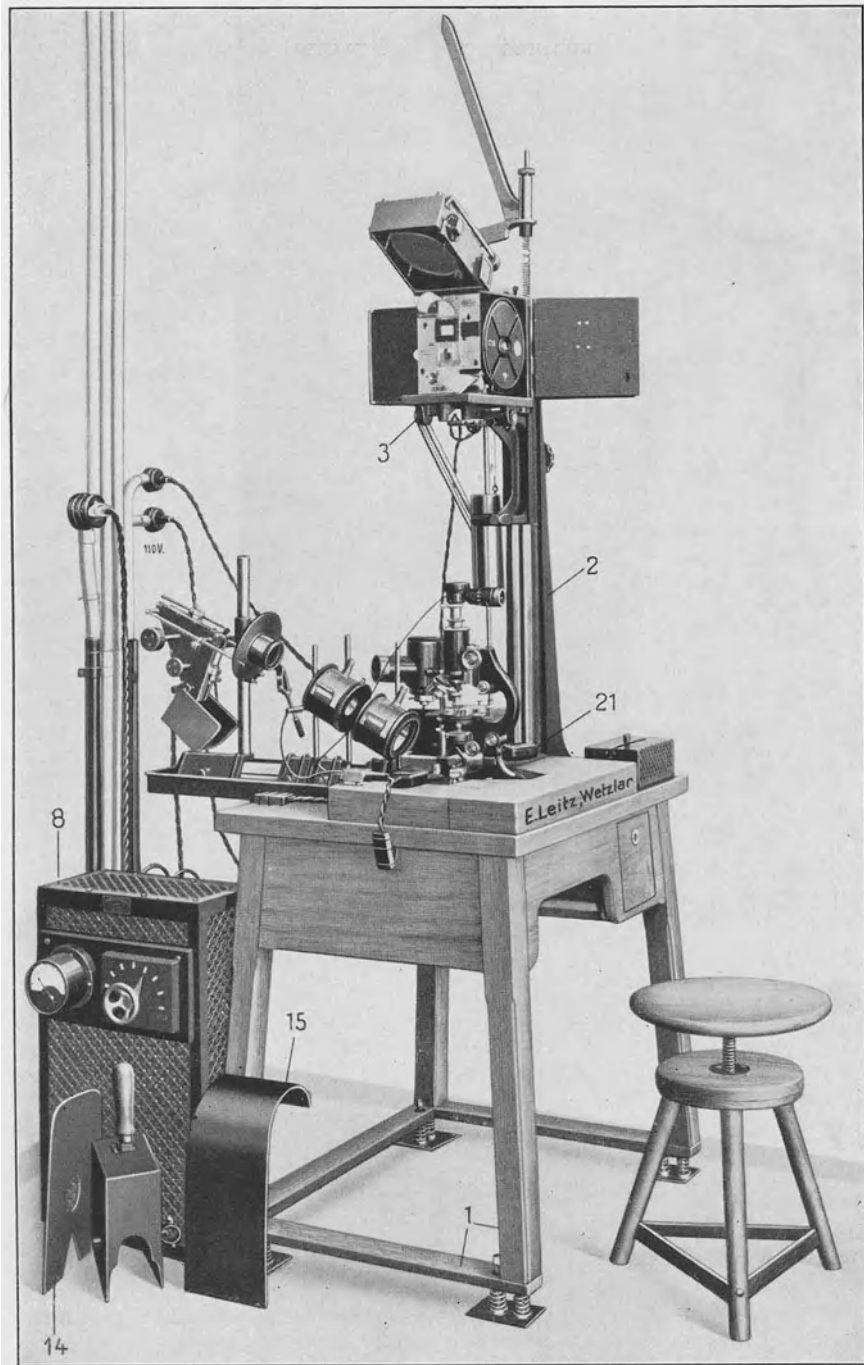
Abb. 223. Mikrokinoeinrichtung (geöffnet) der Firma E. LEITZ.
