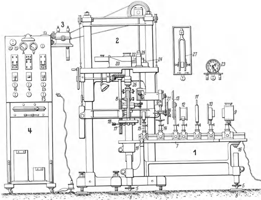
Abb. 224. Schematische Darstellung des mikrokinematographischen Apparates von H. ROSENBERGER.
