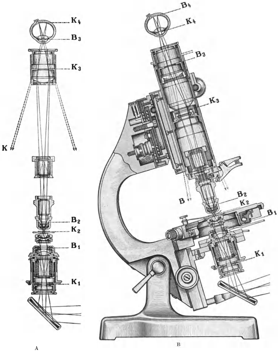
Abb. 176. Strahlengang im Polarisationsmikroskop.
