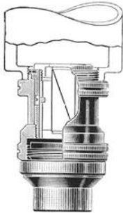
Abb. 184. Analysator VI (Innennikol) in Zwischengewinde. (Aus ZEISS-Druckschrift: Mikro 401.)
