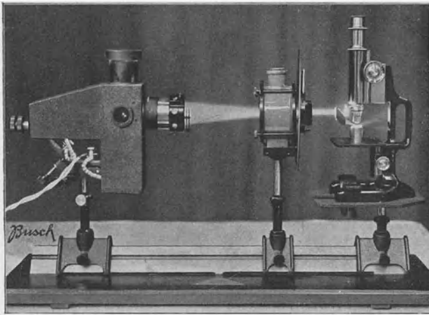
Abb. 132. Beleuchtungsanordnung für Auflichtmikroskopie mit dem Schräglitilluminator nach F. HAUSER. (Aus BUSCH-Druckschrift: Gebrauchsanweisung für den Schräglitilluminator, Abb. 1.)
