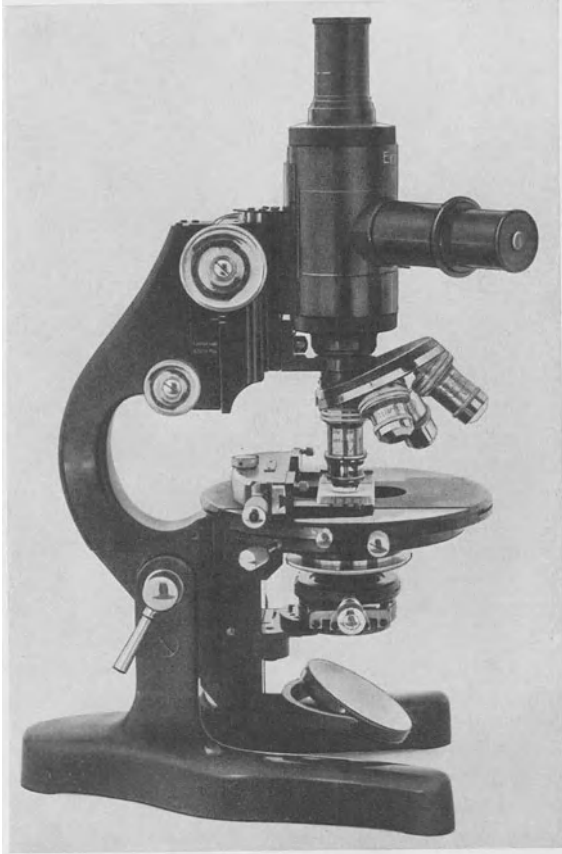
Abb. 2. Großes mikroskopisches Stativ der Firma E. LEITZ mit breitem Tubus, Hilfstubus (vgl. S. 164), Kreuztisch und ABBESchem Beleuchtungsapparat.
