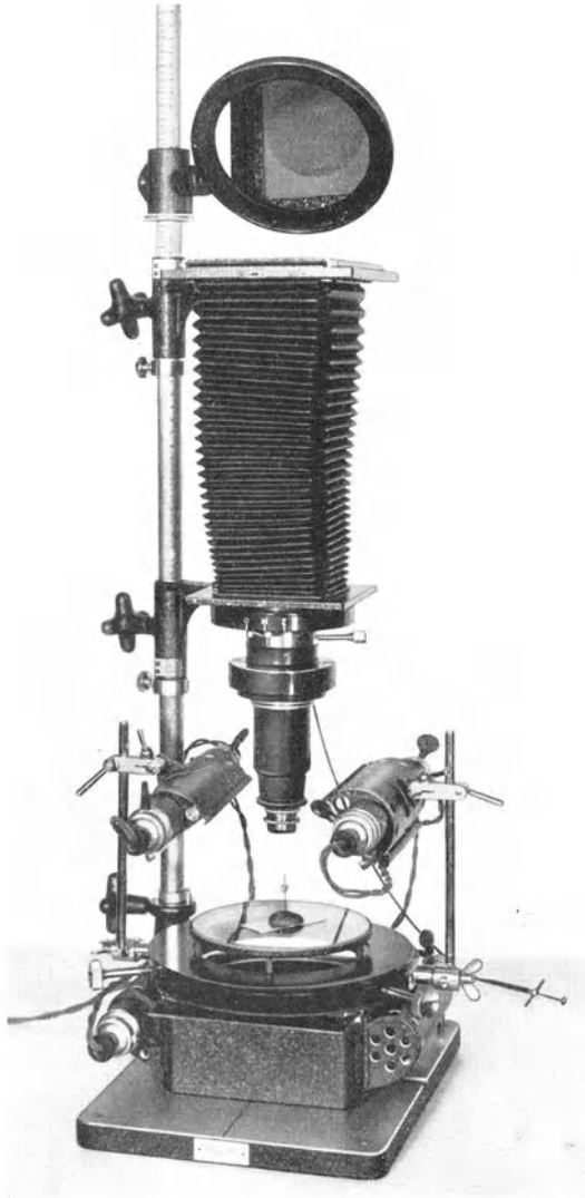
Abb. 101. Aufnahmetisch nach B. ROMEIS der Firma C. REICHERT.
