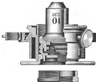
Abb. 21. Beleuchtungsobjektiv mit Zentriervorrichtung. (Aus ZEISS-Druckschrift: Mikro 400.)
