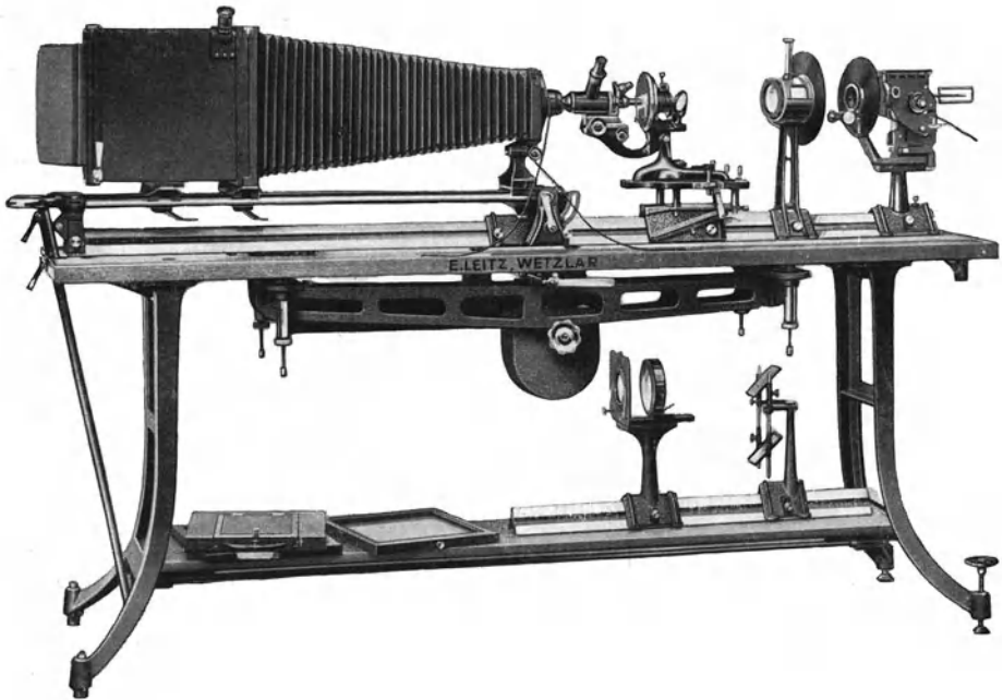
Abb. 73. Großer mikrophotographischer Apparat „Uma“ der Firma E. LEITZ in waagerechter Stellung. (Aus LEITZ-Druckschrift: Liste Nr. 50.)
