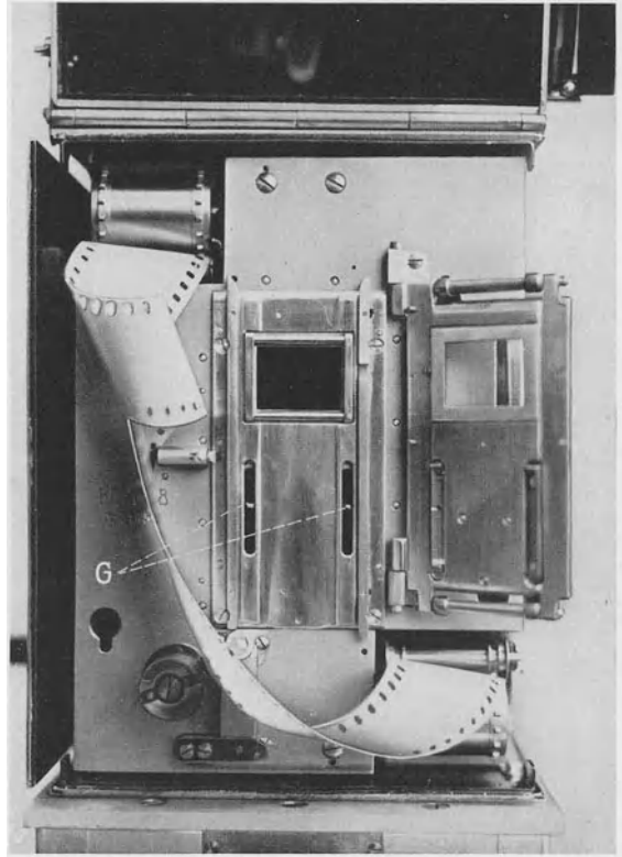
Abb. 226. Filmkanal, geöffnet, mit Bildfenster und Greifer (G). (Aus K. HÖFER [1, Abb. 129, S. 457].)
