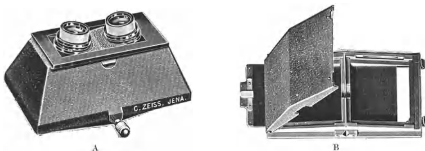
Abb. 160. Vergrößerungsaufsatz (A) und Zwillingkassette zur DRÜNERSchen Kamera. (Aus ZEISS-Druckschrift: Mikro 257.)
