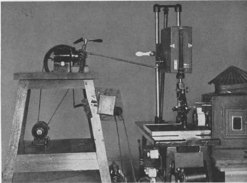
Abb. 232. Zeitraffereinrichtung mit einem Zeitraffer von DEBRIE und dem mikrokinematographischen Apparat der Firma ERNEMANN. (Aus K. HÖFER [1, Abb. 134, S. 467].)
