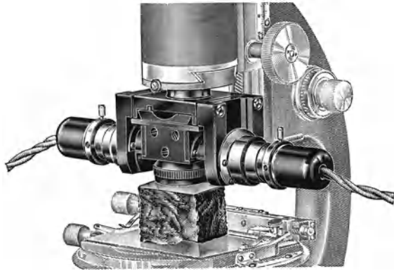
Abb. 146. Der Epi-Kondensator D. (Aus ZEISS-Druckschrift: Mikro 476.)
