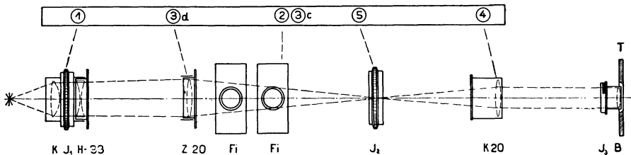
Abb. 67. Anordnung für Mikrotare und Planare und für besonders großes Sehfeld.
