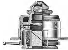
Abb. 181. Polarisationskondensator der Firma C. ZEISS mit Irisblende und abziehbarer Frontlinse.
