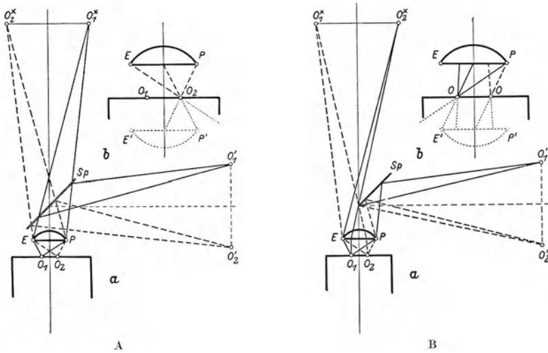
Abb. 128. Schema des Strahlenganges bei dem Vertikalilluminator nach BECK (A a) und beim Vertikalilluminator nach NACHET (B a).
