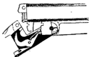
Рис. 86. Замок Гринера «фациле принцепс»
