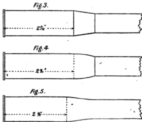
Рис. 45. Формы соединения камер со стволом
