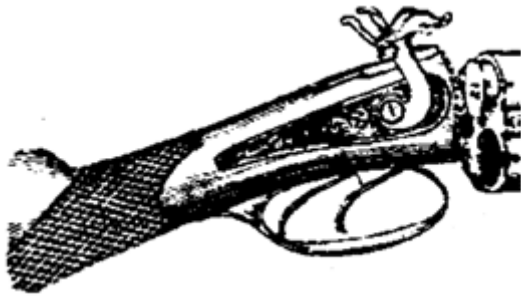
Рис. 11. Стволы на продольной оси
