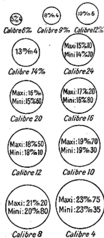
Рис. 43. Калибры французских стволов
