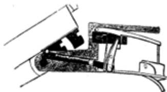
Рис. 94. Бескурковка Валькера
