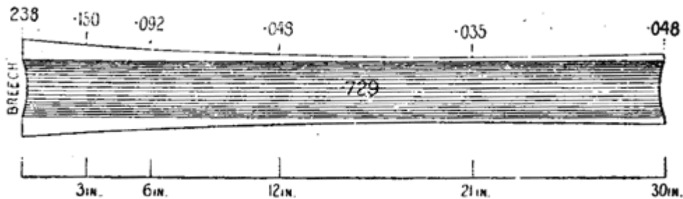
Рис. 44. Разрез ствола 12 калибра
