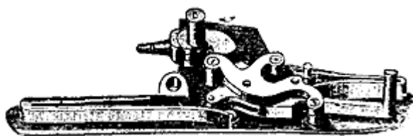
Рис. 85. Подкладной замок бескурковки Мюркотта
