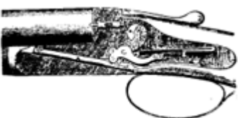
Рис. 92. Бескурковый замок Скотта
