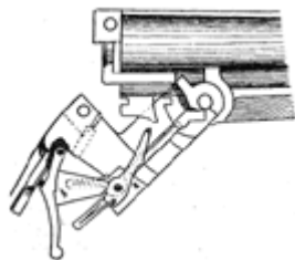
Рис. 95. Внутренний замок
