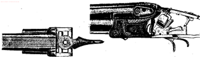
Рис. 72. Немецкий замок «Геркулес»
