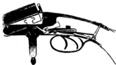
Рис. 96. Бескурковка Альпорта
