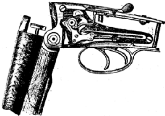
Рис. 12. Система «Фильд»
