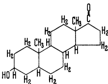
d Androsteron
