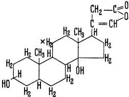
a Digitoxigenin
