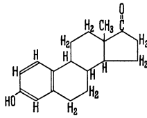
e Follikelhormon
