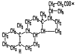
b Cholansäure
