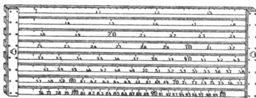
Fig. 62. Rechenschieber von Hannington .
