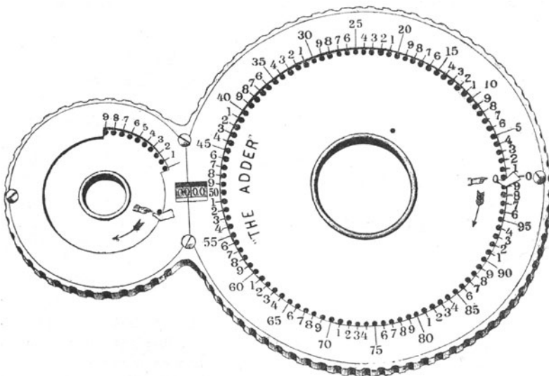
Fig. 5. Webb's Adder .
