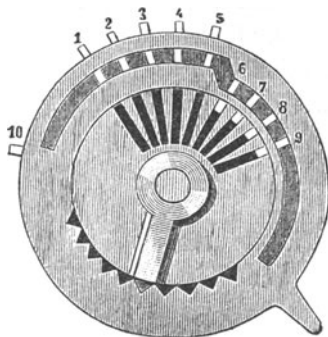
Fig. 9. Schaltrad aus Odhner's Arithmometer.
