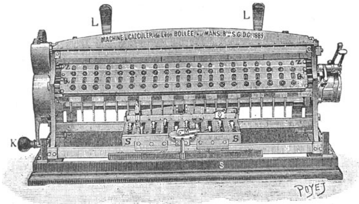
Fig. 18. Rechenmaschine von Bollée (Modell von 1888).
