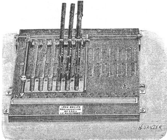
Fig. 3. Arithmograph von Bollée .
