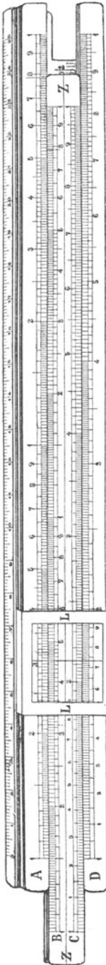
Fig. 59. Logarithmischer Rechenschieber.
