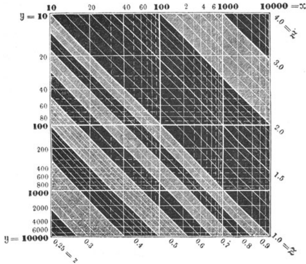
Fig. 44. Vogler's Exponententafel, y^z = x .
