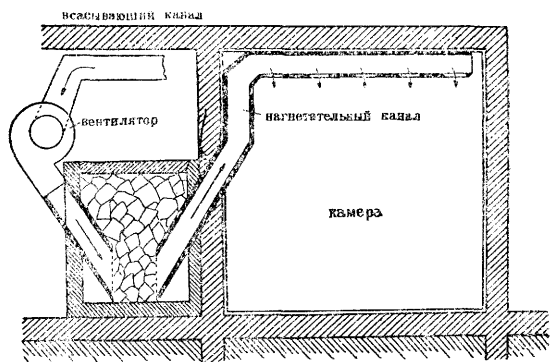
Рис. 5. Воздухоудная система охлаждения.
