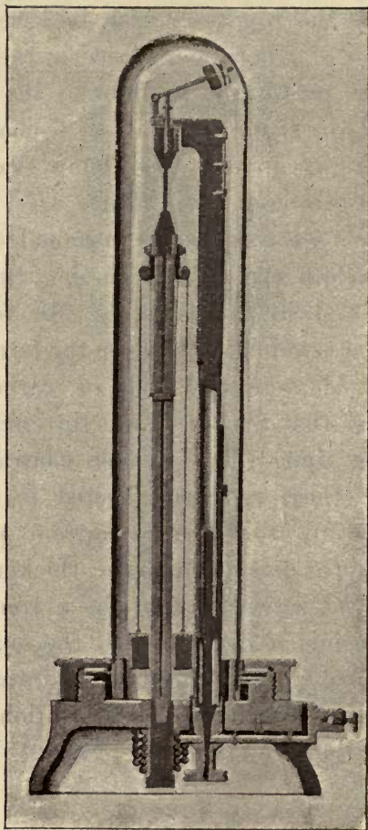
FIG. 4.—BOULIGUINE'S LAMP.
