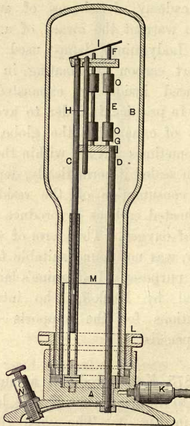
FIG. 3.—KONN'S LAMP.
