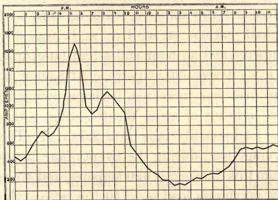
FIG. 118.—LOAD DIAGRAM.
