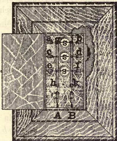
FIG. 92A.—DISTRIBUTION BOX.
