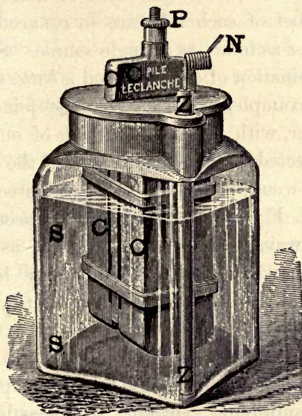
FIG. 10.—LECLANCHÉ CELL.
