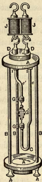
FIG. 1.—DE CHANGY'S LAMP.
