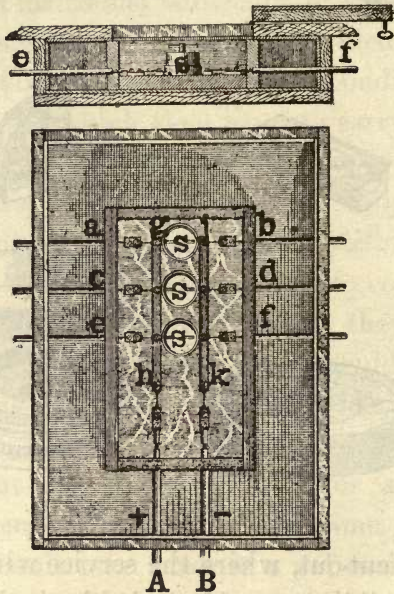
FIG. 92.—DISTRIBUTION BOX.
