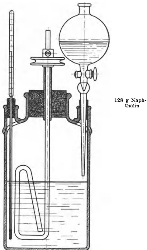
Abb. 6. Autogen geschweißter Sulfurationsapparat besonders für Oleum. Dient auch zur Darstellung von Anilin etc.
