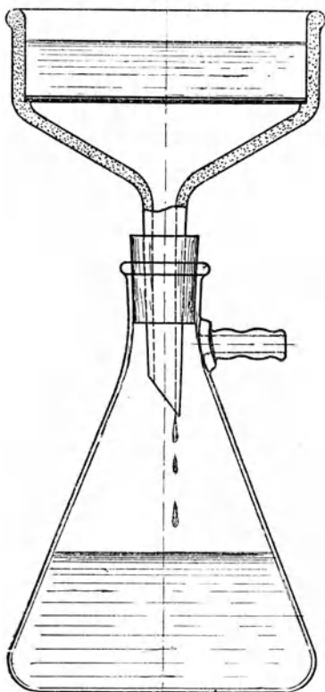
Abb. 23. Laboratoriumsnutsche.
