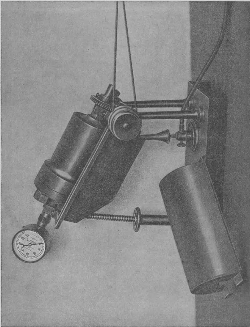
Abb. 37. Drehautoklav aus Schmiedeeisen mit Schneckenantrieb. Ausgeführt von H. Zollinger in Zürich 6. Gewicht: 11 kg; Inhalt 400 ccm; Arbeitsdruck 100 Atm.
