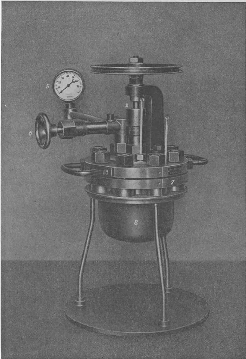
Abb. 34. Laboratoriumsautoklav mit Rührwerk. Stahlguß; Arbeitsdruck 60 Atm. Inhalt 1 Liter. Gewicht 33 kg; Gewicht des Ölbad (aus Kupfer) 11 kg. Konstrukteur: H. Zollinger, Zürich 6.
