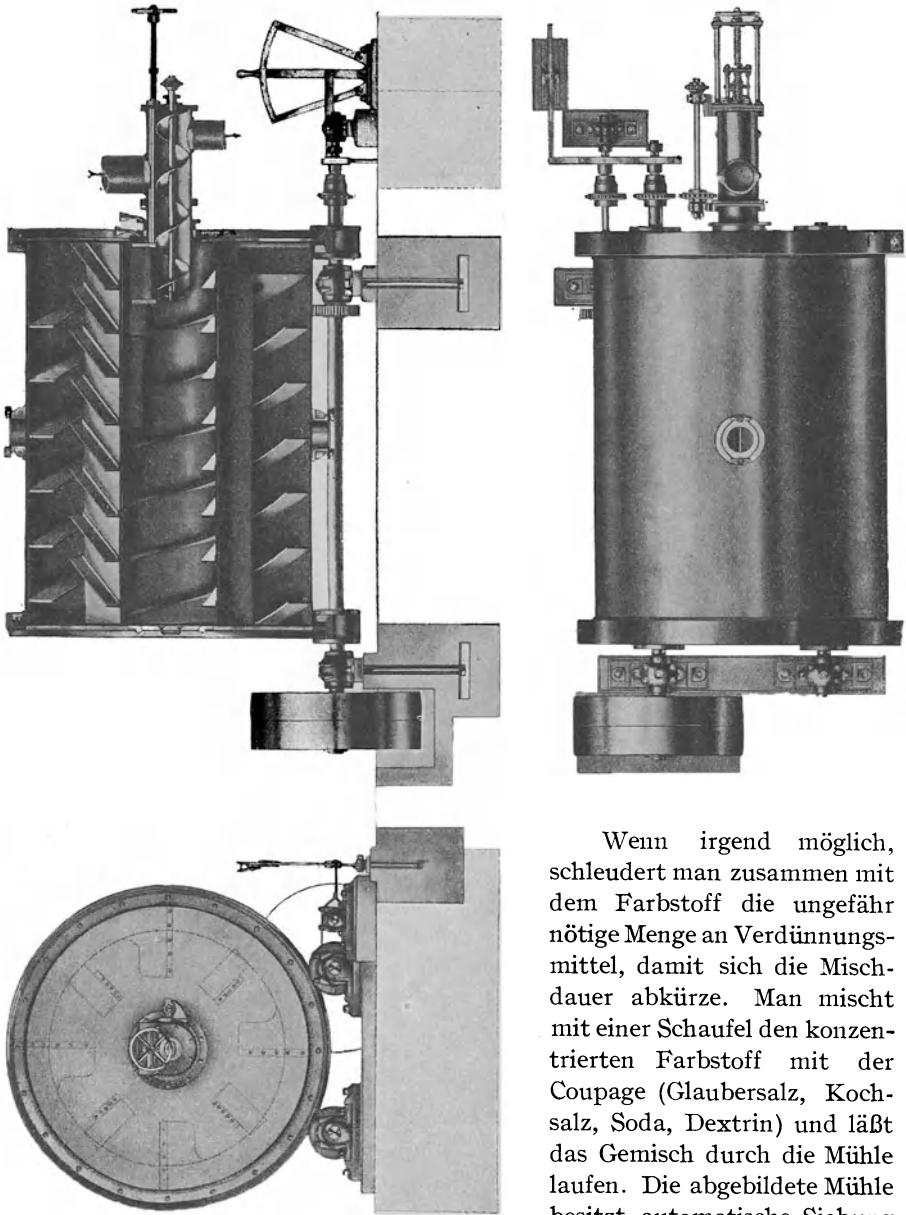
Abb. 45. Farbmischmaschine mit automatischer Füllung und Entleerung (System Hoechst).
