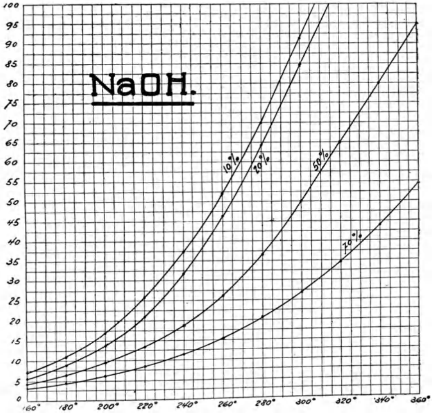
Abb. 40. Temperatur-Druckkurve für wässrige Natronlauge.
