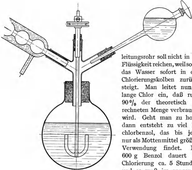
Abb. 18. Erhitzen unter Rückfluß unter Rühren. Der Tropftrichter dient zum Hinzufügen von NaOH, Säuren etc.
