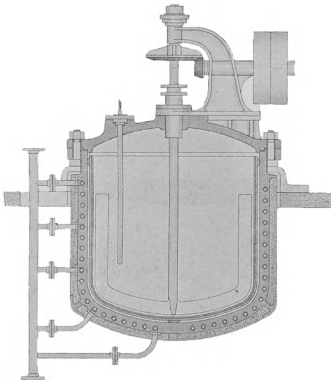
Abb. 25. Kessel mit Dampf- resp. Heißwasserheizung System Frederking.
