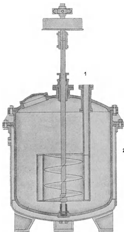
Abb. 10. Nitrierkessel mit Schraubentrührer und Außen- und Innenkühlung (Maßstab 1:30).
