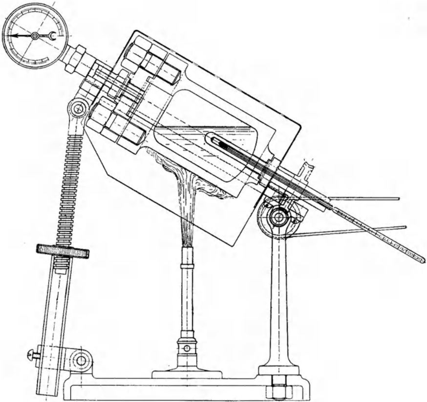
Abb. 38. Durchschnitt durch den Drehautochlor.
