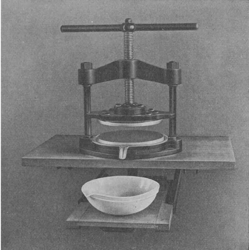
Abb. 2. Spindelpresse mit schmiedeeisernem Bügel von Preiswerk und Esser in Basel.
