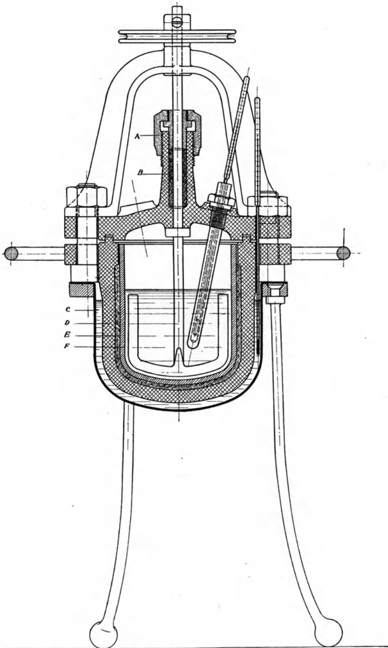
Abb. 36. Durchschnitt durch einen Laboratoriumsautoklaven. A Stopfbüchse, B Packung, C Ölbad, D Stahlgußkufe, E Bleiguß, F Einsatz.
