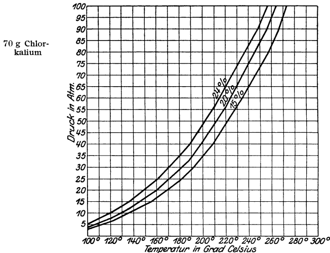
Abb. 26. Druckkurve wässrigen Ammoniaks.
