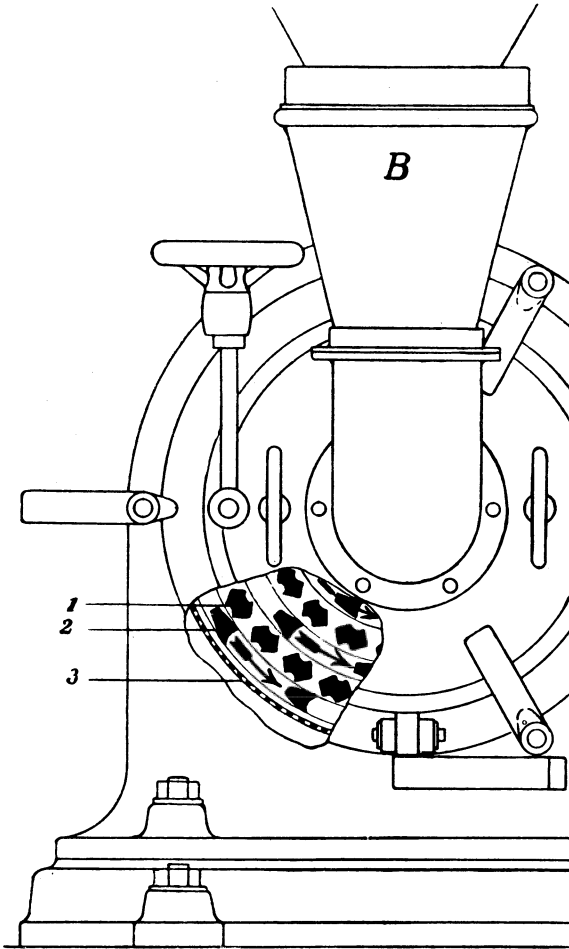
Abb. 43, Skizze des „Perplex“-Desintegrators.
