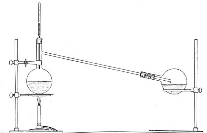
Abb. 46. Wie man hochsiedende Flüssigkeiten destilliert.
