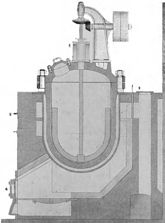
Abb. 32. Durchschnitt durch einen Autoklaven (1:40).
