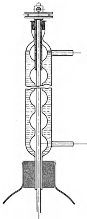
Abb. 19b. Erhitzen unter Rückfluß und Rühren mit einem gewöhnlichen Kugelkühler.
