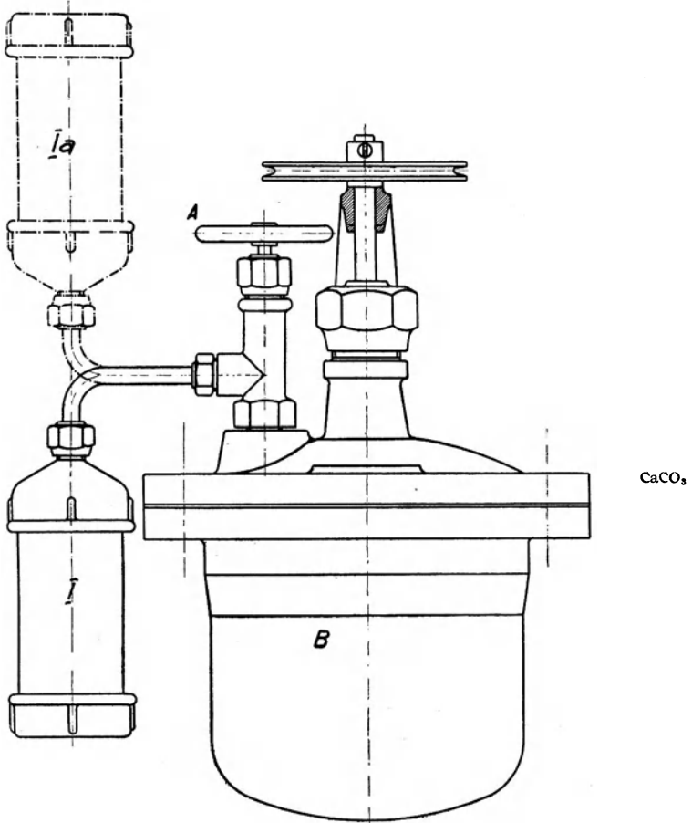
Abb. 16a. Wie man Chloralkyle in einen Laboratoriumsautoklaven einfüllt.
