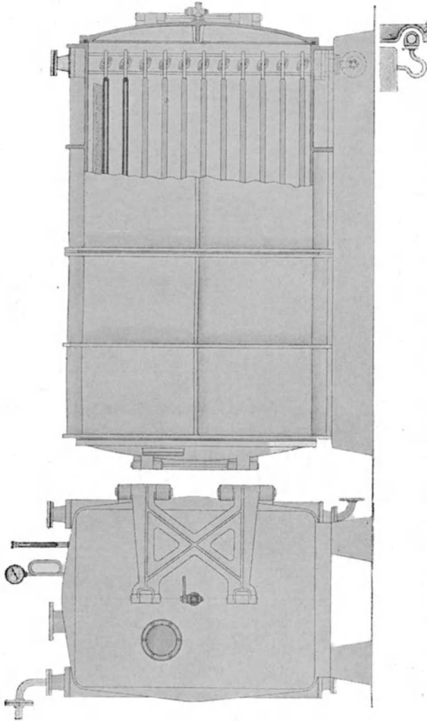
Abb. 42. Vacuumtrockenschrank für Farbstoffe: System Paßburg (1:30).
