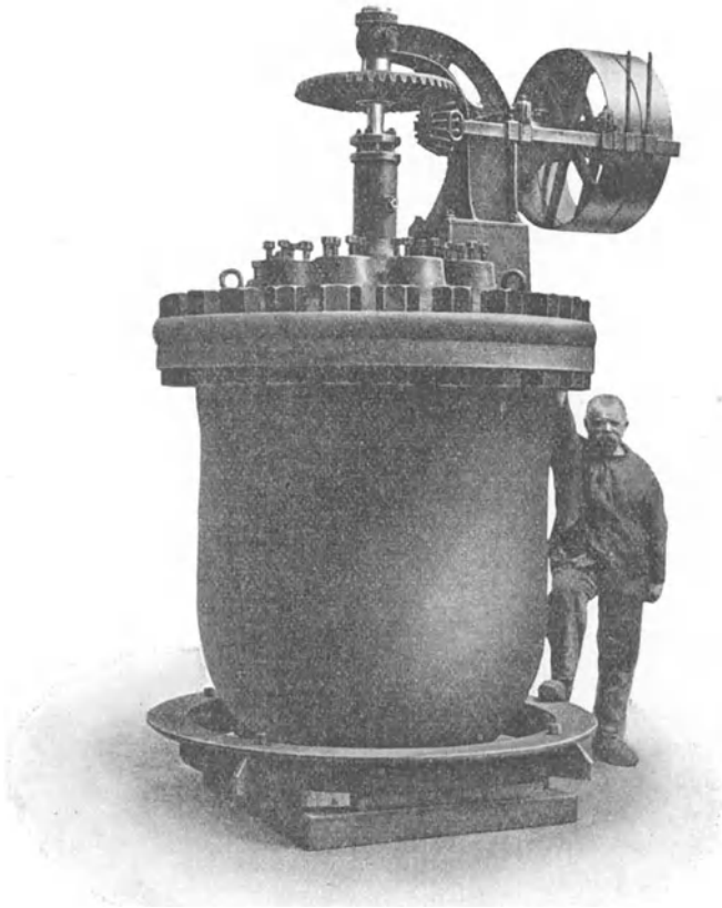
Abb. 30. Großautoklav aus Stahlguß von v. Roll.
