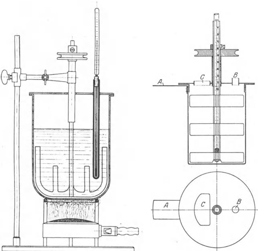
Abb. 3b. Schmelzkessel mit zentralem Thermometerrohr.
