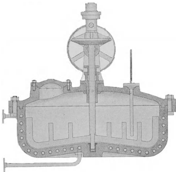
Abb. 24. Kessel mit Dampf- resp. Heißwasserheizung System Frederking.
