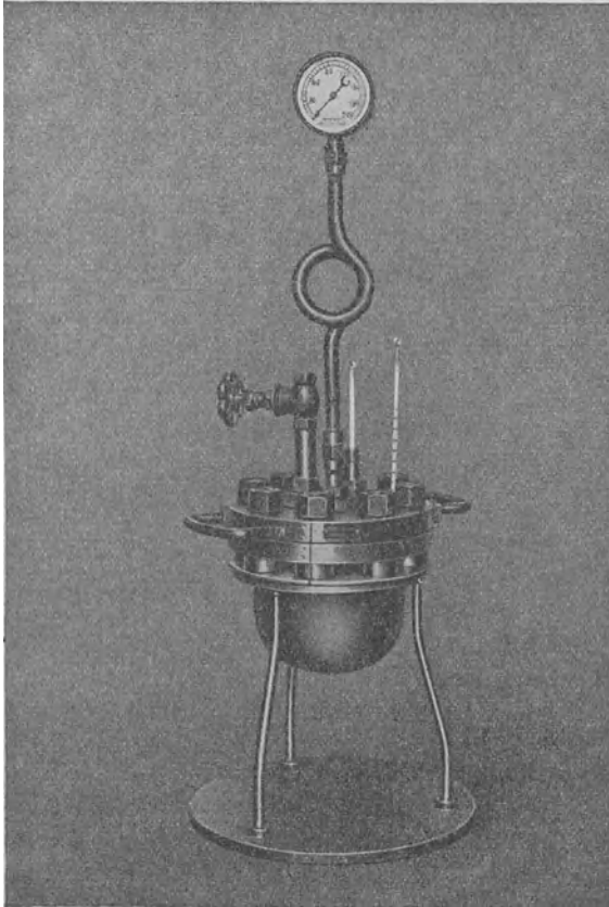
Abb. 33. Stehender Autoklav aus Stahlguß. Arbeitsdruck 60 Atm., Inhalt 1 Liter, Gewicht 30 kg.
