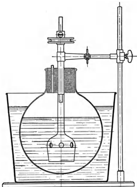
Abb. 19a. Rühren mit Wittschem Glockenrührer. Der Rührer muß sehr rasch laufen.
