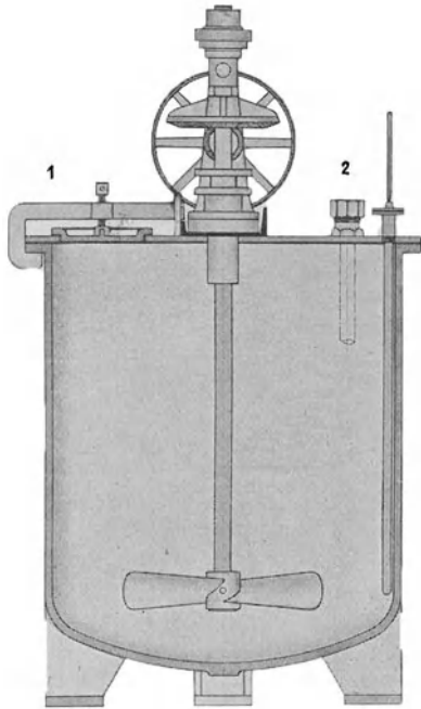
Abb. 9. Reduktionskessel mit Schraubenrührer (Maßstab 1:30).
