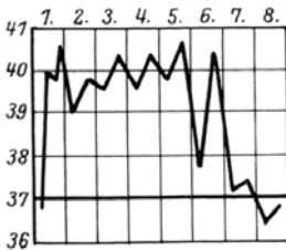
Abb. 94. Temperaturkurve bei Erysipelas.
