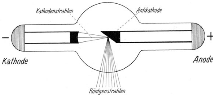
Abb. 1. Röntgenröhre.
