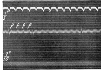
Abb. 40. Arrhythmia absoluta mit Vorhoftsflattern. Zwischen den unregelmäßigen Abständen der R-Zacken erkennt man deutlich die sehr viel häufigeren Vorhofscontraktionen (P-Zacken).
