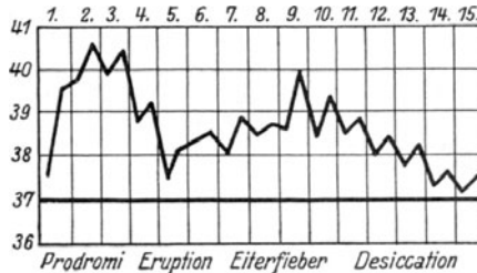
Abb. 112. Temperaturkurve bei Variola.
