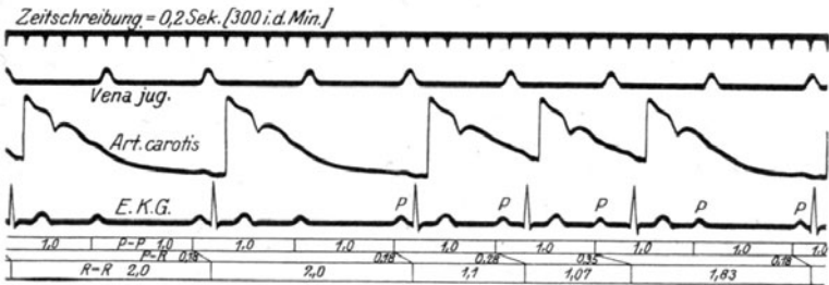
Abb. 48. Partieller Herzblock und Wenckebachsche Periode.
