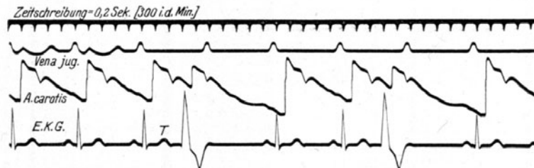
Abb. 45. Ventrikuläre gebante Extrasystolen.
