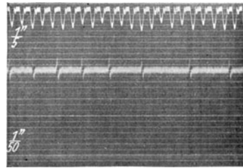
Abb. 41. Arrhythmia absoluta mit Vorhoftsflimmern.
