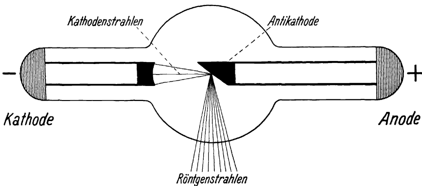
Abb. 1. Röntgenröhre.
