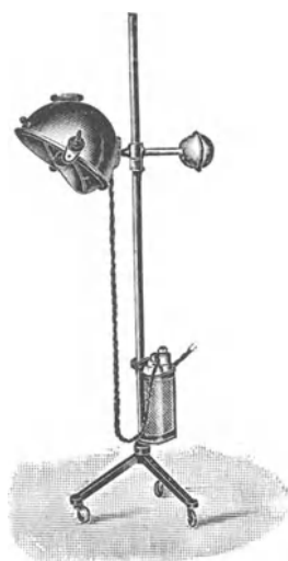
Fig. 69. Künstliche Höhensonne am Stativ (Quarzlampen-Ges.).
