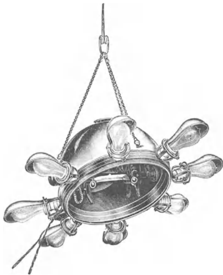
Fig. 68. Künstliche Höhensonne (hängend) mit Hagemannschem Glühlampenring (Quarzlampen-Ges.).
