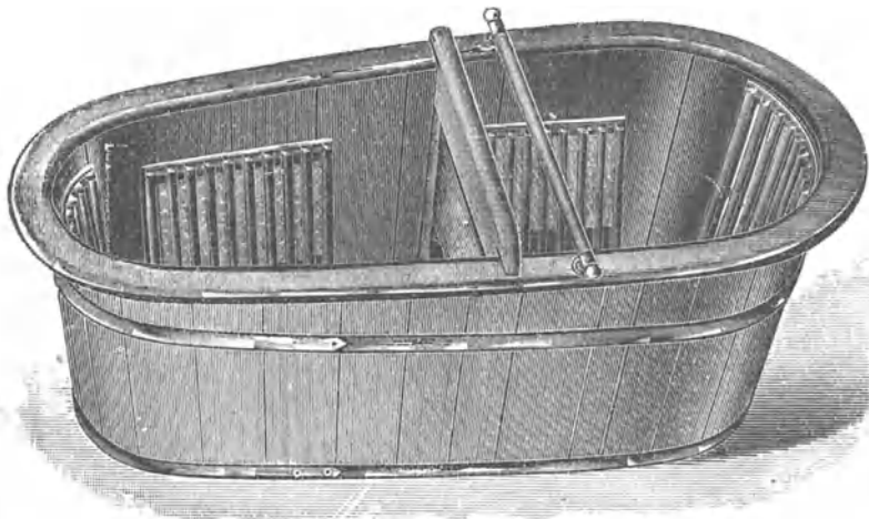
Fig. 61. Wanne für hydro-elektrische Bäder mit eingebauten Elektroden, Diaphragma und Querstange für monopolare Bäder (Sanitas).
