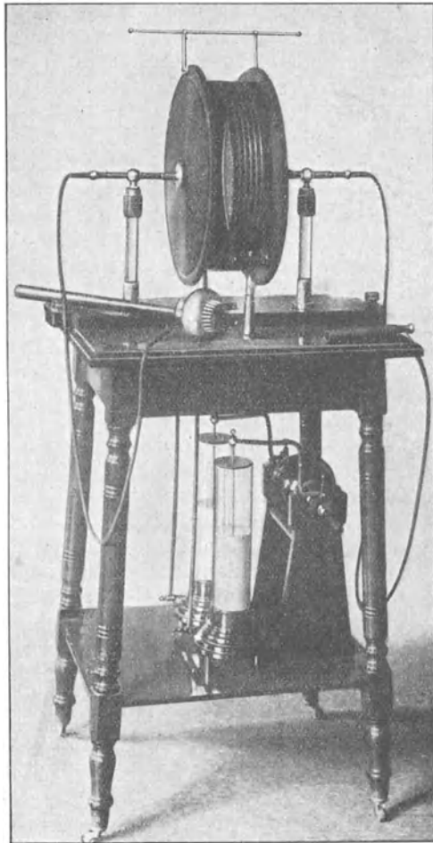
Fig. 84. d'Arsonvalapparat mit Guilleminot'schem Resonator (Sanitas).
