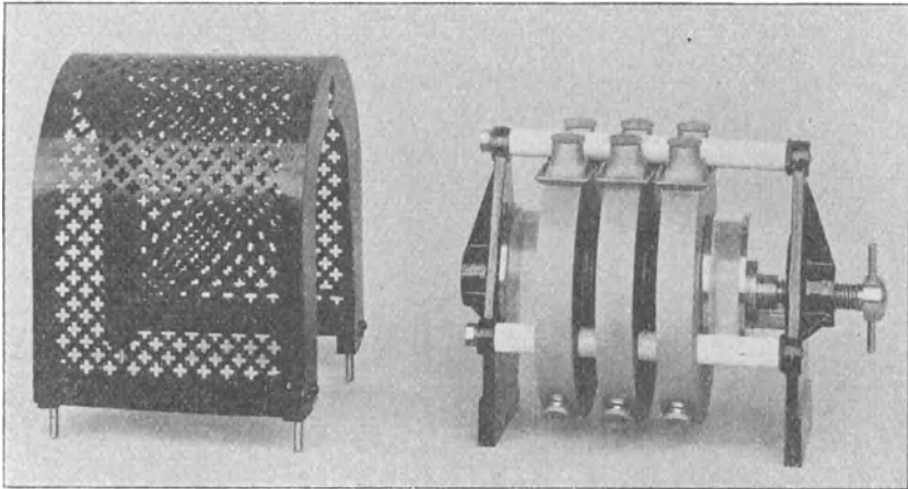
Fig. 45. Funkenstrecke des Diathermie-Apparates von Siemens & Halske. Links Schutzgehäuse.
