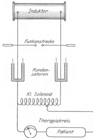
Fig. 79. Schema eines Apparates zur d'Arsonvalisation (aus Kowarschik, Elektrotherapie, 2. Aufl.).
