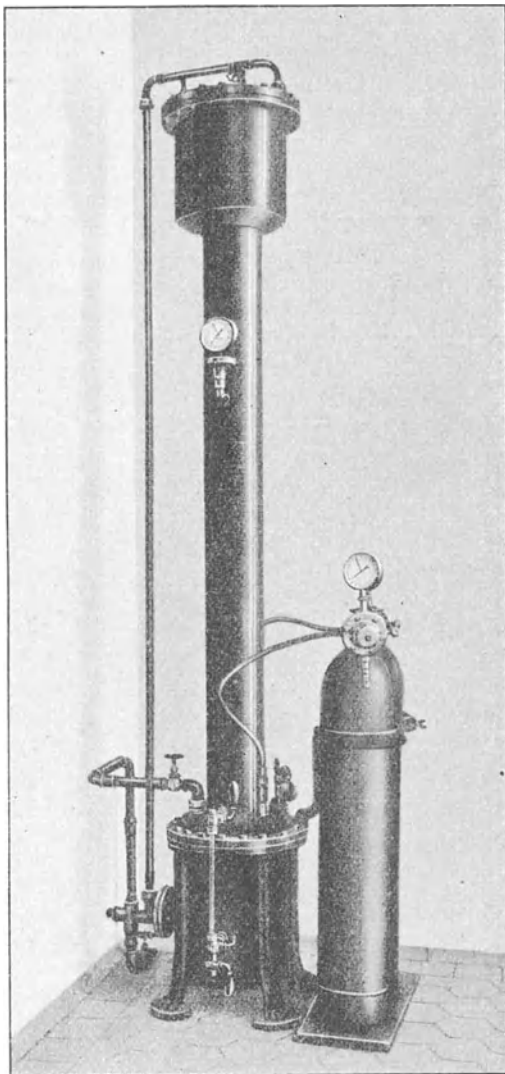
Fig. 58. Apparat zur Bereitung künstlicher Kohlensäurebäder (Fischer & Kiefer, Karlsruhe).
