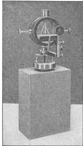
Fig. 59. Instrument zur Bestimmung des Radiumemanationsgehaltes (Fontaktoskop nach Elster & Geitel).
