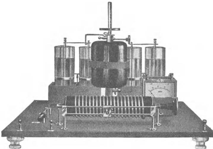
Fig. 80. d'Arsonvalapparat mit Kondensator (Leydener Flaschen), Funkenstrecke und kleinem Solenoid (Veifa-Werke).
