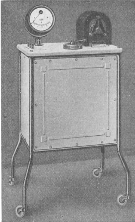
Fig. 47. Diathermieapparat (Siemens & Halske).
