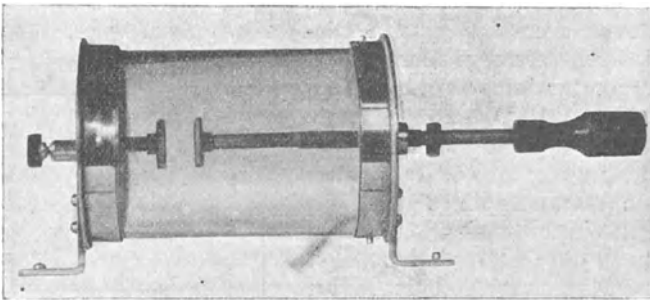
Fig. 78. Funkenstrecke eines d'Arsonval-Apparates (aus Kowarschik, Elektrotherapie, 2. Aufl.).
