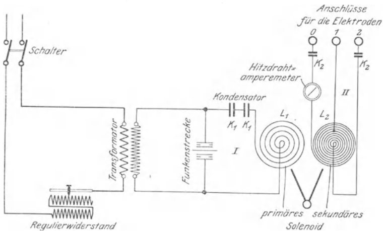
Fig. 46. Schema des Diathermieapparates von Siemens & Halske.
