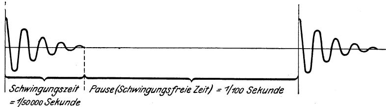
Fig. 44a. Schema der Schwingungsfolge beim d'Arsonvalschen Hochfrequenzstrom (aus Kowarschik, Diathermie 3. Aufl.).
