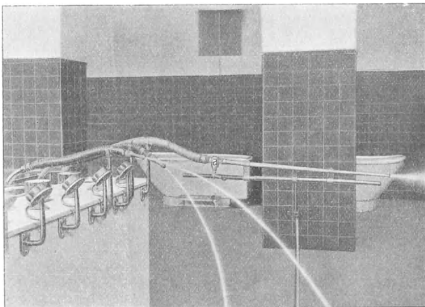
Fig. 25. Strahlenduschen (vorne) und Dampfdusche (hinten) mit Bambusstab zum Dirigieren und Vorrichtung a zum Ablauf des Kondenswassers.
