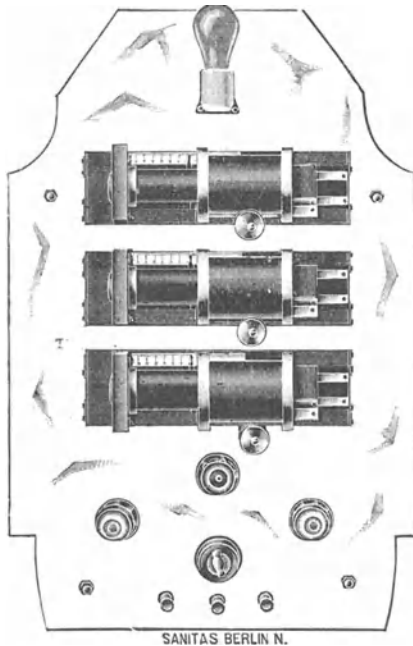
Fig. 62. Schaltbrett zur Regulierung des dreiphasigen Wechselstroms.
