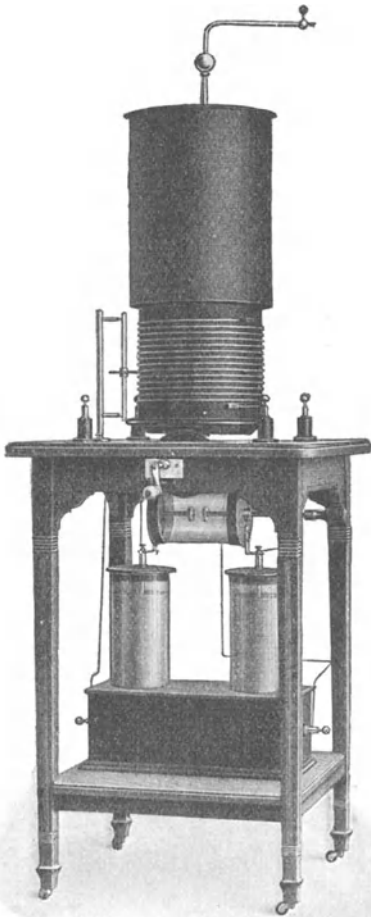
Fig. 81. d'Arsonvalapparat mit Oudinschem Resonator, Funkenstrecke und Leydener Flaschen (Siemens & Halske).
