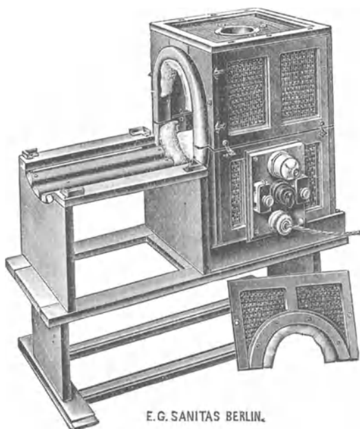
Fig. 32. Lindemannscher Elektrotherm.
