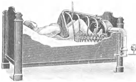
Fig. 30. Bett-Heißluftapparat (Hilzinger-Stuttgart).
