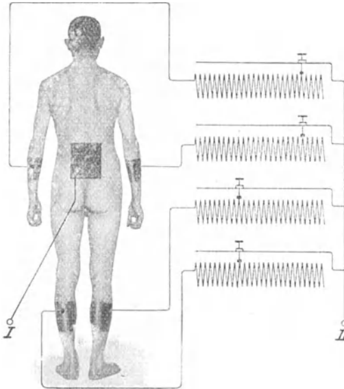
Fig. 55. Schaltungsschema für allgemeine Diathermie (aus Kowarschik, Elektrotherapie. 2. Aufl.).
