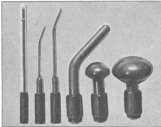
Fig. 87. Kondensatorelektroden (Veifa-Werke).
