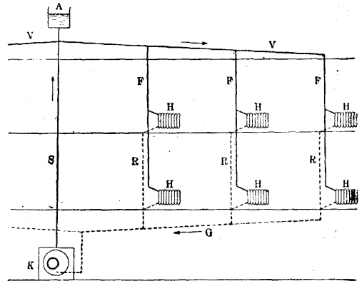
Рис. 5. Водяное отопление низкого давления. Верховая разводка: A —расширительный сосуд; F —нисходящие стояки; G —обратная магистраль; H —нагревательные приборы; K —котел; R —обратные стояки; S —восходящая труба; V —распределительная магистраль.
