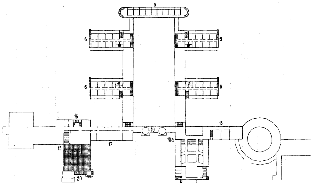
Рис. 3. План дома отдыха: a —первый этаж; б —второй этаж; 1—вестибюль с обслуживающими помещениями; 2—гостиная; 3—мытьевые души; 4—профилакторий; 5—помещение периодических выставок; 6—спальные павильоны, объединенные крытыми галереями; 7—помещение дневного пребывания суточников; 8—физкультурный зал, раскрытый летом, закрытый зимой; 9—фойе; 10—зрительный зал; 10а—балкон зала; 11—столовая; 11а—открытый летний дворик; 12—кухня; 13—внутренний зеленый дворик; 14—галерея; 15—терраса; 16—библиотека и комнаты тихих занятий; 17—лекционный зал; 18—комнаты громких игр и занятий; 19—открытый переход; 20—терраса.
