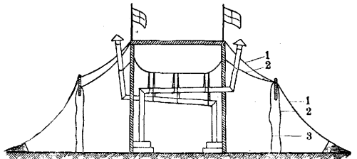
Рис. 4. Разрез гессенской палатки: 1 и 2—наружная и внутренняя оболочки; 3—колья.
