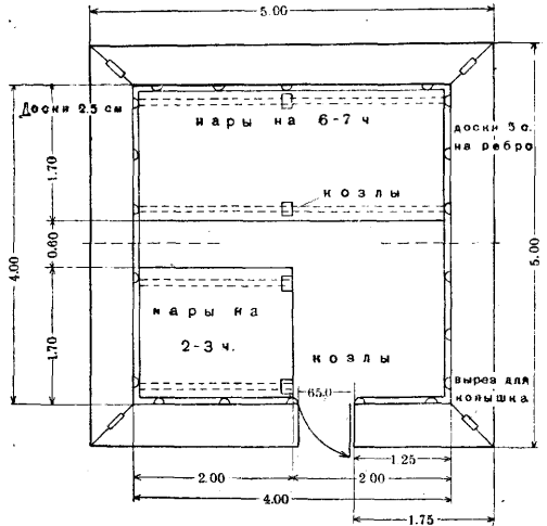
Рис. 3. Лагерная палатка.
