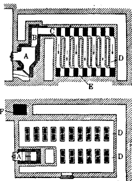
Рис. 7. Разрез кирпичного калорифера: А — топливник; В — восходящий дымоход; С — распределительный канал; D — дымовые колодцы; E — сборный канал; F — дымовая труба.
