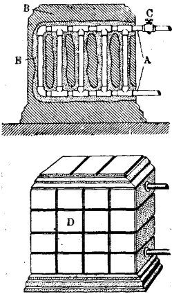
Рис. 4. Комбинированный прибор.
