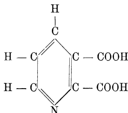
Pyridindicarbonsäure.
