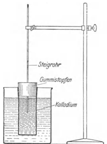
Abb. 8. Einfaches Osmometer.
