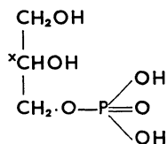
α-Glycerinphosphorsäure
