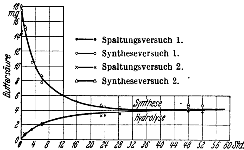
Abb. 55. Enzymatische Spaltung und Synthese von Buttersäurebutylester. (Nach RONA und AMMON.)
