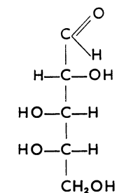
l-(+)-Arabinose
