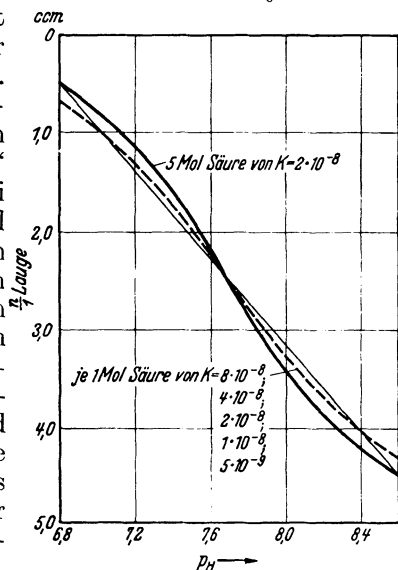
Abb. 14. Pufferkurve eines Gemisches von Säuren mit überlappenden Dissoziationskonstanten im Vergleich mit einer einheitlichen Säurelösung. (Nach HENDERSON.)
