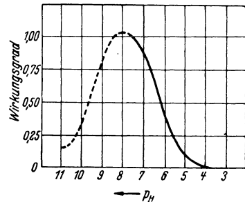
Abb. 57. Aktivitäts-ph-Kurve des Trypsins.
