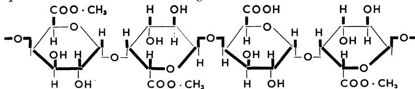
Formel eines Pektins (Methylierungsgrad 75%).
