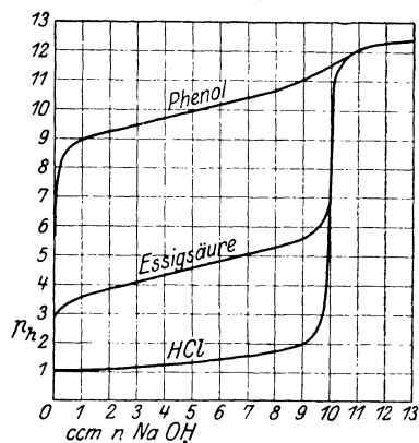
Abb. 10. Elektrotitrationskurven von Salzsäure, Essigsäure und Phenol. Je 10 ccm der betr. Säuren in n/1-Lösung werden mit steigenden Mengen von n NaOH versetzt. Die Kurven ergeben sich aus den einzelnen Laugezusätzen entsprechenden pH-Werten.
