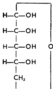
d-(−)-Ribose
