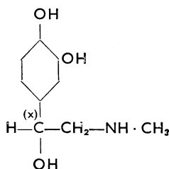
Adrenalin
