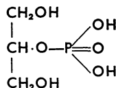
β-Glycerinphosphorsäure
