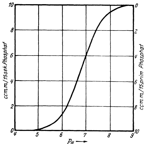
Abb. 11. Änderung des ph-Wertes in einem Puffergemisch aus primärem und sekundärem Phosphat in Abhängigkeit von dem Mischungsverhältnis der beiden Komponenten. Die Volumina der beiden Phosphatlösungen ergänzen sich stets auf 10,0 ccm. (4 ccm. prim. Phosphat + 6 ccm. sekund. Phosphat haben also einen ph-Wert von 7,0.)
