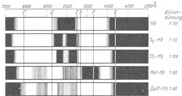
Abb. 87. Absorptionsspektren des Hämoglobins und einiger seiner Verbindungen.
