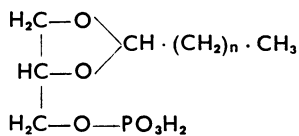
α-Plasmalogensäure
