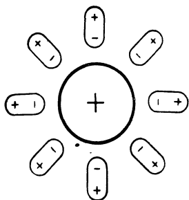
Abb. 20. Richtung der Wasserdipole um ein positiv geladenes Zentrum.
