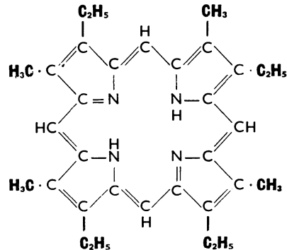
Ätioporphyrin III
