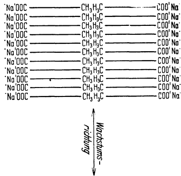
Abb. 18. Aufbau eines kolloiden Seifenteilchens.
