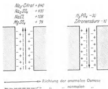
Abb. 17. Anomale Osmose. (Erklärung s. Text.) (Nach LOEB.)
