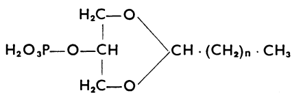
β-Plasmalogensäure
