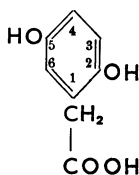
Homogentisinsäure
