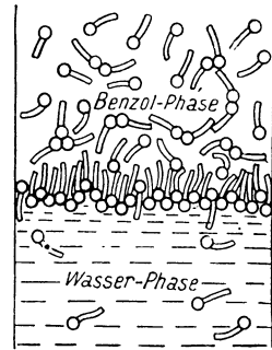
Abb. 15. Gerichtete Adsorption von Fettsäuremolekülen an der Grenzfläche Benzol-Wasser. (Nach PAULI und VALKO.)
