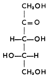
l-(+)-Ketoxylose
