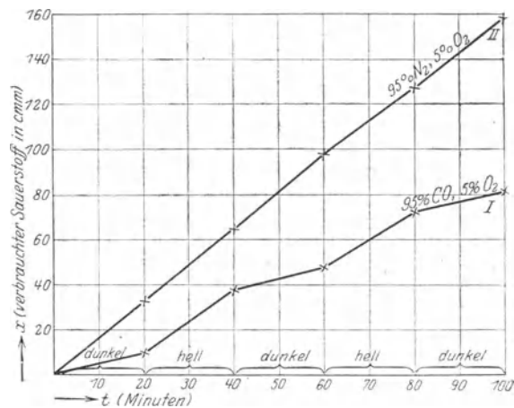
Abb. 61. Hemmung der Atmung von Hefe durch Kohlenoxyd bei Belichtung und im Dunkeln. (Nach WARBURG.)
