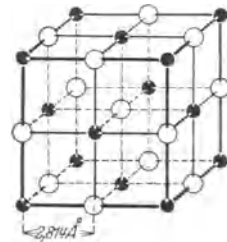
Abb. 9. Ionengitter des Kochsalzkristalls. ● Na-Ionen, ○ Cl-Ionen.
