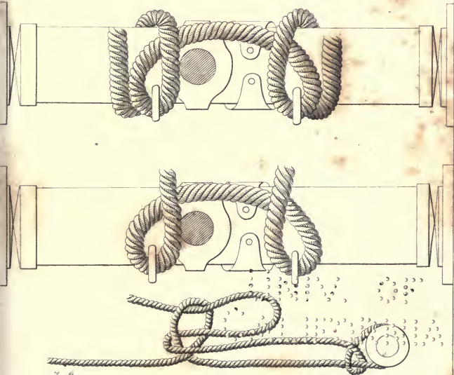
Knot for Manœuvring bolt.
