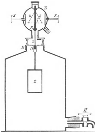
Abb. 40. Fontaktoskop.
