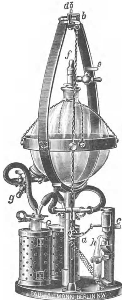
Abb. 22. Großer Wasserentnahmeapparat nach SPITTA-IMHOFF.
