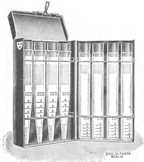
Abb. 32. Klappgestell aus Messing mit Normalplanktongläsern nach KOLKWITZ.
