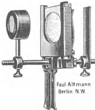
Abb. 38. Neues Planktoskop nach KOLKWITZ.
