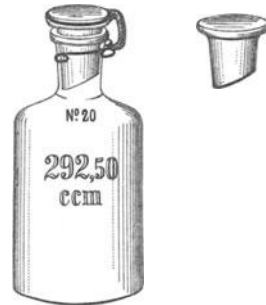
Abb. 26. Sauerstoffflasche.
