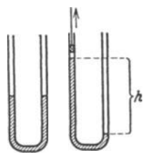
Abb. 1. Torricellis Versuch.
