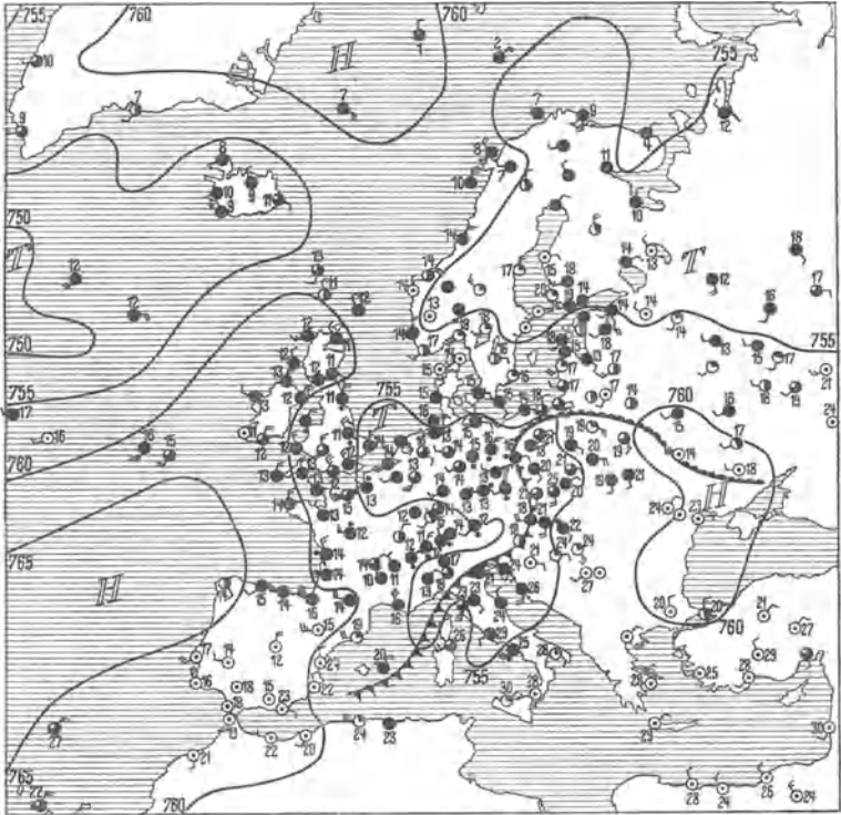
Wetterkarte vom 24. Juli 1930, 8 Uhr vorm. (Sommerliche Schlechtwetterlage für Mitteleuropa.)
