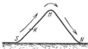
Abb. 18. Strömung über ein Gebirge (Föhn).
