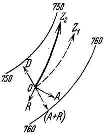
Abb. 8. Kräfteverteilung bei stationärer Bewegung (mit Reibung).
