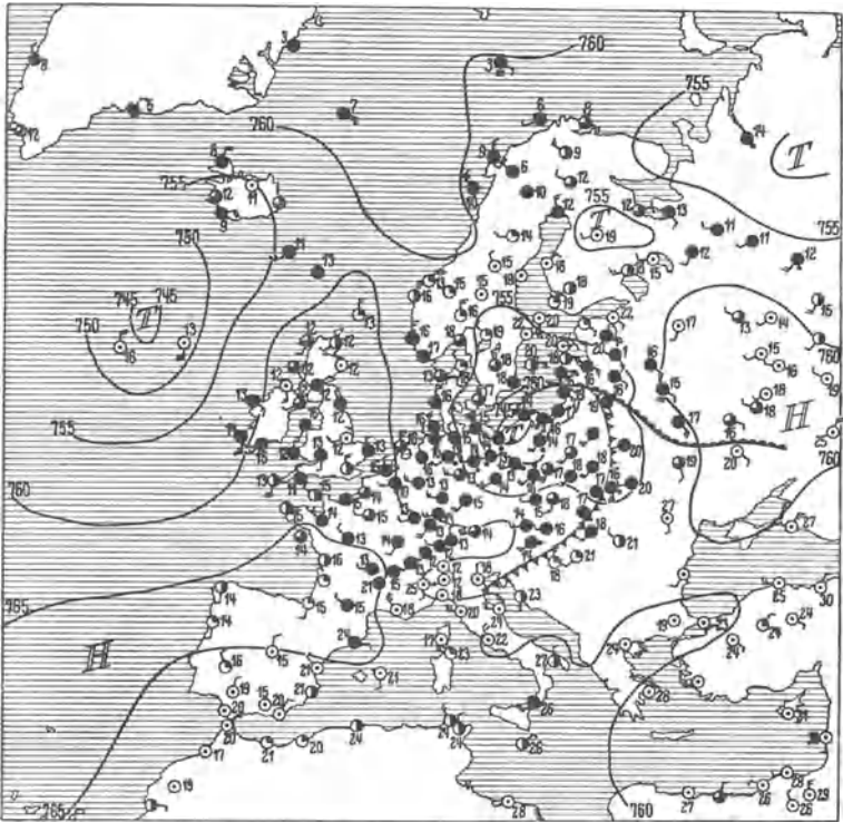
Wetterkarte vom 25. Juli 1930, 8 Uhr vorm. (Sommerliche Schlechtwetterlage für Mitteleuropa.)
