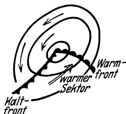
Abb. 28. Zyklone mit Warmsektor.
