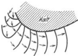
Abb. 17. Ausbreitung einer Kältewelle in Nordasien.
