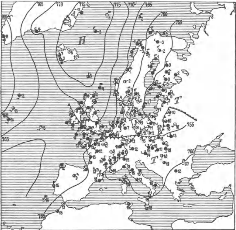
Wetterkarte vom 10. Mai 1927, 8 Uhr vorm. (Kälterückfall im Mai.)
