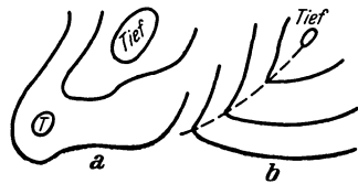
Abb. 37. Randbildungen der Zyklonen.
