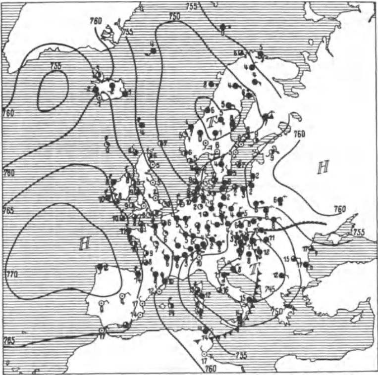
Wetterkarte vom 26. Oktober 1930, 8 Uhr vorm. (Hochwasserlage für des Gebiet der Oder.)
