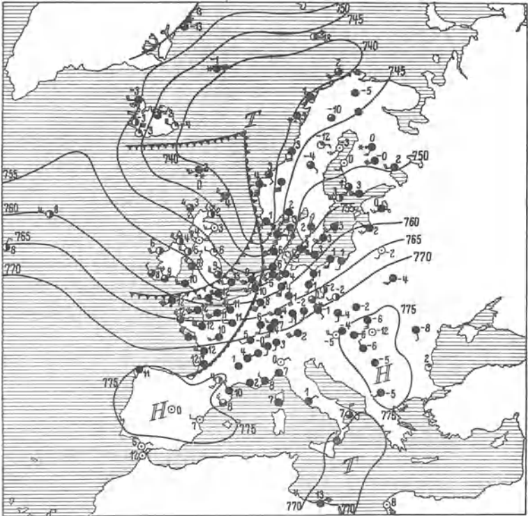
Wetterkarte vom 26. Dezember 1928, 8 Uhr vorm. (Warmsektor vor der Okklusion.)
