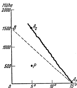
Abb. 22. Stabiles Gleichgewicht in der unteren Troposphäre.
