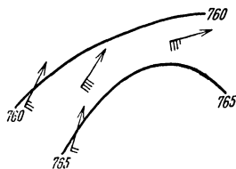
Abb. 9. Abhängigkeit der Windgeschwindigkeit vom Druckgefälle.
