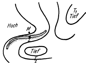
Abb. 35. Entstehung einer [Zyklone südlich der Alpen.
