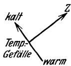
Abb. 31. Abhängigkeit der Zyklonenwanderung vom Temperaturgefälle.
