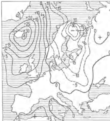
Abb. 36 c. Änderung des Luftdruckes vom 2.—3. Oktober 1931.
