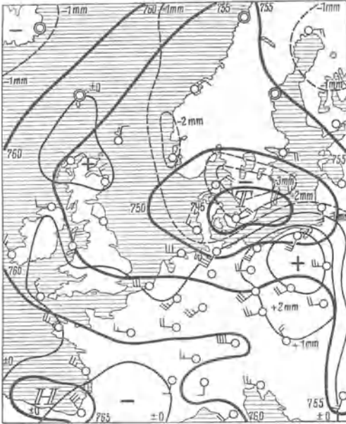
Abb. 32. Isobaren und Isallobaren.
