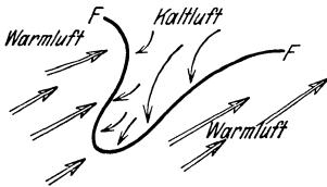
Abb. 13. Vorstoß einer Kaltluftmasse.
