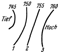
Abb. 26. Zyklonale und antizyklonale Krümmung der Isobaren.
