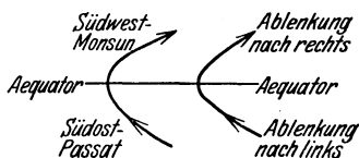
Abb. 5. Übergang des Südostpassats in den Südwestmonsun.
