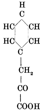
Phenyl- \alpha -Ketopropionsäure (Phenylbrenztraubensäure)
