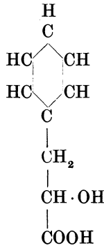
Phenyl- \alpha -Oxypropionsäure (Phenyl- \alpha -Milchsäure)
