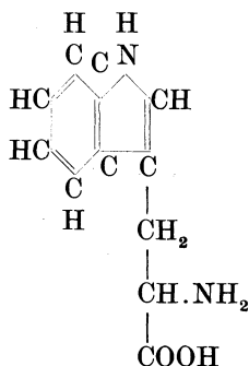
\beta -Indyl- \alpha -Aminopropionsäure (Tryptophan)
