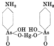
Quecksilbersalz der p-Amidophenylarsinsäure
