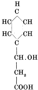
Phenyl- \beta -Oxypropionsäure (Phenyl- \beta -Milchsäure)
