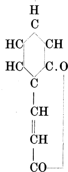
Cumarin (Lacton der o-Cumarsäure)
