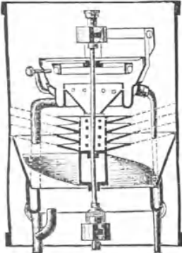
Innerer Apparat.
