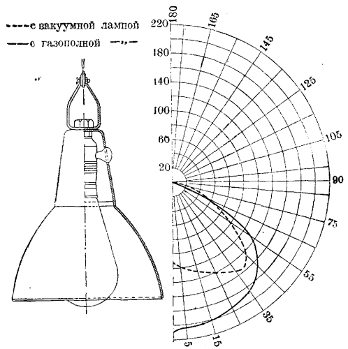
Рис. 13. Арматура «Альфа» с кривой светораспределения.
