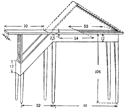
Рис. 2. Стол Делаженьера. Пунктиром обозначено положение крышки при Тренделенбургском положении. Размеры указаны в сантиметрах.
