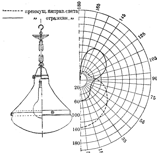
Рис. 10. Арматура «Люцетта» с кривой светораспределения.
