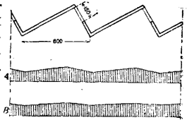
Рис. 8. Шедовые фонари с наклонным остеклением.
