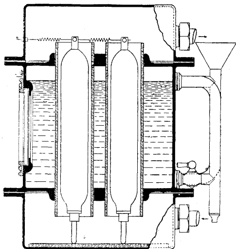
Рис. 1. Озонатор Сименса-Гальсене.
