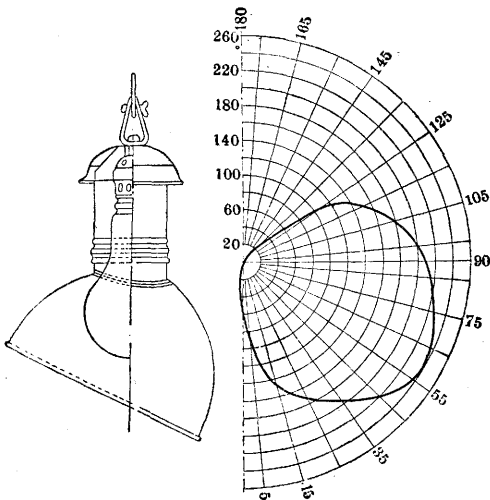
Рис. 12. Арматура «Кососвет» с кривой светораспределения.
