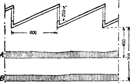
Рис. 7. Шедовые фонари с вертикальным остеклением.
