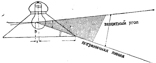
Рис. 3. Защитный угол арматуры.
