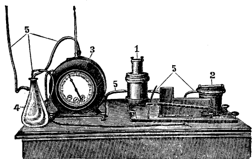
Рис. 9. Прибор Рубнера для определения проницаемости тканей для воздуха: 1—цилиндр с тканью; 2—манометр Рекнагеля; 3—газовые часы; 4—колла для регулировки давления; 5—каучуковые соединительные трубки.
