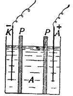
Рис. 2. А—анод; А—пространство, где образуется опресненная вода; К—катод; P—полупроницаемые перегородки.
