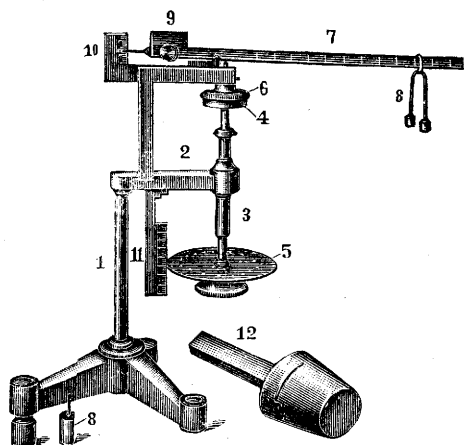
Рис. 7. Сферометр Рубнера с варьирующей нагрузкой: 1—шпатель; 2—горизонтальная перекладина с микрометрическим винтом (3); 4—стойки; 5—диск с делениями; 6—верхний столик, упирающийся в рычаг (7); 8—груз равного веса; 9—подвижной груз для уравнивания рычага; 10—шкала для уравнивания; 11—шкала для отчета миллиметров; 12—пробойчик для получения кружков ткани.
