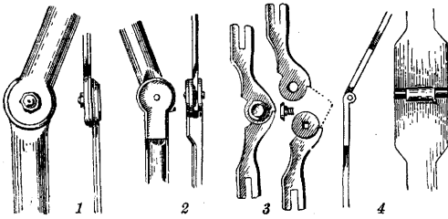
Рис. 3. Конструкции шарниров: 1—накладной; 2—вилкообразный или прорубной; 3—блокообразный (пунктиром обозначены тормозные плечики); 4—петельный.
