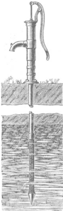
Abbildung 18. Böhrenbrunnen.
