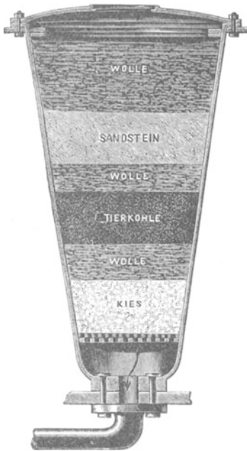
Abbildung 19. Zusammengesetztes Hausfilter.
