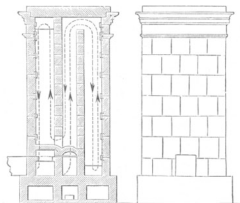
Abbildung 37. Kachelofen im Durchschnittdiagramm von vorn.
