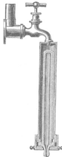
Abbildung 20. Kieselgurfilter nach Vertefeld.
