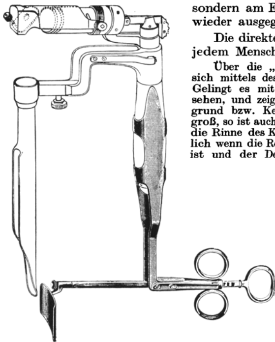
Abb. 298 Handgriff mit Lampe, Rinnenspatel und Gegendrucker. (Nach BRÜNING'S)
