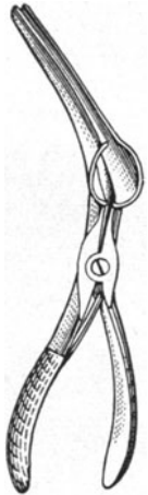
Abb. 164. Speculum für die Rhinoskopie media. (KILLIAN.) \frac{1}{4} .
