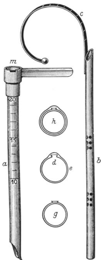
Abb 346 Verlängerbares Doppelrohr. (Nach BRÜNING'S)
