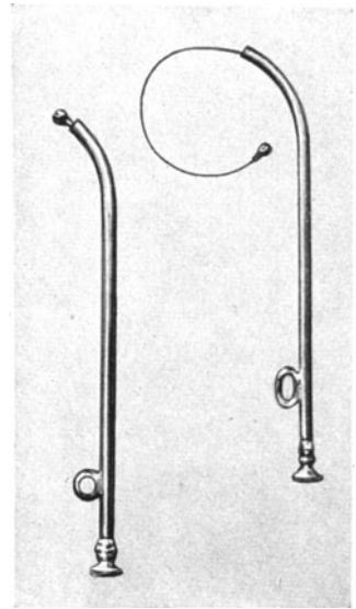
Abb 223 BELLOCSches Röhrchen
