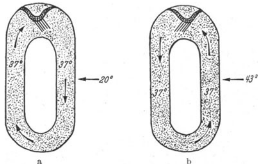
Abb. 43 a und b. Schematische Darstellung der Entstehung des calorischen Nystagmus, a bei Kaltspülung, b bei Heißspülung.
