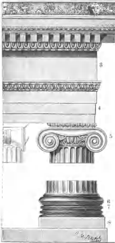
176. Das jonische System.
