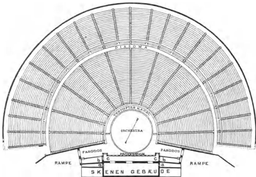
255. Grundriß des Theaters zu Epidauros, als Beispiel einer Bühnenanlage des 4. Jahrhunderts.
