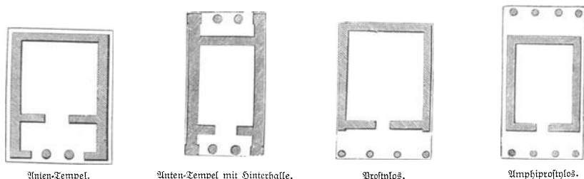
170—173. Die einfachsten Bauformen griechischer Tempel.
