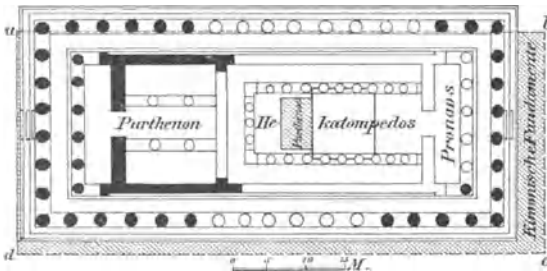
247. Grundriß des Parthenon.
