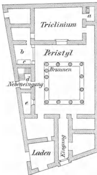
229. Griechisches Wohnhaus auf Delos (2. Jahrh. v. Chr.).
