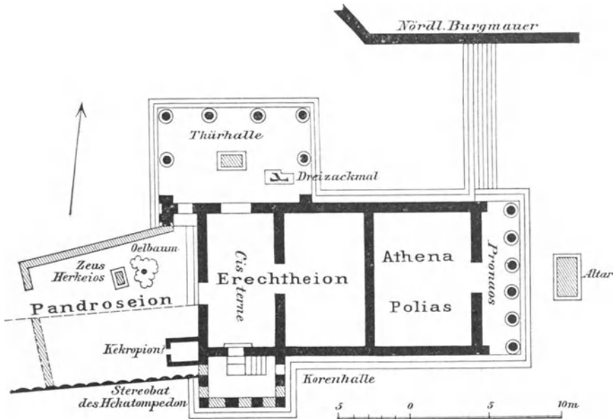
251. Grundriß des Erechtheion.
