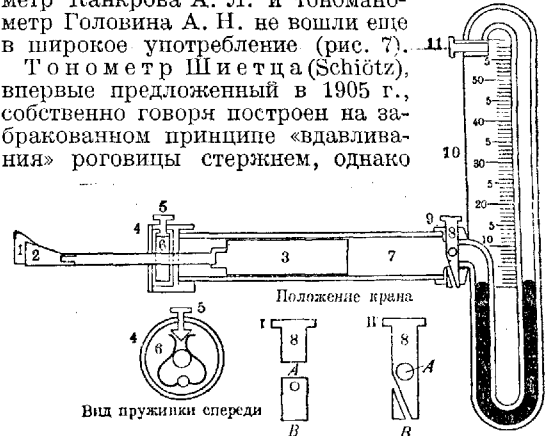
Рис. 7. Тономанометр А. Н. Головина: 1—треугольная стеклянная призмочка; 2—оправа для призмочки; 3—стеклянный поршень; 4—металлическая втулка; 5—цилиндрический стержень; 6—лириобразная пружинка; 7—стеклянный цилиндр; 8—воздуховодный край с двумя отверстиями А и В; 9—втулка для крапа; 10—манометр; 11—крап к нему.
