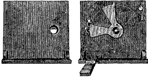
Рис. 2. Тахистоскоп А. П. Нечаева. К деревянному щиту на подставке прикреплены на оси 2 алюминиевых раздвигающихся крыла. Крылья устроены так, что, будучи подняты и удержаны особым зажимом, закрывают окно (нижним крылом). При отнятии зажима крылья падают и открывают на время испытываемому картонку, которая снова закрывается верхним крылом.
