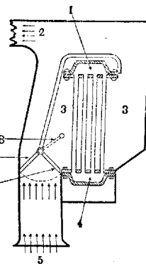
Рис. 3. Схема термотанка: 1—приток пара; 2—выход воздуха; 3—горячий воздух; 4—выход пара; 5—приток воздуха; 6—кулиса открыта; 7—кулиса открыта; 8—рукоятка регулятора.
