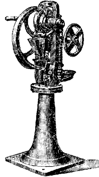
Рис. 3. Салазочная машина.
