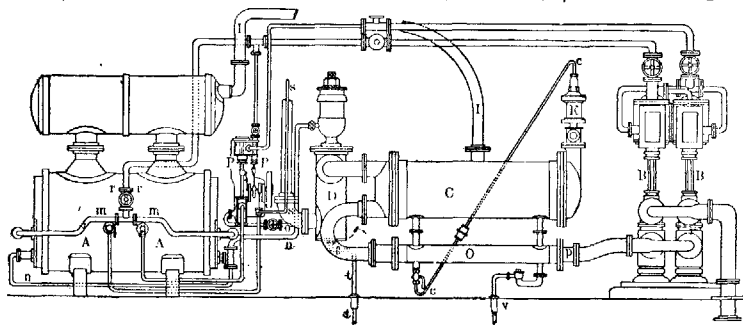
Рис. 1. Опреснитель системы Р. Круга: АА—кипятильник; ВВ—циркуляционный; С—конденсатор; D—удалитель забортной воды; O—охладитель; p—патрубок от циркуляционной помпы к охладителю; m—паровой клапан; mm—парораспределительные трубы; II—труба для отвода вторичного пара в конденсатор С; v—труба для собирания пресной воды, насыщенной газами; K—аппарат для улавливания газов, выделяющихся из циркуляционной воды при нагревании ее; ss—трубка для отвода газов, уловленных аппаратом К, в охладитель, где газы поглощаются пресной водой; tt—труба для удаления конденсационной воды из автоматического удалителя, в к-рый эта вода поступает по трубе n из нагревательной батареи; PP—питательная помпа для пополнения убыли воды в кипятильнике; ss—трубка для удаления охлаждающей воды за борт.
