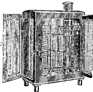
Рис. 3. Метеорограф: а — рычаг для регистрации температуры; б — влажности; с — барометрического давления.
