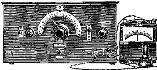
Рис. 2. Внешний вид тонвариатора для испытания слуха.
