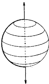
Рис. 3. Образование шаровидного тела. Черный полукруг—образующая шара. (По Fick'у.)
