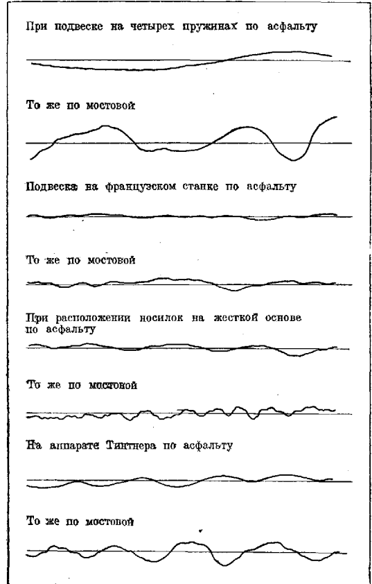
Рис. 11. Запись на кимографе толчков, испытываемых санитарными носилками при перевозке их в грузовом автомобиле.
