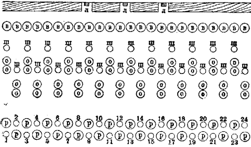
Схема горизонтального поля мультительного стола: ш — шнуры, о — отбойные сигналы, р — ключи, л — общезывывные и общетбойные сигналы.
