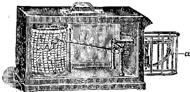
Рис. 1. Термограф Р и ш а р а: а — трубка, наполненная спиртом; б — рычаг с пишущим пером; с — барабан с разграфленной бумагой.
