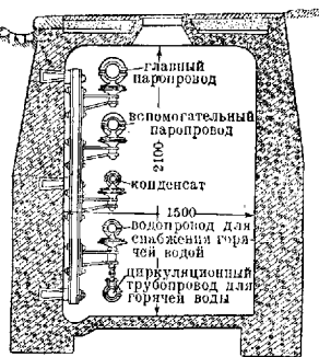
Рис. 1. Проходной подземный канал районного отопления.
