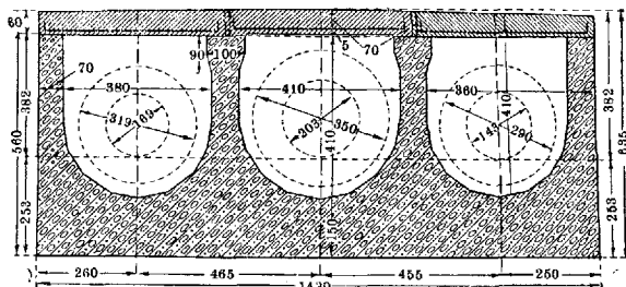
Рис. 2. Канал для трех труб.
