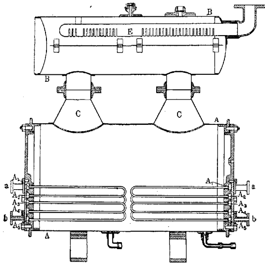
Рис. 2. Вертикальный разрез кипятыльника (AA рис. 1) опреснителя Р. Круга: AA—цилиндрический корпус кипятыльника; BB—сепаратор, соединяющийся с кипятыльником (испарителем) двумя рожками CC; паровая камера разделена перегородками на 5 независимых отделений A... A 5 , собирающихся системой нагревательных трубок, вследствие чего образуется непрерывная циркуляция пара, поступающего в выемные нагревательные батареи через паровые рожки aa; рожки bb служат для отвода наружу конденсационной воды, образовавшейся во время циркуляции пара; сепаратор BB служит для устранения выноса из кипятыльника солоноватых частей воды, что может происходить при усиленном парообразовании; унесенные паром частицы воды стекают вниз через прорезы в нижней части горизонтально расположенной паропроводной трубы E.
