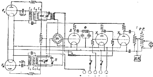
Рис. 1. Принципиальная схема тонвариатора Ленинградского научно-практ. ин-та по болезням уха, горла, носа и речи: G_1 —фиксированный генератор; G_2 —переменный генератор; L_1 —сеточная катушка; L_2 —анодная катушка; L_3 —катушка связи; C_1 —конденсатор для подстройки; C_2 —конденсатор для установки частоты (регулятор частоты); \Pi —переключатель частотных шкал; MC —мостик связи; D —детекторная лампа; \Phi —фильтр для запитывания высоких частот; У_1, У_2 —усилительные лампы; P, Г —регулятор громкости; И. Н. —индикатор напряжения; T —телефонная трубка.
