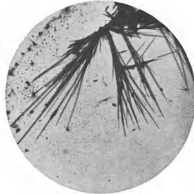
Abb. 8. Reaktionsprodukt von 4,8-Dinitro-1-naphthol mit Ammoniak.
