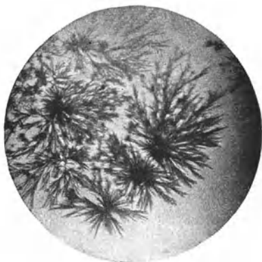
Abb. 16. Trinitroresorcin-Kalium.
