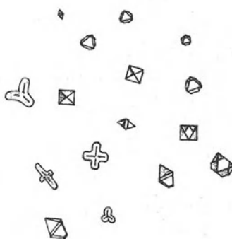
Abb. 7. Caesium-Hexachlorostannat (HUYSSÉ). Vergr. 240fach.
