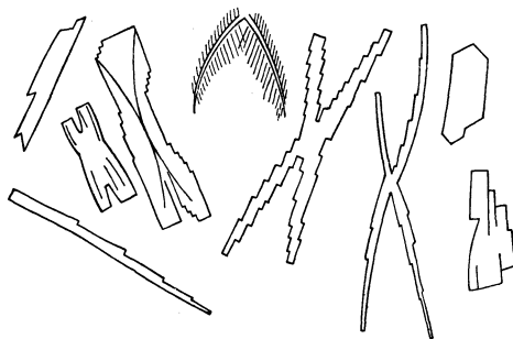
Abb. 10. Fällung mit Pikrinsäure und Kupfersulfat.
