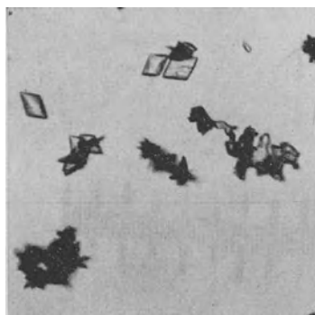
Abb. 15. Kaliumdiliturat. Vergr. 80fach.
