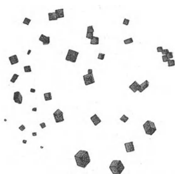
Abb. 6. Caesium-Kupfer-Bleinitrit (HUYSSÉ). Vergr. 325fach.
