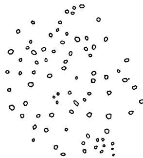
Abb. 18. Kaliumcerosulfat (HUYSSSE). Vergr. 325fach.
