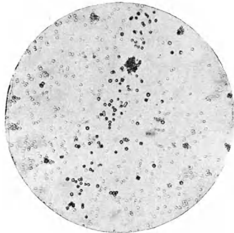
Abb. 10. Abscheidung mit Natr. umbromid und Rhodiumchlorid.
