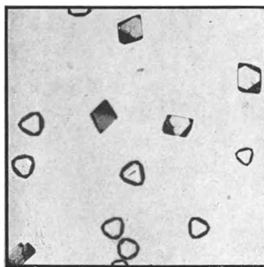
Abb. 1. Kaliumhexachloroplatinat. Vergr. 65fach (nach GEILMANN).
