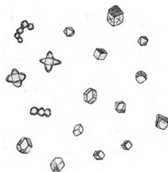
Abb. 5. Kaliumphosphormolybdät (HUYSSÉ). Vergr. 240fach.
