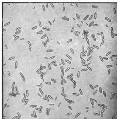
Abb. 11. Natrium-Cerosulfat (nach GEILMANN). Vergr. 260fach.
