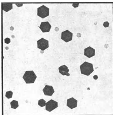
Abb. 1. Caesium-Wismutjodid (nach GEILMANN). Vergr. 80fach.
