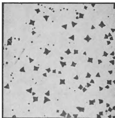
Abb. 4. Caesium-Silber-Goldchlorid (nach GEILMANN). Vergr. 90fach.
