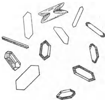
Abb. 6. Rubidiumhydrogentartrat (HUYSSÉ). Vergr. 240fach.
