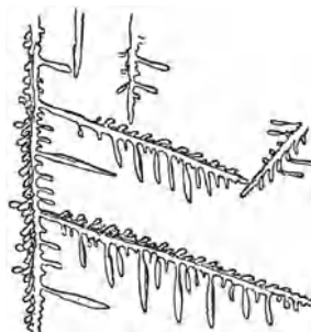
Abb. 20b. \text{NH}_4\text{Cl} -Krystalle (BEHRENS-KLEY).
