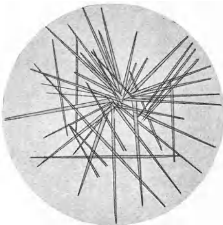
Abb. 14. Kaliumpikrat.
