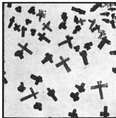
Abb. 3. Ammoniumjodatkrystalle (nach GEILMANN). Vergr. 80fach.
