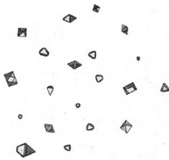
Abb. 3. Rubidiumhexachloroplatinat (HUYSSÉ). Vergr. 420fach.
