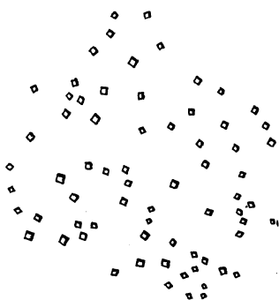
Abb. 10. Kaliumhexafluorosilicat (HUYSSER). Vergr. 325fach.
