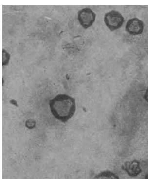
Abb. 1. Oktaedrische Krystalle des Lithiumferricyanid-Urotropinkomplexes.
