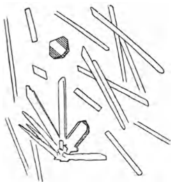
Abb. 21. \text{KNO}_3 -Krystalle (BEHRENS-KLEY).
