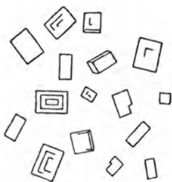
Abb. 20a. KCl- und NaCl-Kristalle (BEHRENS-KLEY).
