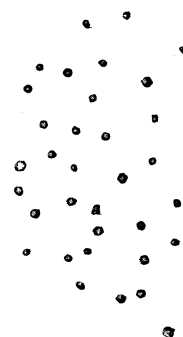
Abb. 4. Rubidium-silicomolybdat (HUYSSÉ). Vergr. 420fach.
