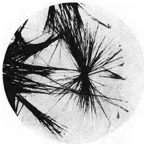
Abb. 12. Natriumpikrat.
