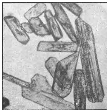
Abb. 14. Einige gut ausgebildete Krystalle von Na_2PtCl_6 \cdot 6H_2O (nach GEILMANN). Vergr. 65fach.
