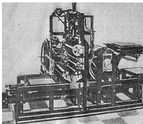
МАШИНА КЕНИГА
