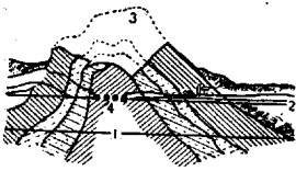
Геологический разрез (антиклиналь) источника Ваден (Швейцария): 1—уров. моря; 2—долина реки; 3—размытая антиклиналь; 4—источники (по Мухометову).
