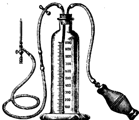
Рис. 3. Аппарат Штинцинга.
