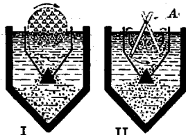
Рис. 8. Затопляемые фильтры (схемы поперечных разрезов) в лотках Эмшерских бассейнов: I—решетчатый барабан, заполненный хворостом и вращающийся 1 раз в мин.; II—подвешенный ящик, заполненный шлаком или хворостом. Воздух подводится маятникообразно качающейся дырчатой трубой (А).
