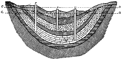
Е—скважина № 1; F—скважина № 2; H—скважина № 3; А и В—артезианские горизонты; CD—линия давления для артезианского горизонта В; C, D,—линия давления для горизонта А; А, В,—области питания; а, б, с—водонепроницаемые слои.
