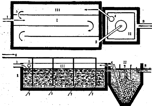
Рис. 2. Аэротанк (схема): I—аэротанк; II—отстойник; III—регенератор; 1—впуск сточной жидкости в I; 2—впуск очищенной жидкости в II; 3—впуск очищенной воды; 4—эжектор для акт. ила из II в III; 5—впуск регенер. акт. ила; 6—воздухопровод; 7—аэраторы.
