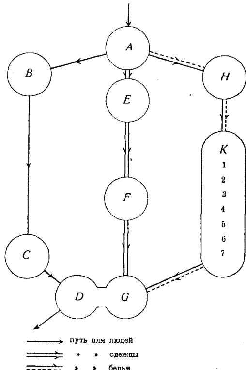
Рис. 3. Схема банно-прачечной и дезинфекционной установки: А—раздевальня бани; В—парикмахерская; С—бани; Е—приемник при дез. камере; F—дезинф. камера; Н—приемник грязного белья при прачечной; К—обработка белья (1—дезинсекция, 2—замачивание, 3—булечение, 4—стирка, 5—сушка, 6—починка, 7—глажение); G—склад чистого белья и одежды; D—одевальня.
