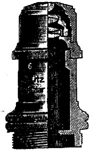
Рис. 2. Объектив представляет тип сильных сухих систем, характеризующихся передней линзой в виде полушария, за которой следуют две двойные или тройные силенные линзы.
