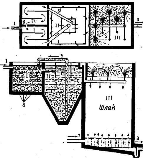
Рис. 6. «Аэрофильтр» московского типа (схема): I—аэротэнк-коагулятор; II—отстойник; III—аэрофильтры, заполненные мелким шлаком; IV—регенератор для акт. ила; 1—впуск сточной жидкости в аэротэнк; 2—впуск сточной жидкости на аэрофильтры (разбрызгиватели); 3—выпуск очищенной жидкости; 4—колосники второго днища; 5—подача ила в регенератор; 6—подача активн. ила в аэротэнк; 7—подача воздуха в аэрофильтр; 8—подача воздуха в коагулятор.
