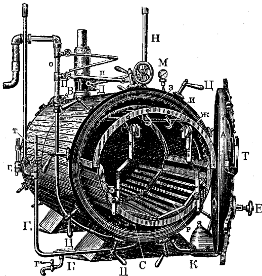
Рис. 2. Паровая дезинфекционная камера Крупина: А—дверь; В—паровая труба для змеевика; Г, Г 1 —пароотводная труба; Д и Е—вытяжное и приточное вентиляционные отверстия; К—конденсационный горшок для змеевика; М—манометр; Н—предохранительный клапан; о—паровая магистраль; П—кран для впуска пара; С—змеевик; Т—термометр аппарата; Ц—откидные болты для закрывания; э—кран для спуска конденсационной воды; е 1 —кран пароотводной трубы; жс—выдвижная тележка с откидными ножками; и—крючки для вещей; з—защитный зонт; и 1 —паропроводная труба; р—съемные деревянные решетки; т—термометр пароотводной трубы; К—вытяжная труба.
