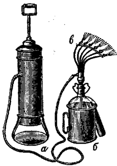
Рис. 2. Шестиструйный пульверизатор: а—пневматическ. насос; б—склянка для жидкости в футляре; в—распыляющий прибор.
