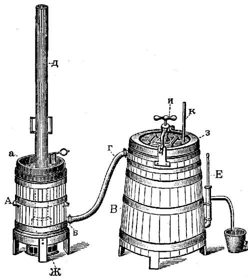
Рис. 1. Камера-бочка Юнга-Буйвида: А — самовар-парообразователь; а — тарелка для воды; Б — отверстие для выхода пара; Д — труба; Ж — зольник; В — камера-бочка; Г — гибкий шланг; з — съемная крышка; и — винт для прижатия крышки; Е и к — термометры.
