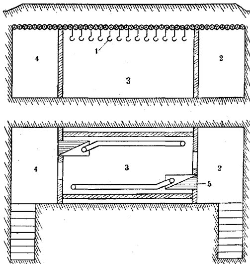
Рис. 5. Камера-землянка: 1—вешалки; 2—входы в загрузочное отделение; 3—камера; 4—выход и разгрузочное отделение; 5—топка. (По Сысину.)
