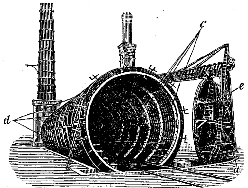
Рис. 3. Камера системы «Юлиус Пинч» для дезинфекции вагонов в Потсдаме: а—рукоятка для закрытия двигающейся по рельсам двери; с—трубы паронагревательной сети, ведущие от верхнего трубопровода и сходящиеся в общей конденсационной трубе; d—ребра камеры; e—лесенка для развешивания верхних зажимов крышки.
