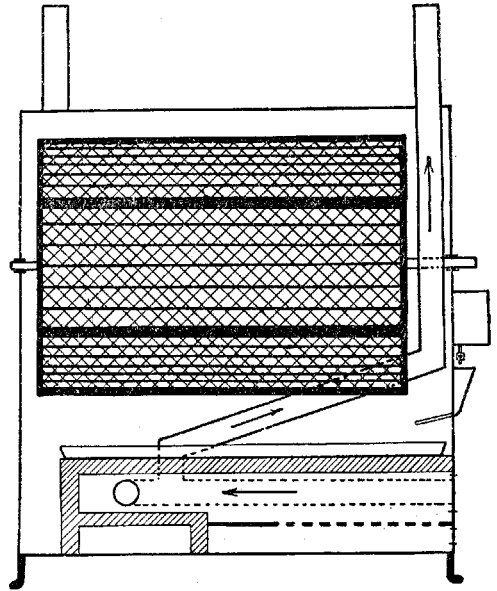
Рис. 7. Стационарный аппарат «Гелиос» и схематический продольный разрез его.
