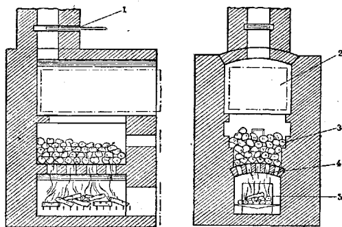
Рис. 6. Камера-каменка: 1—завдвижка трубы; 2—выдвижная кулиса; 3—бульжник; 4—кирпич; 5—топка. (По Сысину.)
