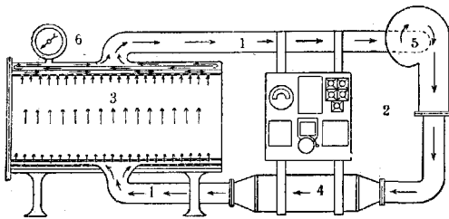
Рис. 8. Фондрановская дезинфекционная камера для быстро текущего горячего воздуха (схема): 1—каналы, подводящие горячий воздух; 2—распределительная доска; 3—камера для размещения объектов дезинсекции; 4—система грейных батарей; 5—вентилятор с электромотором; 6—пружинный термометр.
