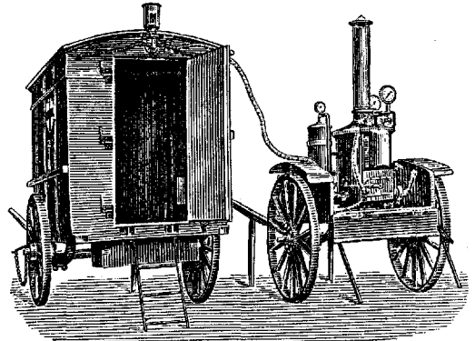
Рис. 10. Подвижная паро-формалиновая «японская» дезинфекционная камера типа Балтвода образца 1925 года с паробразователем.
