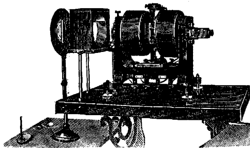
Рис. 2. Струнный гальванометр. Фотографическая запись движений струны. Слева—гальванометр, межполюсное пространство которого освещается сильным пучком света (дуговая лампа слева не изображена). Этот сходящийся пучок света превращается проецирующим окуляром в расходящийся пучок, который падает на переднюю стенку регистрирующего аппарата (ящик в верхней части изображенного справа прибора). Внутри ящика помещен рулон светочувствительной бумаги, развертывающийся с помощью электромотора (внизу).
