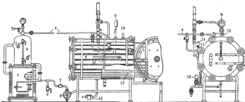
Рис. 4. Схема установки дезинфекционной камеры «Универсаль» с парообразователем системы Прохорова образца 1928 г.: 1—парообразователь; 2—змеевик парообразователя; 3—паро-водный резервуар; 4—питательная паровая трубка; 5—пробные краны; 6—насос; 7—питательный клапан; 8—камера; 9—мановакуумметр; 10—воздушный фильтр; 11—форсунка; 12—змеевик камеры; 13—предохранительный клапан; 14—воронка для формалина и аммиака; 15—конденсационный горшок.
