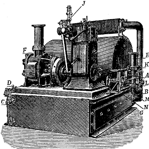
Рис. 13. Аппарат Клейтона: А и F—кран для выпуска газа; В и D—отверстия для термометра; С—впуск воды в холодильник; Е—трубка для воздуха; G—холодильник; J—рычаг; К—рычаг «в помещении»; L—рычаг «к генератору»; М—рычаг «свежий воздух»; N—рычаг «к холодильнику».
