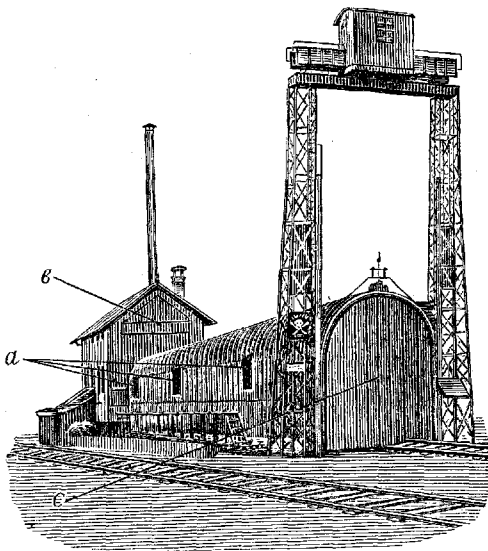
Рис. 4. Ангар системы Бюринг для дезинфекции и дезинсекции вагонов в Бслаграде: а—распылительные ниши; б—машинное здание; с—затвор.
