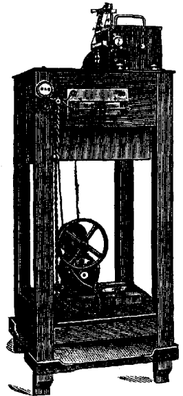
Рис. 2. Струнный гальванометр. Фотографическая запись движений струны. Слева—гальванометр, межполюсное пространство которого освещается сильным пучком света (дуговая лампа слева не изображена). Этот сходящийся пучок света превращается проецирующим окуляром в расходящийся пучок, который падает на переднюю стенку регистрирующего аппарата (ящик в верхней части изображенного справа прибора). Внутри ящика помещен рулон светочувствительной бумаги, развертывающийся с помощью электромотора (внизу).
