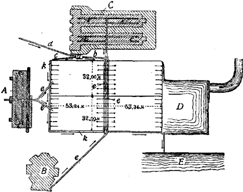
Рис. 2. План грязерегенеративных бассейнов в Ст. Руссе: А и В—ванны бассейна № 3 и № 2; С—грязелечебница имени Н. А. Семашко; D и E—нижнее и среднее озера; а—отстойник; б—лоток в бассейн с минеральной водой; с—лоток к водянному колесу; d—трубопровод из источника; e—грязевые лотки; k—водоотводный лоток.
