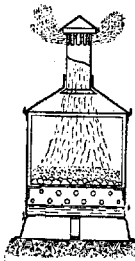
Рис. 10. Аппарат Заусайлова и Теличенко в разрезе.
