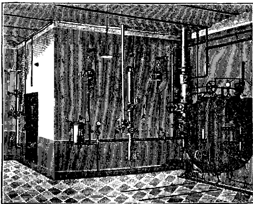
Рис. 9. Общий вид и внешнее оборудование бетонной паро-формалиновой дезинфекционной камеры японского типа: а — паровая магистраль; б — трубка для впуска пара; в — форсунки; г — вытяжная вентиляционная труба; д — паровой побудитель; е — эксгаузер; и — сосуды для формалина; жс — дверь в чистое отделение помещения; з — приточные вентиляционные отверстия.
