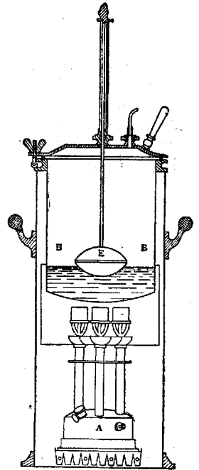
Рис. 4а. Аппарат Хотона в разрезе: А—керосиновый примус; Б—формалиновый бак; Е—поплавок.
