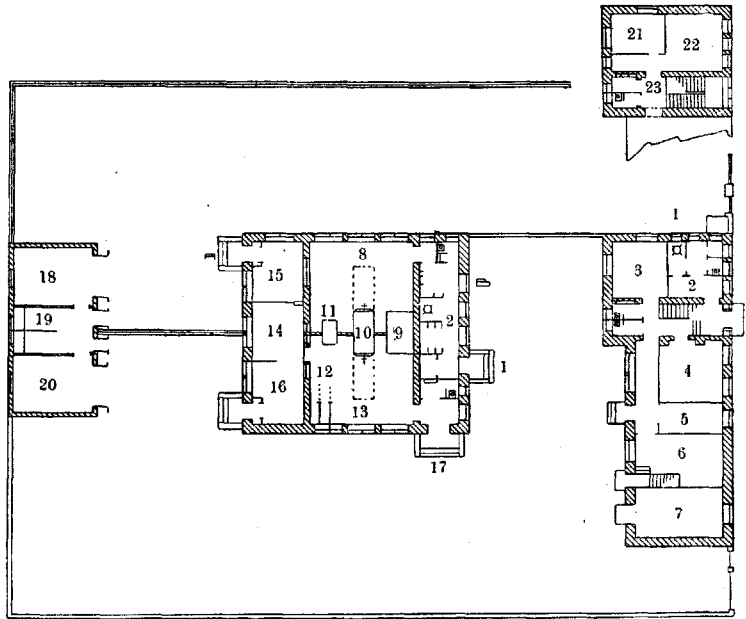
Рис. 3. Проект дезинфекционного пункта: 1—вход в шлюз; 2—шлюз; 3—сторон; 4—капцелярия; 5—хранение хлорной извести и т. п.; 6—склад химических веществ; 7—сарай; 8—инфекционное отделение; 9—японская камера; 10—паровая; 11—бучильник; 12—сушильня; 13—чистое отделение; 14—заведующий; 15—сдача; 16—выдача; 17—вход в чистое отделение; 18—инфекционный транспорт; 19—стойла; 20—чистый транспорт; 21—дежурный персонал; 22—санитары; 23—умывальня.
