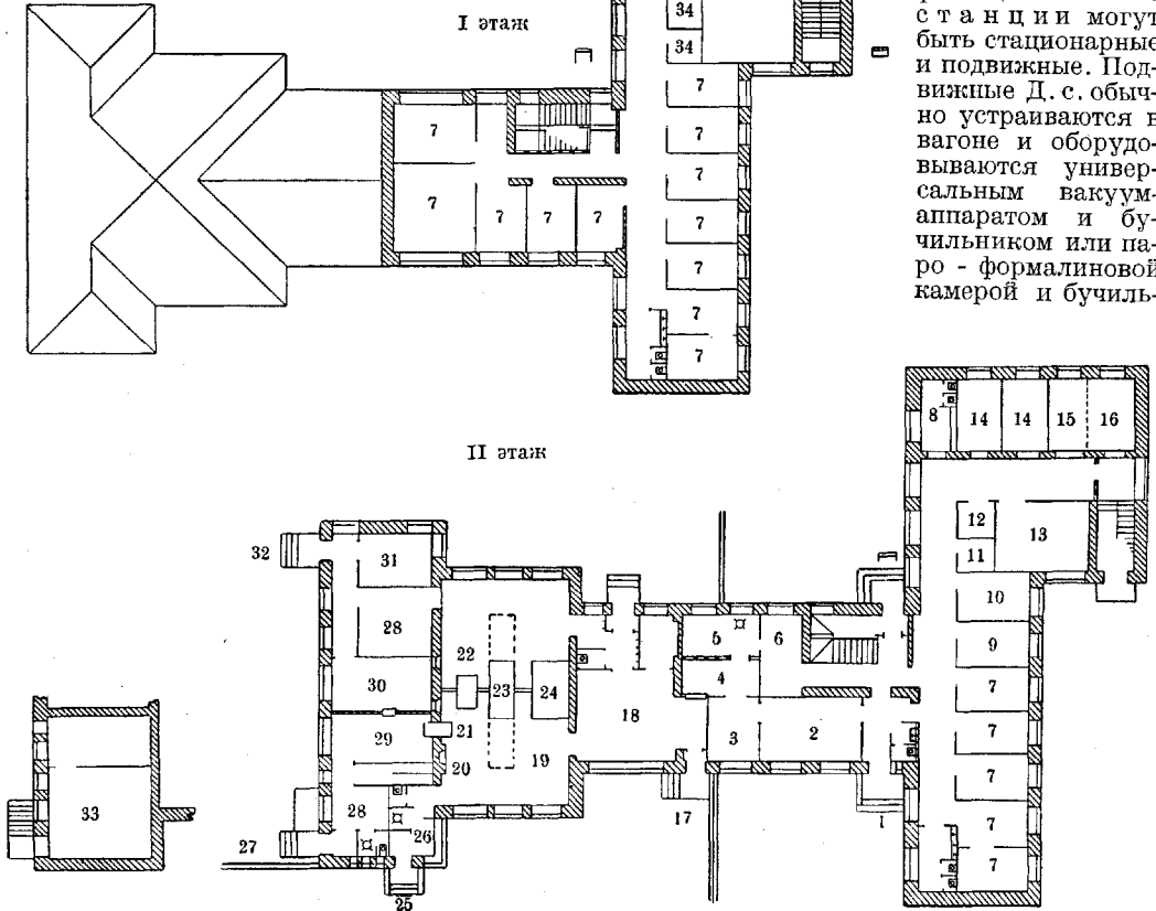
Рис. 2. Проект дезинфекционной станции и изоляционного дома: 1—вход в изолятор; 2—онидальня; 3—комната для осмотра; 4—раздевальня; 5—ванная; 6—одевальня; 7—комнаты для изолируемых; 8—умывальня; 9—вещевой склад; 10—контора; 11—чулан; 12—бельевая; 13—столовая; 14—служебные помещения; 15—буфет; 16—кухня; 17—вход в грязное отделение; 18—разборочная; 19—инфекционное отделение; 20—камин; 21—бучильник; 22—дезинфекционная камера; 23—паровая камера; 24—японская камера; 25—вход в инфекционное отделение камеры; 26—шлюз; 27—вход в прачечную; 28—комната для хранения белья; 29—стиральня; 30—комната заведующего; 31—сторож; 32—служебный вход; 33—котельная; 34—кладовая.
