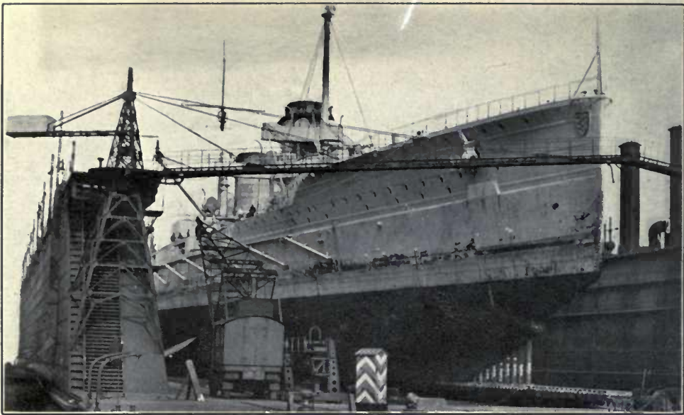
H. M. Ship Seydlitz in Dry-Dock
