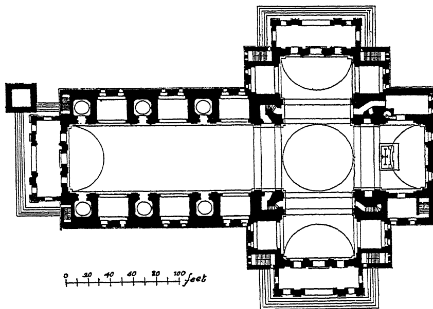
50. LEONE BATTISTA ALBERTI: S. ANDREA, MANTUA, BEGUN 1470.
