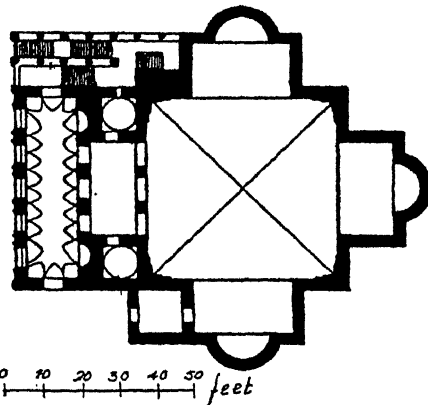
51. LEONE BATTISTA ALBERTI: S. SEBASTIANO, MANTUA, BEGUN 1460.
