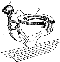
Рис. 5. Консольный клозет: а—чаша; б—сиденье; в—аппарат для промывки прибора.
