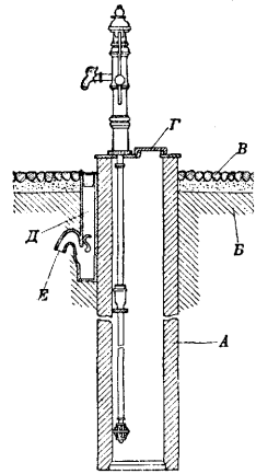
Резервуарный колодец: А—бетонная или каменная на цементной обделка; В—изоляционный слой глины; В—замошение; Г—крышка; Д—сливная шахта; Е—выпуск воды из сливной шахты.
