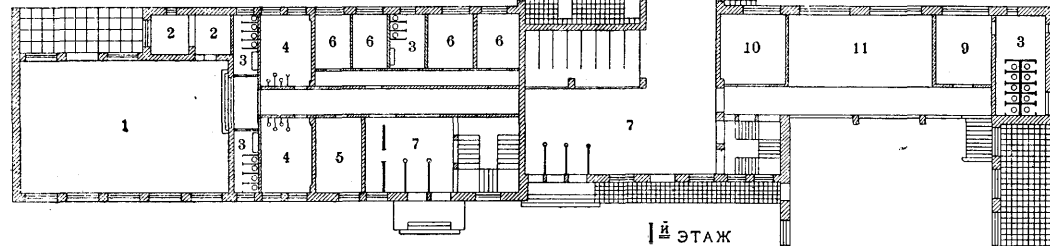
I ЭТАЖ
