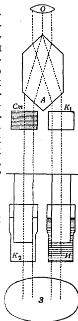
Рис. 3. Схема хода лучей в колориметре Бюркера: О—окуляр; А—тело Гюфнер-Альбрехта; См—сосуд со стандартным раствором; K_1 —сосуд с компенсирующей жидкостью; И—исследуемый раствор; K_2 —компенсирующая жидкость; 3—зеркало.
