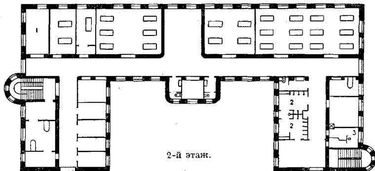
Рис. 27. Павильон на 25 коек—одна инфекция (из проекта вновь строящейся инфекционной больницы в память С. П. Боткина в Ленинграде): 1—перевозочная; 2—пропускные для персонала; 3—пропускная для больных при выписке (душ).
