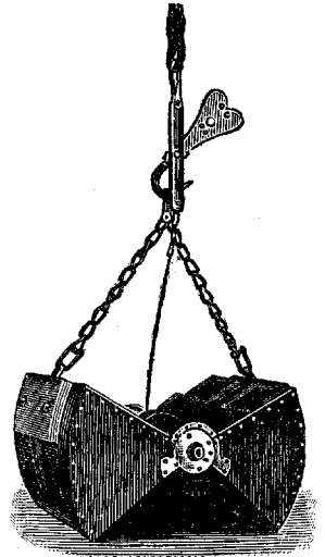
Рис. 10. Дночерпатель Петерсена на площадь захвата \frac{1}{10} кв. м поверхности дна, в открытом положении ( \frac{1}{10} натур. величины).
