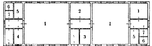
Рис. 5. Схематический план госпитального барака (постоянного): 1—палаты; 2—церевизионная; 3—дежурная; 4—буфетная; 5—ванная; 6—уборная; 7—умывальня.
