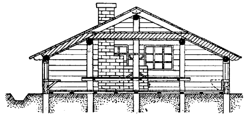
Рис. 6. Зимний досчатый стойчатый барак (в разрезе).
