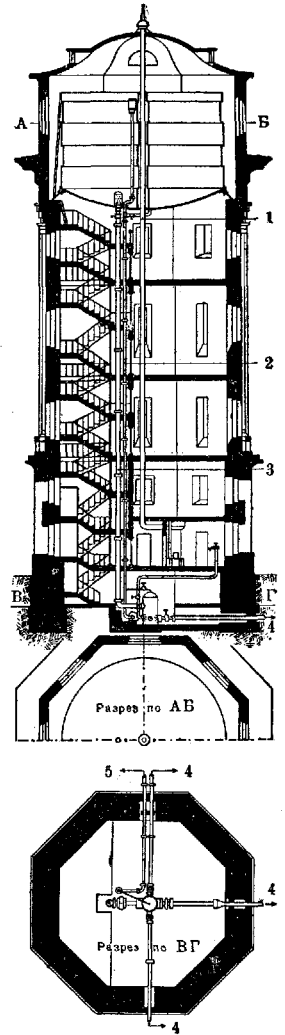
Рис. 2. Башня водонапорная (высота—25 м, объем бака—500 куб. м): 1—дымовая труба; 2—сливная труба; 3—разводящая и питательная труба; 4—в сеть; 5—в канализацию.
