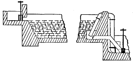
Рис. 2. Схема пластинчат. окислителя Дибдина.
