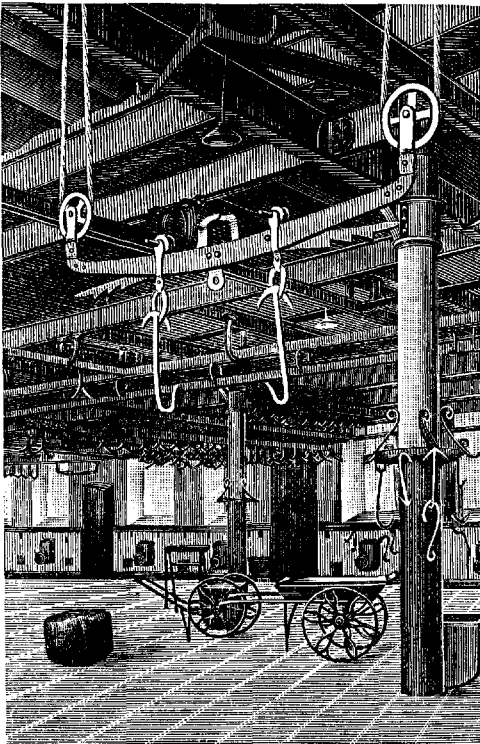
Рис. 4. Разнога лебедня убойного зала для крупного рогатого скота в Ростове-на-Дону.
