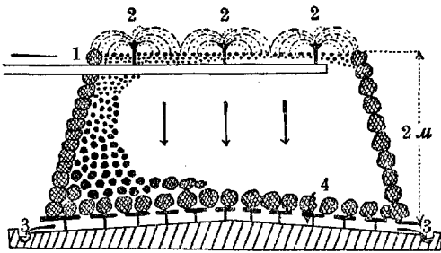
Рис. 3. Схема перколятора: 1—подача воды, осветленной в отстойнике; 2—разбрызгиватели (сифон периодич. действия не показан); 3—жюлоб для очищенной воды; 4—пространство под вторым дном.
