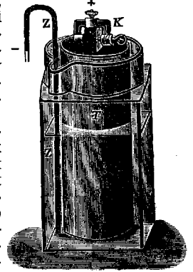
Рис. 1. Первоначальная форма элемента Лекланше: Z—цинковый электрод; T—пористый сосуд, наполненный деполяризующей смесью; K—угольный электрод.
