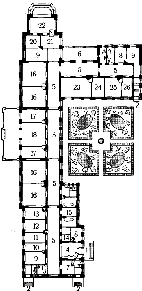
Рис. 6. План сельской б-цы на 25 коек: 1—парадный ход; 2—служебный ход; 3—раздевальня; 4—вестибюль; 5—коридоры; 6—веранда; 7—буфет; 8—смотровые; 9—изолятор; 10—хозяйственная кладовая; 11—лаборатория; 12—кабинет врача; 13—комната дежурного мед. персонала; 14—грязное белье; 15—бельевая; 16—палаты на 4 койки; 17—палаты на 2 койки; 18—столовая, она же и комната для дневного пребывания; 19—перевязочная; 20—стерилизационная; 21—предоперационная; 22—операционная; 23—палата на 5 коек; 24—детская; 25—родовая; 26—предродовая.
