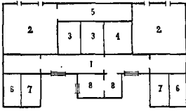
Рис. 12. План заразного барака сельской больницы в Швейцарии: 1—коридор; 2 и 3—палаты; 4—комната сиделки; 5—веранда; 6—уборная; 7—ванная; 8—помещение для приготовления пищи.
