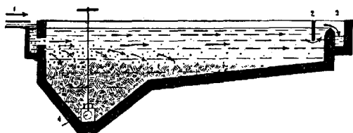
Рис. 3. Схема отстойника с горизонтальным течением: 1—впуск жидкости; 2—полуогруженная перегородка; 3—выпуск осветленной воды; 4—выпуск осадка.
