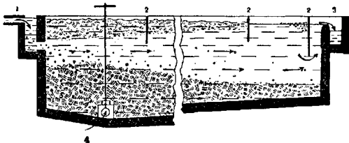
Рис. 4. Схема септик-тэнка: 1—впуск жидкости; 2—полуогруженные перегородки; 3—выпуск осветленной воды; 4—выпуск осадка. На поверхности всплывает осадок, на дне—гниющий осадок.
