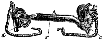
Рис. 1. Ртутно-кварцевая горелка: а—полусные сосуды; б—световая трубка.
