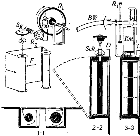
Рис. 6. Схема кимоциклографа и разрезы его (1-1—поперечный разрез, 2-2 и 3-3—продольные разрезы). F—светочувствительная пленка; Sg—передача движения к пленке; R 1 , R 2 —колесики, при соприкосновении которых пленка приходит в движение; Em—электромагнит, прижимающий колесо R 1 к R 2 ; BW—гибкий вал, соединяющий прибор с мотором; Sch—кнопка, D—задвижка аппарата. Весь прибор вставляется в обычный фотоаппарат на место кассеты.
