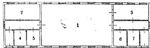
Рис. 3. Схематический план военного барака: 1—рогное помещение; 2—класс; 3—Ленинский уголок; 4—цейхауз; 5 и 6—умывальня; 7—канцелярия.
