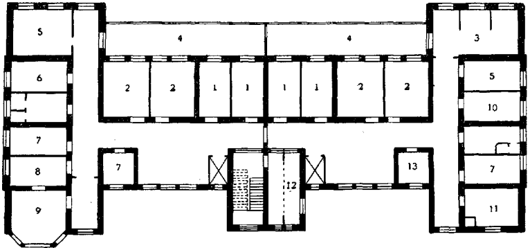
Рис. 22. Пляц второго этажа главн. здания инфенц. Б. в Дюссельдорфе: 1—палаты на 2 кровати; 2—палаты на 4 кровати; 3—палаты на 6 кроватей; 4—веранда; 5—комнаты сестер; 6—служебная комната; 7—ван-ные; 8—предоперационная; 9—операционная; 10—грязное белье; 11—буфет; 12—комната для посетителей; 13—комната для детей со стенозом.
