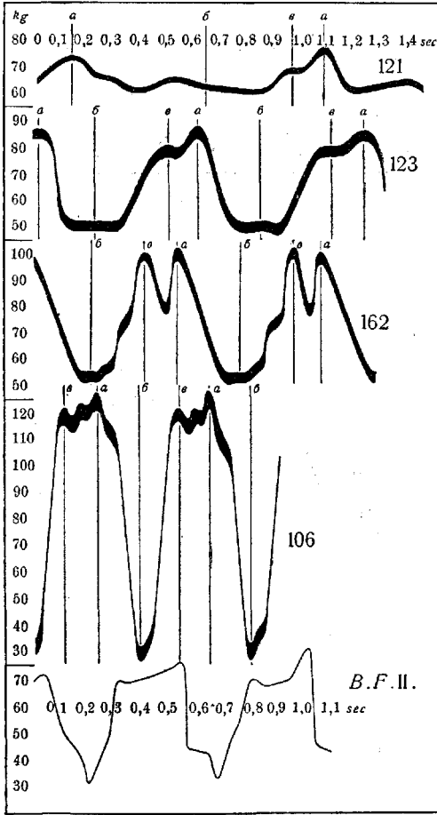
Рис. 3. Кривые опорных реакций при ходьбе. Вертикальное давление ног на путевую поверхность. 121—медленный шаг, 123, 162 и В.Ф.И.—средний, 106—быстрый шаг. Абсциссы—время в десятых долях секунды, ординаты—давление в килограммах. Ординаты а, б, в соответствуют фазам ходьбы по рис. 2.
