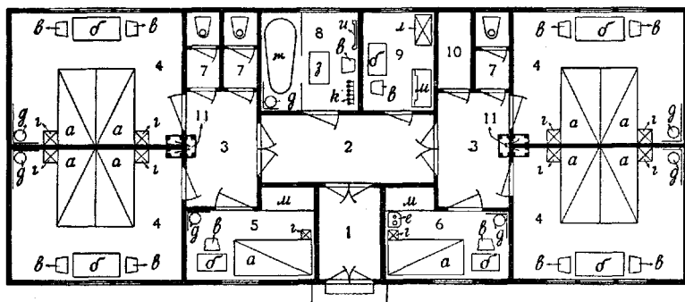
Рис. 2. План Деревянного заразного барака: 1—вход; 2—коридор; 3—тамбуры; 4—палаты на две кровати; 5—палата на одну кровать; 6—дежурная; 7—кладовая; 8—ванная комната; 9—буфетная; 10—инвентарная; 11—вентиляционные каналы. а—кровать; б—стол; в—стул; г—ночная стол; д—печь; е—умывальник; ж—ванна; з—мат; и—зеркало; к—вешалка для платья; л—плитка; м—шкаф.
