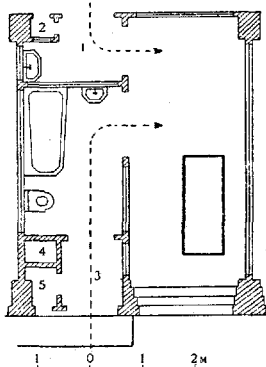
Рис. 24. Изолятор (по сист. пняж. Э. Мельдера, чертёж из проекта инф. больницы в Ленинграде): 1—шлюз для персонала; 2—подача пищи; 3—сени; 4—вентил. кап.; 5—грязное бельё и посуда.
