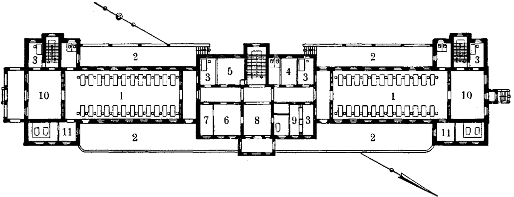
Рис. 9. Отдельный павильон для терапевтических больных городской больницы св. Георга в Лейпциге: 1—палаты-залы для больных; 2—открытые (с.-в.) и крытые (ю.-в.) террасы; 3—однокоечные палаты; 4—дежурные комнаты; 5—мойна; 6—перевязочная; 7—лаборатория; 8—проход на террасы; 9—бельея; 10—дневное пребывание; 11—умывальные.
