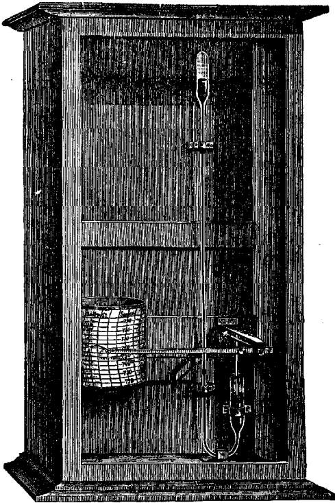
Рис. 1. Ртутный барограф.
