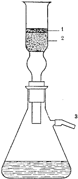
Прибор для определения сахара по Бертрану: 1—асбест; 2—стеклянная вата; 3—к насосу.
