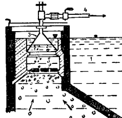
Рис. 7. Деталь устройства для улавливания газа: 1—отстойный лоток; 2—деревянная решетка; 3—железный конус; 4—газовый отвод.
