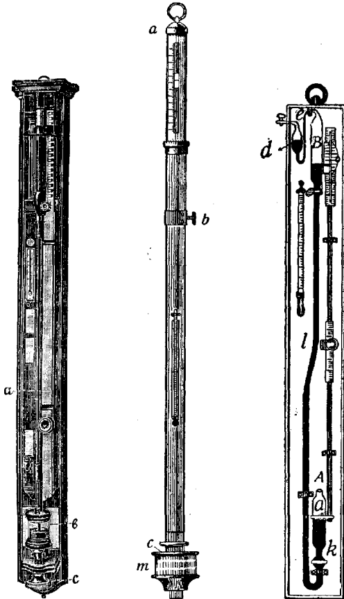
Рис. 1. Ртутный чашечный барометр Фортена. Рис. 2. Ртутный чашечный барометр Тонелло: а—кольцо для подвешивания; б—кремальера для передвижения кольца с нониусом; с—винт, разведирующий чашку с наружным воздухом; т—чашка. Рис. 3. Ртутный сифонный барометр Краевича: А—короткое колено; к—кран, разведирующий короткое колено (барометрической трубки) от длинного; В—барометрическая камера; d—маленькая камера, наполненная ртутью; e—верхний кран; l—длинное колено; против l (справа)—кремальера, передвижающая трубки шкалы; над l слева—термометр.
