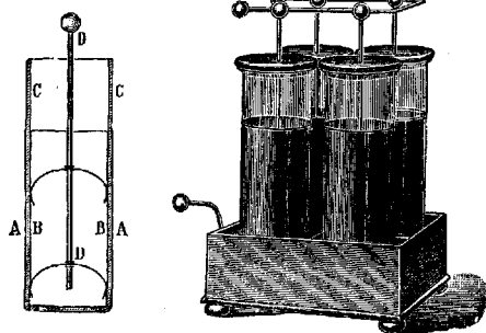
Рис. 4. Батарея лейденских банок: А и В—внешняя и внутренняя обкладки из станиоля; С—стеклянные стенки; D—электрод, сообщающийся с внутренней обкладкой.
