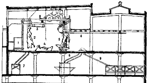
Рис. 2. Разрез скотобойни американского типа (для крупного рогатого скота): 1—бухта (вагон) для оглушения животных; 2—животное подвешено для лучшего обескровливания при разрезе; 3—рельс обескровливания; 4—туша в начале разделки уложена на пол бойни; 5—туша освобождается от внутренностей; 6—рельс у потолка в холодильник; 7—желоб для спуска крови; 8—желоб для спуска желудков и кишков; 9—желоб для спуска кож; 10—система моторных фрикционных лебедок.
