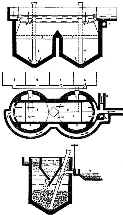
Рис. 5. Схематический план Эмшерского бассейна: 1—впуск жидкости в отстойный лоток; 2—продольная щель на дне лотка; 3—«газовые отдушины» (здесь собирается «корна»); 4—иловые трубы; 5—сушильные площадки; 6—выпуск осветленной воды. Расположение подводных и отводящих каналов допускает пустить жидкость в обратном направлении.
