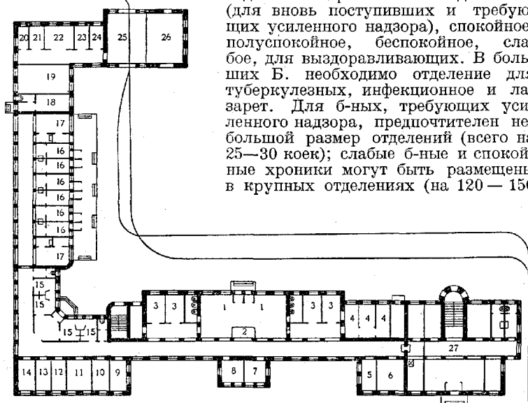
Рис. 25. Приемный покой (из проекта вновь строящейся инфекционной больницы в память С. П. Боткина в Ленинграде): 1—ошица общего приемного покоя; 2—регистрация; 3—осмотр больных; 4—проезничная для больных; 5—комната младшего персонала; 6—врач; 7—перевязочная; 8—средний персонал; 9—врач; 10—средний персонал; 11—младший персонал; 12—уборщица; 13—кипяильник; 14—бельевая; 15—пропускная для персонала муж. и жен.; 16 и 17—индивидуальные смотровые (для так наз. летучих инфекций); 18—комната узельщица; 19—узельная (суточная); 20—уборная; 21—кладовая; 22—комната дезинфектора; 23 и 24—комнаты санит. транспорта (перевоз.); 25—дезинфекция автомобилей; 26—хранение тележек для развозки больных; 27—нижний этаж конторы.
