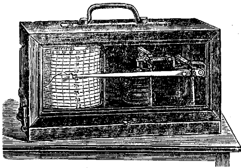
Рис. 2. Барограф-анероид.
