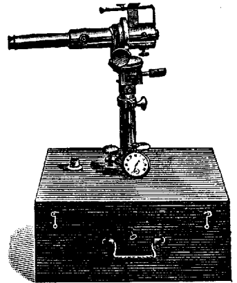
Рис. 3. Актинометр Михельсона.
