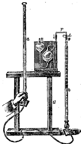
Рис. 4. Бюретка Гемпеля для измерения объема газа. Поднятием бюретки a переводят исследуемый газ при открытом запянке d в пипетку Гемпеля c , наполненную поглотителем одной из составных частей газа.
