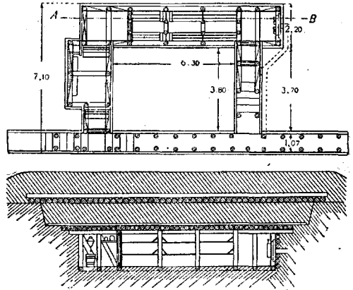
Рис. 8. Вентиляционное убежище котлованного типа.
