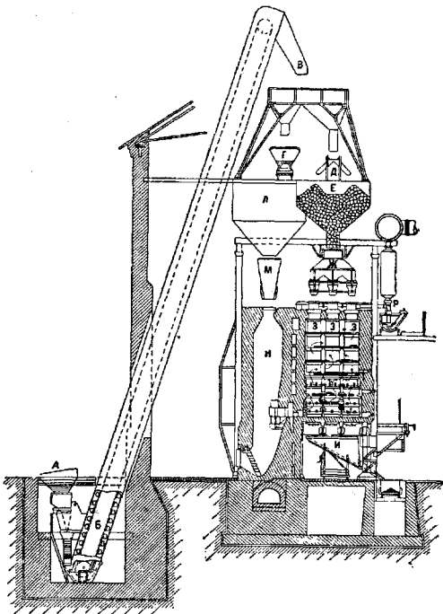
Рис. 1. Разрез газовой печи с вертикальными ретортами: А—присыпная воронка элеватора; Б—ковши, поднимающие уголь наверх здания ретортного отделения; В—верхнее отверстие элеватора; Г—тележка,двигающаяся вдоль всего ретортного здания; Д—самотаска; Е—закрома; Ж—воронки-вагонетки, устанавливаемые над отверстиями реторт; 333—вертикальные реторты; Н—генератор; Л—консольные закрома; М—воронка для загрузки коксом генератора; И—тележка, на к-рую падает кокс при открывании нижней крышки реторт; Р—гидравлический затвор, через к-рый проходит газ, прежде чем попасть в сборную трубу.
