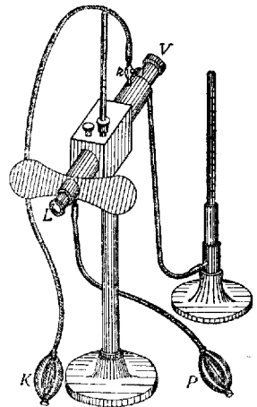
Рис. 5. Конденсационный гигрометр Крова.
