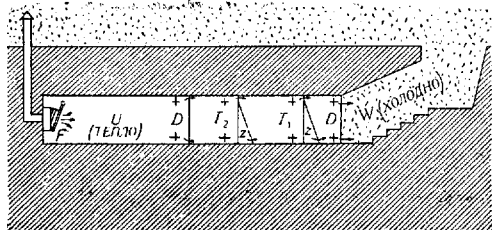
Рис. 4. Схема вентиляционн. убежища: T_1, T_2 —тамбуры; DD —двери; Z, Z —непроницаемые занавеси; F —фильтр; U —убежище.
