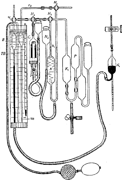
Рис. 7. Аппарат Голдейна.
