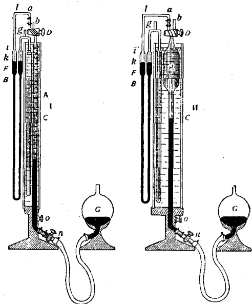
Рис. 5. Термобарометр Гемпеля. Исследуемый газ находится в бюретке A . Слева от нее находится закрытая снизу трубка (термобарометр), сообщающаяся с измерительной бюреткой через ртутный манометр B и кран D . Термобарометр и измерительная трубка находятся в общем сосуде, наполненном водой. Шар G , наполненный ртутью, позволяет устанавливать ртуть в бюретке A на желаемом уровне.
