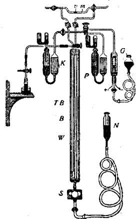
Рис. 6. Аппарат Бор-Тобизена. m — дифференциальный манометр; v — капля вазелинового масла; K и P — сосуды с поглощающими веществами; G — сосуд для сжигания; N — давящий сосуд со ртутью.
