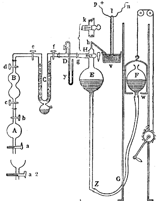
Рис. 1. Схема ртутного насоса для извлечения газов крови (построен на принципе И. М. Сеченова и модифицирован Пфлюгером). Объяснение действия—в тексте.
