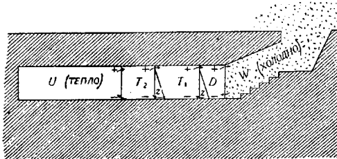
Рис. 3. Схема герметич. убежища: U—убежище; T_1, T_2 —тамбуры; D—двери; Z—непроницаемые занавесы.
