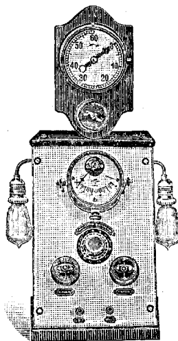
Рис. 2. Распределительный попитра образца Гос. ин-та физиотерапии и ортопедии в Москве.
