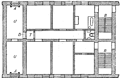
Рис. 9. Противохимическое оборудование квартирного убежища: А,А—заделанные окна; В,В—лестничные клетки входа; Т—тамбур; D—герметическая дверь; U,U—убежища.
