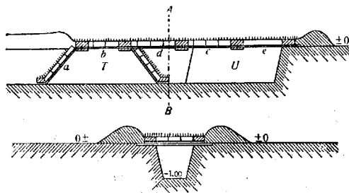
Рис. 6. Щель, оборудованная в противохим. отношении (проект инж. Тимонова): а, б, с, d, e—полотноща походных палаток.
