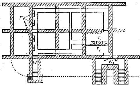
Рис. 10. Противохимическое оборудование подвала: F —фильтры; T 1 , T 2 —тамбуры; W —запасный вход; W 1 —действующий вход.
