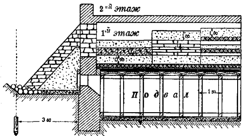
Рис. 1. Типовые перекрытия убежищ для защиты от аэробомб весом до 100 кг.
