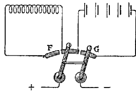
Коммутатор de Wattewille'я для гальвано-фарадического тока.
