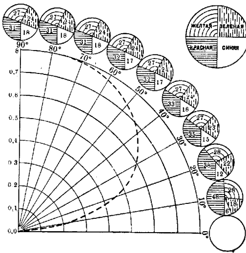
Рис. 1. Распределение энергии отдельных частей спектра при разных высотах солнца.
