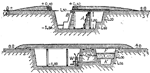
Рис. 7а. Легкое полевое убежище с фильтром из растительной земли на 8—10 человек: А—занавес опущен; В—занавес на полке поднят; С—фильтрующий слой; F—надфильтровая камера, куда поступают О. В.; К—камера очищенного от О. В. воздуха; Т—трубопровод в убежище; W—вентилятор.
