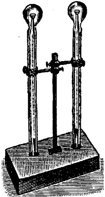
Рис. 2. Актинометр Араго-Девя-Калитяна.
