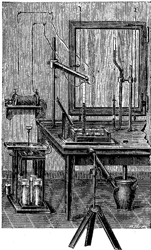
Рис. 2. Эвдиометр Бунзена. В центре рис. видны эвдиометрическая трубка и ванна со ртутью. Слева—катушка Румшорфа, дающая искру, зажигающую газ. На переднем плане—труба, с помощью к-рой производится отсчет делений.
